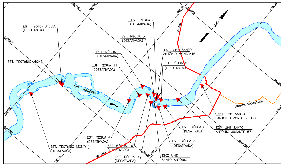
DETALHE-1 ESC:1:125.000
