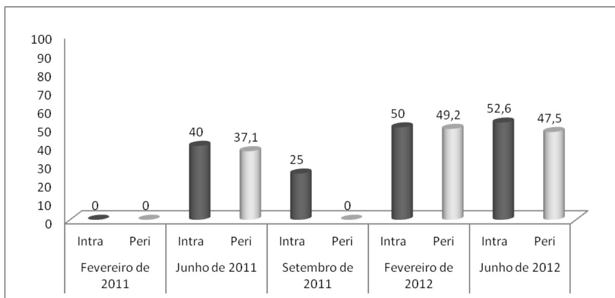
Figura 58. Paridade de An. darlingi na Vila Franciscana em cinco campanhas de campo, nas áreas de influência da UHE Santo Antônio, Porto Velho – RO.
