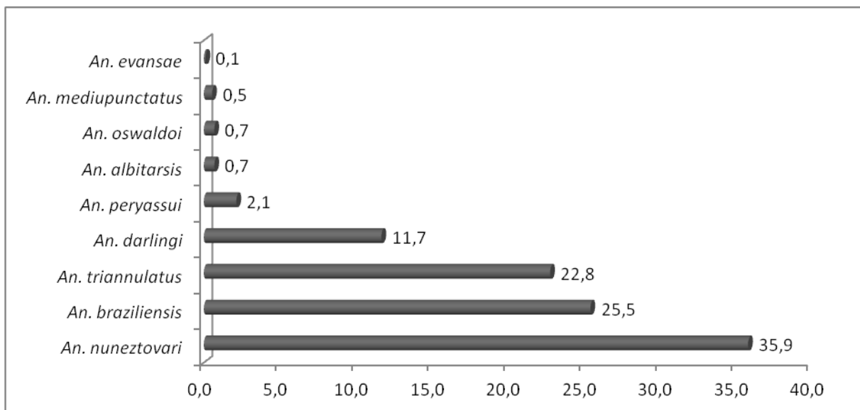
Figura 64. Percentual de larvas de Anopheles coletadas em cinco de campo nas áreas de influência da UHE Santo Antônio, Porto Velho – RO.
