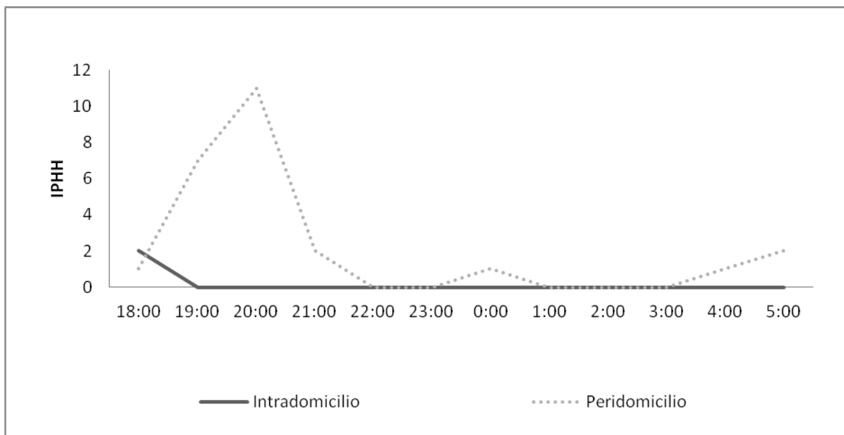
Figura 37. IPHH (índice de picada homem/hora) de Anopheles darlingi capturados no Intra e Peridomicílio, nas áreas de influência da UHE Santo Antônio, Porto Velho – RO.
