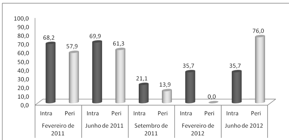
Figura 60. Paridade de An. darlingi na Vila Santo Antônio em cinco campanhas de campo, nas áreas de influência da UHE Santo Antônio, Porto Velho – RO.
