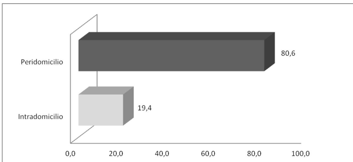
Figura 28. Percentual de Anopheles darlingi capturados no Intra e Peridomicílio, nas áreas de influência da UHE Santo Antônio, Porto Velho - RO.
