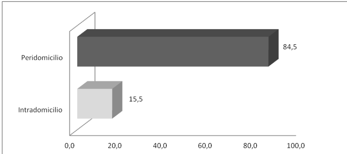
Figura 20. Percentual de Anopheles darlingi capturados no Intra e Peridomicílio nas áreas de influência da UHE Santo Antônio, Porto Velho - RO.
