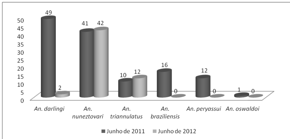
Figura 72. Número de larvas/pupas do gênero Anopheles coletados em pesquisas larvárias na segunda e quinta campanha de campo realizada em junho de 2011 e 2012 nas áreas de influências da UHE Santo Antônio, Porto Velho – RO.
