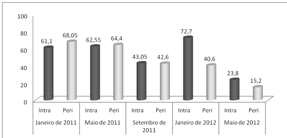
Figura 51. Paridade de An. darlingi na Comunidade ao longo do rio Jaci em cinco campanhas de campo, nas áreas de influência da UHE Santo Antônio, Porto Velho – RO.
