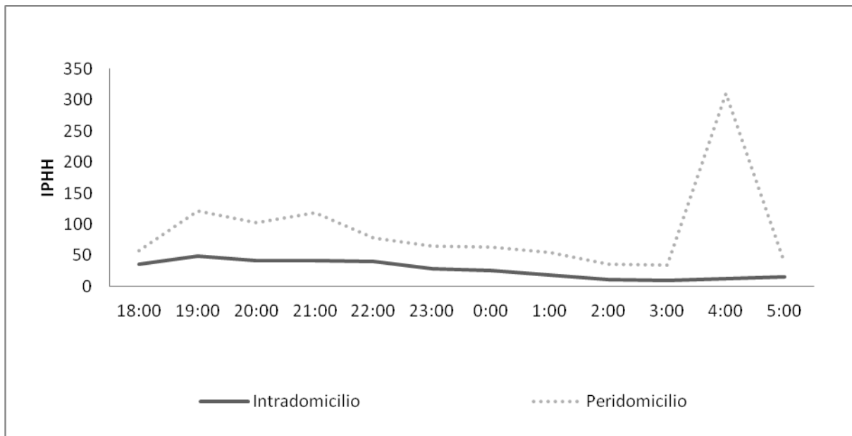
Figura 13. IPHH (índice de picada homem/hora) de Anopheles darlingi capturados no Intra e Peridomicílio, nas áreas de influência da UHE Santo Antônio, Porto Velho – RO.
