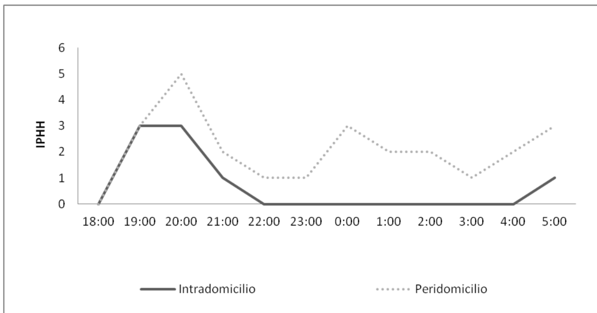
Figura 15. IPHH (índice de picada homem/hora) de Anopheles darlingi capturados no Intra e Peridomicílio, nas áreas de influência da UHE Santo Antônio, Porto Velho – RO.
