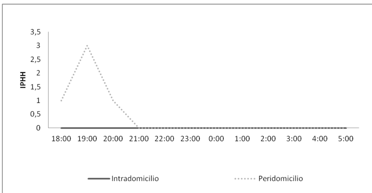
Figura 34. IPHH (índice de picada homem/hora) de Anopheles darlingi capturados no Intra e Peridomicilio, nas áreas de influência da UHE Santo Antônio, Porto Velho - RO.
