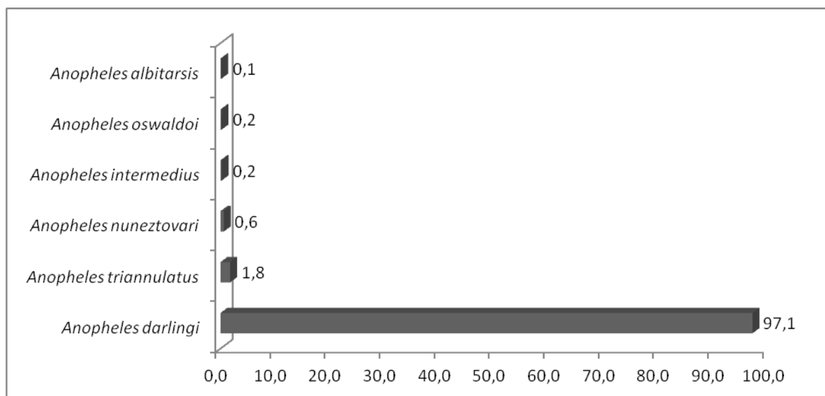
Figura 8. Percentual de espécies coletados em maio e junho de 2012 (quinta campanha), na área do empreendimento e seu entorno, nas áreas de influência da UHE Santo Antônio, Porto Velho - RO.
