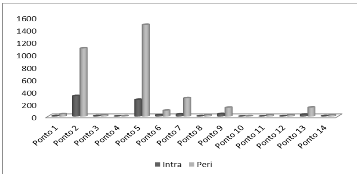
Figura 9. Número de mosquitos adultos do gênero Anopheles coletados em capturas de 12 e 4 h na quinta campanha de campo, realizadas em maio e junho de 2012 nas áreas de influências da UHE Santo Antônio, Porto Velho – RO.
