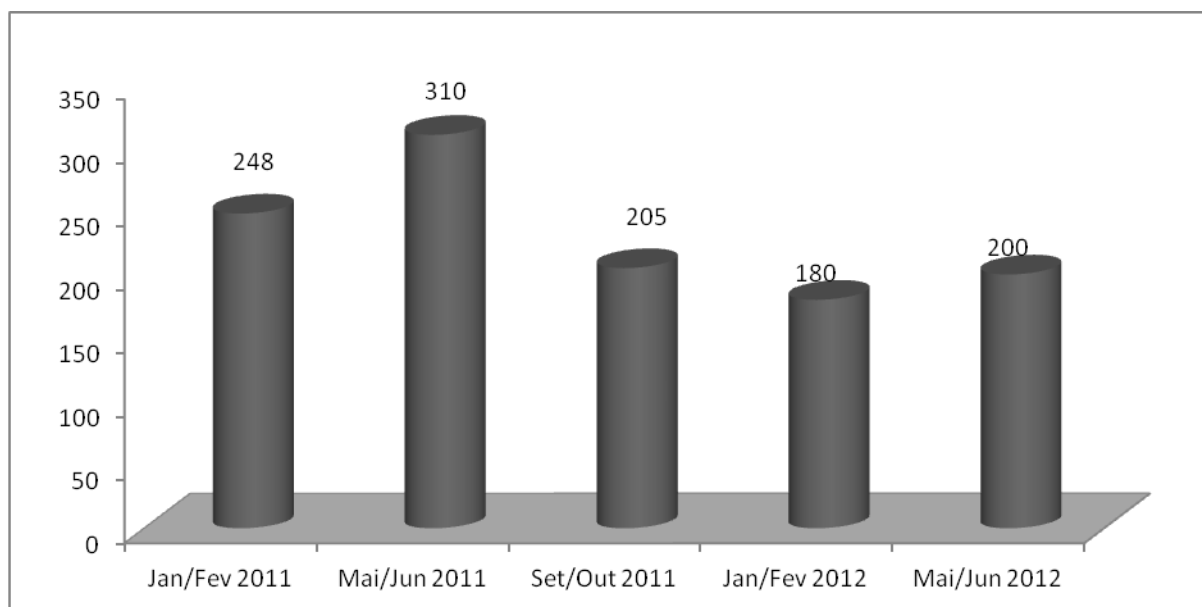
Figura 48. Número de espécimes do gênero Anopheles capturados em armadilhas Shannon em coletas de 4h em dois dias consecutivos nas cinco campanhas de campo, nas áreas de influência da UHE Santo Antônio, Porto Velho – RO.
