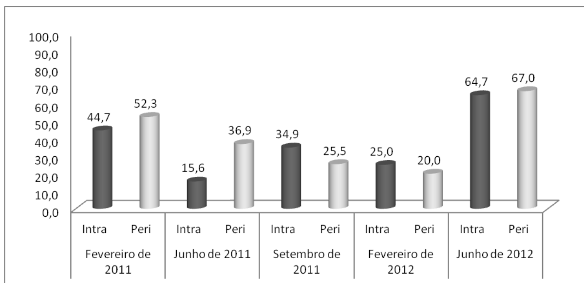
Figura 62. Paridade de An. darlingi no Novo Engenho Velho em cinco campanhas de campo, nas áreas de influência da UHE Santo Antônio, Porto Velho – RO.
