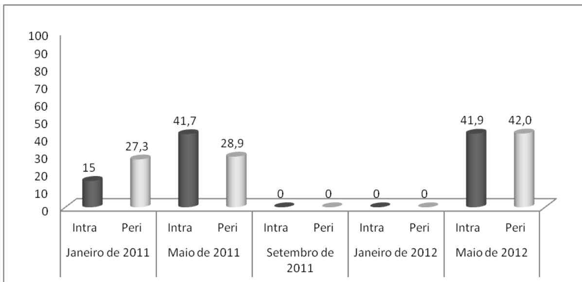
Figura 55. Paridade de An. darlingi na Cachoeira do Macaco (2011) Reassentamento Morrinhos (2012) em cinco campanhas de campo, nas áreas de influência da UHE Santo Antônio, Porto Velho – RO.
