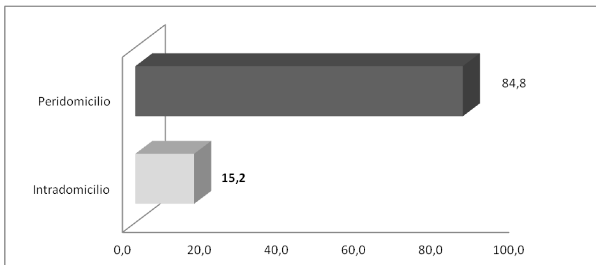
Figura 10. Percentual de Anopheles darlingi capturados no Intra e Peridomicílio, nas áreas de influência da UHE Santo Antônio, Porto Velho – RO.
