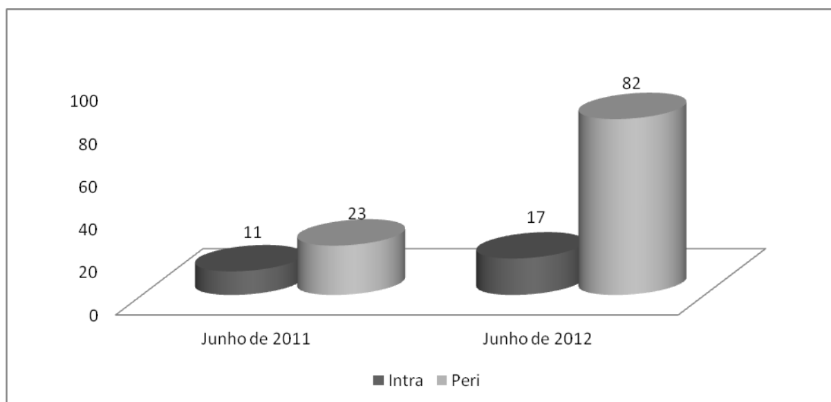
Figura 47. Número de espécimes do gênero Anopheles capturados no Intra e Peridomicílio antes (junho de 2011) e após o enchimento da barragem (junho de 2012), nas áreas de influência da UHE Santo Antônio, Porto Velho – RO.
