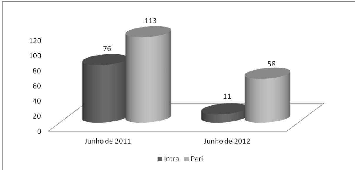
Figura 41. Número de espécimes do gênero Anopheles capturados no Intra e Peridomicílio antes (junho de 2011) e após o enchimento da barragem (junho de 2012), nas áreas de influência da UHE Santo Antônio, Porto Velho – RO.
