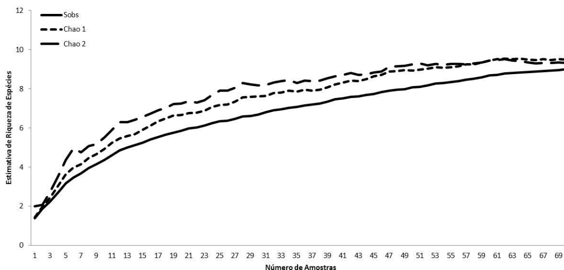
Figura 6. Curva de acumulação das espécies de anofelinos por número de amostras obtidas nos meses de Jan/Fev 2011 (1ª campanha), mai/jun /2011 (2ª campanha), Set/Out 2011 (3ª campanha), Jan/Fev2012(4ª campanha) e mai/jun /2012 (5ª campanha), nas áreas diretamente afetadas e de influência do projeto UHE Santo Antônio Energia, RO.
