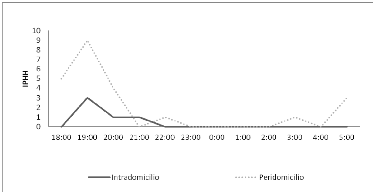
Figura 40. IPHH (índice de picada homem/hora) de Anopheles darlingi capturados no Intra e Peridomicilio, nas áreas de influência da UHE Santo Antônio, Porto Velho – RO.
