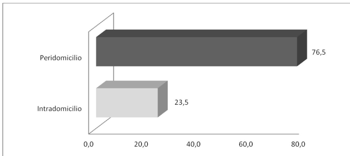
Figura 12. Percentual de Anopheles darlingi capturados no Intra e Peridomicílio, nas áreas de influência da UHE Santo Antônio, Porto Velho - RO.
