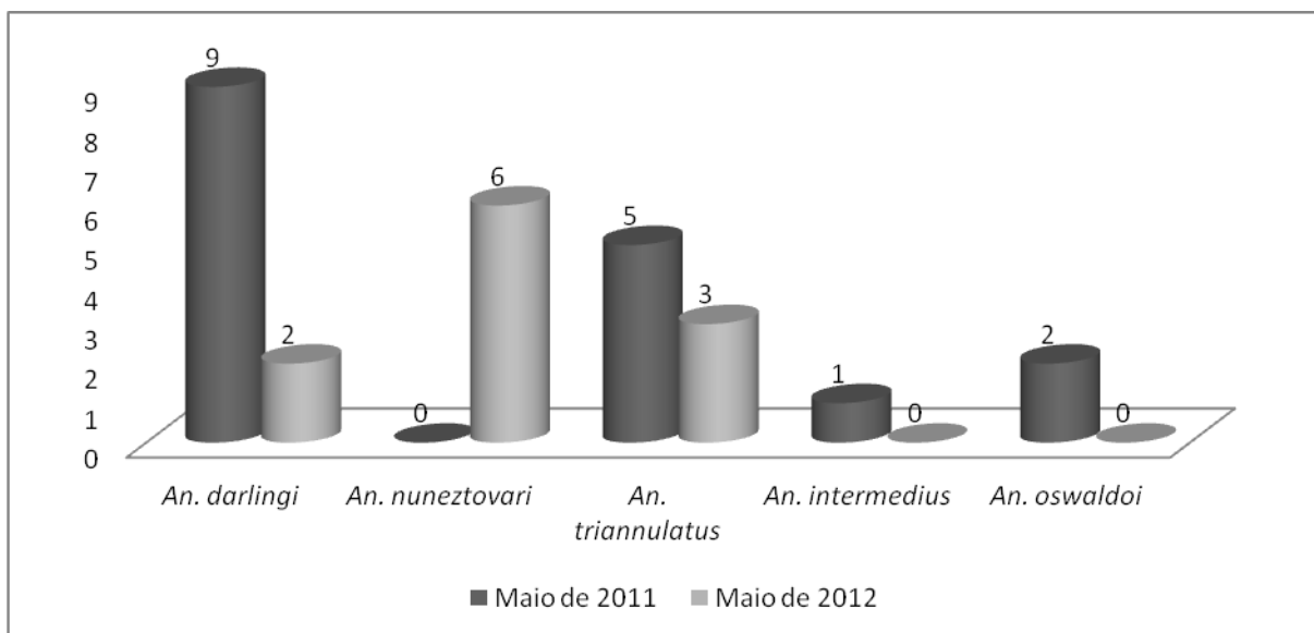
Figura 66. Número de larvas/pupas do gênero Anopheles coletados em pesquisas larvárias na segunda e quinta campanha de campo realizada em maio de 2012 nas áreas de influências da UHE Santo Antônio, Porto Velho – RO.
