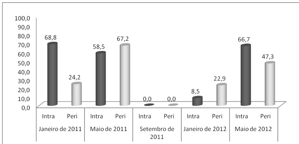
Figura 57. Paridade de An. darlingi na Cachoeira do Teotônio (2011) Vila Nova Teotônio (2012) em cinco campanhas de campo, nas áreas de influência da UHE Santo Antônio, Porto Velho – RO.
