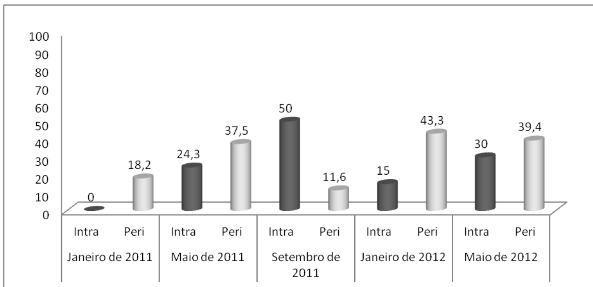
Figura 53. Paridade de An. darlingi Bairro Alto Alegre (Jaci Paraná) em cinco campanhas de campo, nas áreas de influência da UHE Santo Antônio, Porto Velho – RO.
