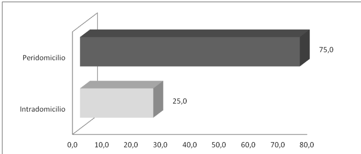
Figura 17. Percentual de Anopheles darlingi capturados no Intra e Peridomicilio, nas áreas de influência da UHE Santo Antônio, Porto Velho - RO.
