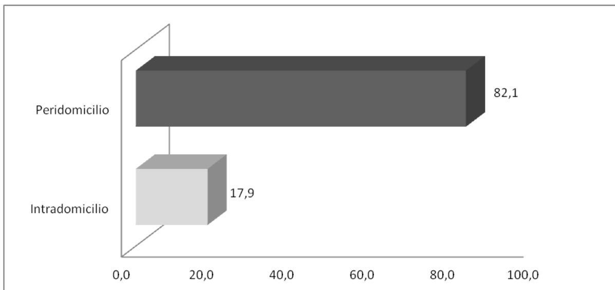
Figura 39. Percentual de Anopheles darlingi capturados no Intra e Peridomicilio, nas áreas de influência da UHE Santo Antônio, Porto Velho - RO.
