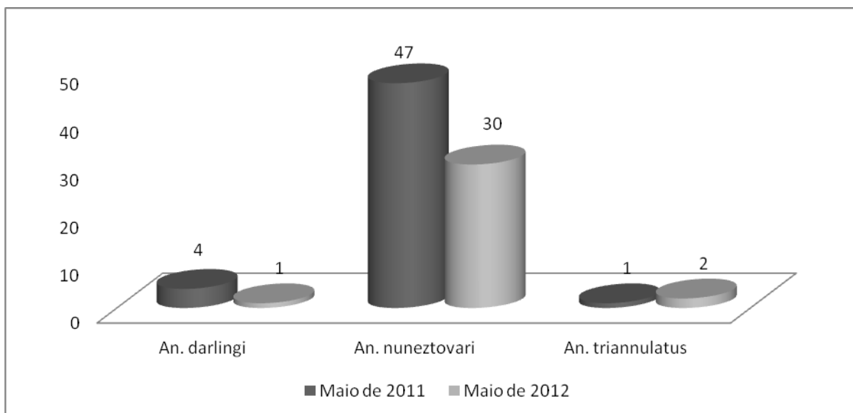
Figura 68. Número de larvas/pupas do gênero Anopheles coletados em pesquisas larvárias na segunda e quinta campanha de campo realizada em maio de 2011 e 2012 nas áreas de influências da UHE Santo Antônio, Porto Velho – RO.
