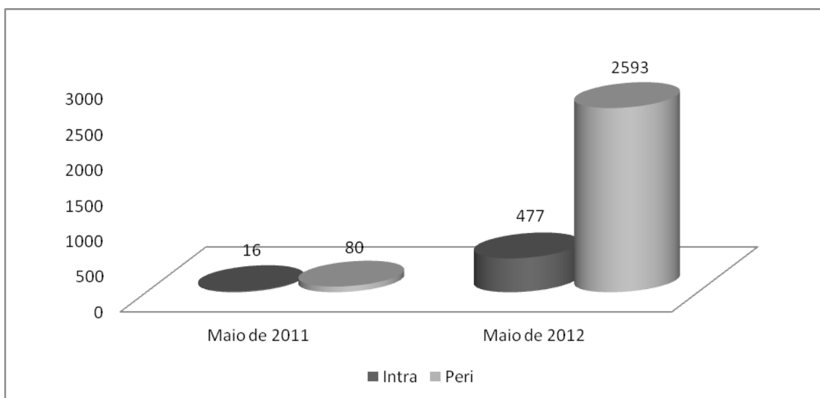
Figura 22. Número de espécimes do gênero Anopheles capturados no Intra e Peridomicílio antes (maio de 2011) e após o enchimento da barragem (maio de 2012), nas áreas de influência da UHE Santo Antônio, Porto Velho – RO.
