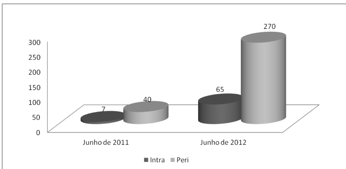
Figura 32. Número de espécimes do gênero Anopheles capturados no Intra e Peridomicílio antes (junho de 2011) e após o enchimento da barragem (junho de 2012), nas áreas de influência da UHE Santo Antônio, Porto Velho – RO.
