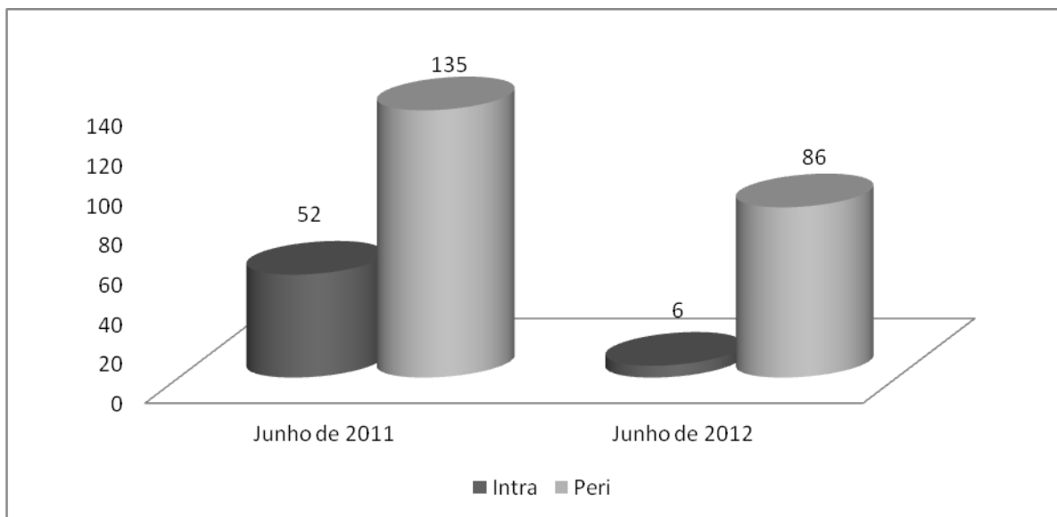
Figura 35. Número de espécimes do gênero Anopheles capturados no Intra e Peridomicílio antes (junho de 2011) e após o enchimento da barragem (junho de 2012), nas áreas de influência da UHE Santo Antônio, Porto Velho – RO.
