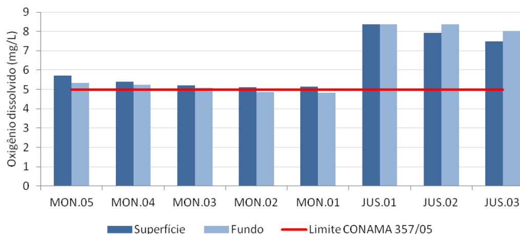
Figura 2-16 - Concentrações de oxigênio dissolvido nos rio Madeira em março de 2012 (águas altas).
