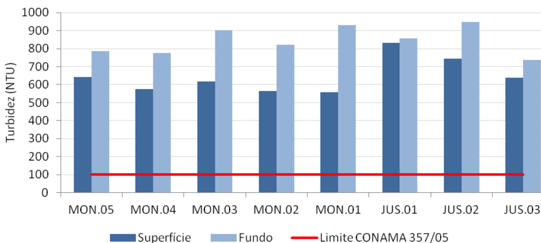
Figura 2-8 - Valores de turbidez no rio Madeira em março de 2012 (águas altas).
