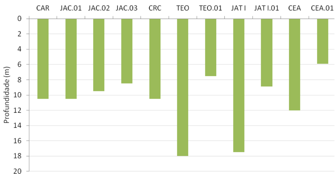
Figura 2-2 - Profundidade da coluna d'água nos tributários em março de 2012 (águas altas).
