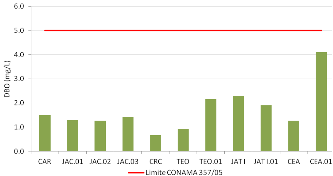
Figura 2-21 - Demanda bioquímica de oxigênio (DBO 5 ) nos tributários em março de 2012 (águas altas).
