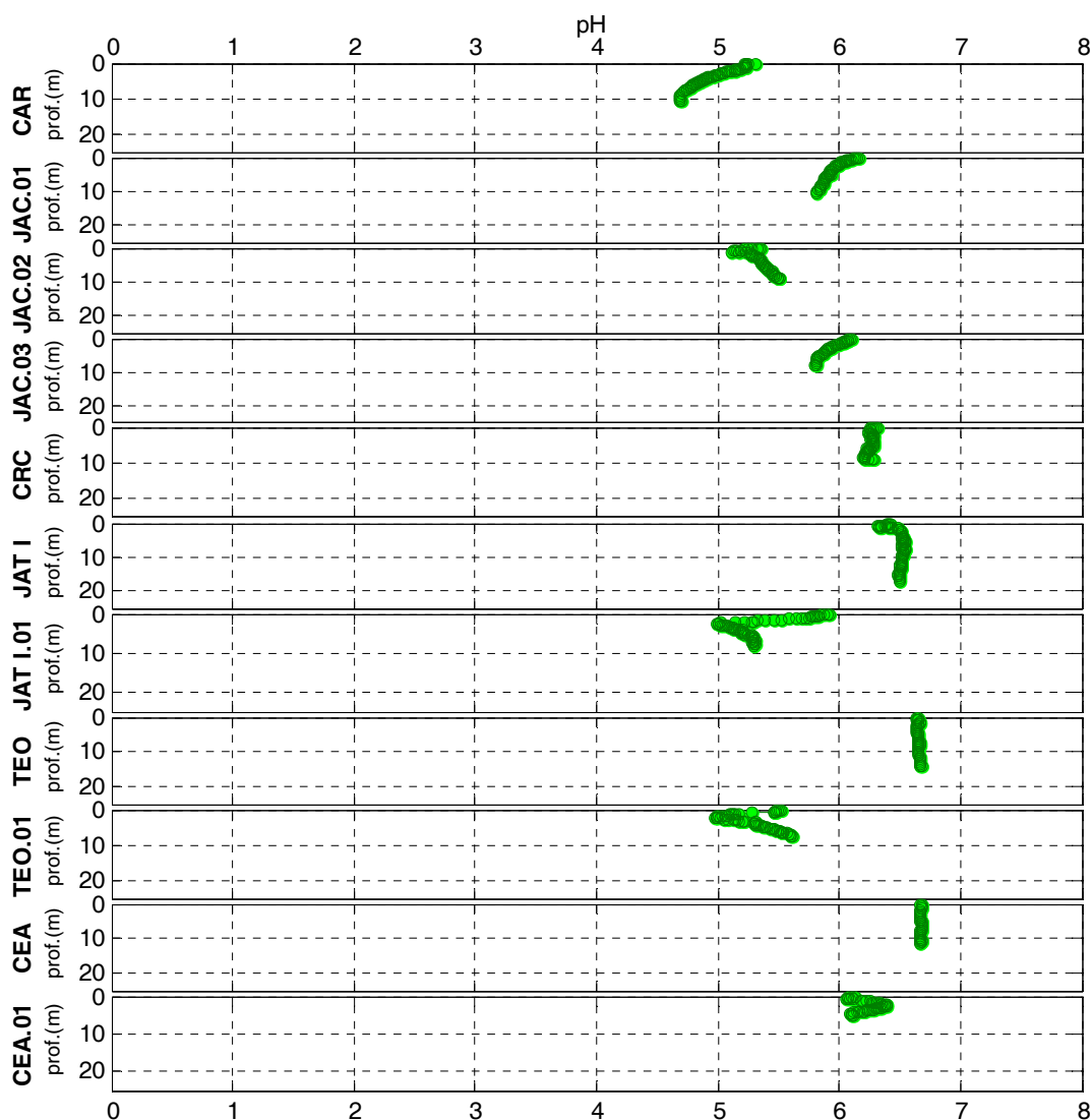
Figura 2-15 - Perfis de pH nos tributários em março de 2012 (águas altas).
