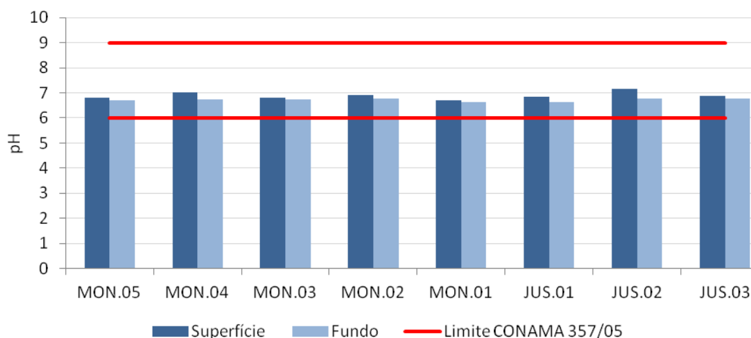
Figura 2-12 - Valores de pH no rio Madeira em março de 2012 (águas altas).
