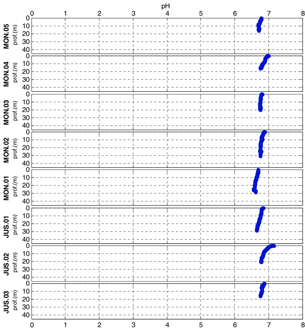
Figura 2-13 - Perfis de pH nos rio Madeira em março de 2012 (águas altas).
