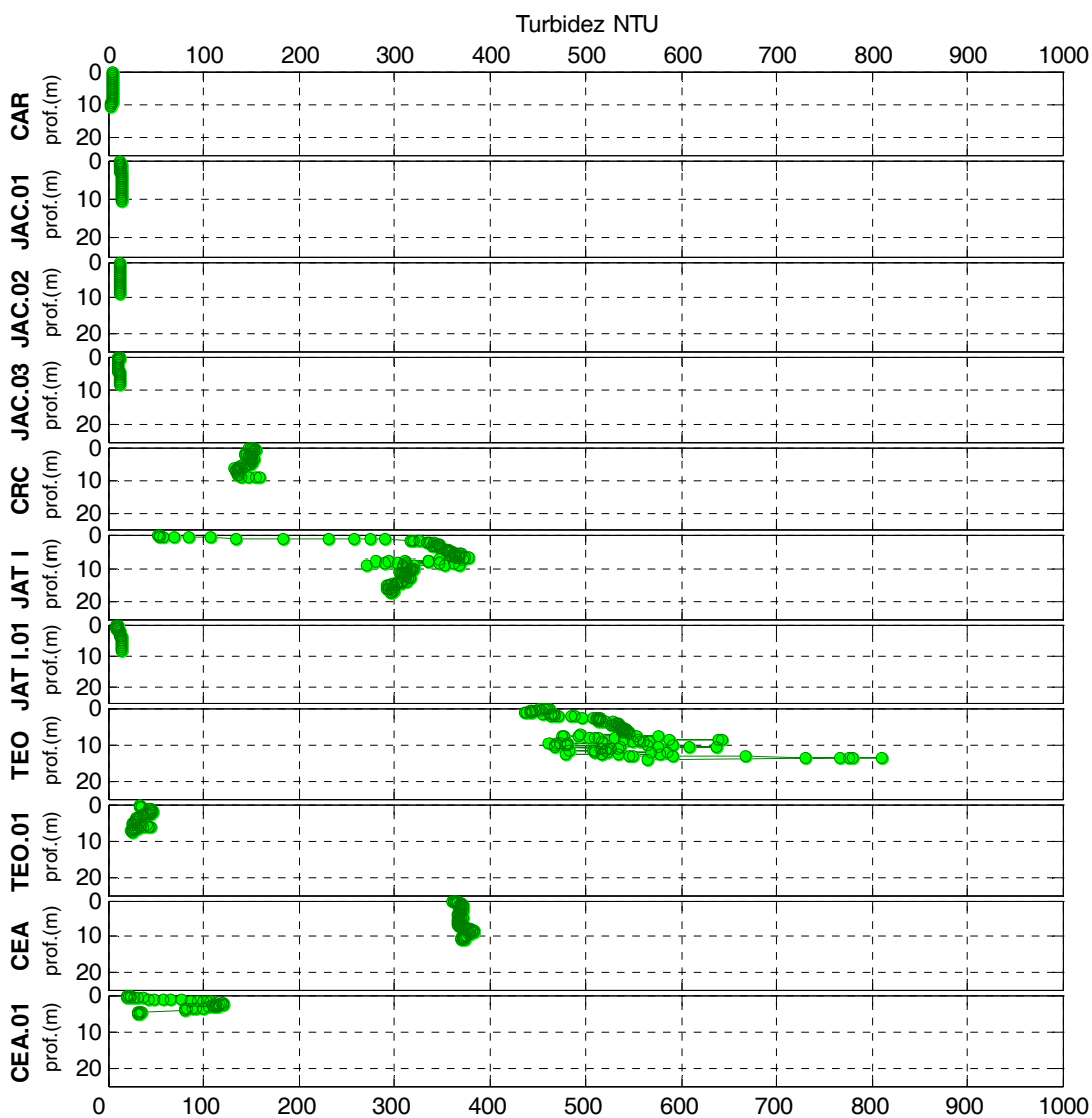
Figura 2-11 - Perfis de turbidez nos tributários em março de 2012 (águas altas).
