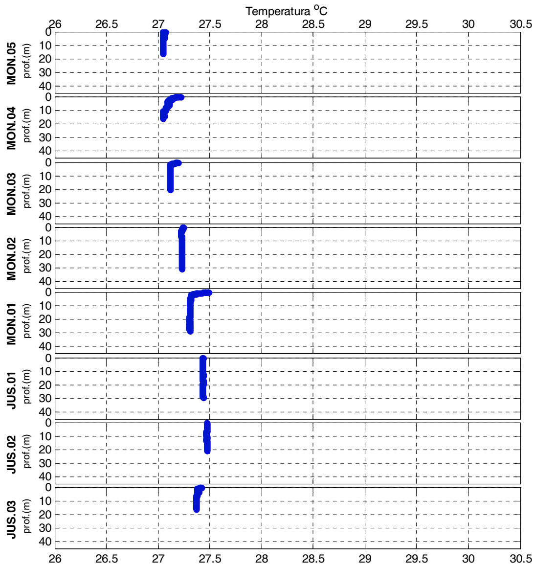
Figura 2-5 - Perfis de temperatura no rio Madeira em março de 2012 (águas altas).
