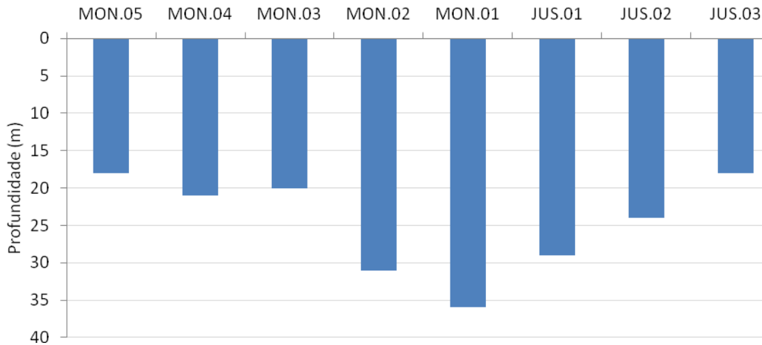
Figura 2-1 - Profundidade da coluna d'água no rio Madeira em março de 2012 (águas altas).
