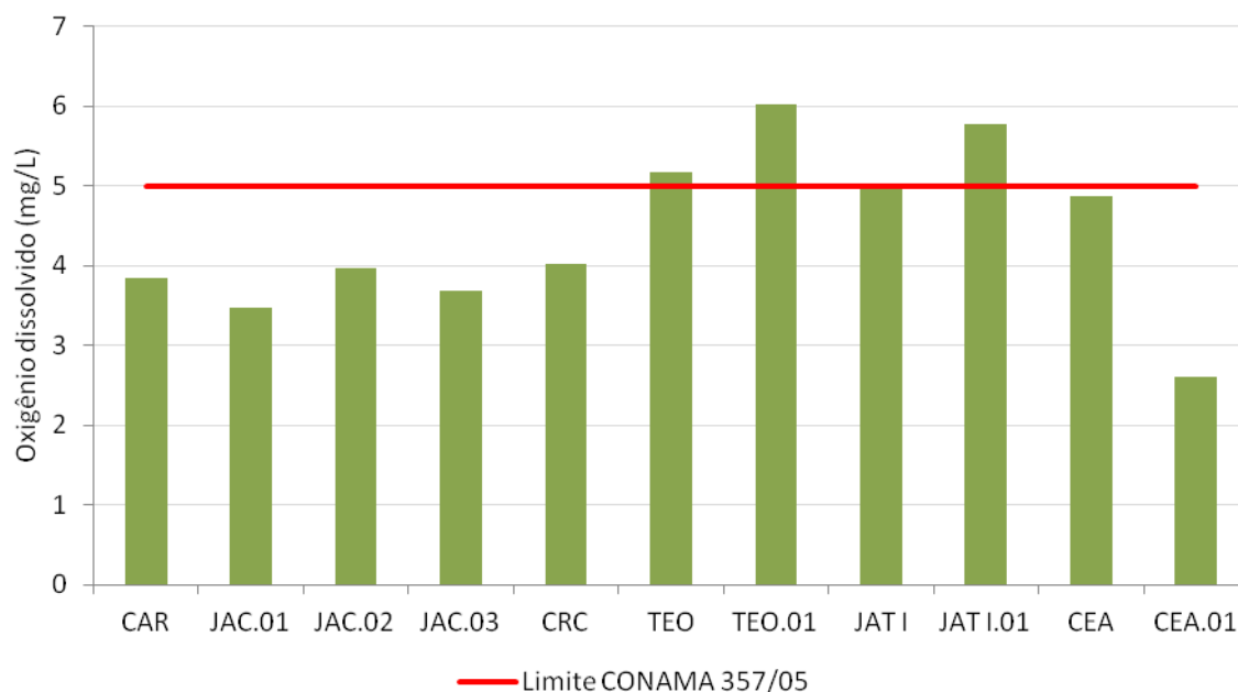
Figura 2-18 - Concentrações de oxigênio dissolvido nos tributários em março de 2012 (águas altas).
