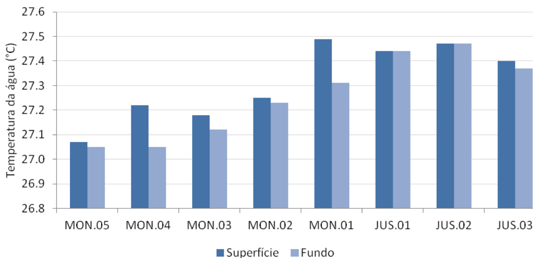
Figura 2-4 - Temperatura da água no rio Madeira em março de 2012 (águas altas).
