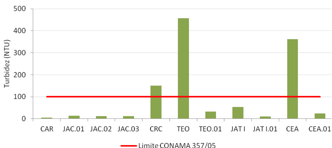
Figura 2-10 - Valores de turbidez nos tributários em março de 2012 (águas altas).
