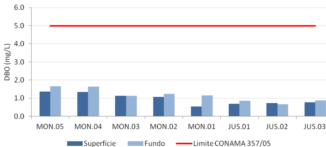
Figura 2-20 - Demanda bioquímica de oxigênio (DBO) nos rio Madeira em março de 2012 (águas altas).
