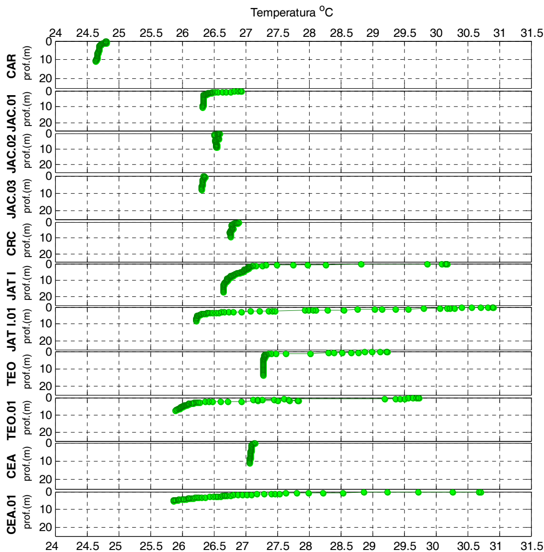
Figura 2-7 - Perfis de temperatura nos tributários em março de 2012 (águas altas).
