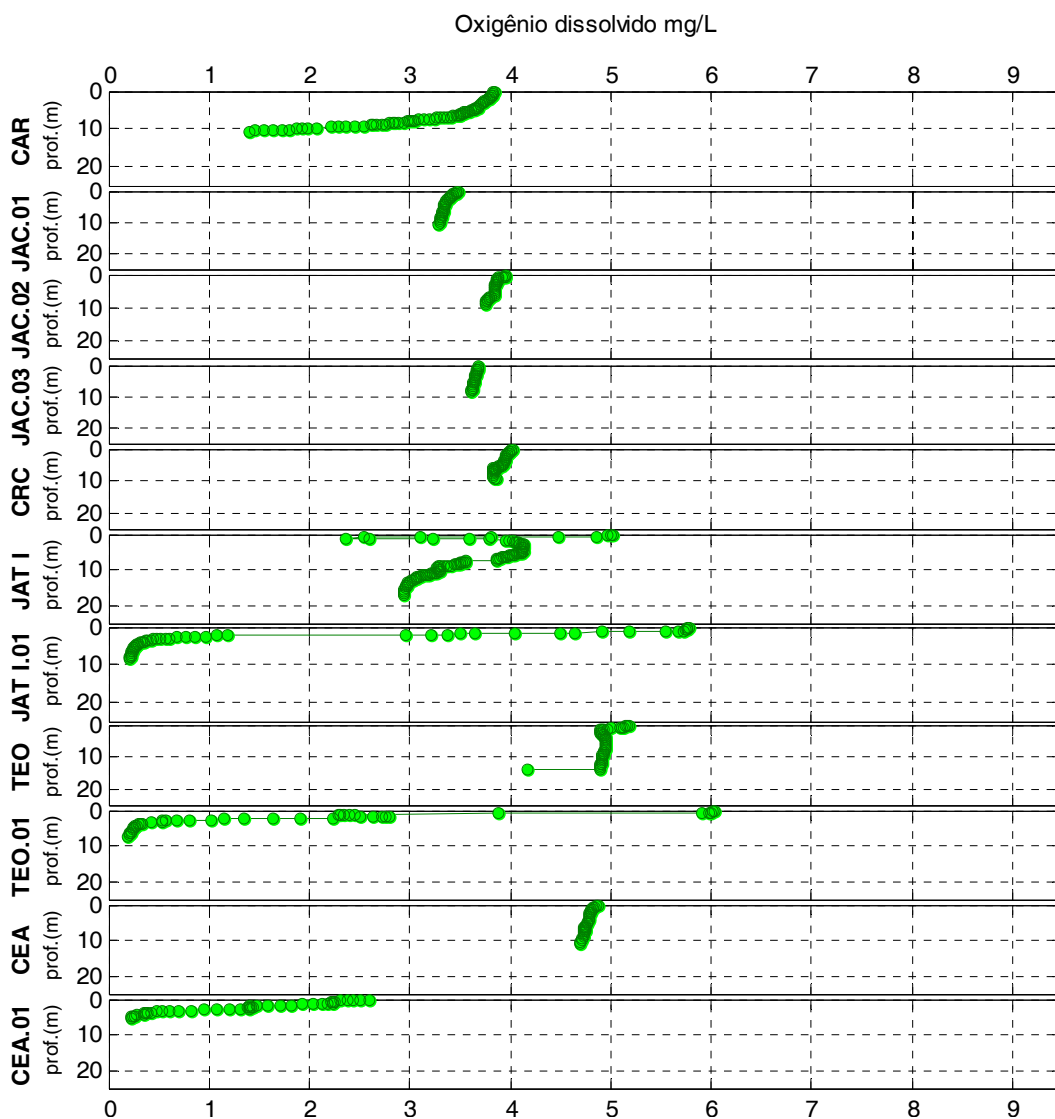
Figura 2-19 - Perfis de oxigênio dissolvido nos tributários em março de 2012 (águas altas).
