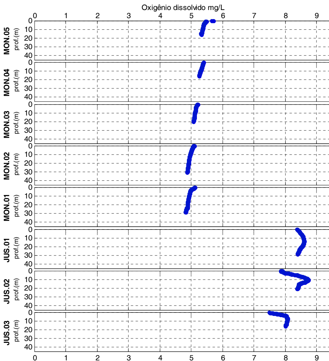
Figura 2-17 - Perfis de concentração de oxigênio dissolvido no rio Madeira em março de 2012 (águas altas).
