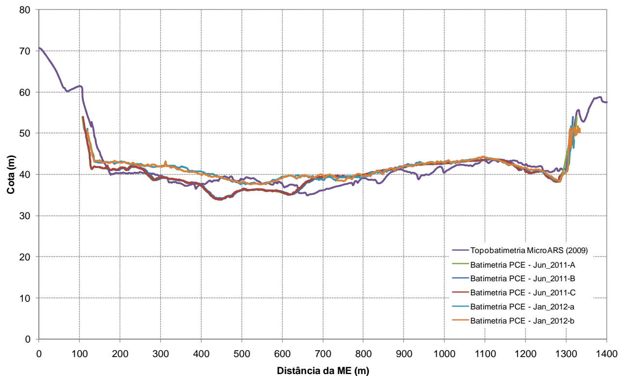
Figura 3.5. Avaliação Comparativa da Batimetria da Seção Transversal ST 255,1 para Diferentes Momentos: março/2009, junho/2011 e janeiro/2012
