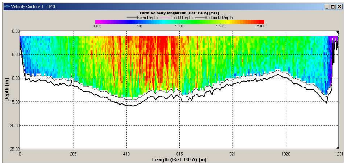
Figura 3.4. Medição de ADCP na Seção ST 255,1
