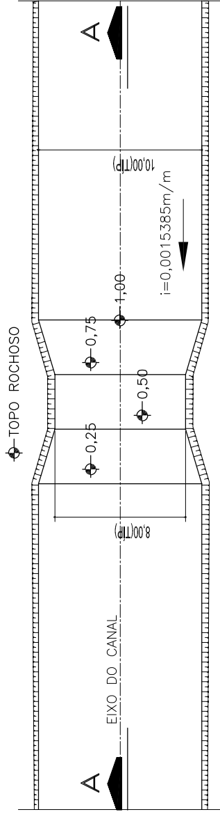
PLANTA
