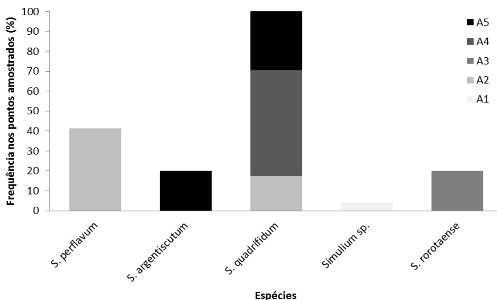
Figura 10. Frequência de espécies de simuliídeos nos macro-habitats: A1, A2, A3, A4 e A5, expressos em percentuais de pontos amostrados na UHE Santo Antônio, Porto Velho - RO, durante o período chuvoso (sétima campanha - março de 2013).
