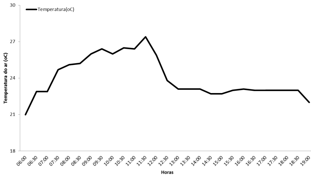
Figura 30. Relação da hora do dia e obtidos de temperatura do ar obtidos na margem esquerda do rio Caracol na área da UHE Santo Antônio, Porto Velho – RO, na décima segunda campanha de monitoramento, no período seco (19/09/2014).
