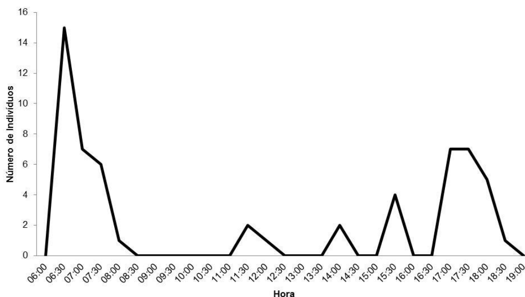
Figura 32. Atividade antropofílica de S. argentiscutum desenvolvida na margem esquerda do rio Caracol na área da UHE Santo Antônio, Porto Velho – RO, na décima terceira campanha de monitoramento, no período chuvoso (13/02/2015).
