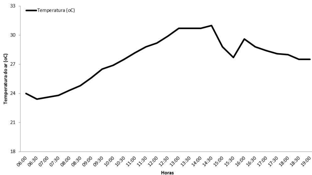
Figura 33. Relação da hora do dia e obtidos de temperatura do ar obtidos na margem esquerda do rio Caracol na área da UHE Santo Antônio, Porto Velho – RO, na décima terceira campanha de monitoramento, no período chuvoso (13/02/2015).
