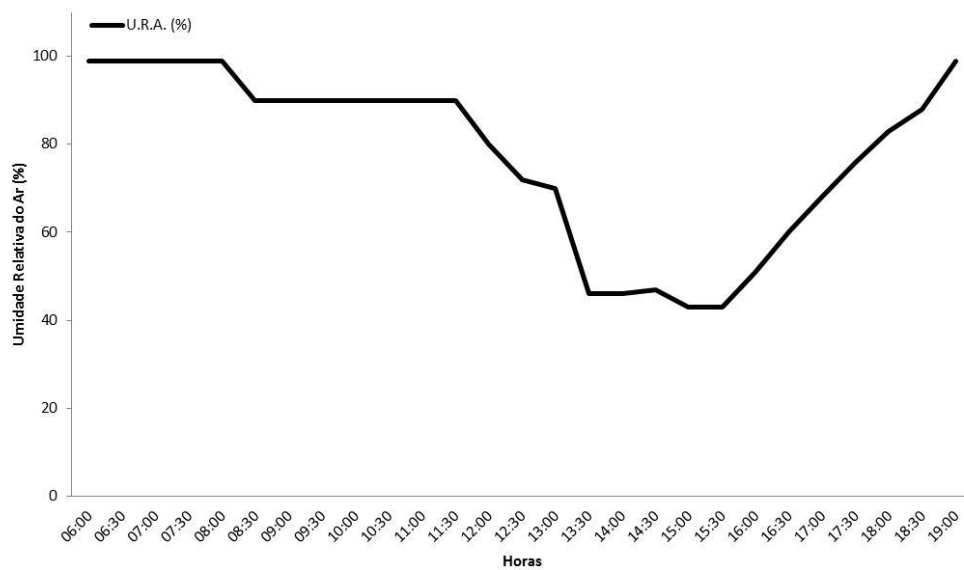
Figura 22. Relação da hora do dia e obtidos de umidade relativa do ar obtidos na margem esquerda do rio Caracol na área da UHE Santo Antônio, Porto Velho – RO, durante a sétima campanha de monitoramento, período chuvoso (25/03/2013).
