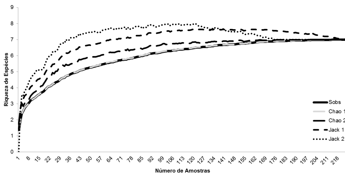
Figura 9. Curva de acumulação de espécies e estimadores de riqueza das espécies de simúlídeos por número de amostras obtidas nas áreas da UHE Santo Antônio, Porto Velho - RO.
