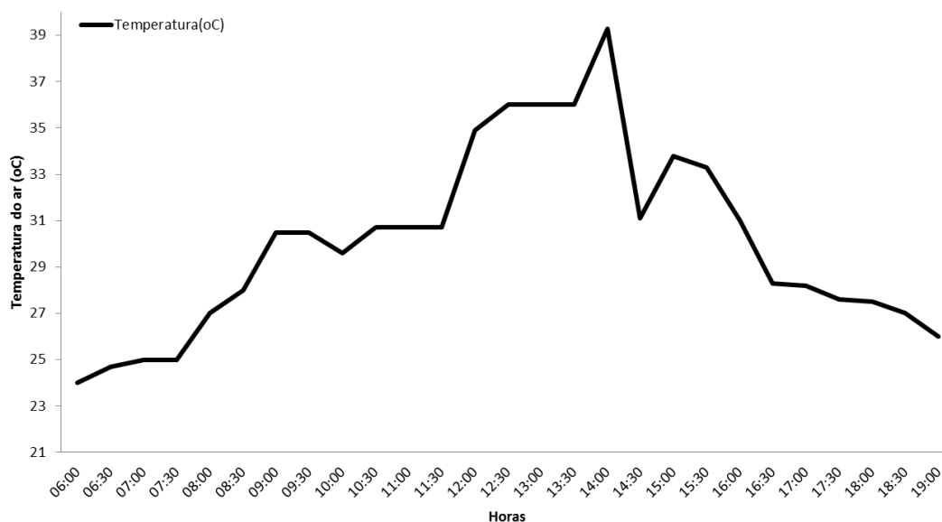
Figura 24. Relação da hora do dia e obtidos de temperatura do ar obtidos na margem esquerda do rio Caracol na área da UHE Santo Antônio, Porto Velho – RO, durante a nona campanha de monitoramento, período seco (21/09/2013).
