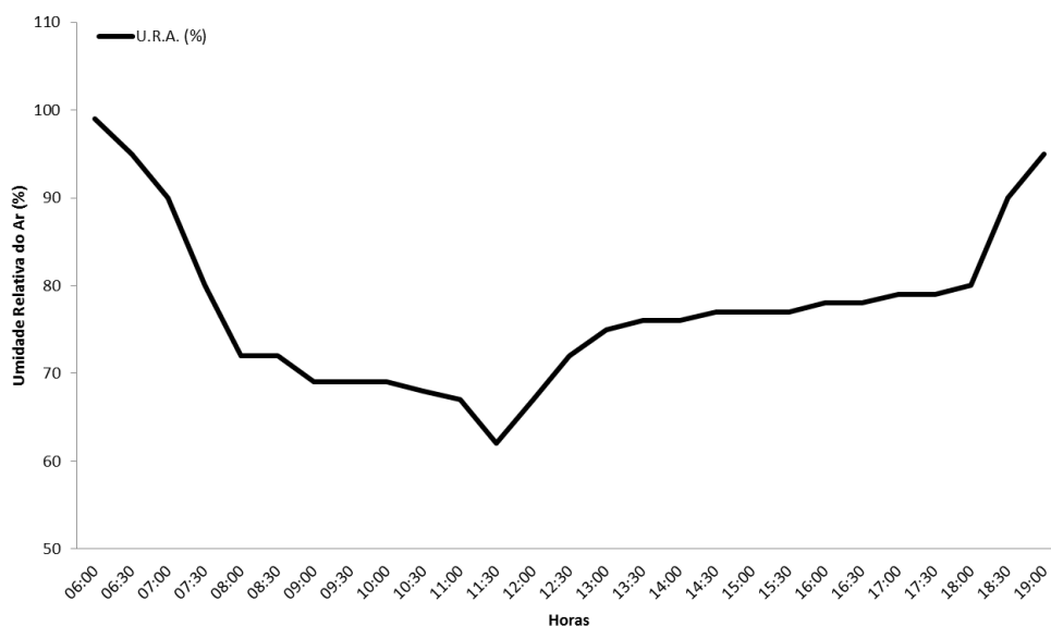
Figura 28. Relação da hora do dia e obtidos de umidade relativa do ar obtidos na margem esquerda do rio Caracol na área da UHE Santo Antônio, Porto Velho – RO, na décima campanha de monitoramento, início do período chuvoso (27/01/2014).
