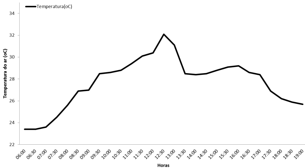
Figura 36. Relação da hora do dia e obtidos de temperatura do ar obtidos na margem esquerda do rio Caracol na área da UHE Santo Antônio, Porto Velho – RO, na décima quarta campanha de monitoramento, no período chuvoso (24/05/2015).
