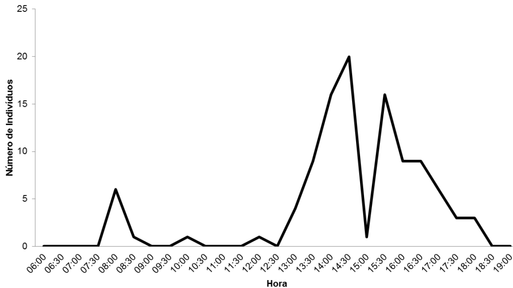
Figura 26. Atividade antropofílica de S. argentiscutum desenvolvida na margem esquerda do rio Caracol na área da UHE Santo Antônio, Porto Velho – RO, na décima campanha de monitoramento, início do período chuvoso (27/01/2014).
