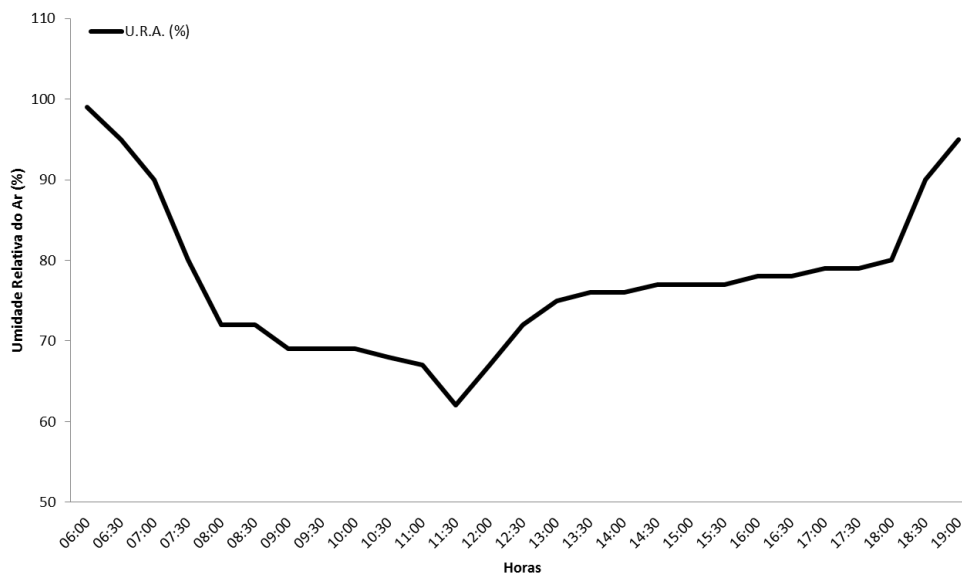
Figura 31. Relação da hora do dia e obtidos de umidade relativa do ar obtidos na margem esquerda do rio Caracol na área da UHE Santo Antônio, Porto Velho – RO, na décima segunda campanha de monitoramento, no período seco (19/09/2014).
