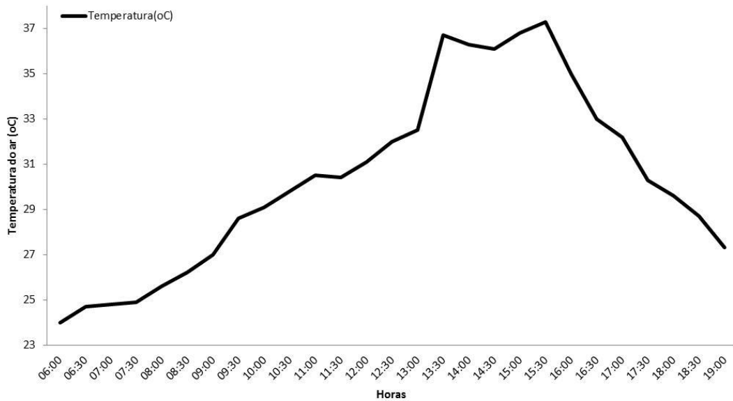
Figura 21. Relação da hora do dia e obtidos de temperatura do ar obtidos na margem esquerda do rio Caracol na área da UHE Santo Antônio, Porto Velho – RO, durante a sétima campanha de monitoramento, período chuvoso (25/03/2013).
