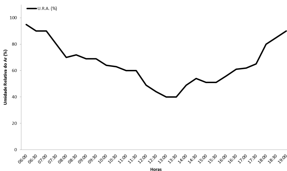
Figura 25. Relação da hora do dia e obtidos de umidade relativa do ar obtidos na margem esquerda do rio Caracol na área da UHE Santo Antônio, Porto Velho – RO, durante a nona campanha de monitoramento, período seco (21/09/2013).
