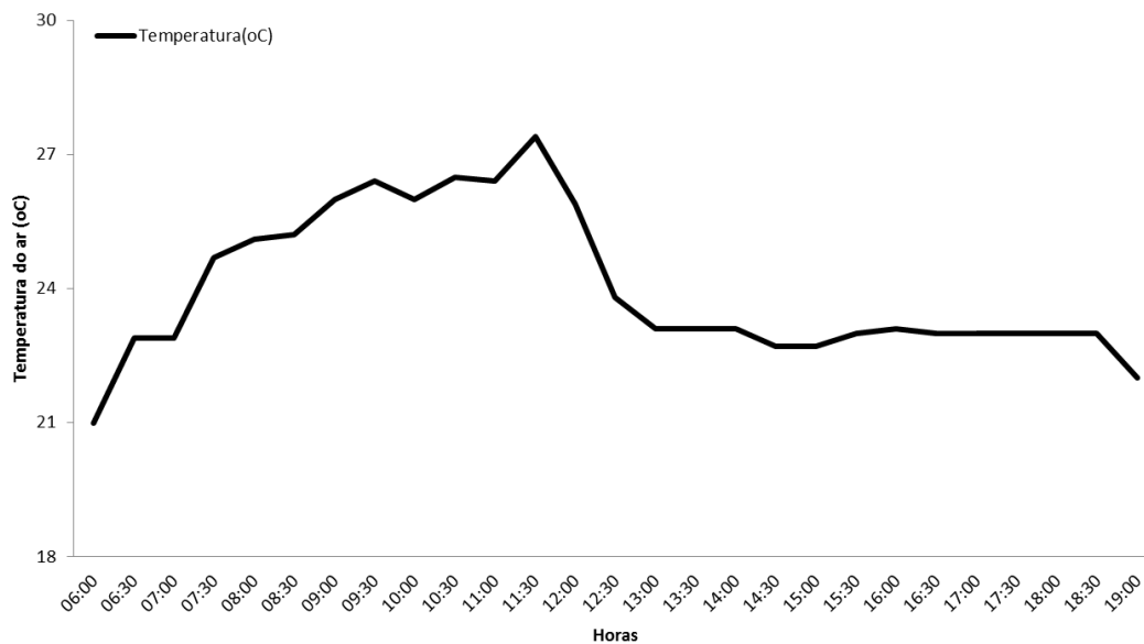
Figura 27. Relação da hora do dia e obtidos de temperatura do ar obtidos na margem esquerda do rio Caracol na área da UHE Santo Antônio, Porto Velho – RO, na décima campanha de monitoramento, início do período chuvoso (27/01/2014).
