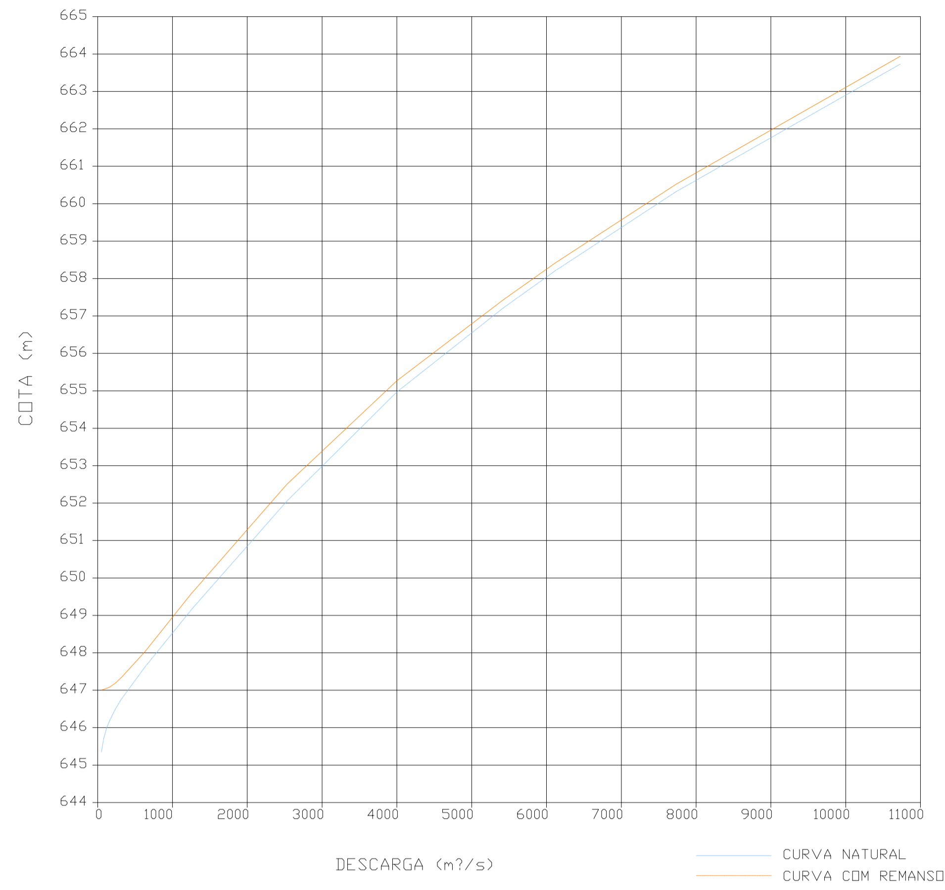
CURVAS DE DESCARGA NA SEÇÃO 05
