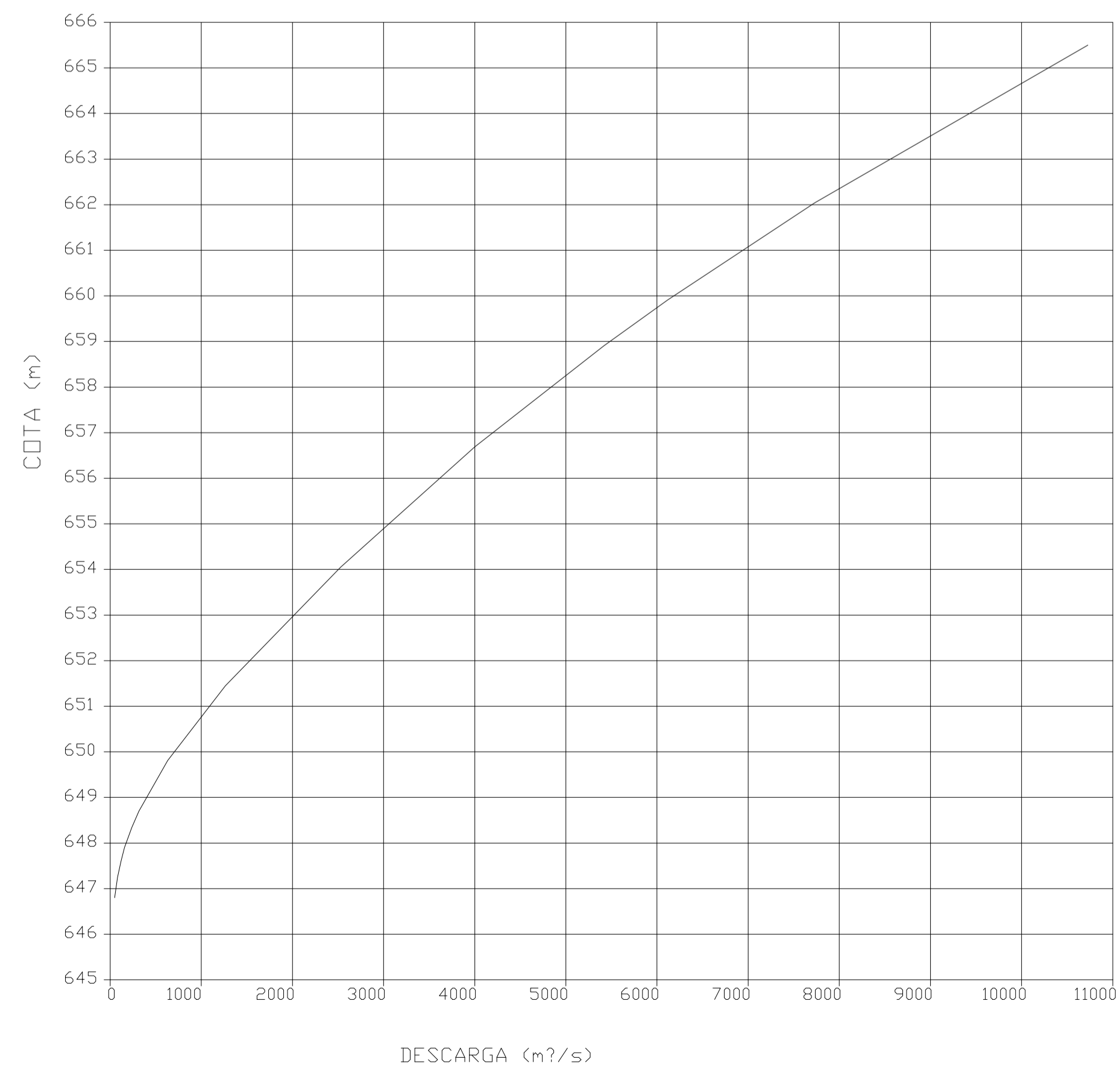
CURVA DE DESCARGA NA SEÇÃO 12
