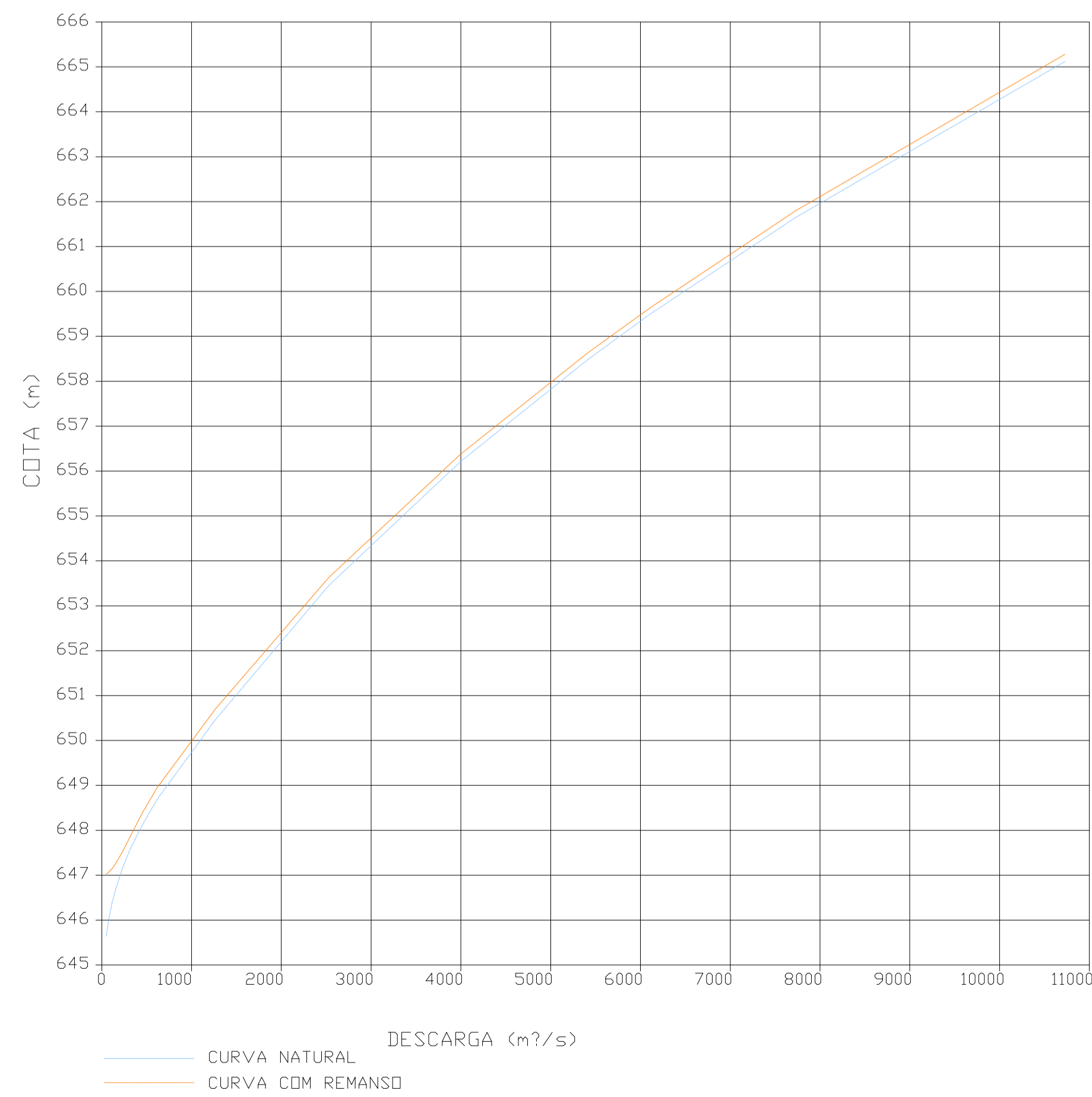
CURVAS DE DESCARGA NA SEÇÃO 11
