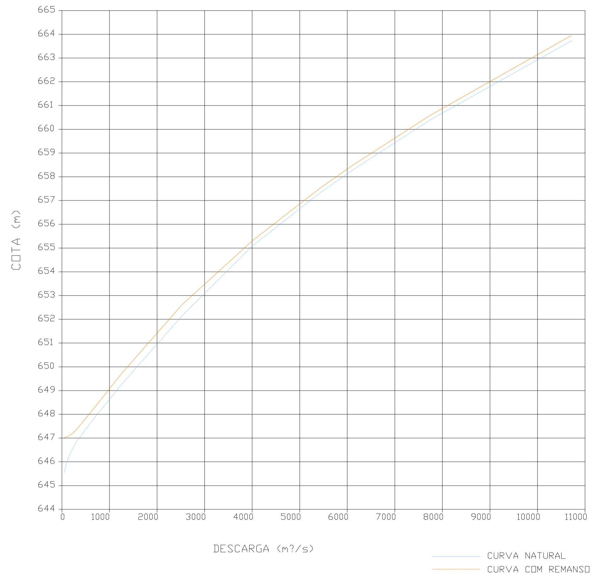
CURVAS DE DESCARGA NA SEÇÃO 06
