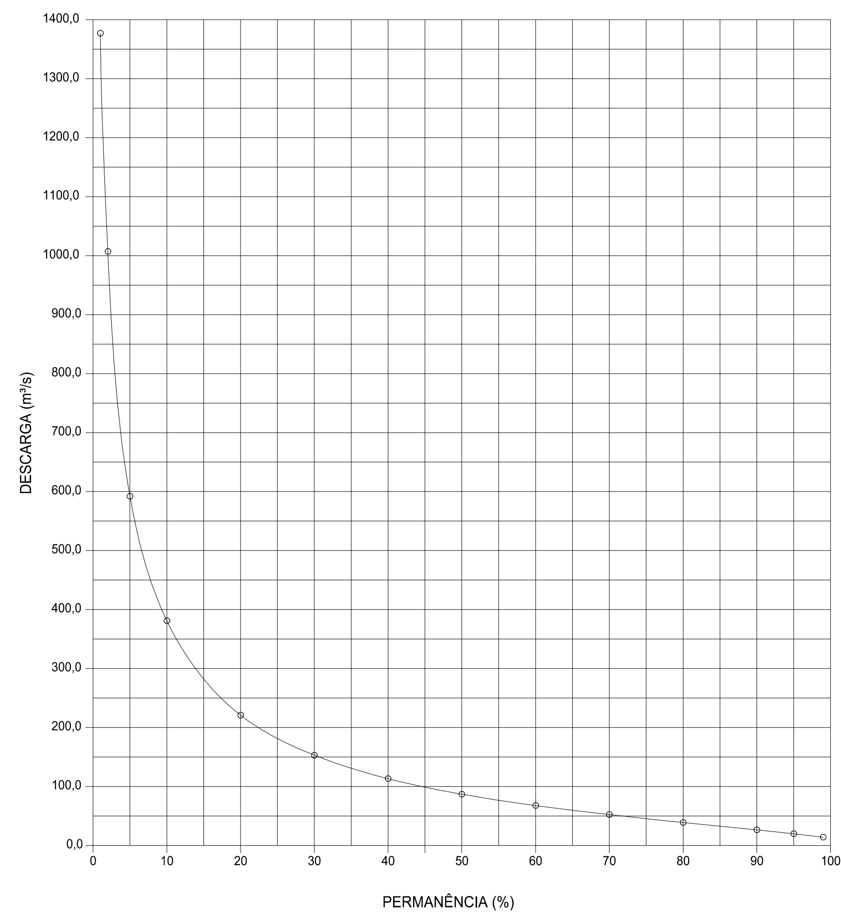
CURVA DE PERMANÊNCIA DE DESCARGAS MÉDIAS DIÁRIAS
