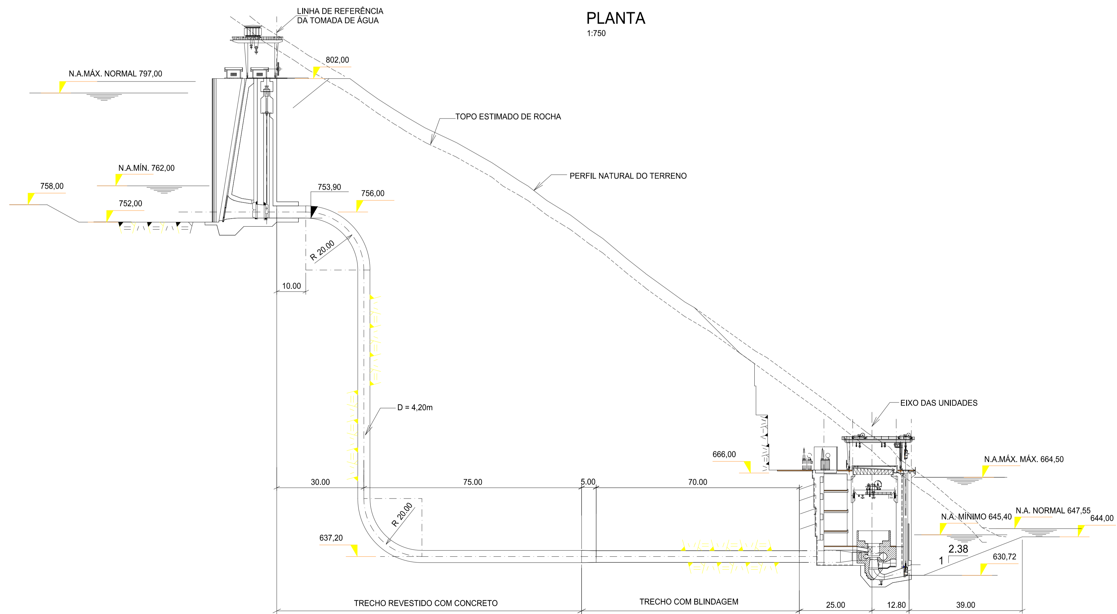
PERFIL DO CIRCUITO HIDRÁULICO DE GERAÇÃO TUNEL FORÇADO Nº 02 1:750
