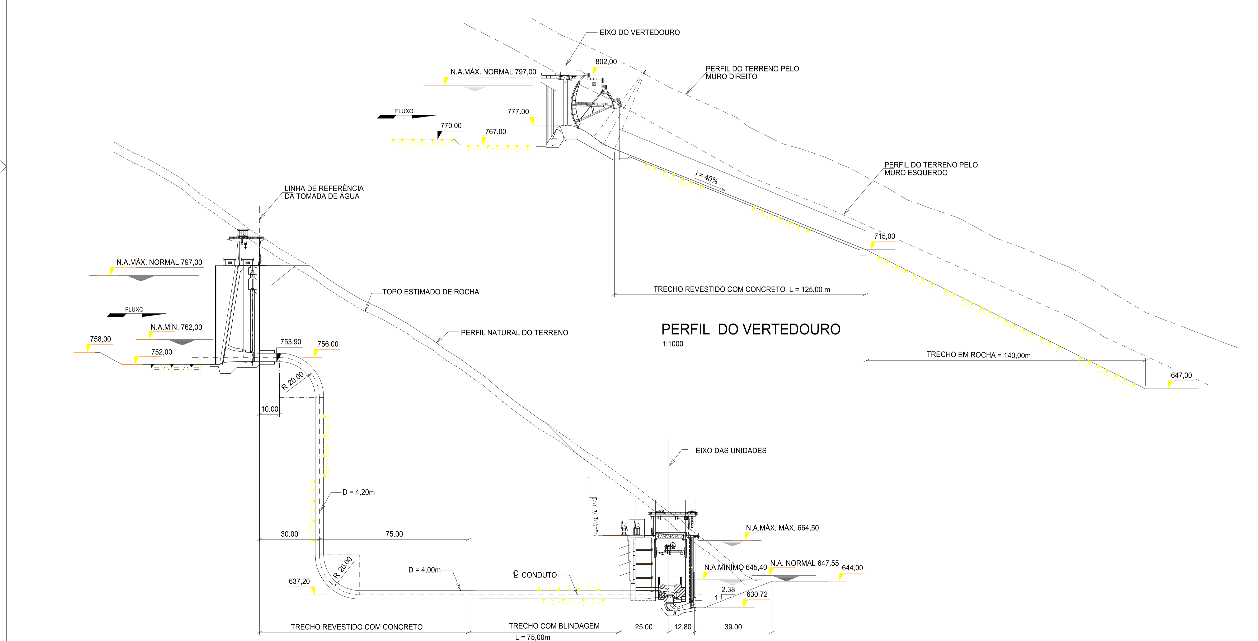
PERFIL DO CIRCUITO HIDRÁULICO DE GERAÇÃO TÚNEL FORÇADO Nº 01 1:1000
