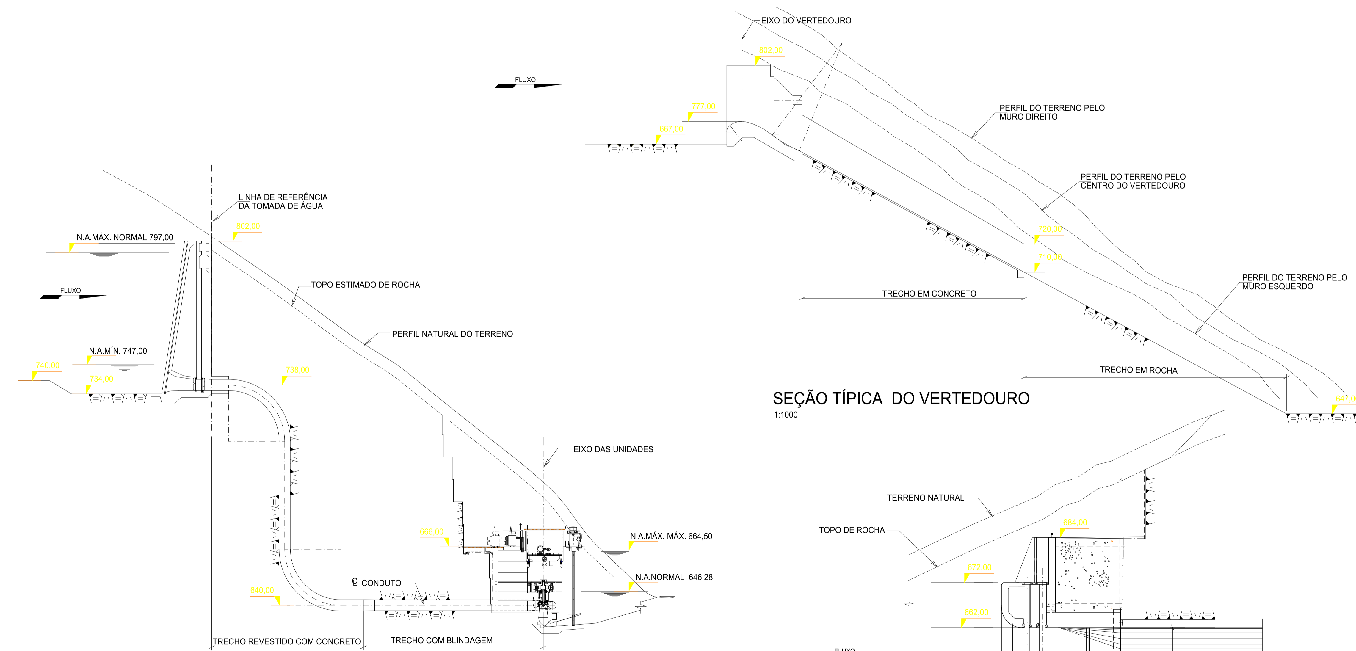
PERFIL DO CIRCUITO HIDRÁULICO DE GERAÇÃO 1:1000
