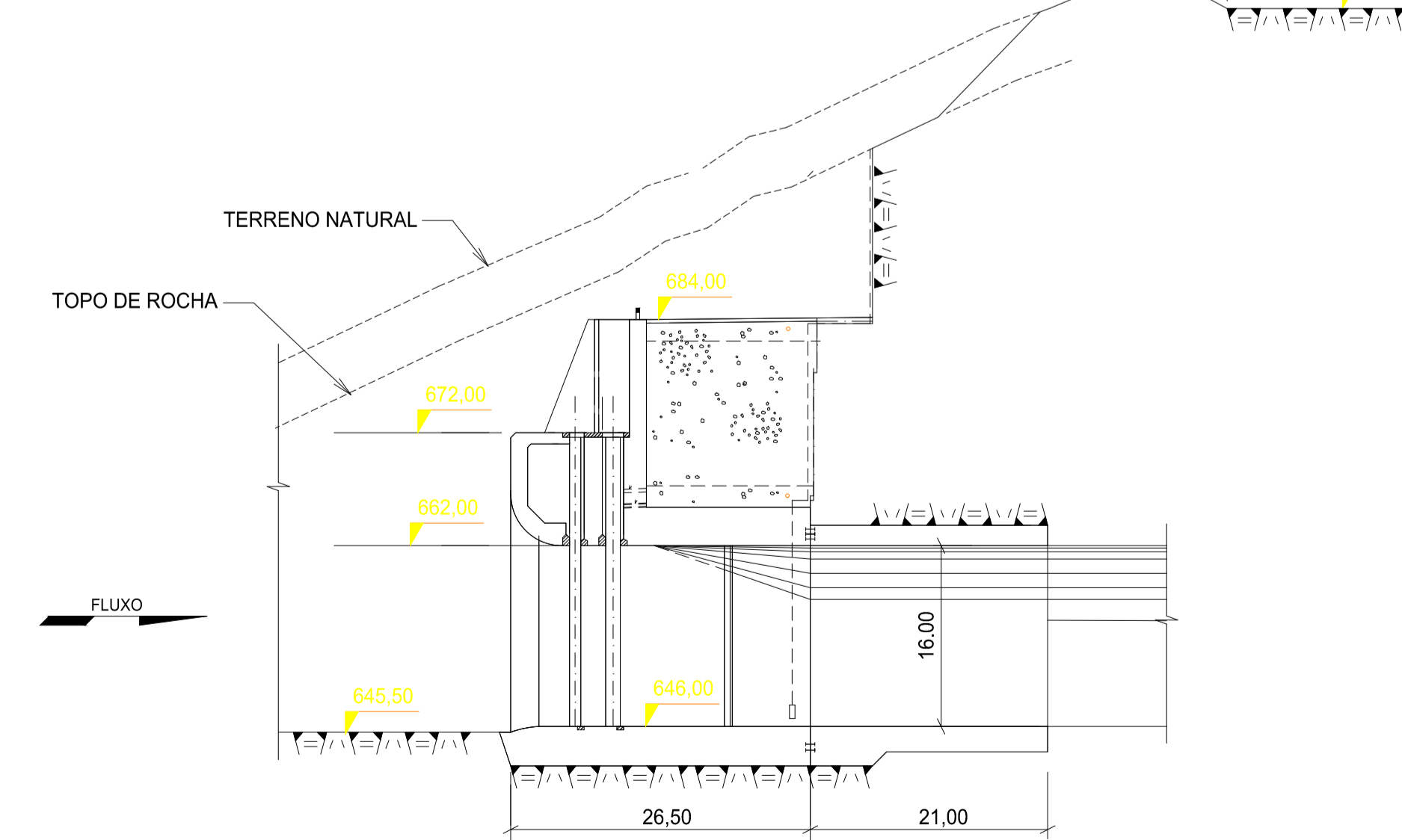
SEÇÃO TÍPICA DAS ESTRUTURAS DE FECHAMENTO 1:500
