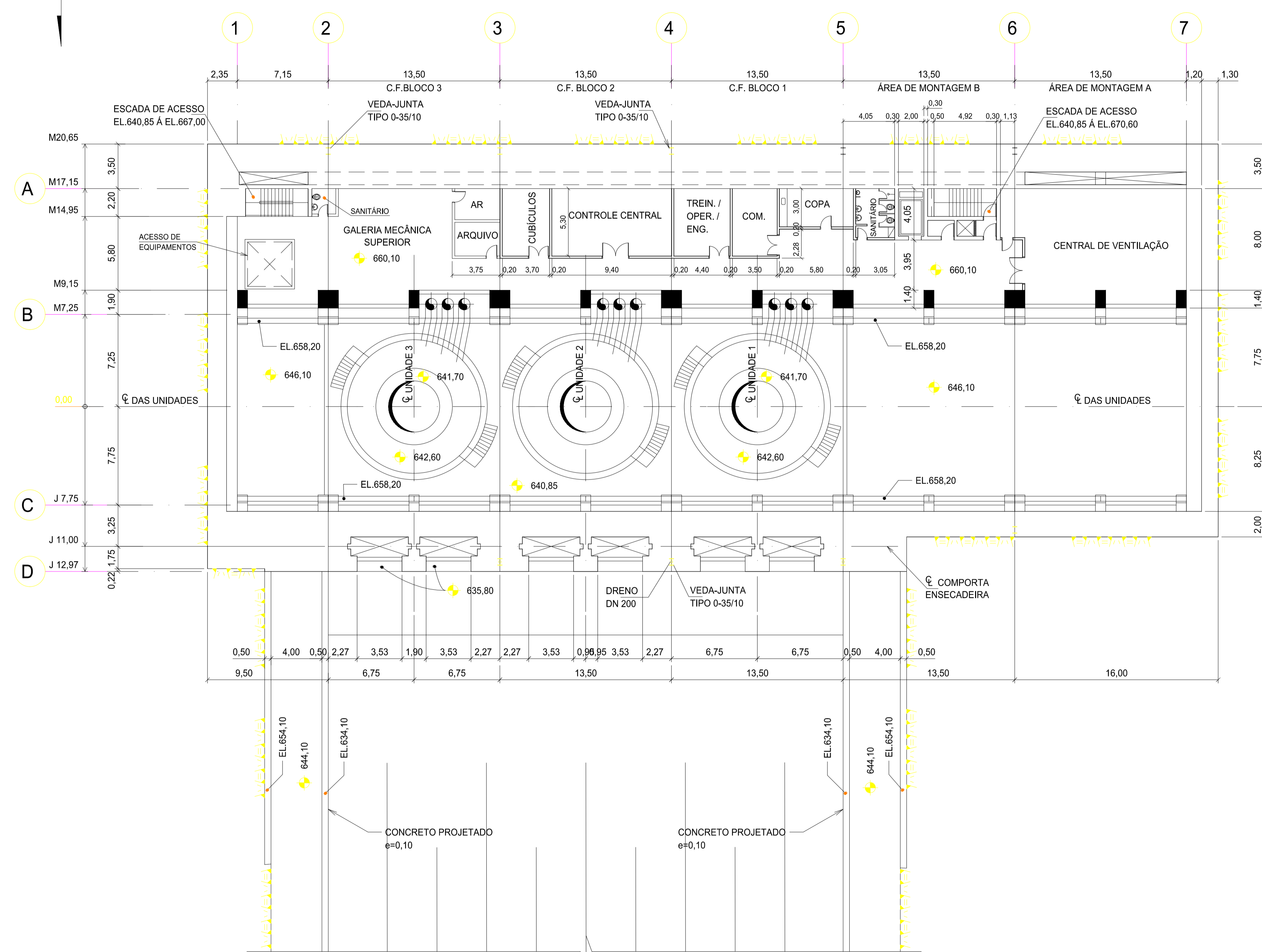
PLANTA NA EL.660,10
