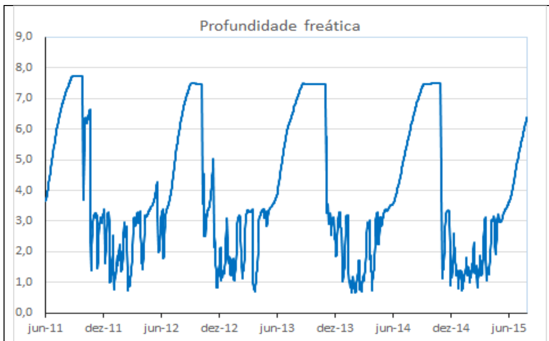
Gráfico 65 - Profundidade freática do PZ-33 do período de 01/06/2011 a 10/09/2015.
