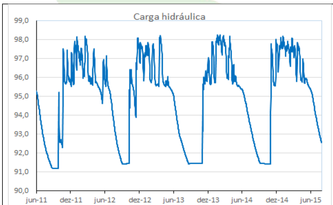
Gráfico 66 - Carga hidráulica do PZ-33 no período de 01/06/2011 a 10/09/2015.
