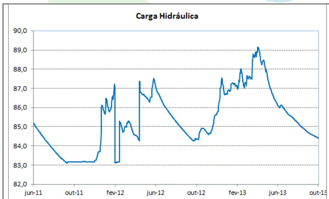
Gráfico 32 - Carga hidráulica do PZ-16 no período de 01/06/2011 a 01/10/2013.
