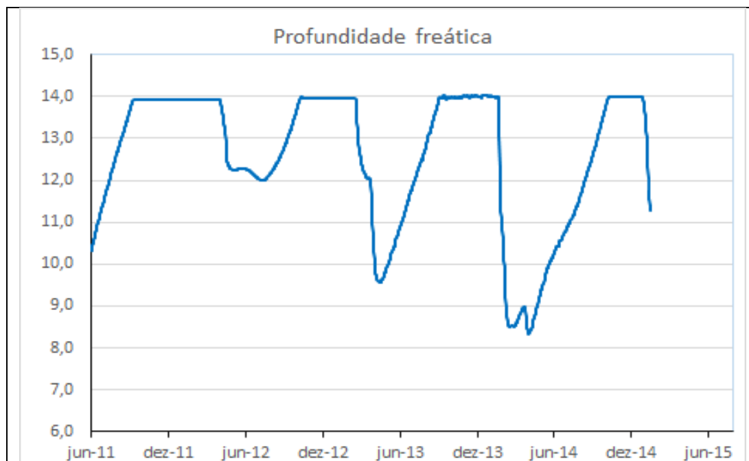
Gráfico 69 - Profundidade freática do PZ-35 do período de 01/06/2011 a 14/01/2015.
