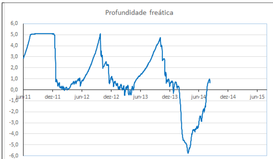
Gráfico 37 - Profundidade freática do PZ-19 do período de 01/06/2011 a 10/08/2014
