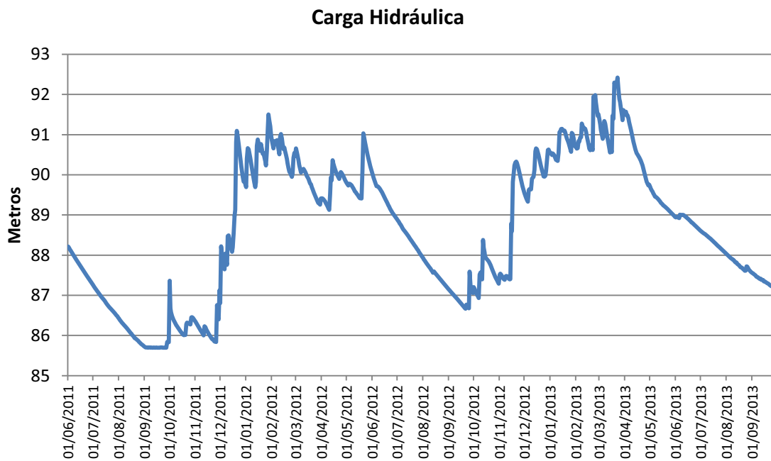
Gráfico 34 - Carga hidráulica do PZ-17 no período de 01/06/2011 a 01/09/2013
