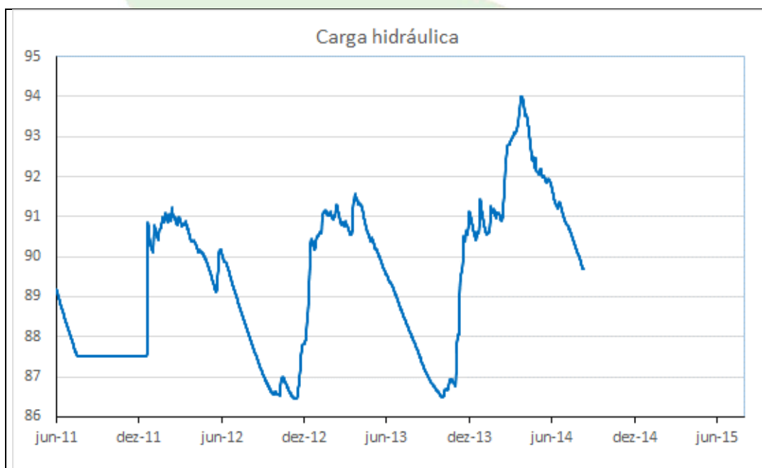
Gráfico 26 - Carga hidráulica do PZ-13 no período de 01/06/2011 a 09/08/2014.
