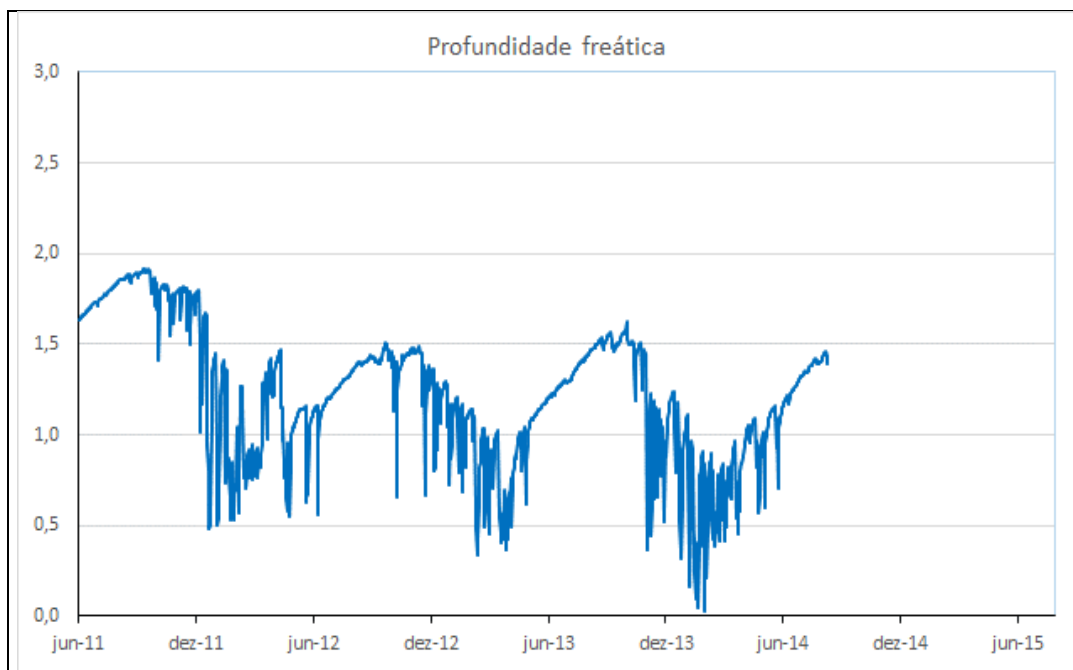
Gráfico 47 - Profundidade freática do PZ-24 do período de 01/06/2011 a 09/08/2014.
