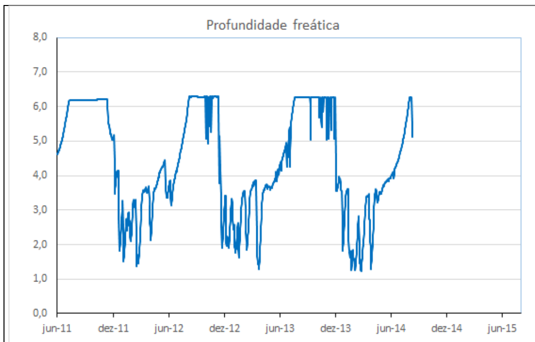
Gráfico 63 - Profundidade freática do PZ-32 do período de 01/06/2011 a 27/09/2014.
