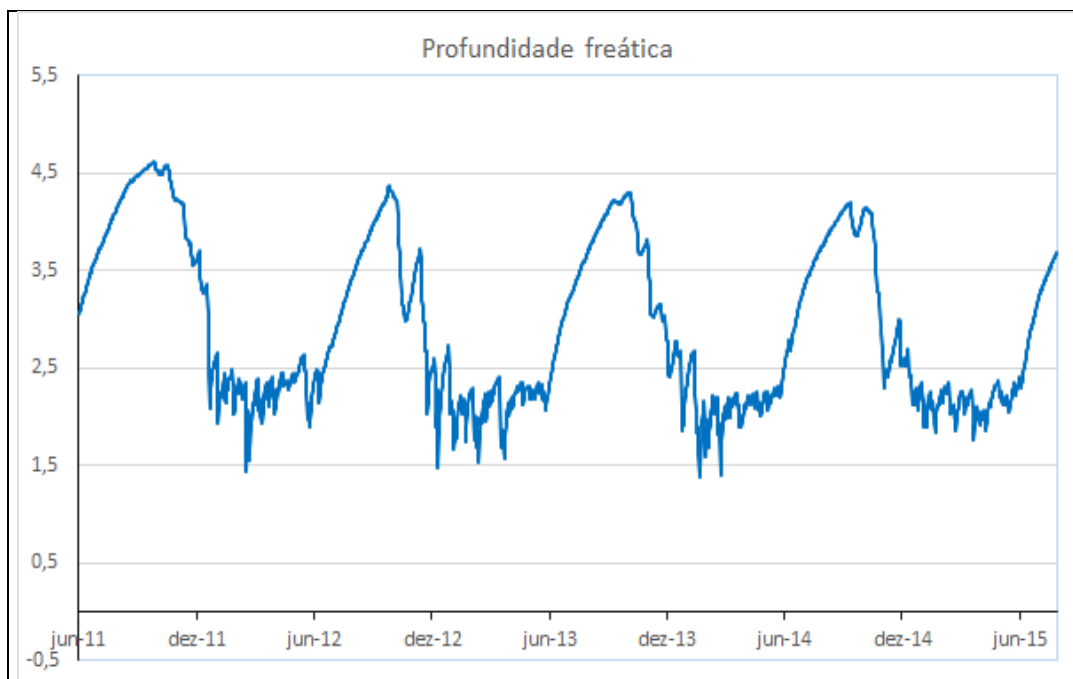
Gráfico 81 - Profundidade freática do PZ-41 do período de 01/06/2011 a 28/07/2015.
