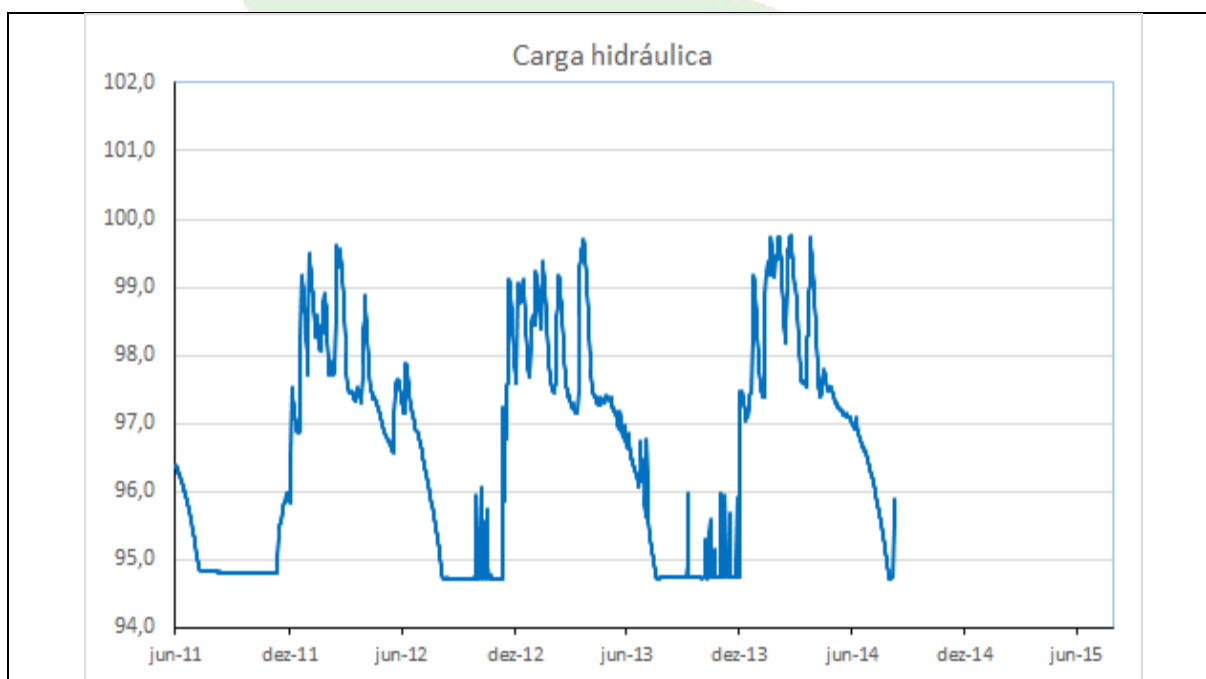
Gráfico 72 - Carga hidráulica do PZ-36 no período de 01/06/2011 a 27/09/2014.
