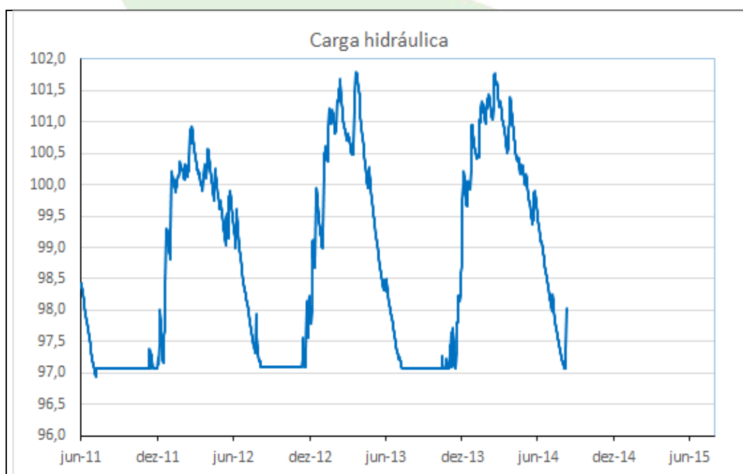
Gráfico 74 - Carga hidráulica do PZ-37 no período de 01/06/2011 a 27/09/2014.
