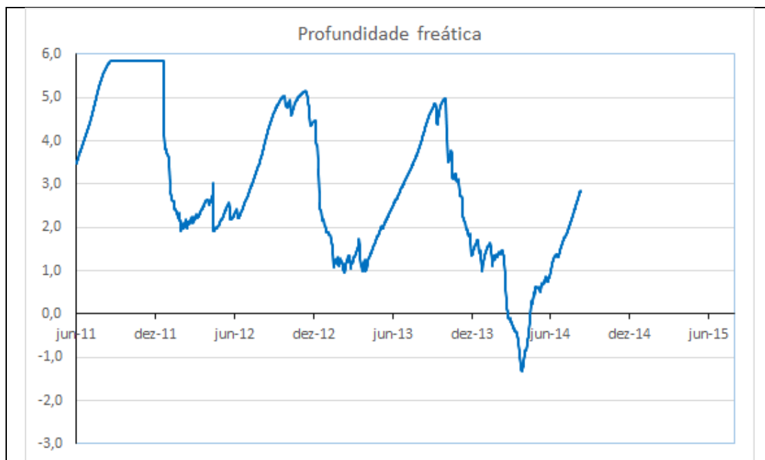
Gráfico 57 - Profundidade freática do PZ-29 do período de 01/06/2011 a 09/08/2014.
