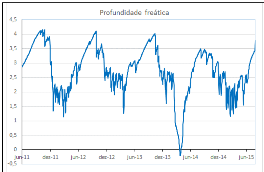
Gráfico 21 - Profundidade freática do PZ-11 do período de 01/06/2011 a 27/07/2015.
