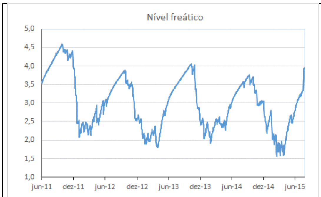
Gráfico 13 - Profundidade freática do PZ-07 do período de 01/06/2011 a 26/07/2015.
