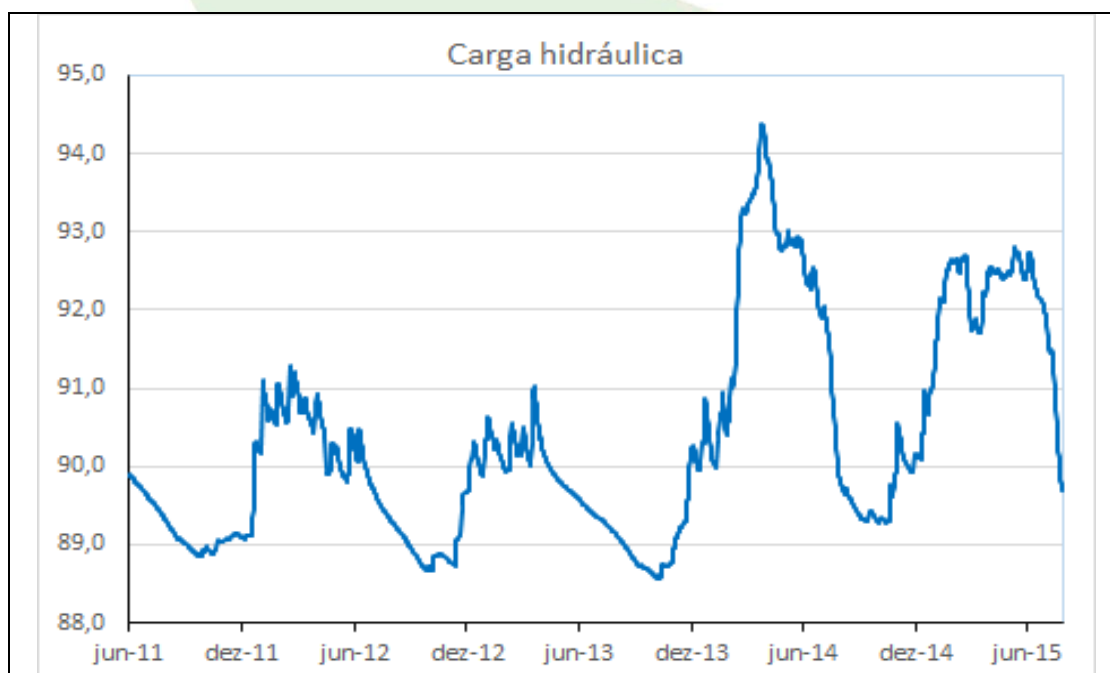
Gráfico 76 - Carga hidráulica do PZ-38 no período de 01/06/2011 a 29/07/2015.
