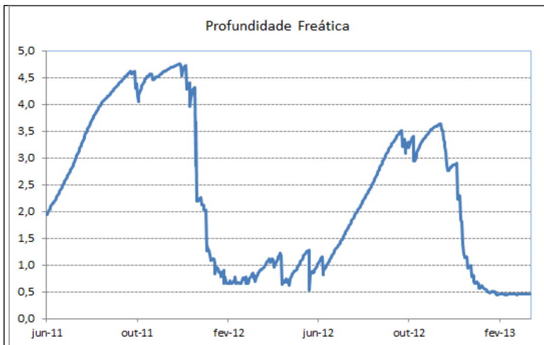
Gráfico 59 - Profundidade freática do PZ-30 do período de 01/06/2011 a 01/03/2013
