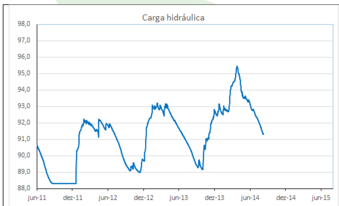
Gráfico 58 - Carga hidráulica do PZ-29 no período de 01/06/2011 a 09/08/2014.
