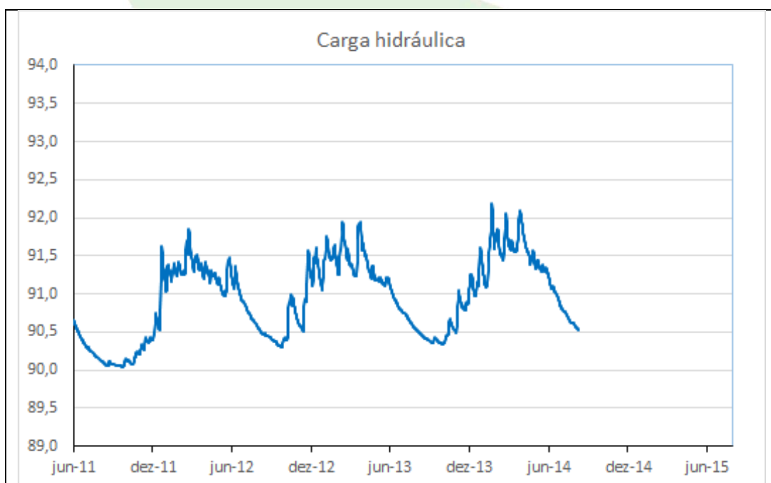
Gráfico 80 - Carga hidráulica do PZ-40 no período de 01/06/2011 a 10/08/2014.
