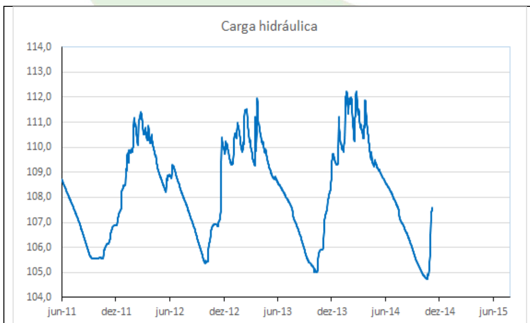
Gráfico 86 - Carga hidráulica do PZ-43 do período de 01/06/2011 a 07/11/2014.
