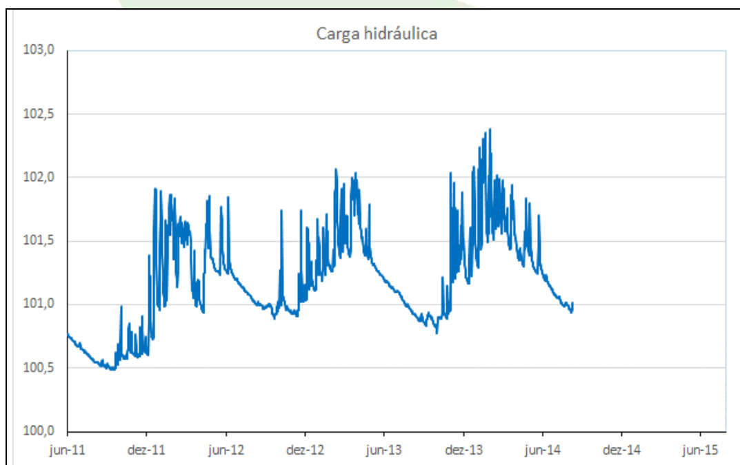
Gráfico 48 - Carga hidráulica do PZ-24 no período de 01/06/2011 a 09/08/2014.
