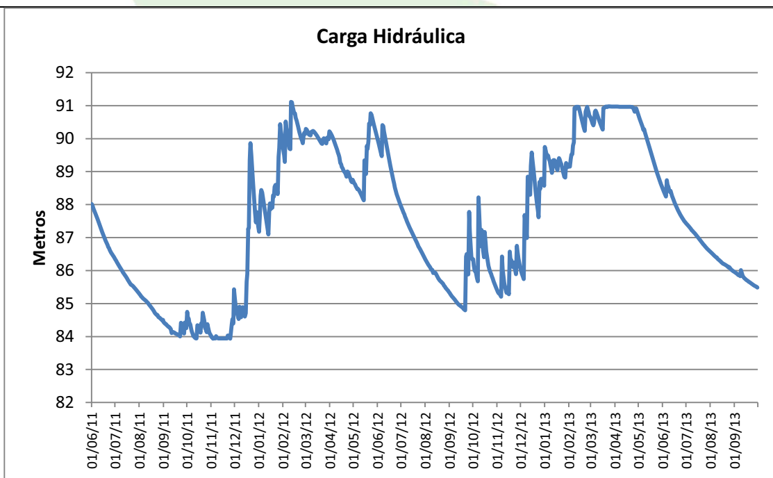
Gráfico 44 - Carga hidráulica do PZ-22 no período de 01/06/2011 a 01/09/2013
