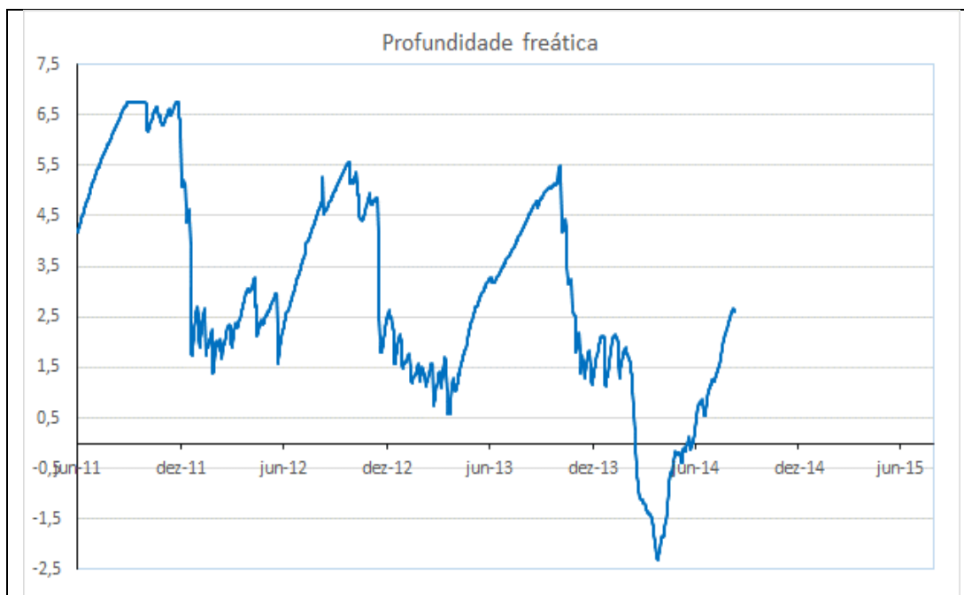
Gráfico 41 - Profundidade freática do PZ-21 do período de 01/06/2011 a 10/08/2014.
