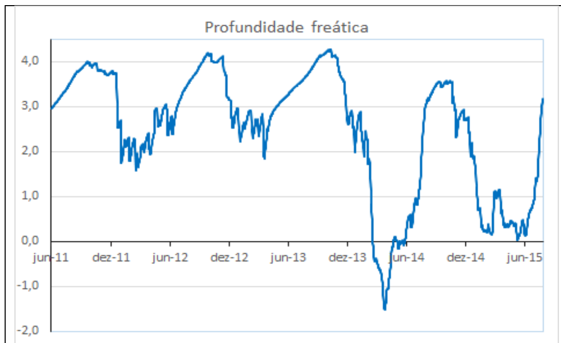
Gráfico 75 - Profundidade freática do PZ-38 do período de 01/06/2011 a 29/07/2015.
