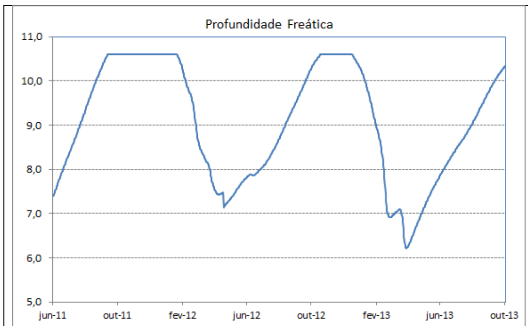
Gráfico 87 - Profundidade freática do PZ-44 do período de 01/06/2011 a 01/10/2013
