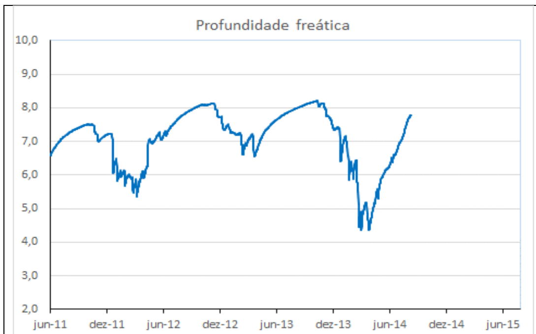
Gráfico 55 - Profundidade freática do PZ-28 do período de 01/06/2011 a 09/08/2014.
