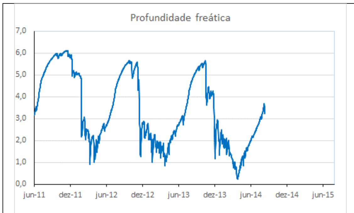
Gráfico 7 - Profundidade freática do PZ-04 do período de 01/06/2011 a 09/08/2014
