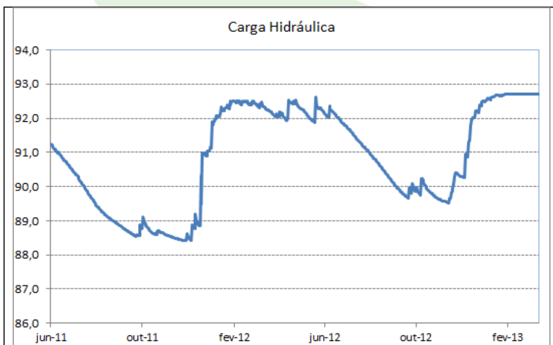
Gráfico 60 - Carga hidráulica do PZ-30 no período de 01/06/2011 a 01/03/2013
