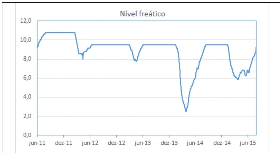
Gráfico 1 - Profundidade freática do PZ-01 do período de 01/06/2011 a 27/07/2015.
