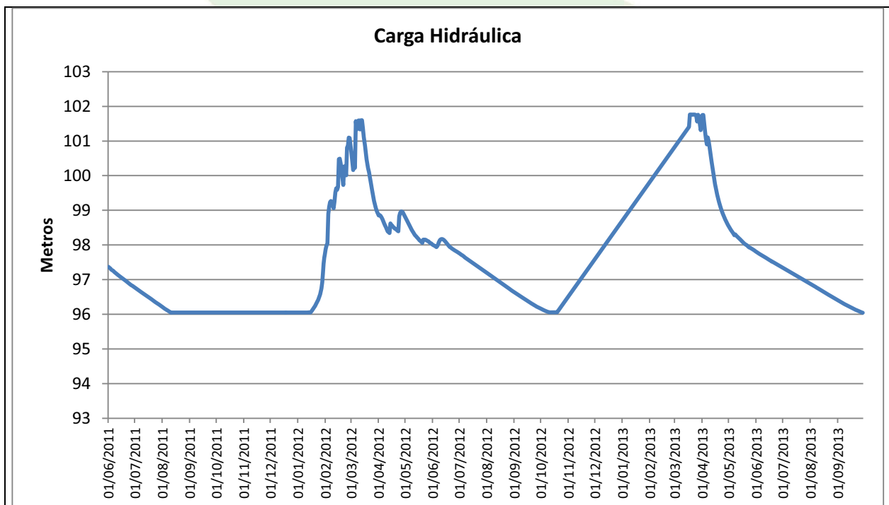
Gráfico 12 - Carga hidráulica do PZ-06 no período de 01/06/2011 a 01/09/2013
