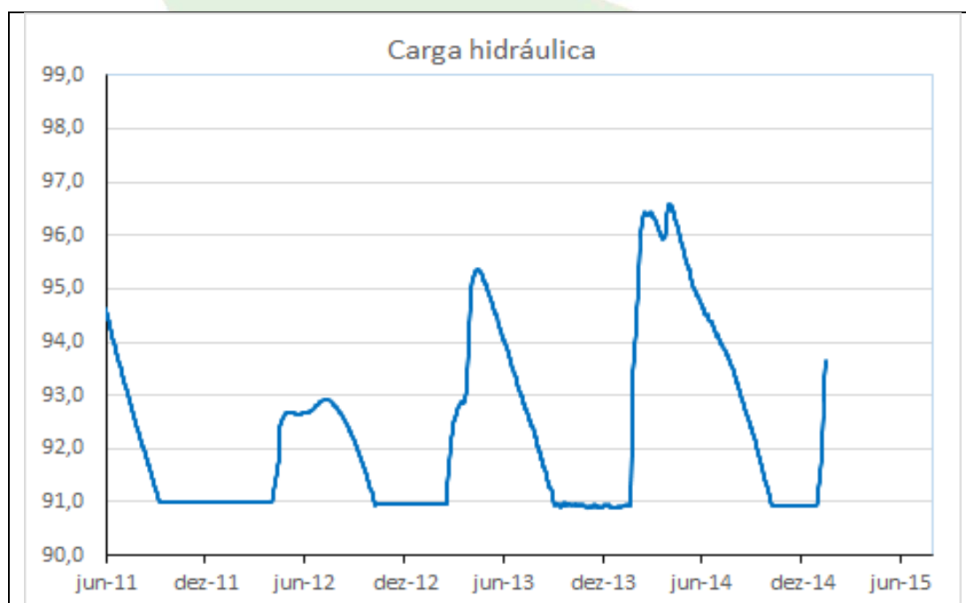
Gráfico 70 - Carga hidráulica do PZ-35 no período de 01/06/2011 a 14/01/2015.
