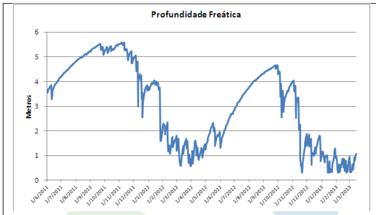
Gráfico 5 – Profundidade freática do PZ-03 do período de 01/06/2011 a 01/03/2013
