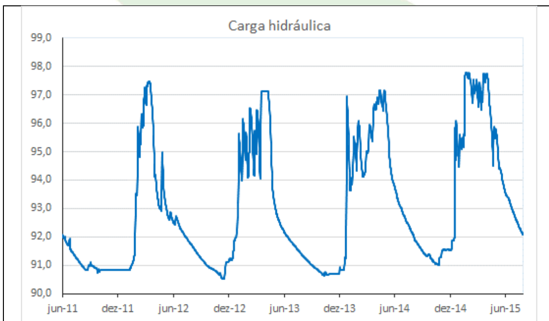
Gráfico 10 - Carga hidráulica do PZ-05 no período de 01/06/2011 a 28/07/2015.
