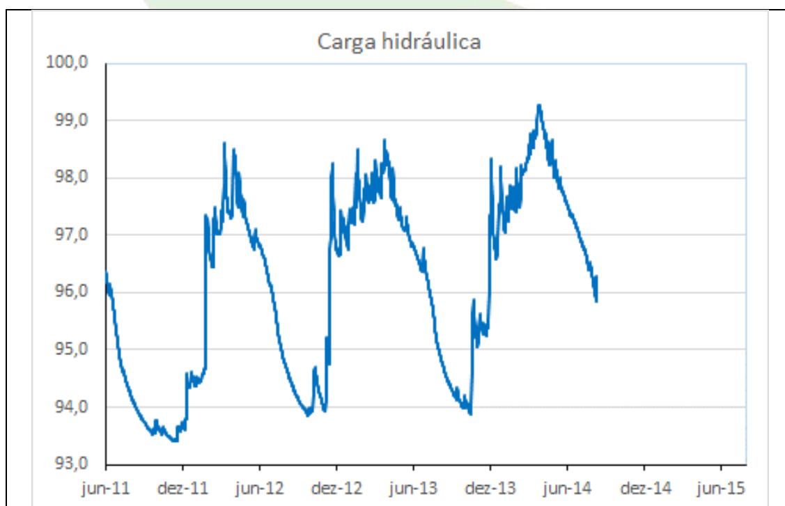
Gráfico 8 - Carga hidráulica do PZ-04 no período de 01/06/2011 a 09/08/2014
