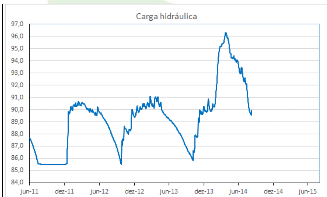
Gráfico 38 - Carga hidráulica do PZ-19 no período de 01/06/2011 a 10/08/2014
