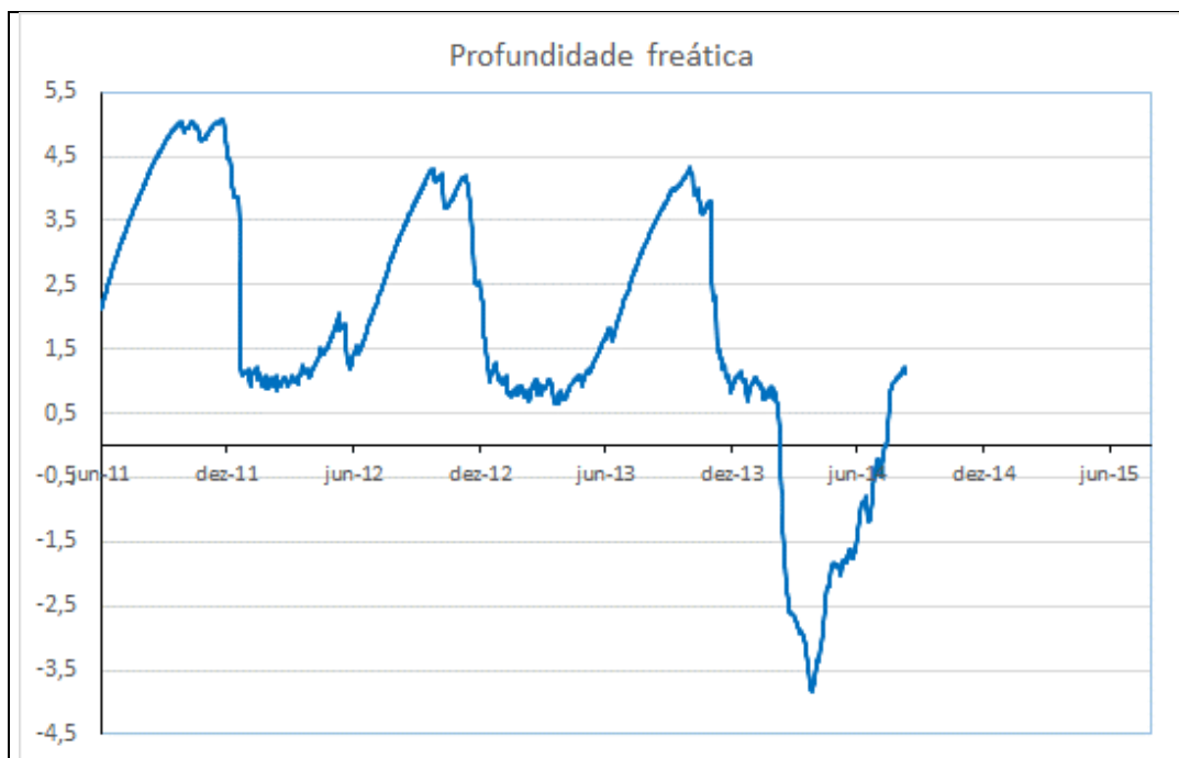
Gráfico 27 - Profundidade freática do PZ-14 do período de 01/06/2011 a 09/08/2014.
