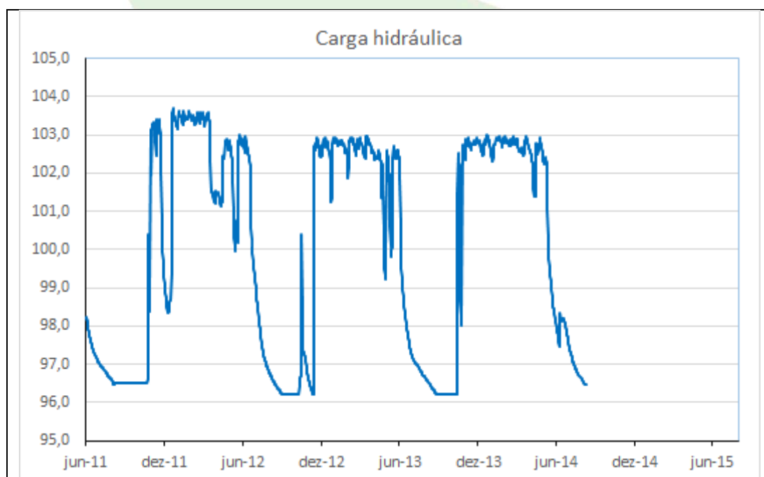
Gráfico 78 - Carga hidráulica do PZ-39 no período de 01/06/2011 a 09/08/2014.
