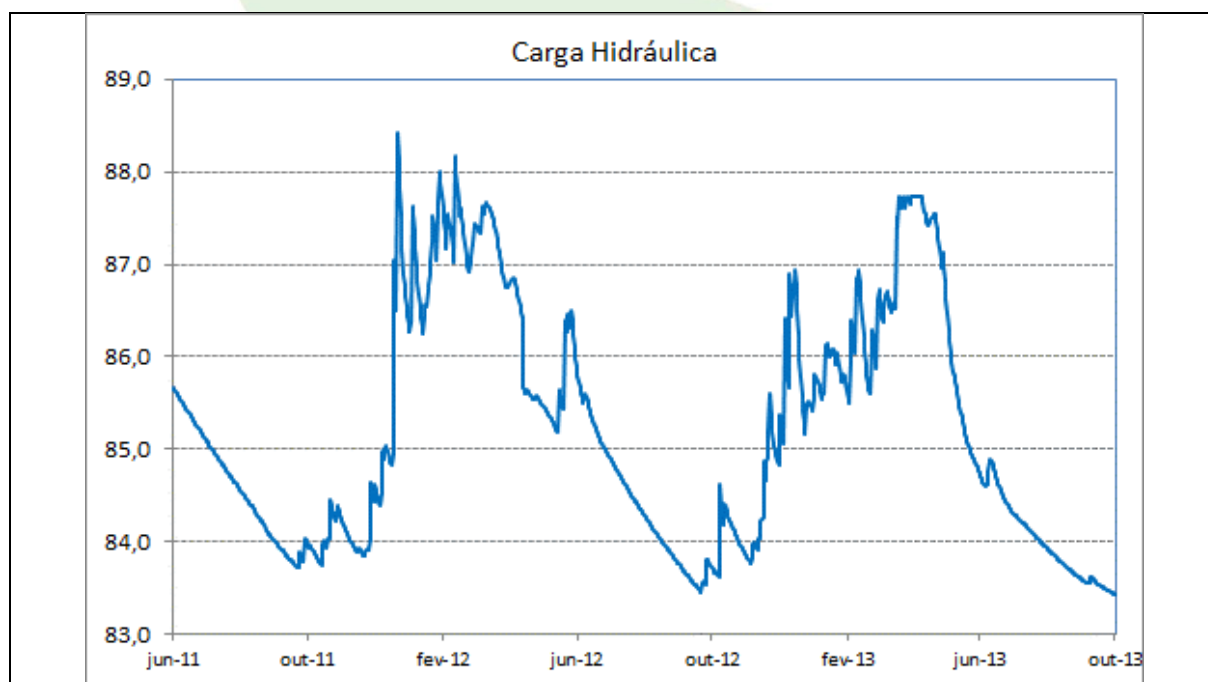
Gráfico 52 - Carga hidráulica do PZ-26 no período de 01/06/2011 a 01/10/2013.
