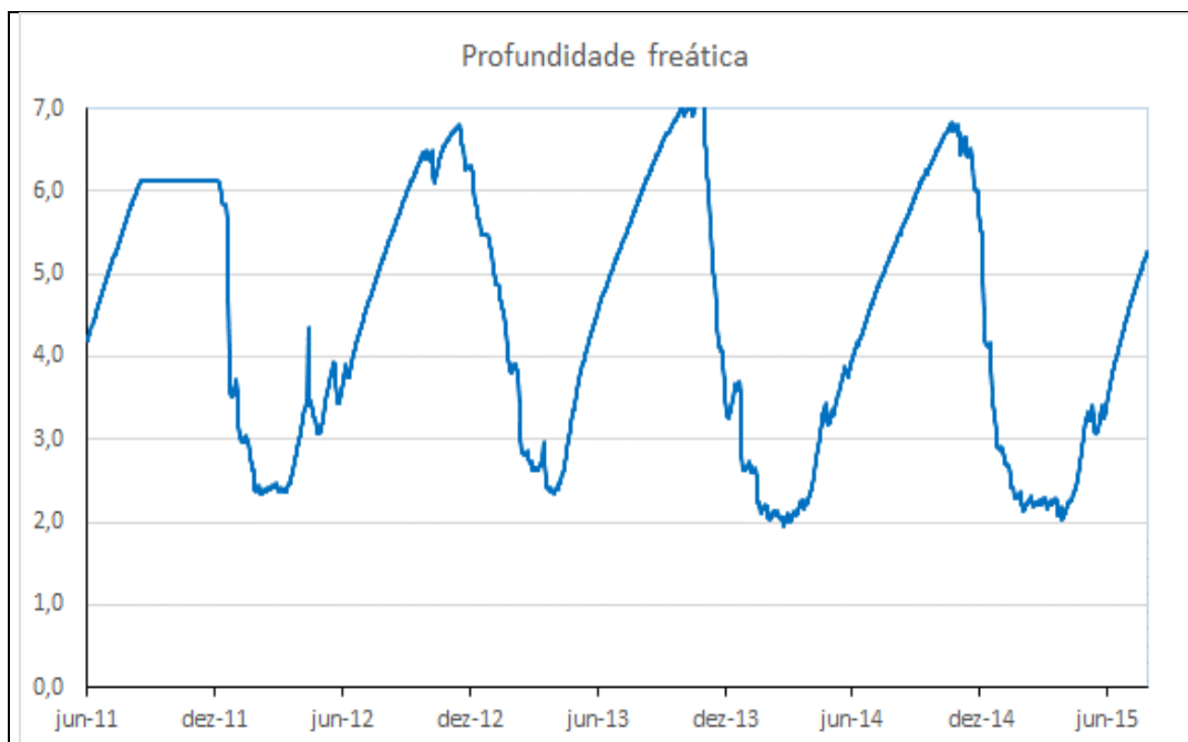
Gráfico 49 - Profundidade freática do PZ-25 do período de 01/06/2011 a 29/07/2015.
