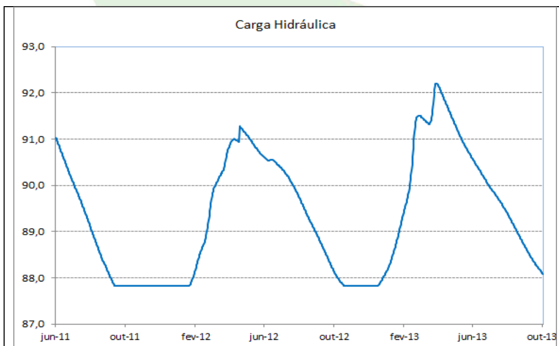
Gráfico 88 - Carga hidráulica do PZ-44 no período de 01/06/2011 a 01/10/2013
