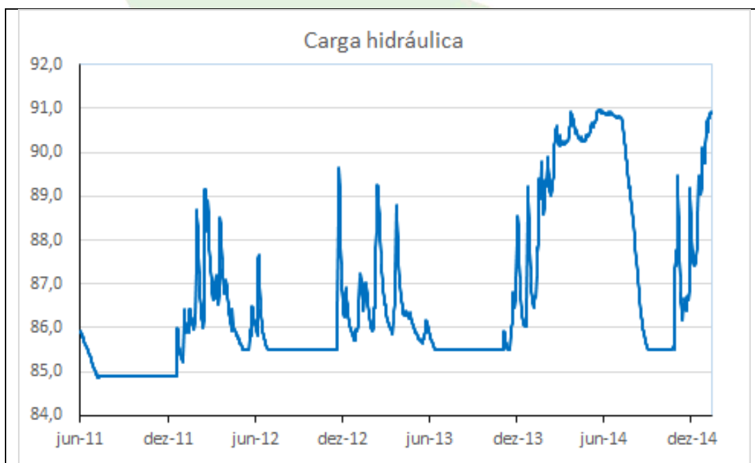
Gráfico 84 - Carga hidráulica do PZ-42 no período de 01/06/2011 a 13/01/2015.
