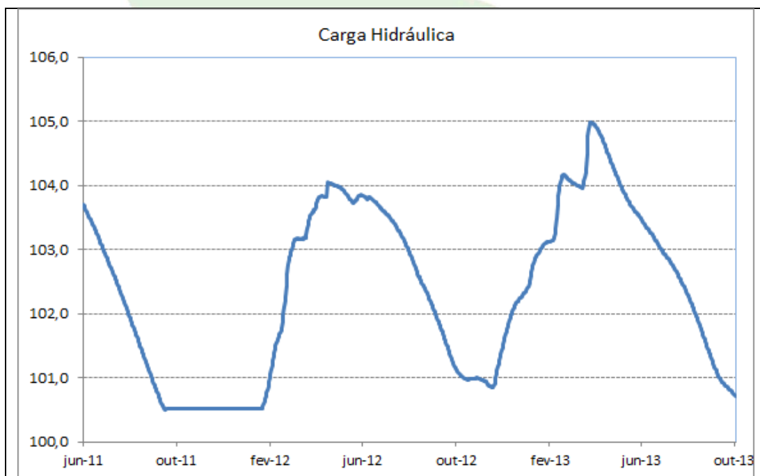
Gráfico 68 - Carga hidráulica do PZ-34 no período de 01/06/2011 a 01/10/2013.
