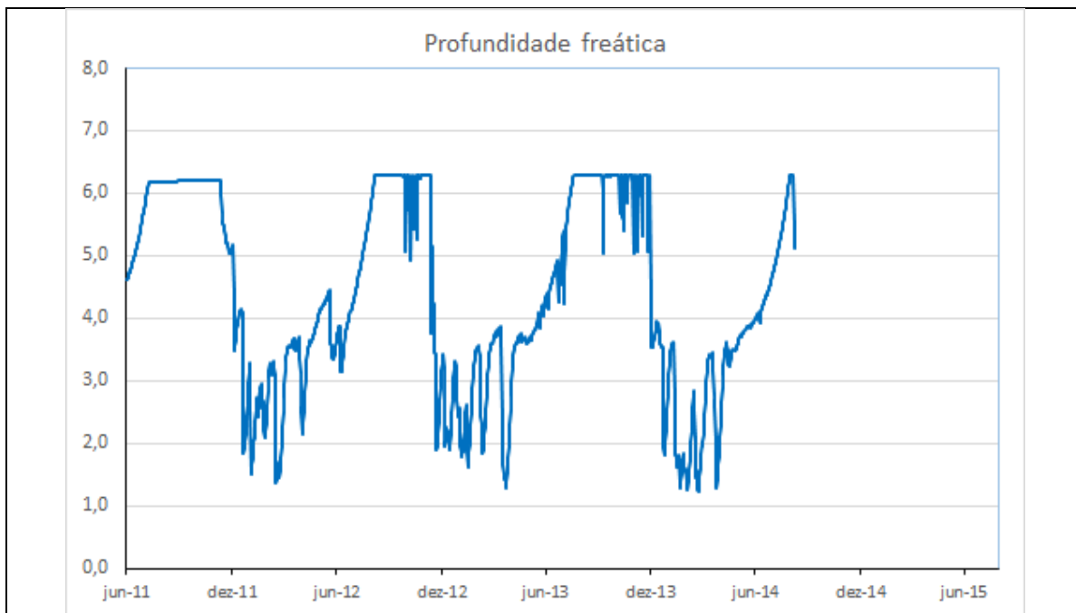
Gráfico 71 - Profundidade freática do PZ-36 do período de 01/06/2011 a 27/09/2014.
