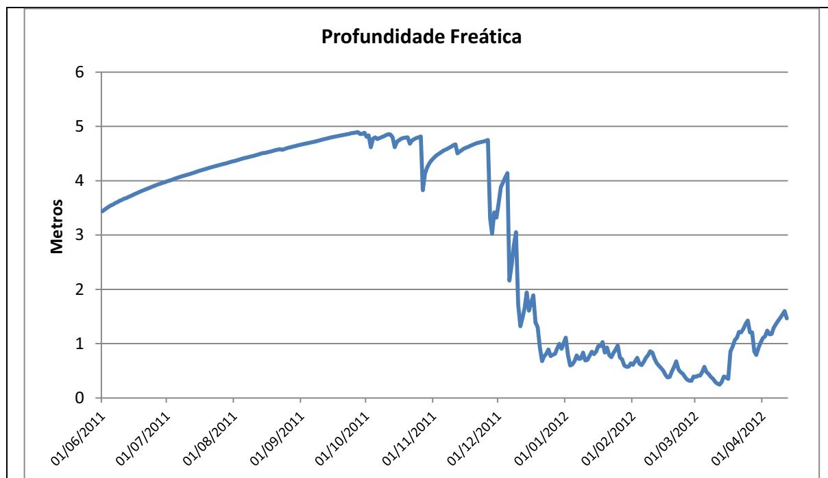
Gráfico 15 - Profundidade freática do PZ-08 do período de 01/06/2011 a 01/04/2012
