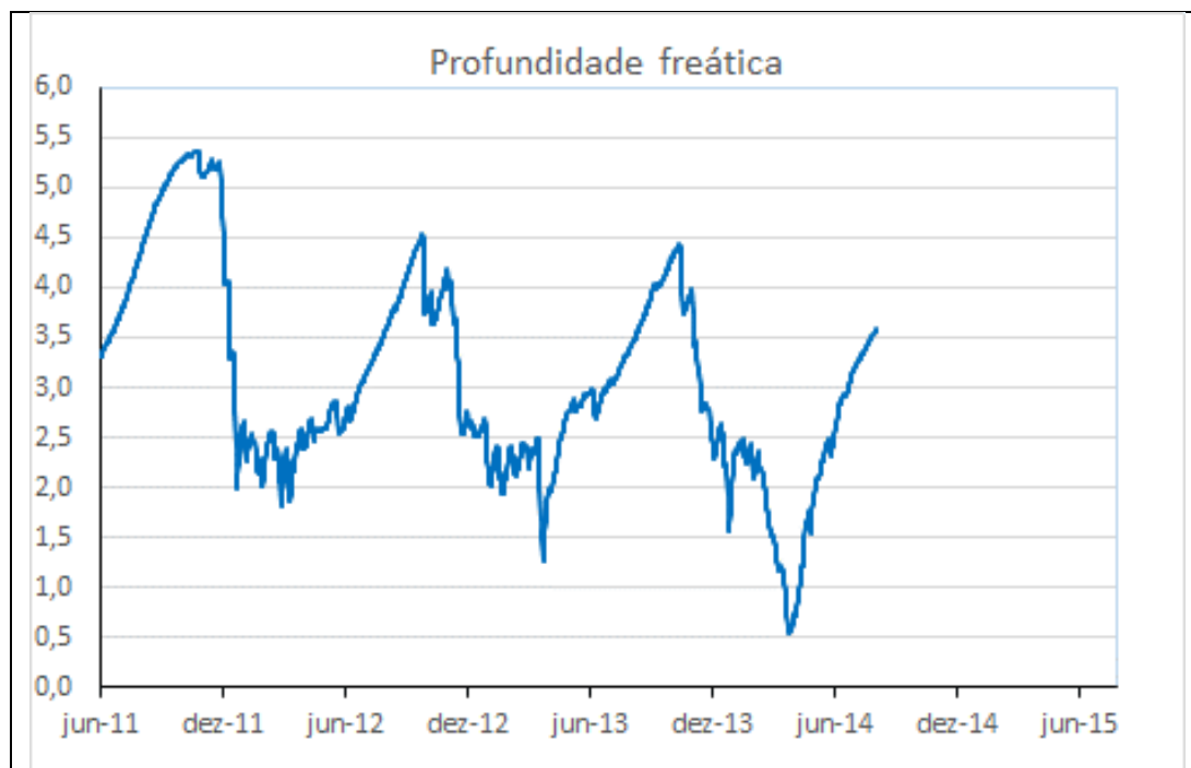
Gráfico 23 - Profundidade freática do PZ-12 do período de 01/06/2011 a 02/08/2014.
