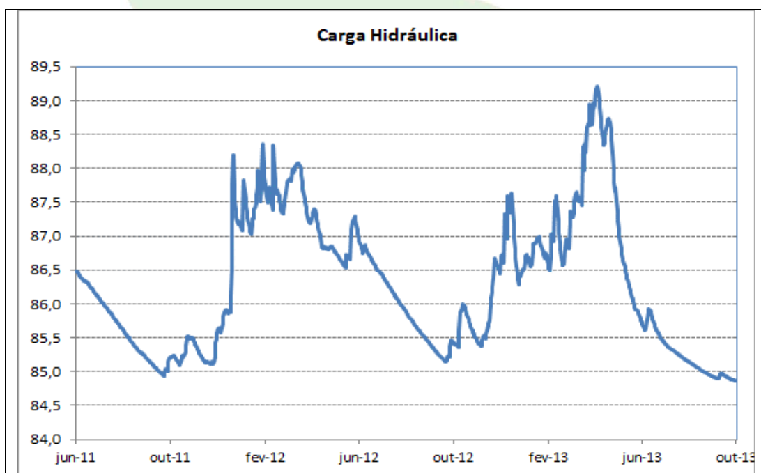
Gráfico 30 - Carga hidráulica do PZ-15 no período de 01/06/2011 a 01/10/2013.
