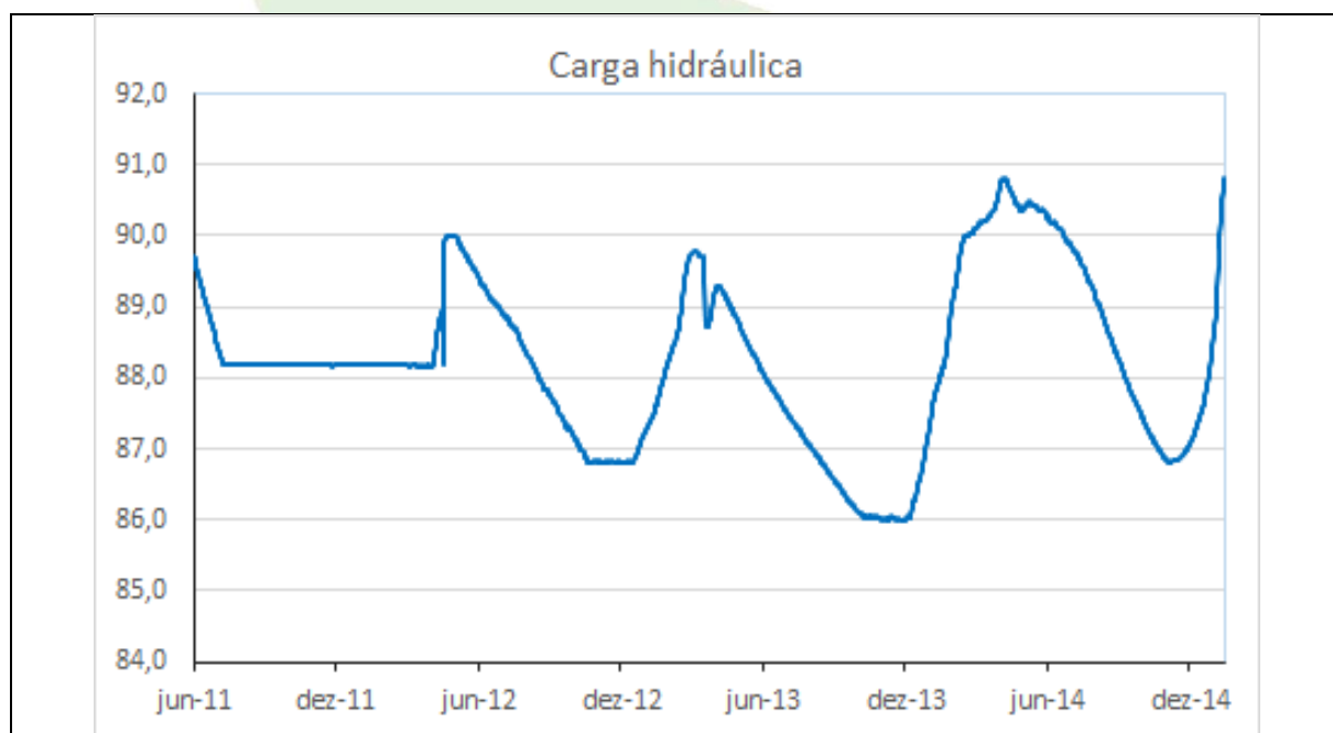
Gráfico 90 - Carga hidráulica do PZ-45 no período de 01/06/2011 a 14/01/2015.
