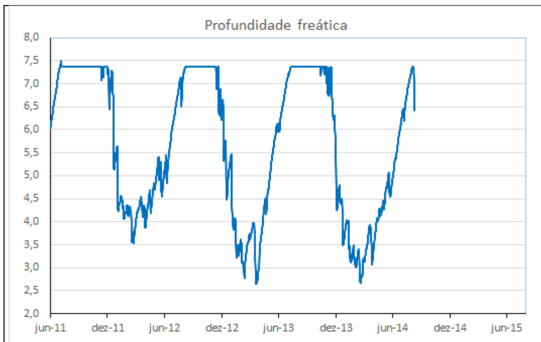
Gráfico 73 - Profundidade freática do PZ-37 do período de 01/06/2011 a 27/09/2014.
