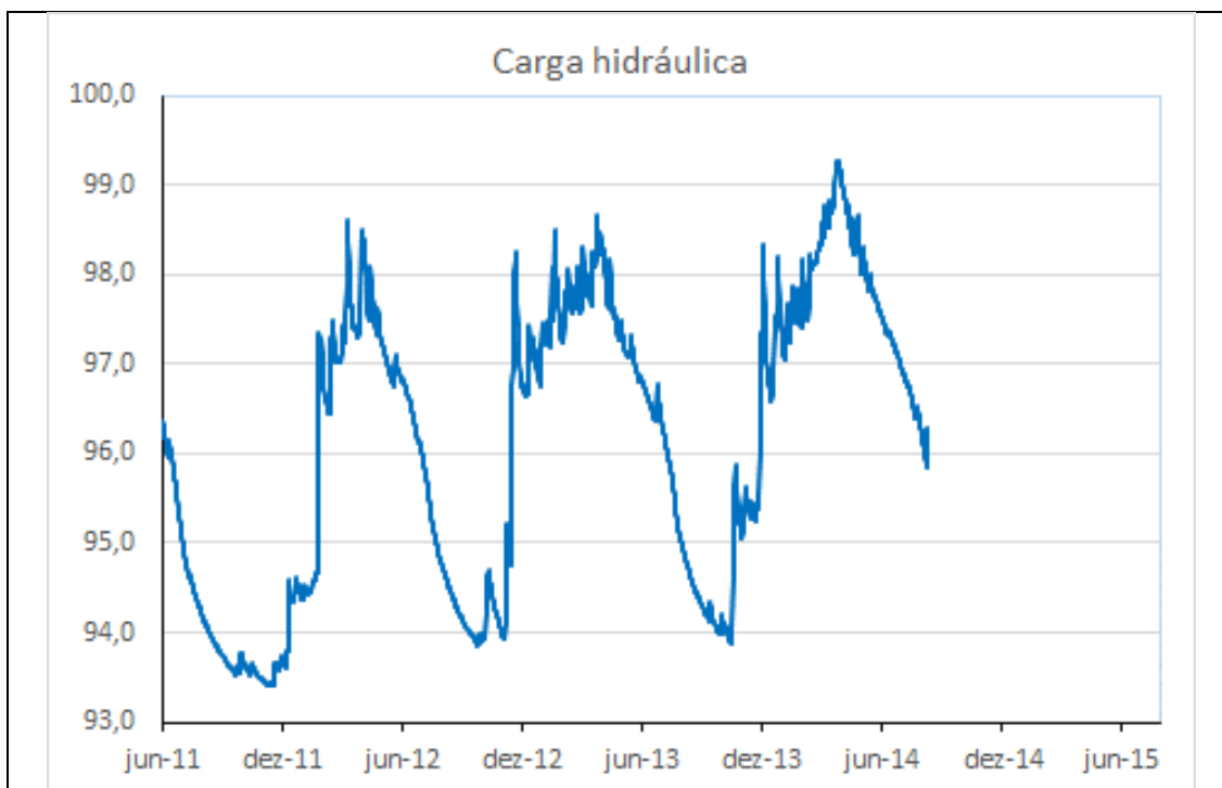
Gráfico 9 - Profundidade freática do PZ-05 do período de 01/06/2011 a 28/07/2015.
