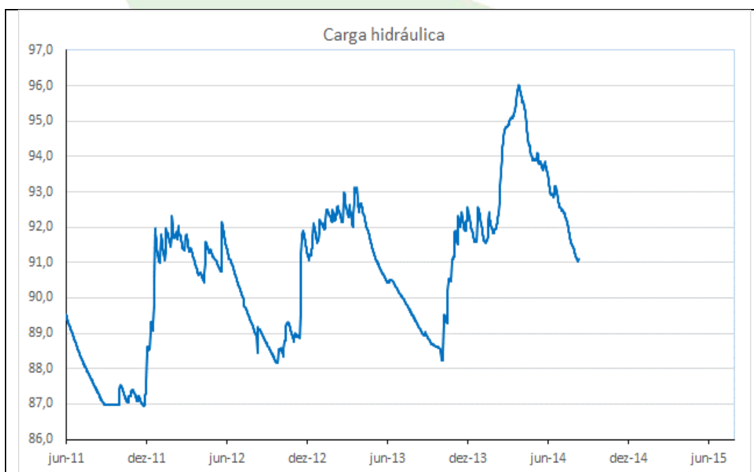
Gráfico 42 - Carga hidráulica do PZ-21 no período de 01/06/2011 a 10/08/2014.
