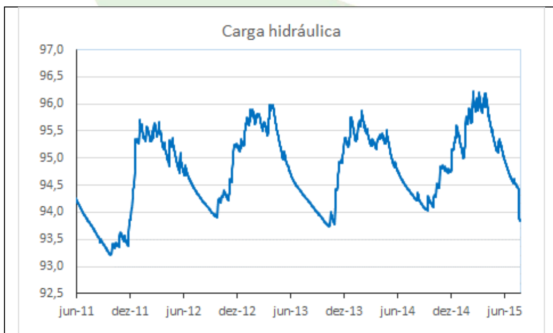
Gráfico 14 - Carga hidráulica do PZ-07 no período de 01/06/2011 a 26/07/2015.
