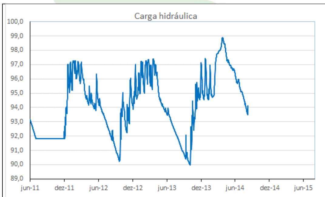
Gráfico 36 - Carga hidráulica do PZ-18 no período de 01/06/2011 a 01/08/2014
