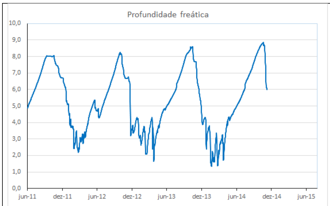
Gráfico 85 - Profundidade freática do PZ-43 do período de 01/06/2011 a 07/11/2014.
