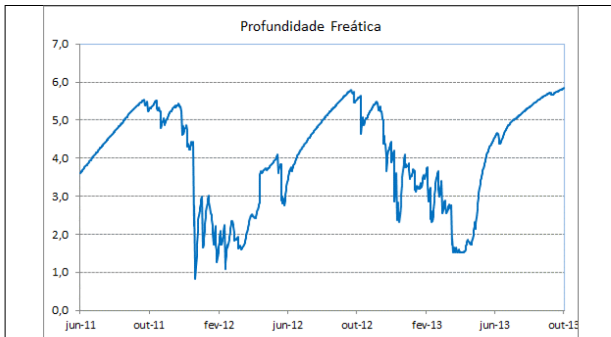
Gráfico 51 - Profundidade freática do PZ-26 do período de 01/06/2011 a 01/10/2013.
