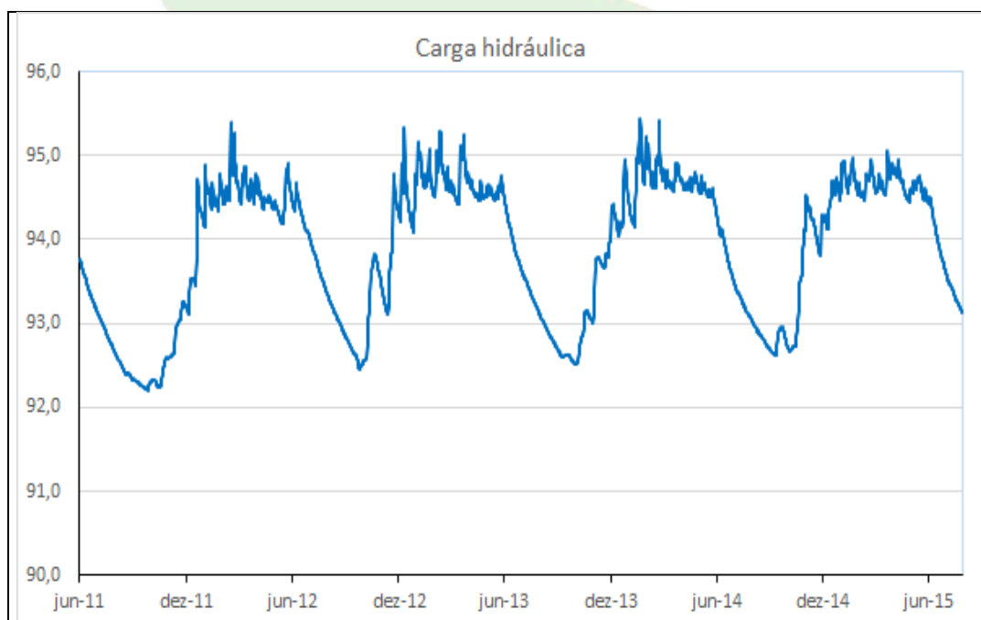
Gráfico 82 - Carga hidráulica do PZ-41 no período de 01/06/2011 a 28/07/2015.
