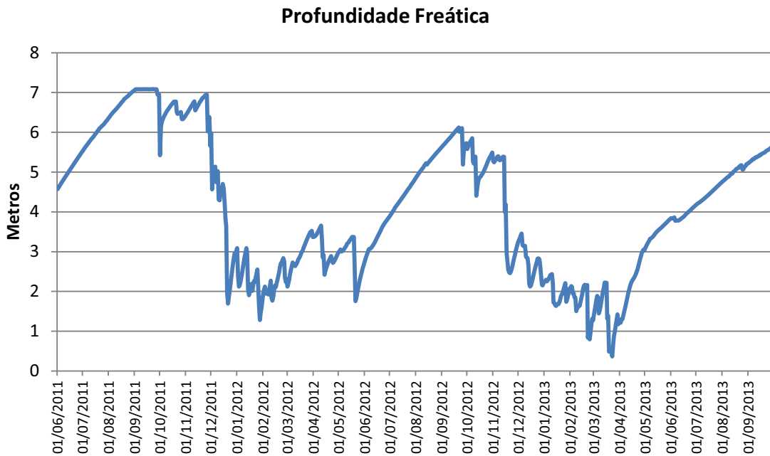
Gráfico 33 - Profundidade freática do PZ-17 do período de 01/06/2011 a 01/09/2013
