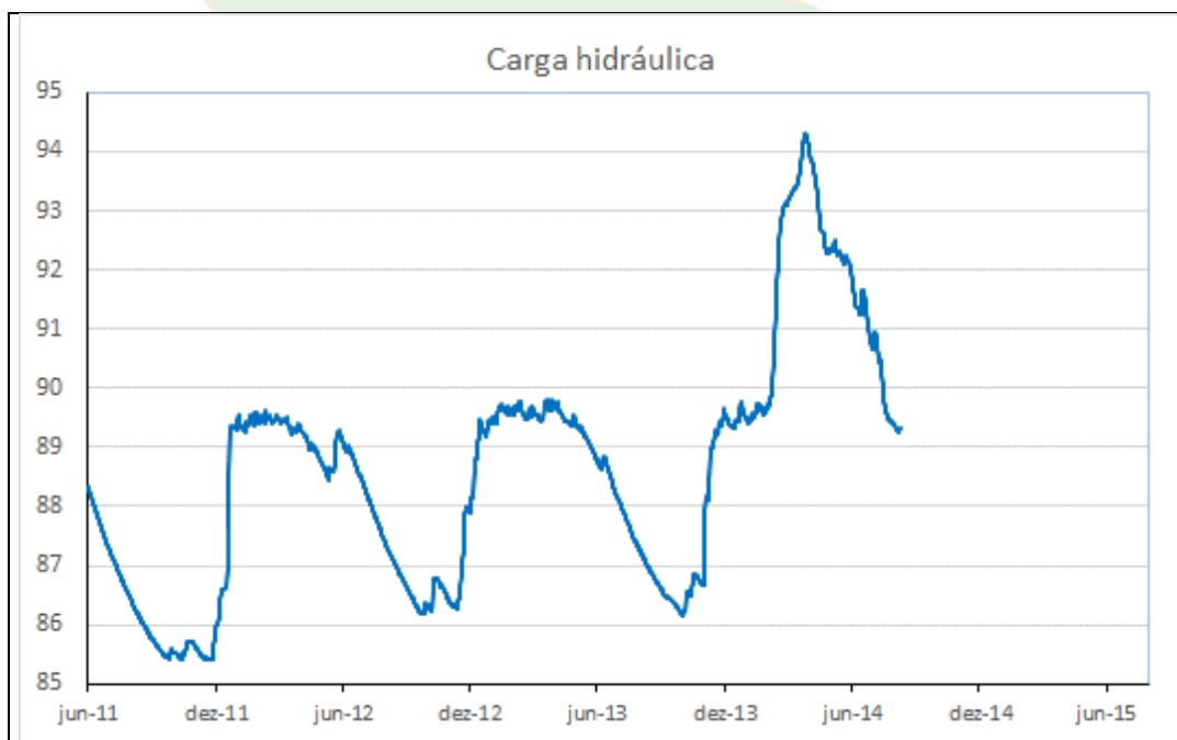
Gráfico 28 - Carga hidráulica do PZ-14 no período de 01/06/2011 a 09/08/2014.
