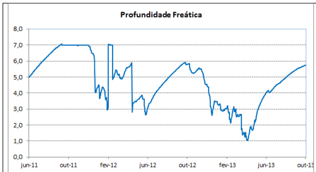
Gráfico 31 - Profundidade freática do PZ-16 do período de 01/06/2011 a 01/10/2013.
