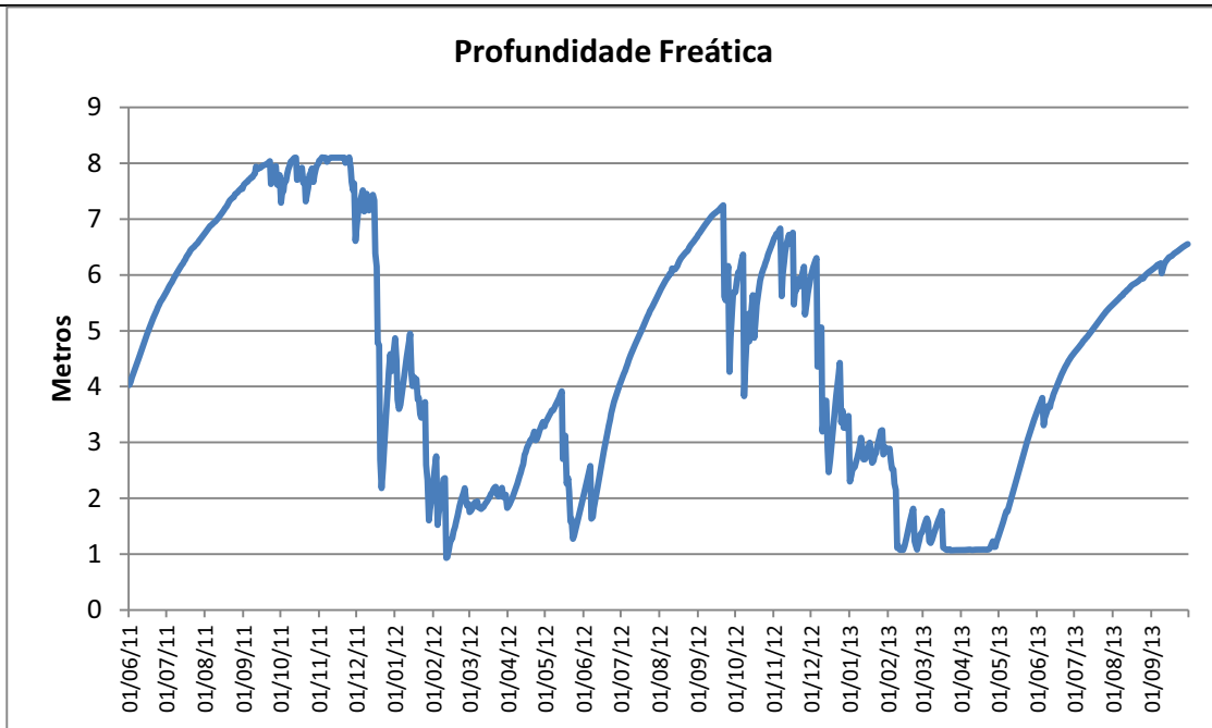
Gráfico 43 - Profundidade freática do PZ-22 do período de 01/06/2011 a 01/09/2013
