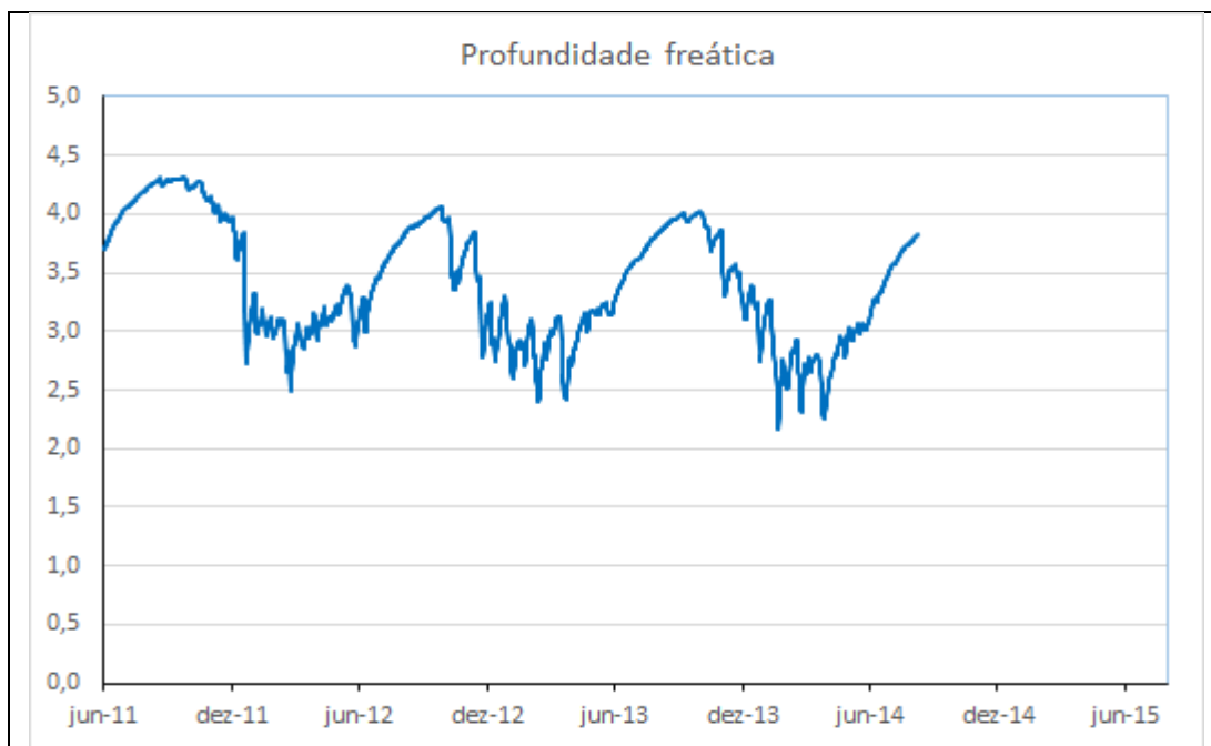
Gráfico 79 - Profundidade freática do PZ-40 do período de 01/06/2011 a 10/08/2014.
