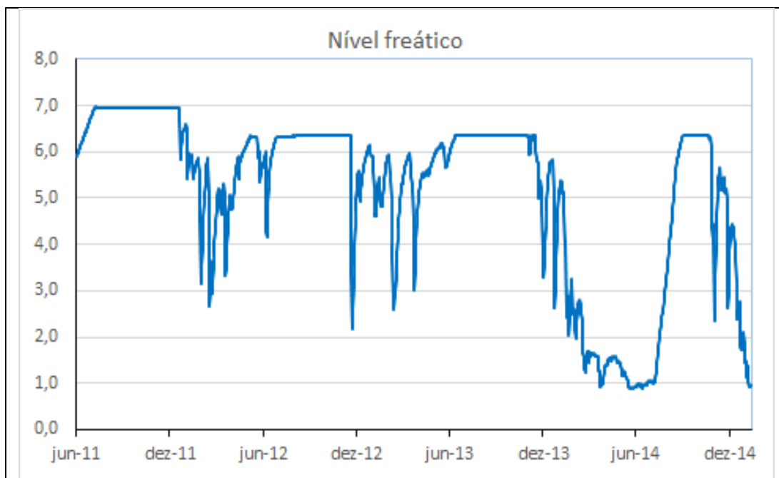
Gráfico 83 - Profundidade freática do PZ-42 do período de 01/06/2011 a 13/01/2015.
