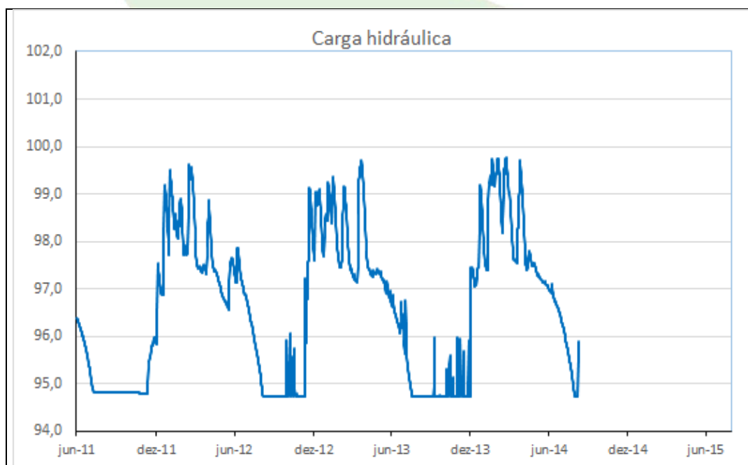
Gráfico 64 - Carga hidráulica do PZ-32 no período de 01/06/2011 a 27/09/2014.
