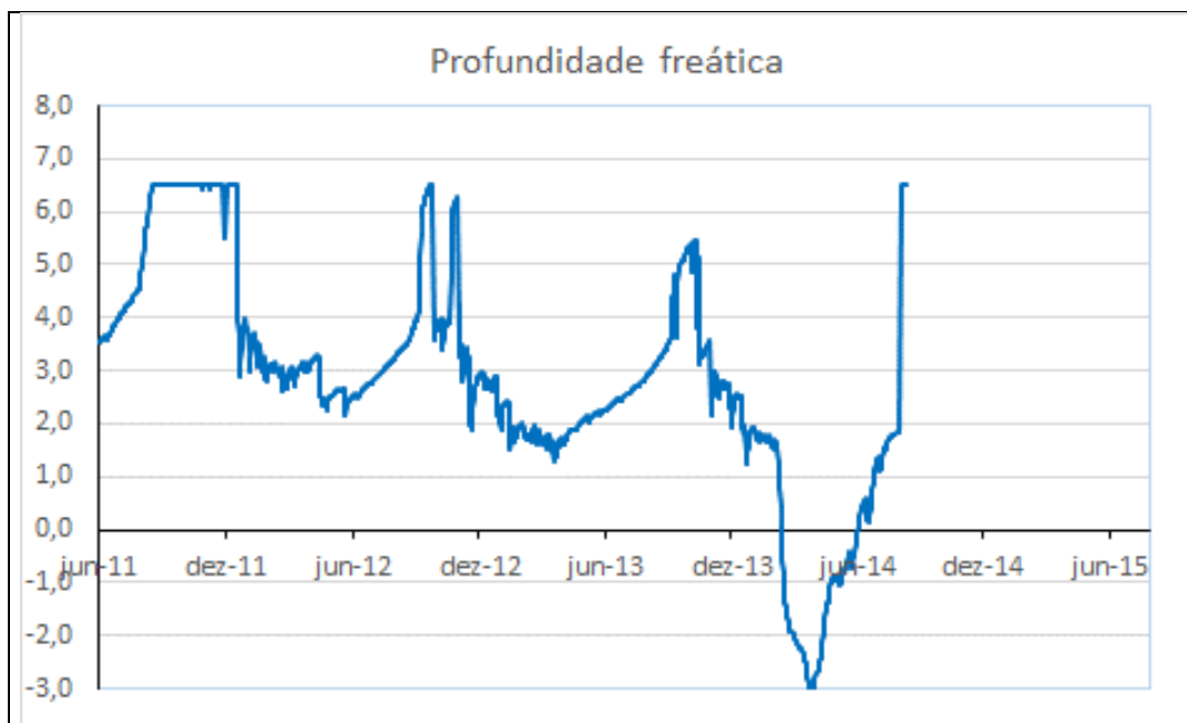
Gráfico 17 - Profundidade freática do PZ-09 do período de 01/06/2011 a 02/08/2014.
