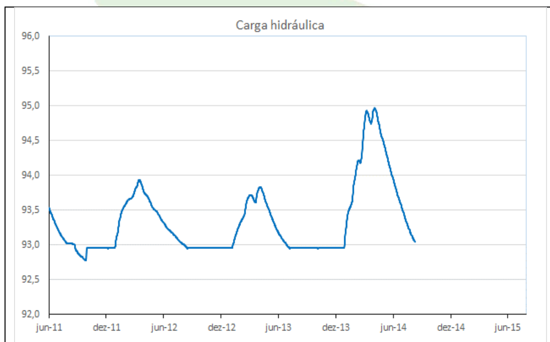
Gráfico 54 - Carga hidráulica do PZ-27 no período de 01/06/2011 a 09/08/2014.
