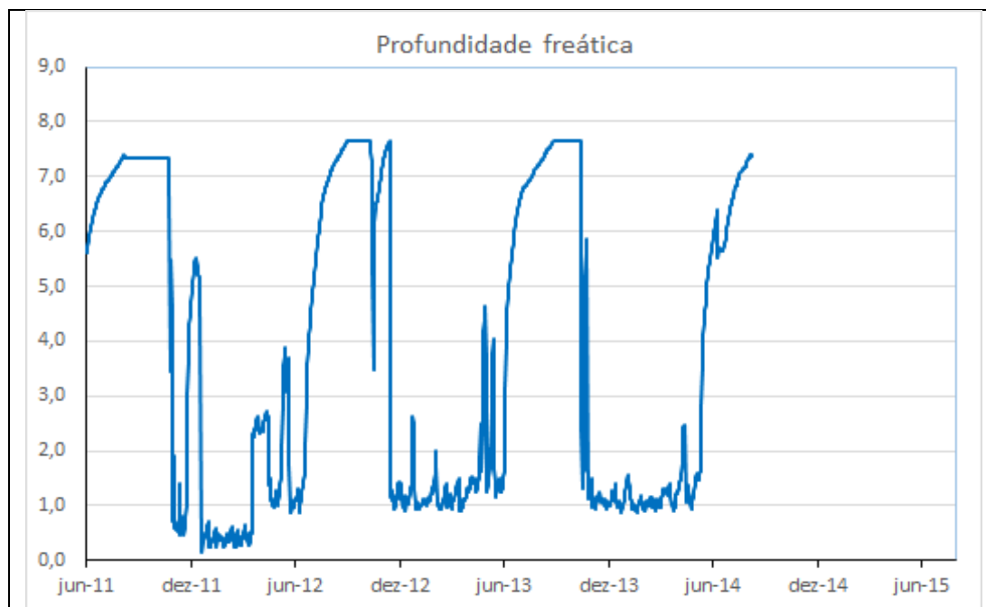
Gráfico 77 - Profundidade freática do PZ-39 do período de 01/06/2011 a 09/08/2014.
