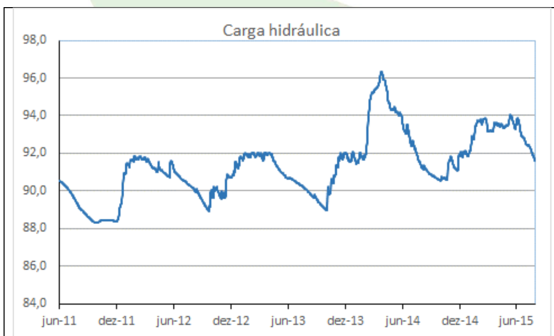
Gráfico 40 - Carga hidráulica do PZ-20 no período de 01/06/2011 a 28/07/2015.
