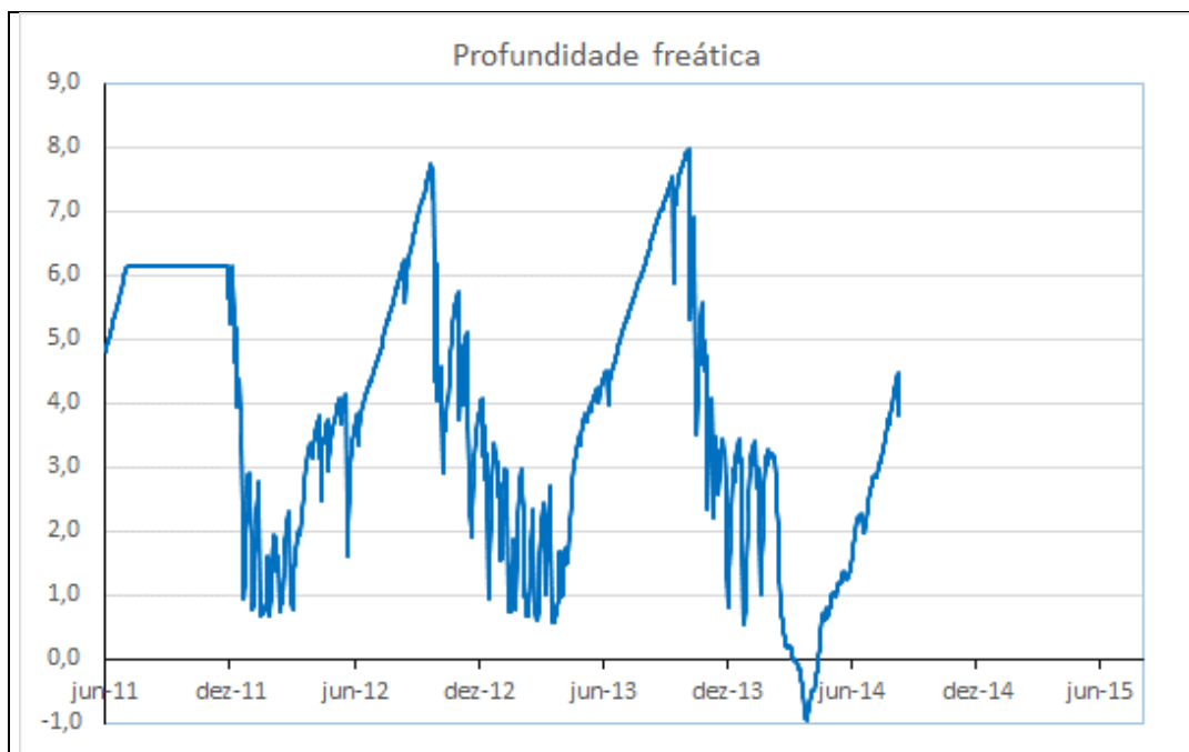
Gráfico 35 - Profundidade freática do PZ-18 do período de 01/06/2011 a 10/08/2014.
