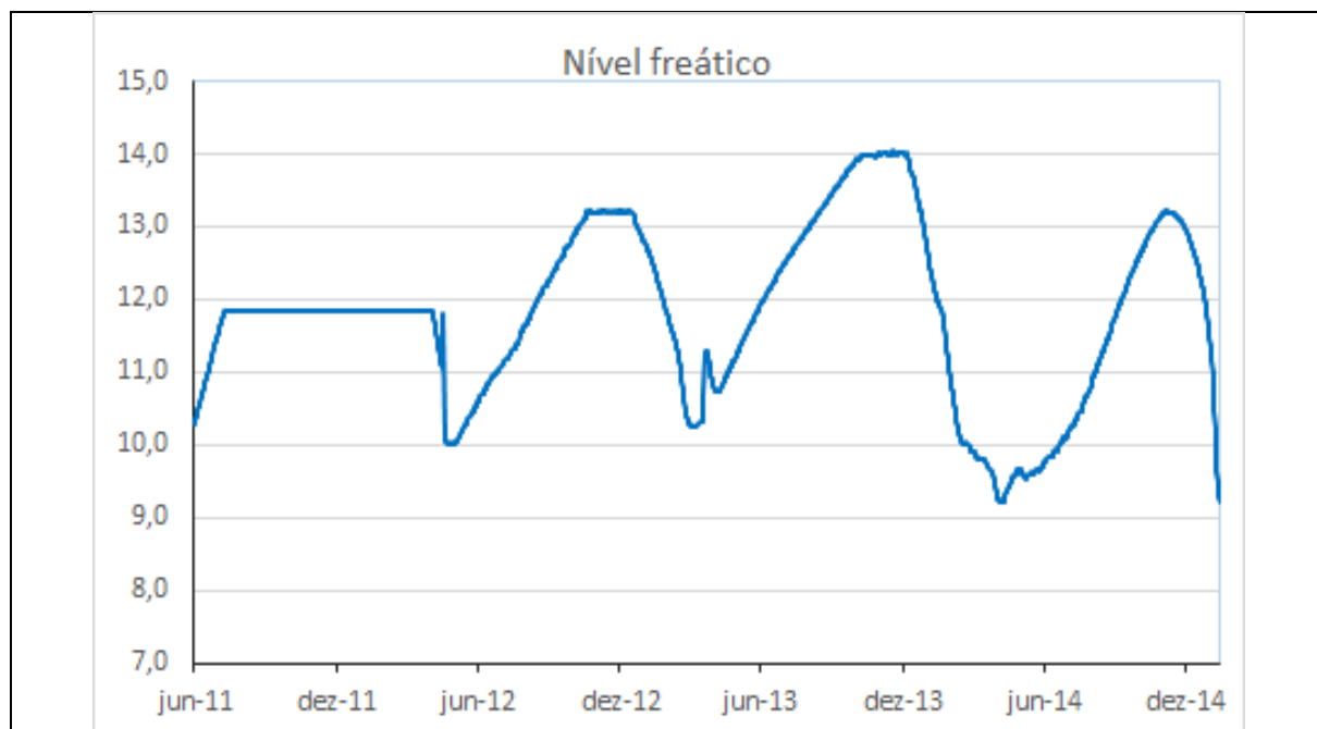
Gráfico 89 - Carga hidráulica do PZ-45 no período de 01/06/2011 a 14/01/2015.
