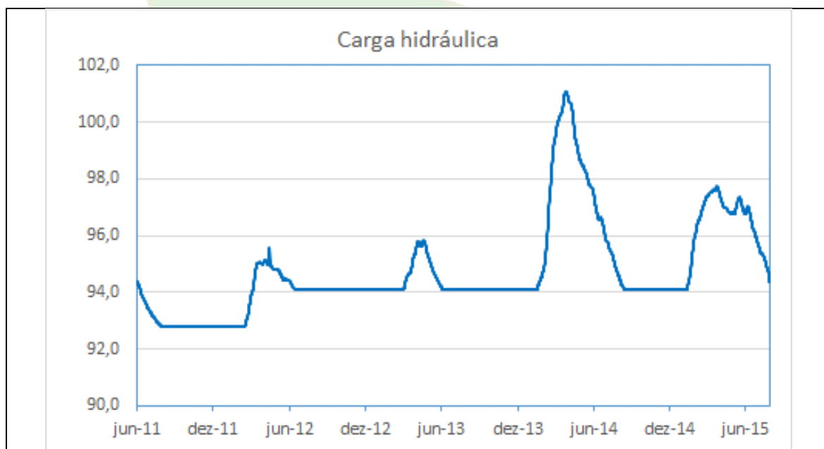
Gráfico 2 - Carga hidráulica do PZ-01 do período de 01/06/2011 a 27/07/2015.
