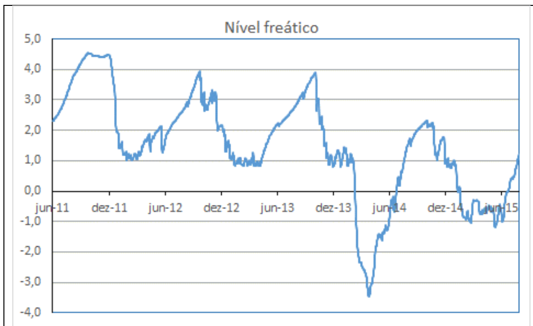
Gráfico 39 - Profundidade freática do PZ-20 do período de 01/06/2011 a 28/07/2015.
