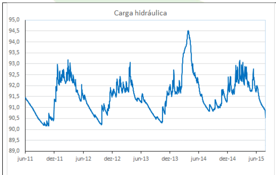
Gráfico 22 - Carga hidráulica do PZ-11 no período de 01/06/2011 a 27/07/2015.
