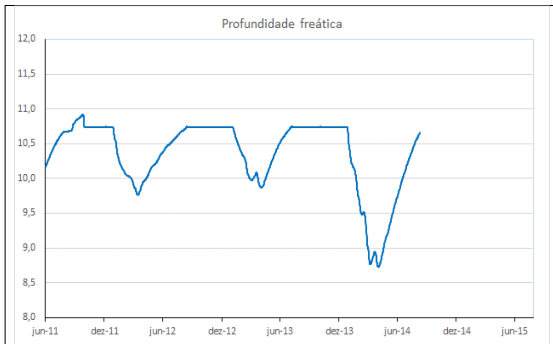
Gráfico 53 - Profundidade freática do PZ-27 do período de 01/06/2011 a 09/08/2014.
