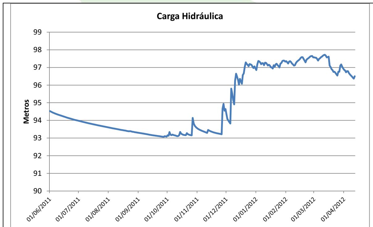
Gráfico 16 - Carga hidráulica do PZ-08 no período de 01/06/2011 a 01/04/2012
