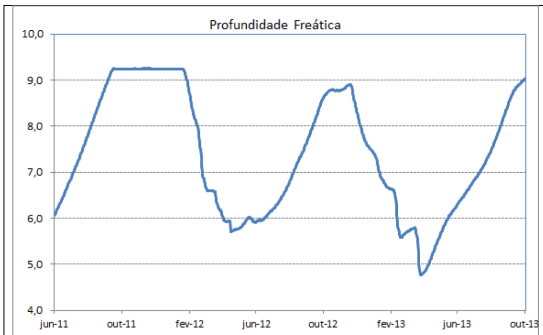
Gráfico 67 - Profundidade freática do PZ-34 do período de 01/06/2011 a 01/10/2013.
