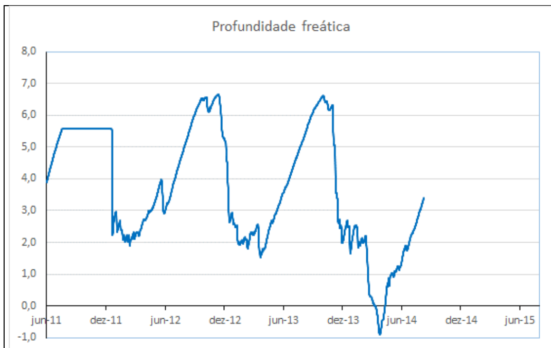
Gráfico 25 - Profundidade freática do PZ-13 do período de 01/06/2011 a 09/08/2014.
