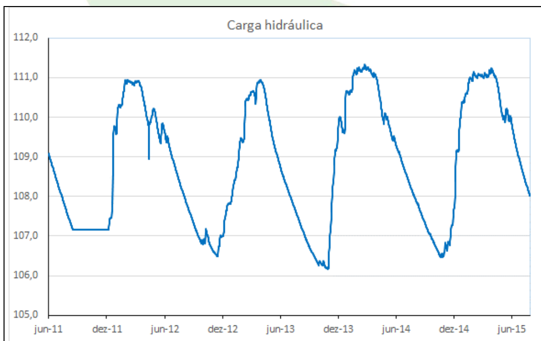
Gráfico 50 - Carga hidráulica do PZ-25 no período de 01/06/2011 a 29/07/2015.
