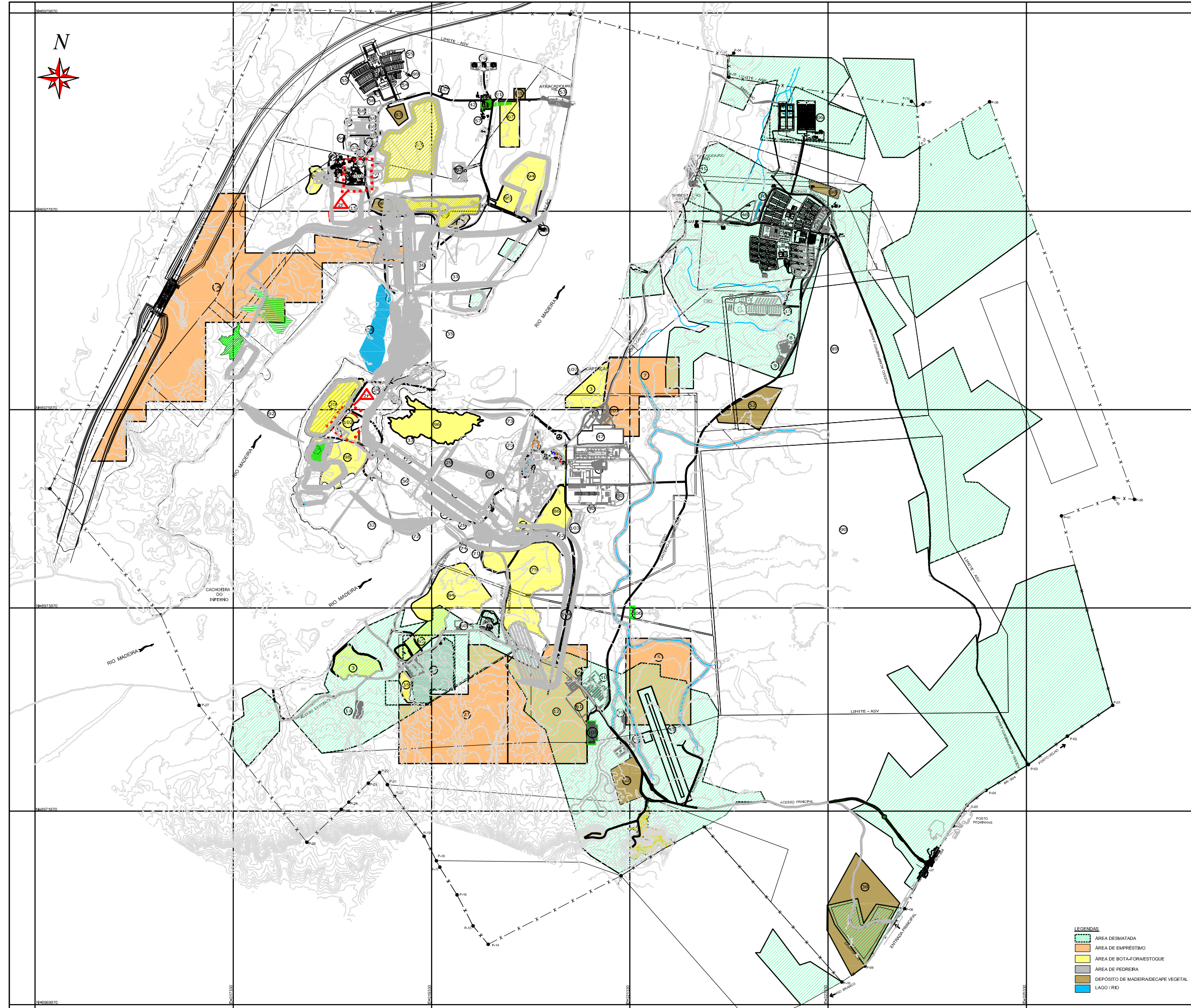
PLANTA BAIXA ESC. 1/13000
