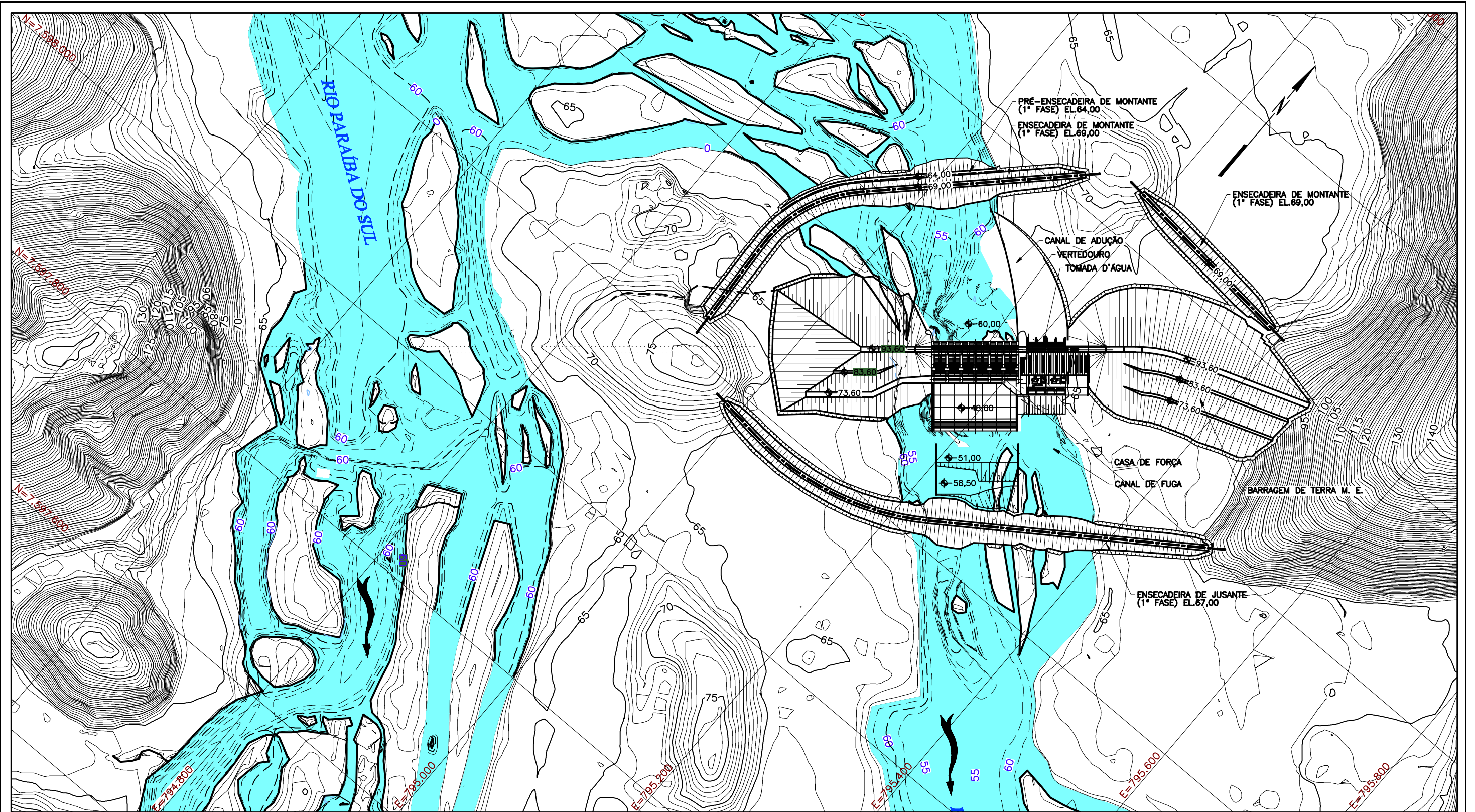
PLANTA ESC.1:4000
