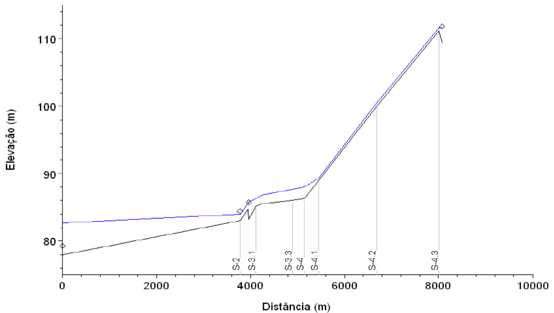
Figura 4.41 - Perfis de Linha D'Água Observado em 14/02/2.009 no Rio Pitapetinga e Simulado.
