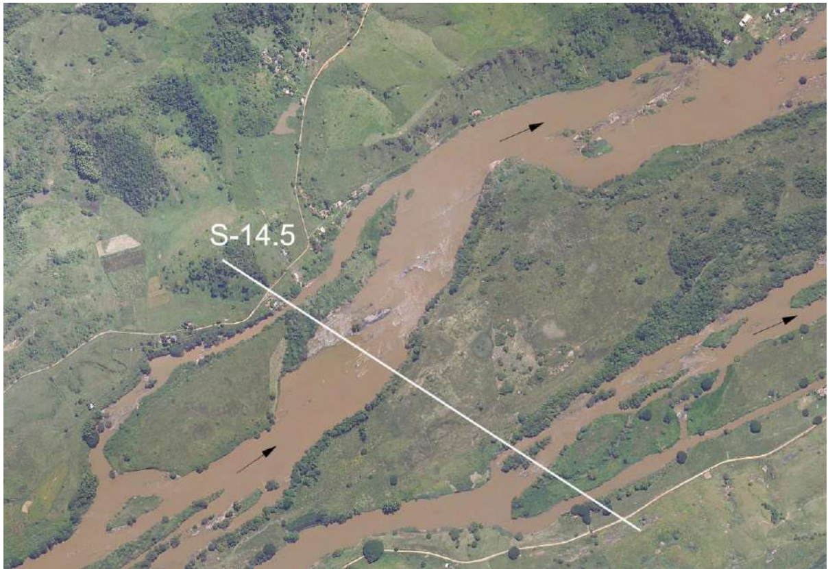
Figura 4.1 - Seção Topobatimétrica S-14.5.
