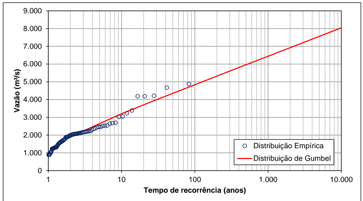
Figura 4.10 - Resultado do Ajuste das Amostras à Distribuição de Gumbel.
