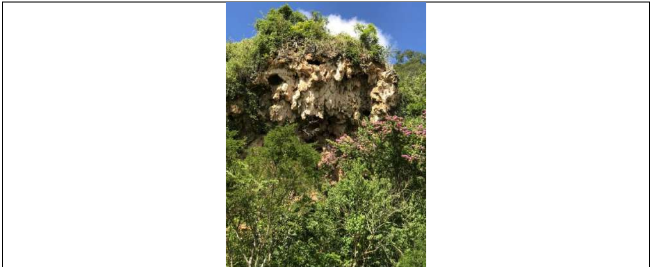
Figura 60: Presença de cavidade em mármore calcítico na Serra do Cândido.
