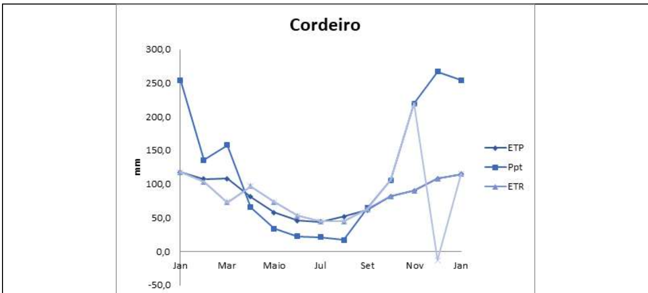
Figura 89: Balanço Hídrico Climatológico da estação Cordeiro. Elaboração própria a partir de dados do INMET [s.d.].
