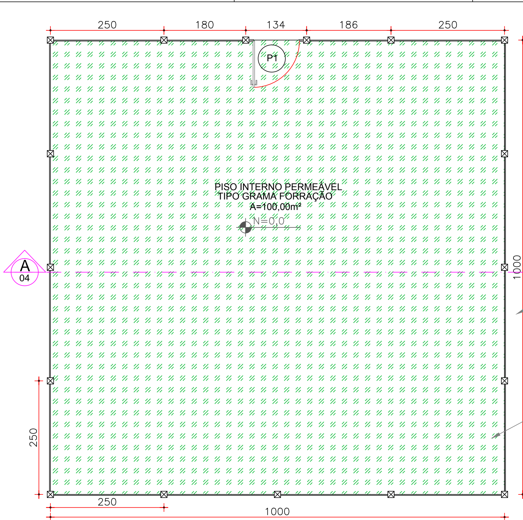
01 PLANTA BAIXA ESC: 1/50
