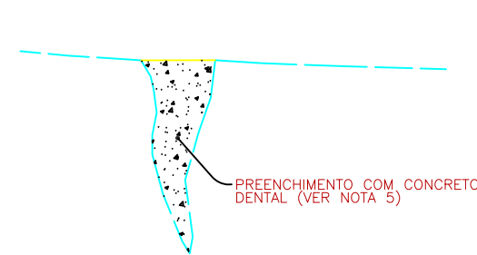
REENTRÂNCIAS, FENDAS OU DESCONTINUIDADES ABERTAS SEM ESC.
