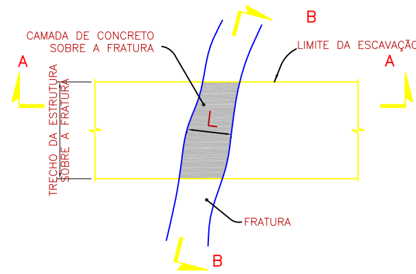
TRATAMENTO DE FRATURAS DE GRANDE PORTE OU FAIXA SUBVERTICAL INTENSAMENTE FRATURADA OU ALTERADA PLANTA ESQUEMÁTICA SEM ESC.
