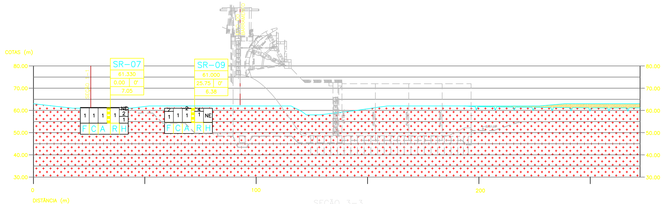
PERFIL TRANSVERSAL PELO BARRAMENTO ESCALA 1:1000
