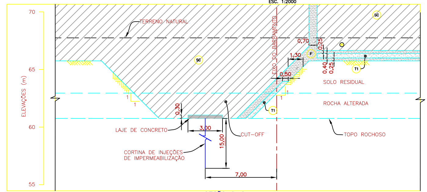
SEÇÃO 2-2 ESC. 1:200
