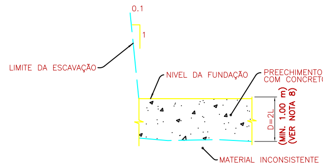
TRATAMENTO DE FRATURAS DE GRANDE PORTE SEÇÃO A-A SEM ESC.
