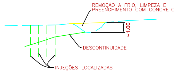
DESCONTINUIDADE DE PEQUENO MERGULHO SEM ESC.
