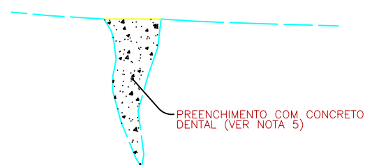
REENTRÂNCIAS, FENDAS OU DESCONTINUIDADES ABERTAS SEM ESC.
