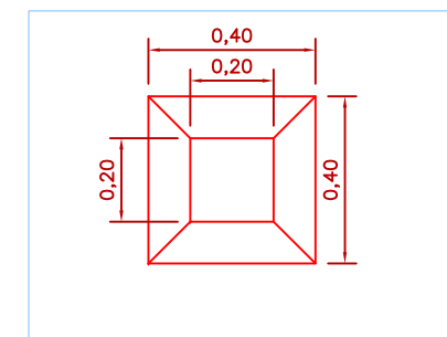
DETALHE DA PROTEÇÃO DA CABEÇA DOS TIRANTES ESC. 1:20
