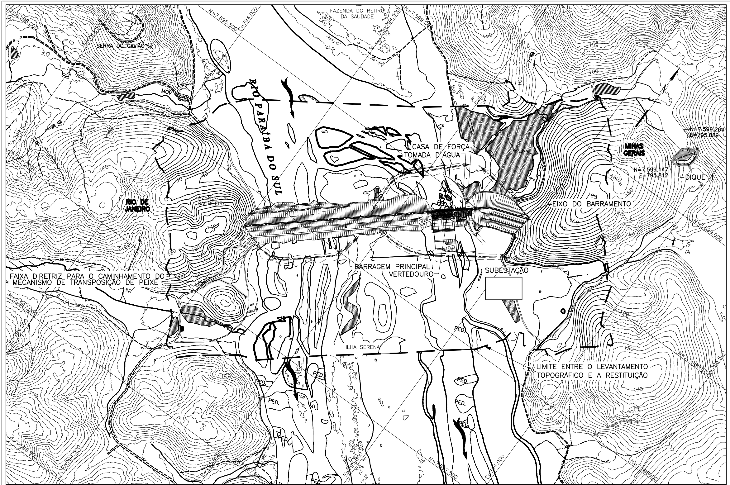
PLANTA
