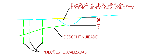
DESCONTINUIDADE DE PEQUENO MERGULHO SEM ESC.
