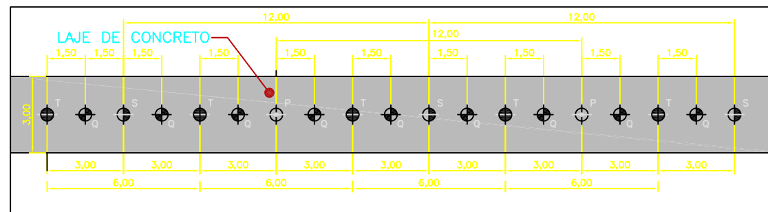
DISTRIBUIÇÃO DOS FUCOS DE INJEÇÃO - DETALHE TÍPICO ESC. 1:200
