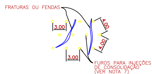
FRATURAS OU FENDAS INJEÇÕES DE CONSOLIDAÇÃO DISPOSIÇÃO TÍPICA EM PLANTA SEM ESC.
