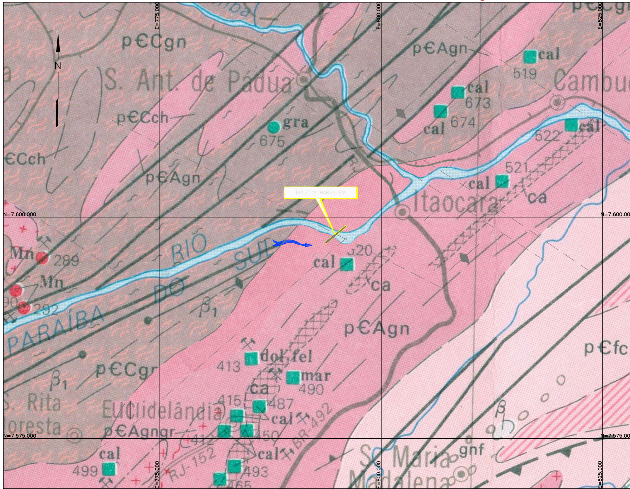
MAPA GEOLÓGICO REGIONAL ESCALA 1:250000
