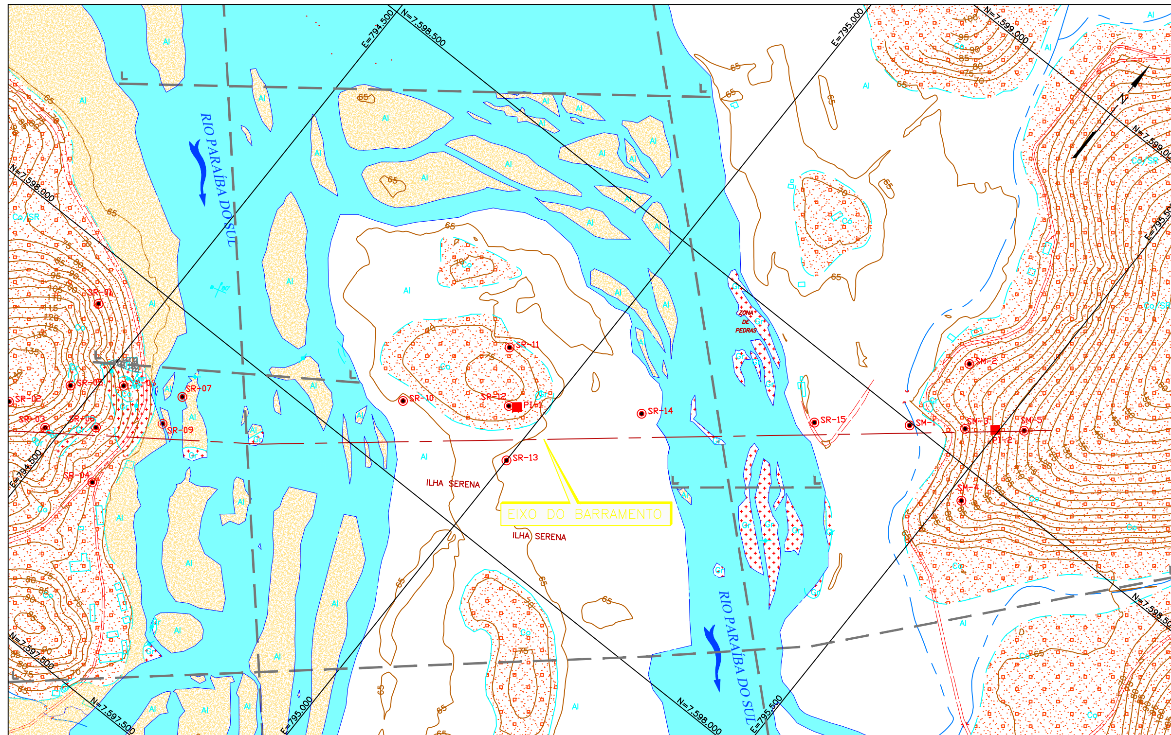
MAPA GEOLÓGICO-GEOTÉCNICO LOCAL ESCALA 1:5000
