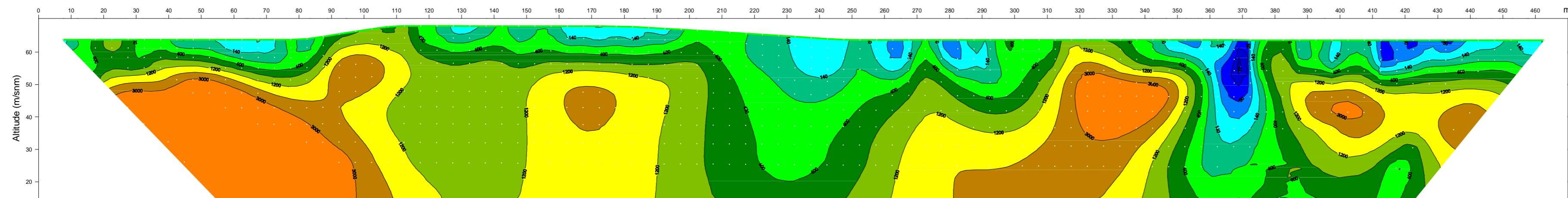
Modelo de resistividade real do terreno
