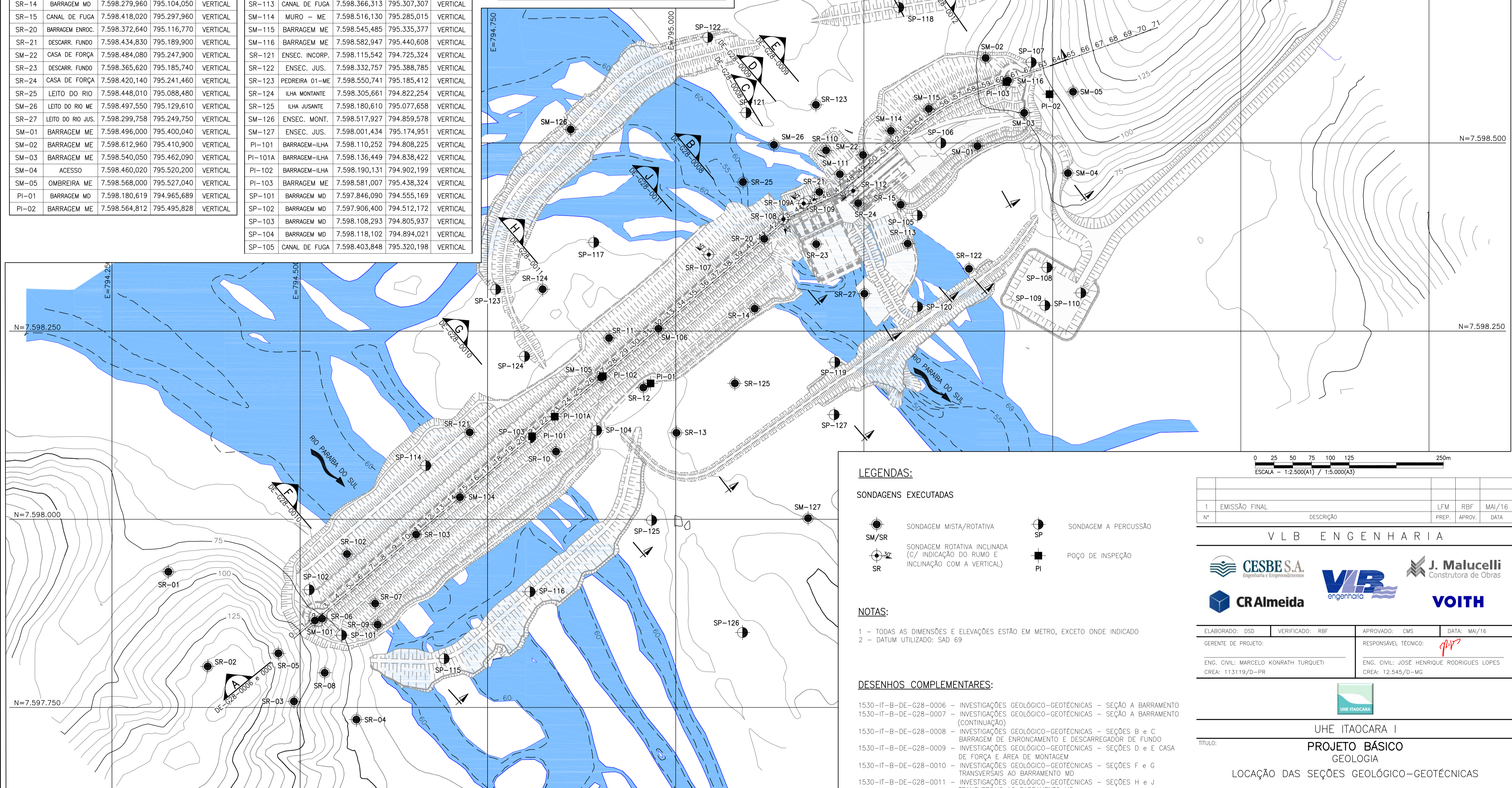
PLANTA
