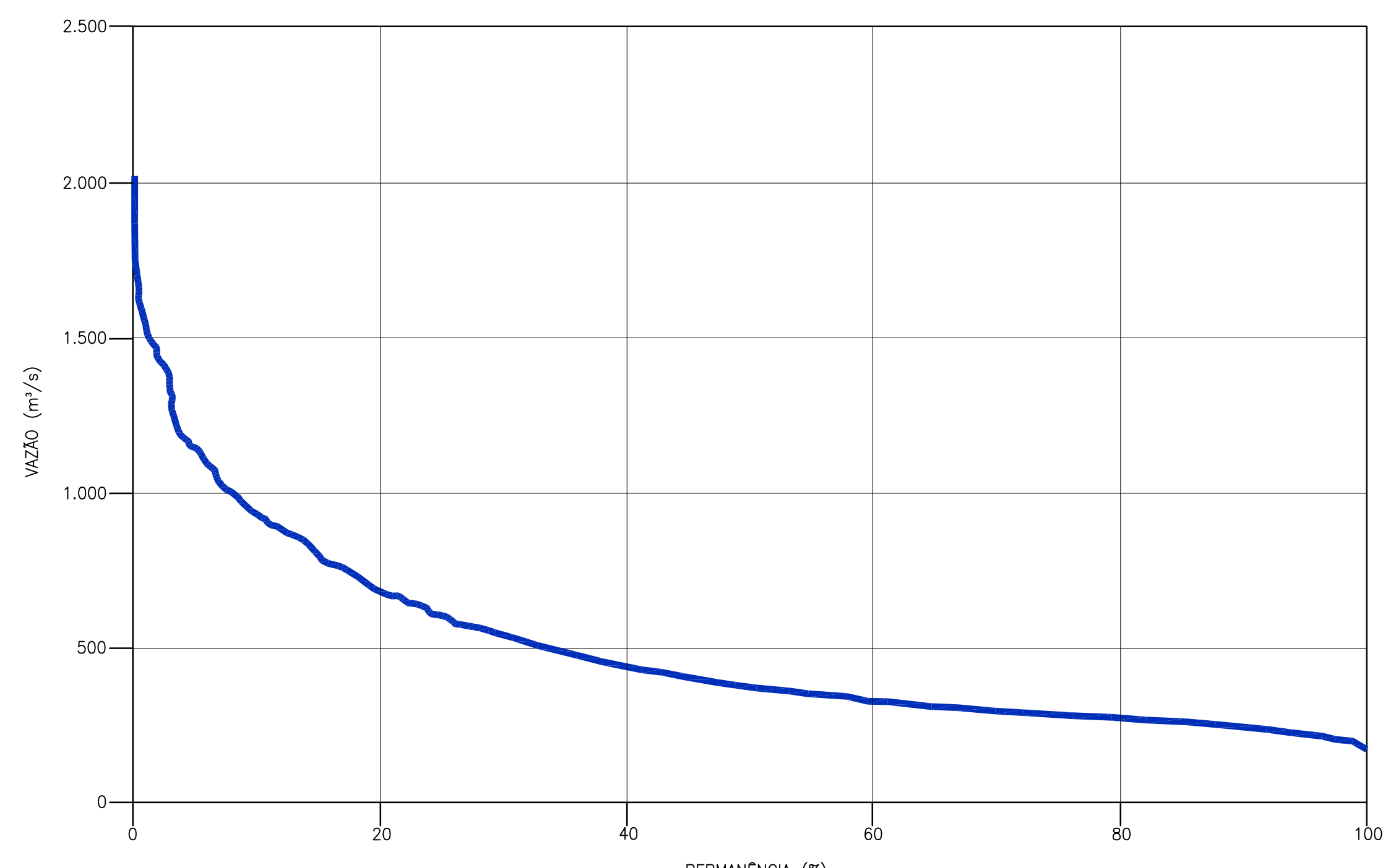
PERMANÊNCIA DE VAZÕES MÉDIAS MENSIS ARTIFICIAIS
