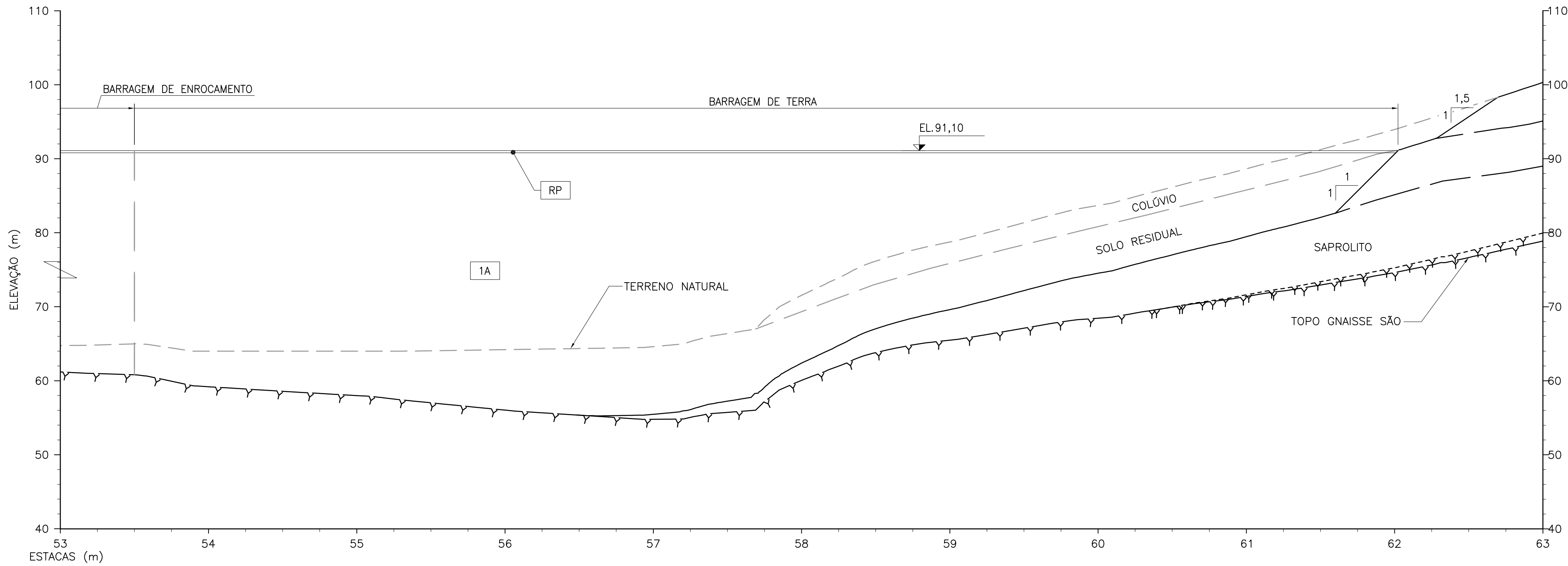
SEÇÃO LONGITUDINAL AO BARRAMENTO ESC.1:400 (CONTINUAÇÃO) B11-0001
