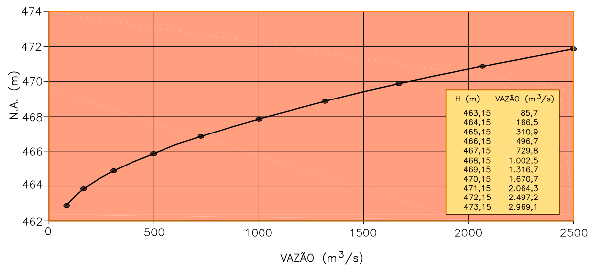
Curva Chave no Canal de Fuga
