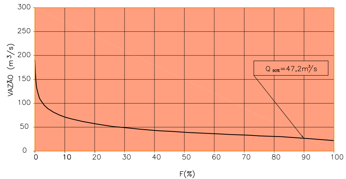
Curva de Permanência – Vazões Médias Diárias Posto: Cachoeira Grande Período: 1963 a 1991
