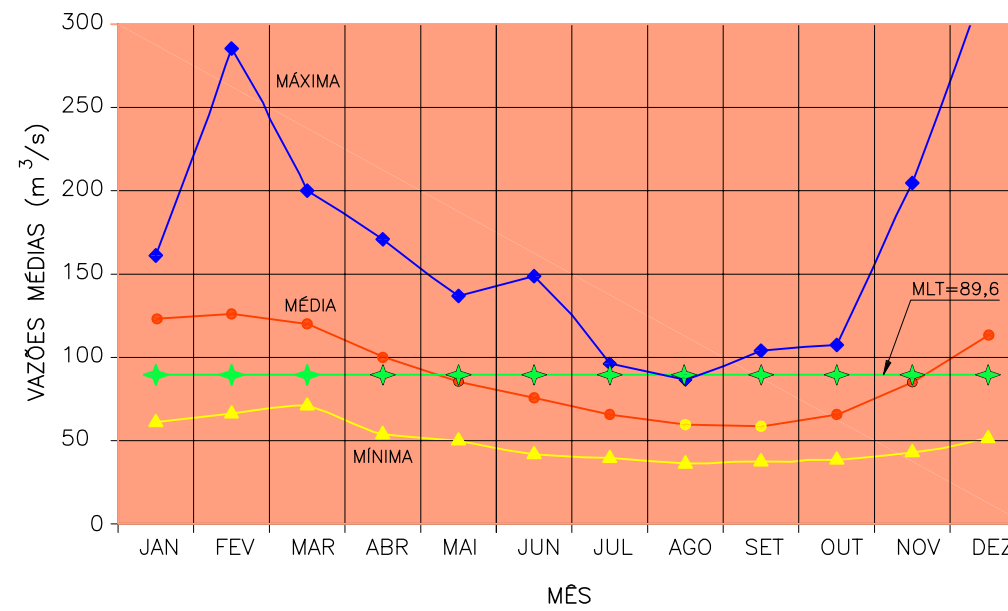
Histograma de Vazões Médias Mensais na Barragem de Couto Magalhães Período: 1931 a 1997
