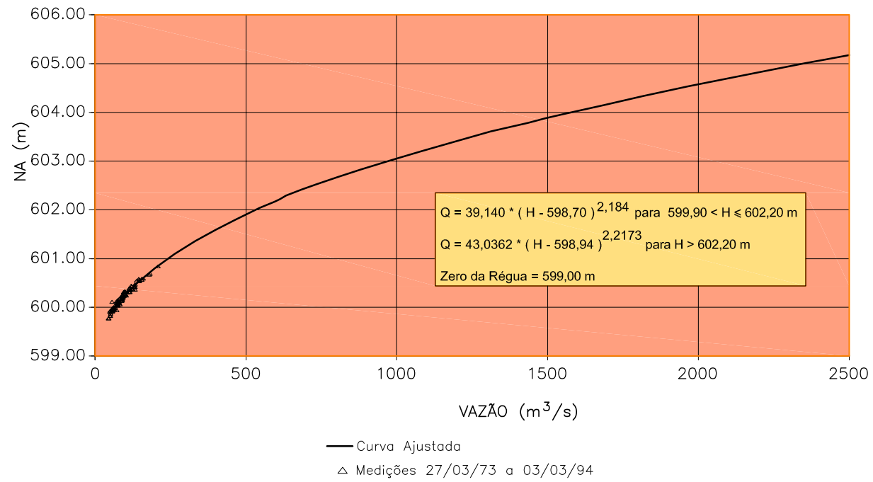
Curva Chave no Local da Barragem
