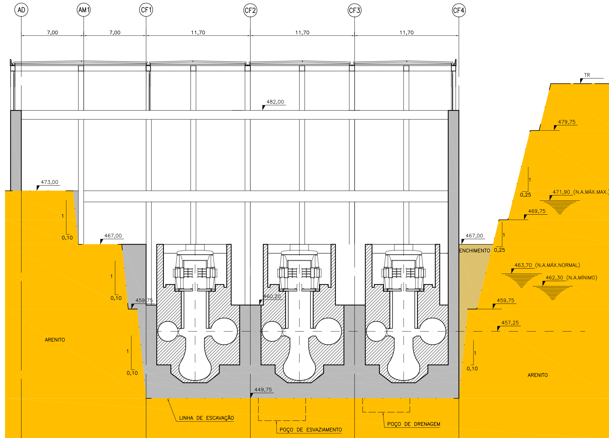
CORTE LONGITUDINAL ESC. 1:250
