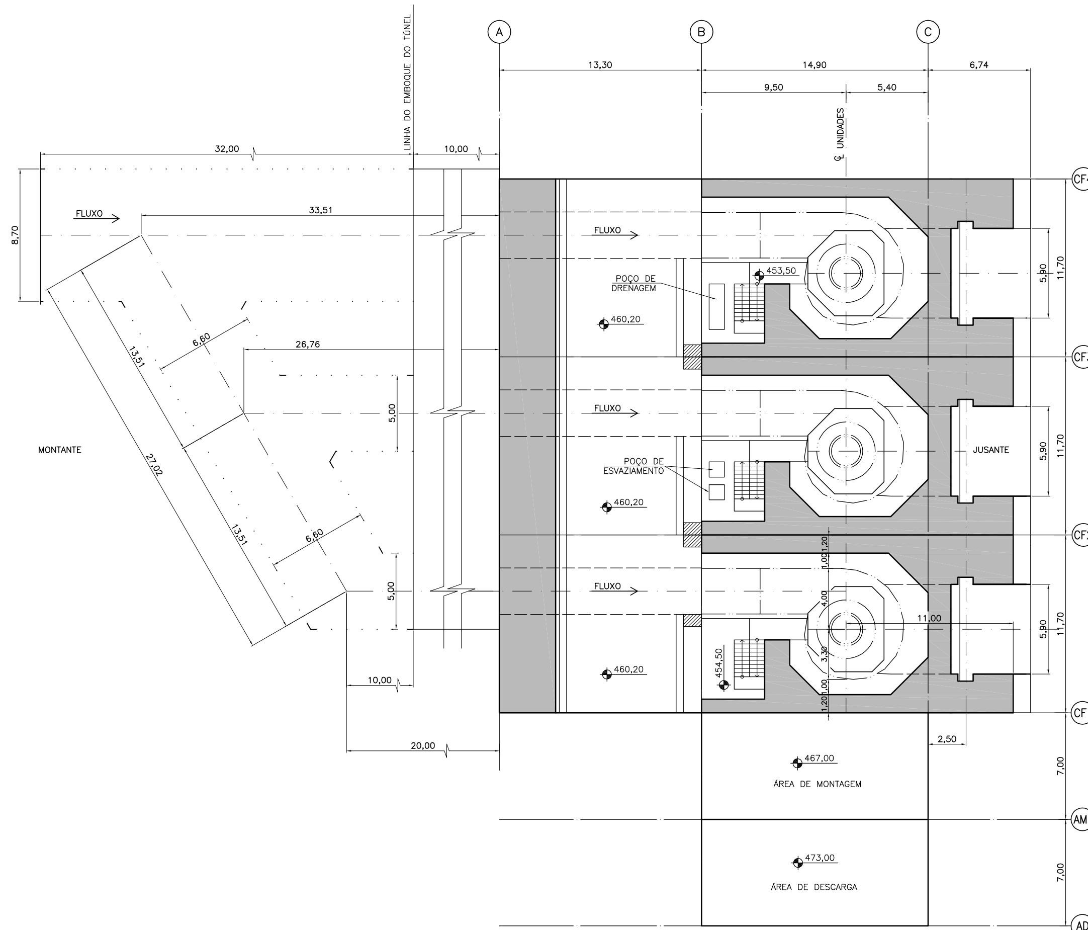
PLANTA EL. 460,20 ESC. 1:250
