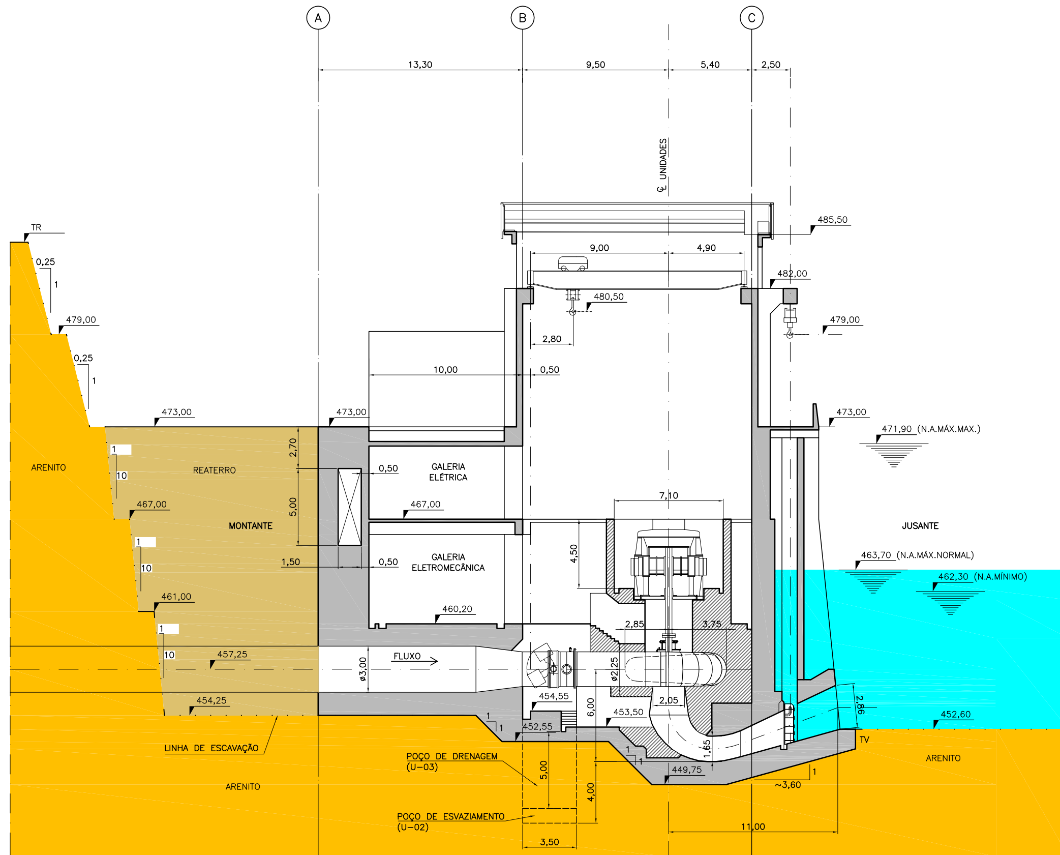
CORTE TRANSVERSAL
