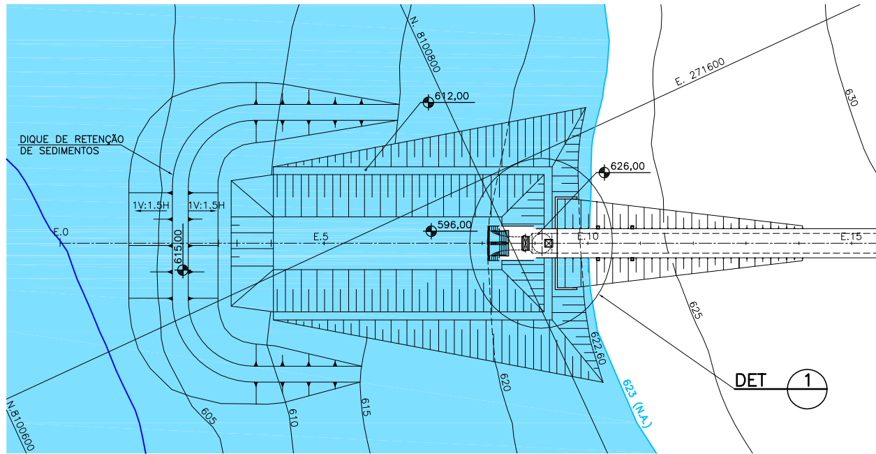
PLANTA 1:2000
