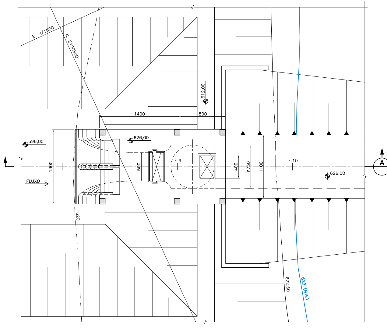
DETALHE 1 1:400
