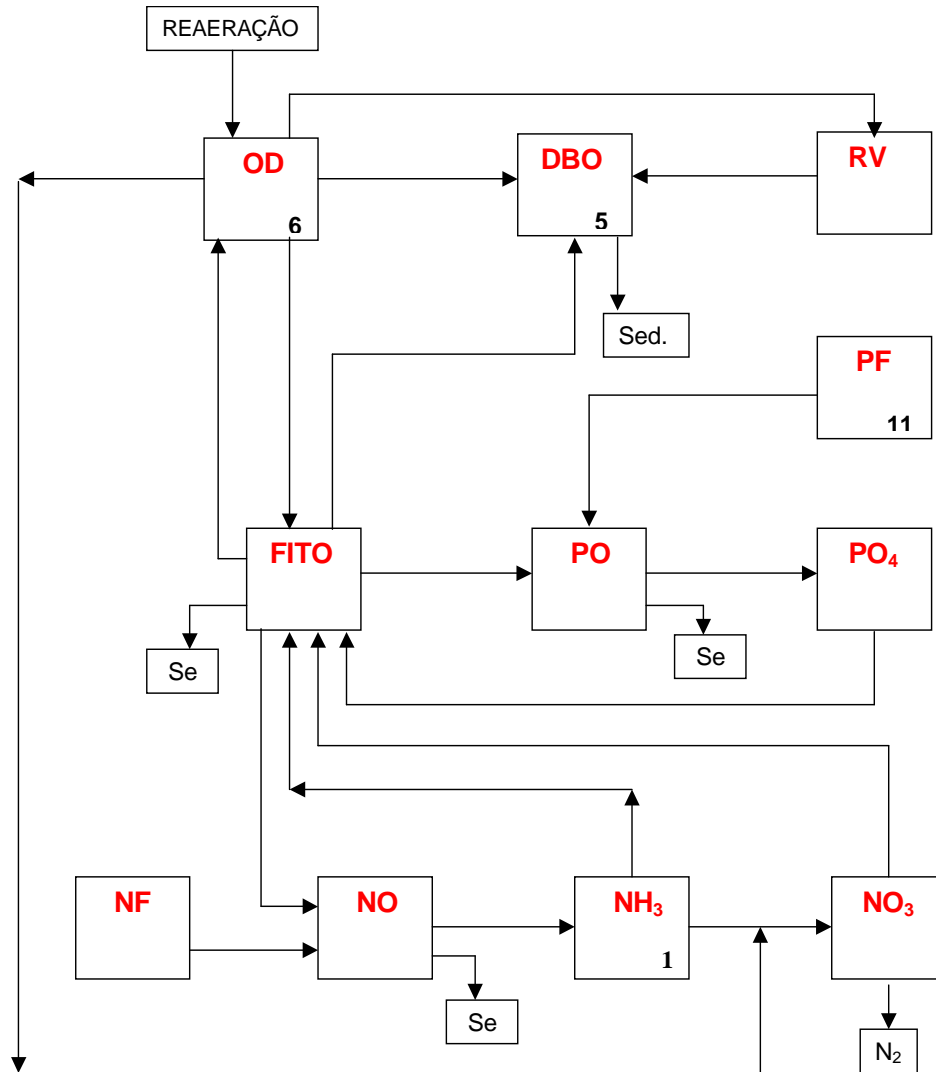
Figura 1.2-2 Estrutura do Módulo EUTRO4 Modificado
