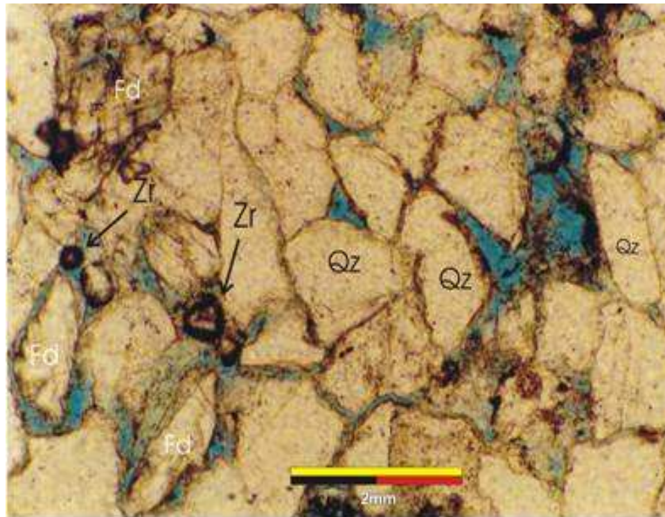
Figura 1.1-4 - Fotografia de lâmina delgada de arenito subarcosiano cimentado por sílica e crescimento secundário. Fd = feldspato; Zr = zircão. Espaço poroso em azul (aumento 10x)
