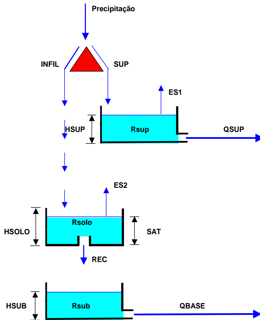
Figura 1.1-1 Figura Representação Esquemática do Modelo de Simulação
