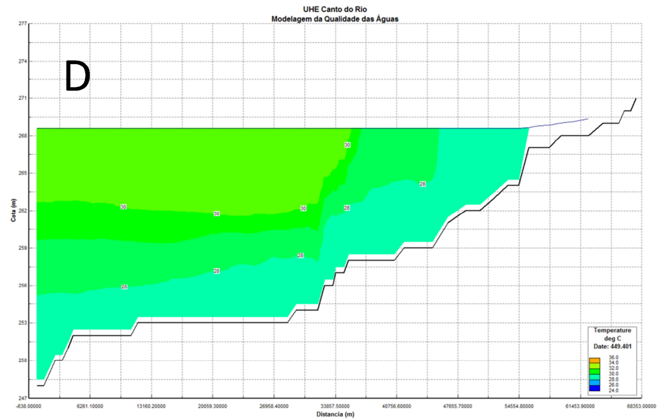
Figura 6.1.10.3.54 (Continuação) - Perfis longitudinais da Temperatura da água no braço Parnaíba (principal) - Cenário sem remoção – Período após o início da simulação: (C) 50 dias; (D) 75 dias.
