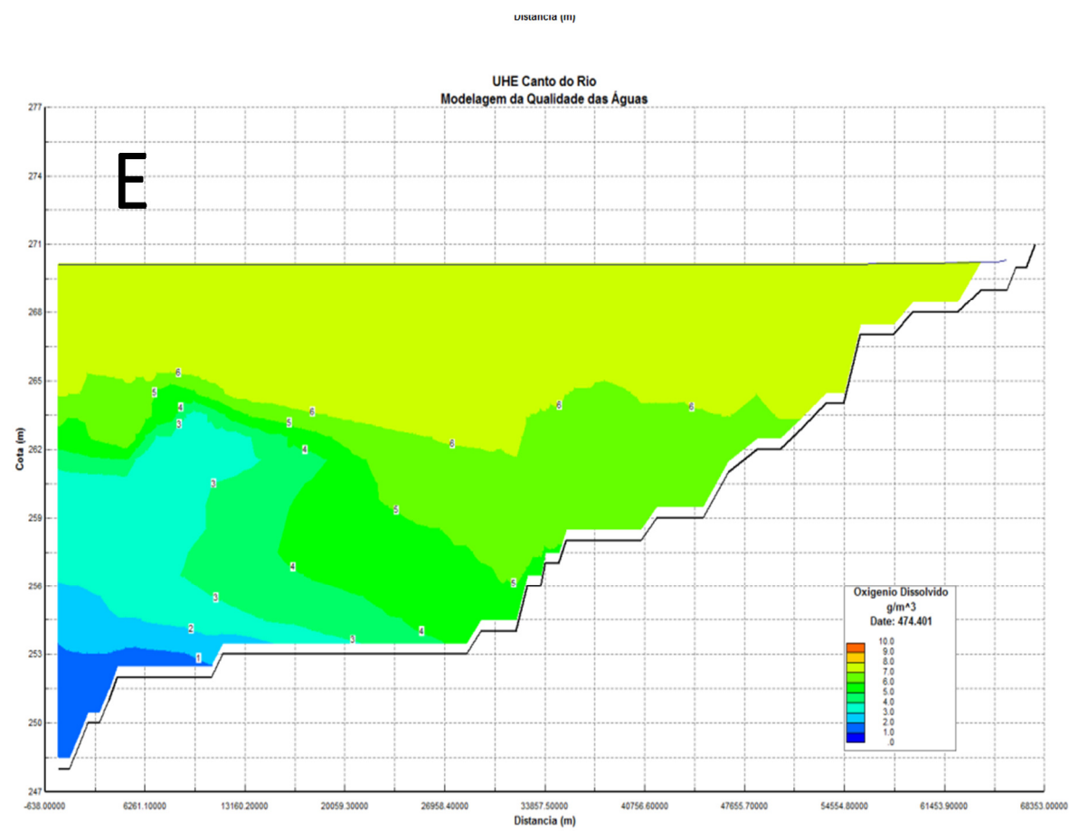
Figura 6.1.10.3.55 (Continuação) - Perfis longitudinais do OD no braço Parnaíba (principal) - Cenário sem remoção – Período após o início da simulação: (E) 100 dias.
