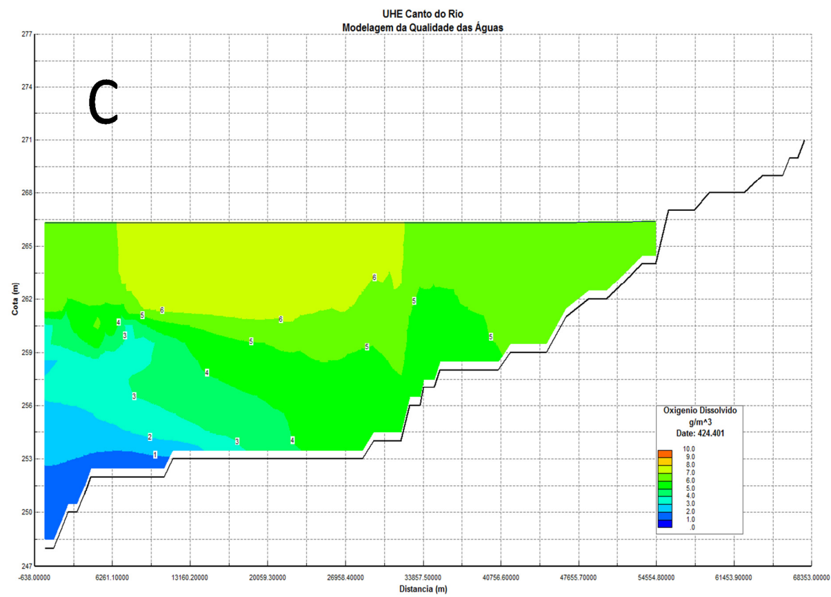
Figura 6.1.10.3.55 (Continuação) - Perfis longitudinais do OD no braço Parnaíba (principal) - Cenário sem remoção – Período após o início da simulação: (C) 50 dias; (D) 75 dias.
