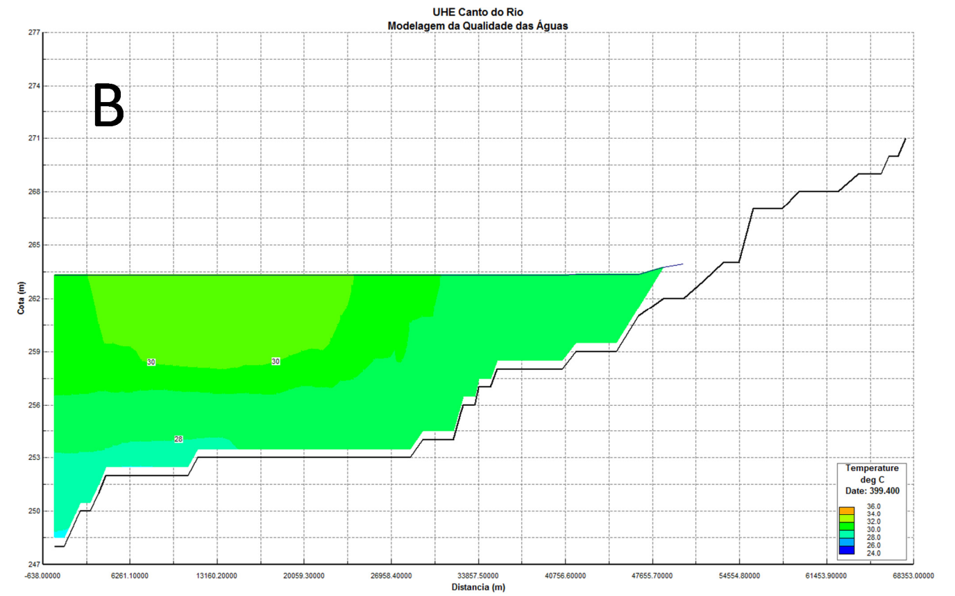
Figura 6.1.10.3.54 - Perfis longitudinais da Temperatura da água no braço Parnaíba (principal) - Cenário sem remoção – Período após o início da simulação: (A) 1 dia; (B) 25 dias.
