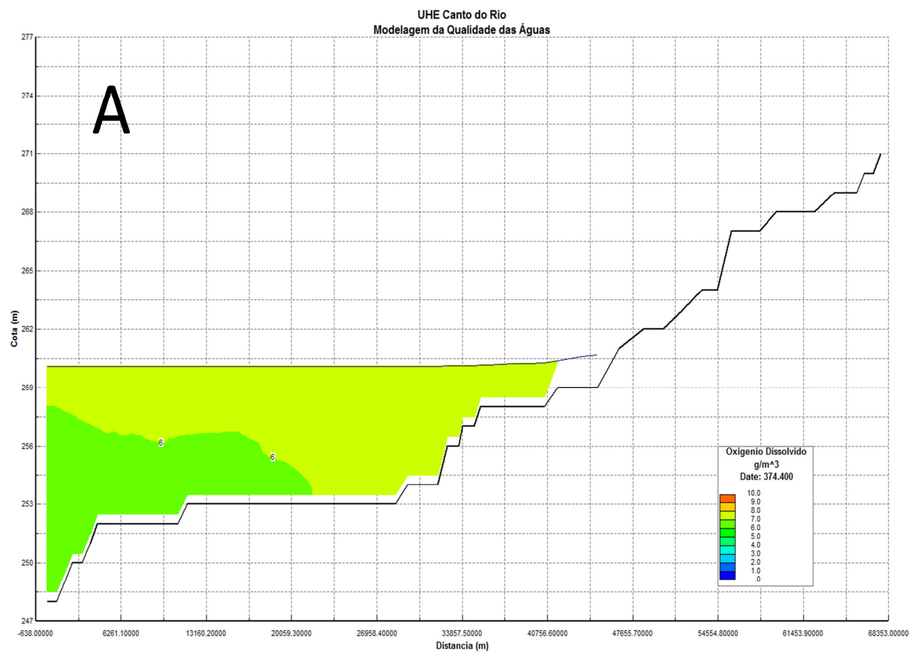
Figura 6.1.10.3.55 - Perfis longitudinais do OD no braço Parnaíba (principal) - Cenário sem remoção – Período após o início da simulação: (A) 1 dia; (B) 25 dias.
