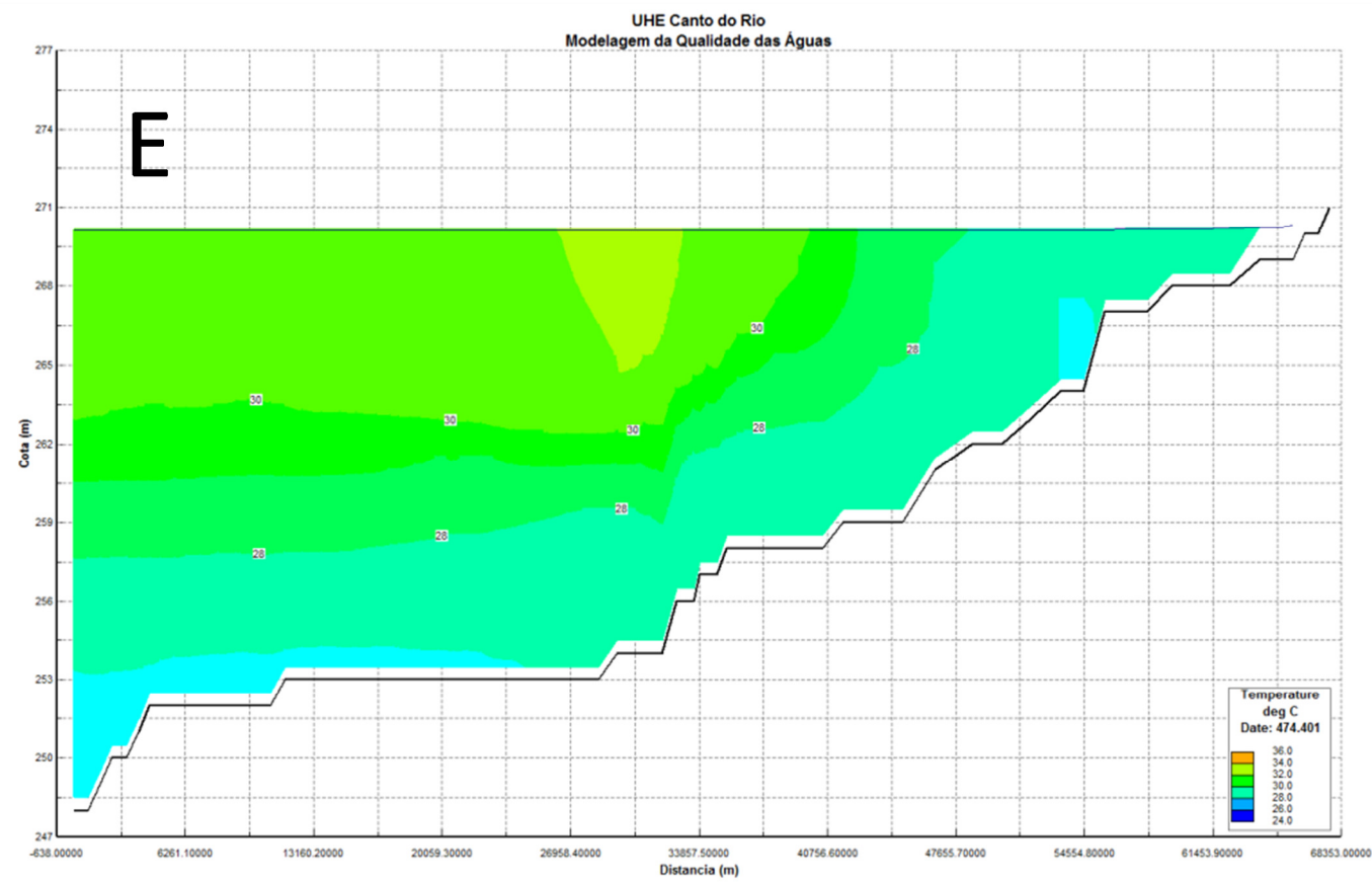
Figura 6.1.10.3.54 (Continuação) - Perfis longitudinais da Temperatura da água no braço Parnaíba (principal) - Cenário sem remoção – Período após o início da simulação: (E) 100 dias.
