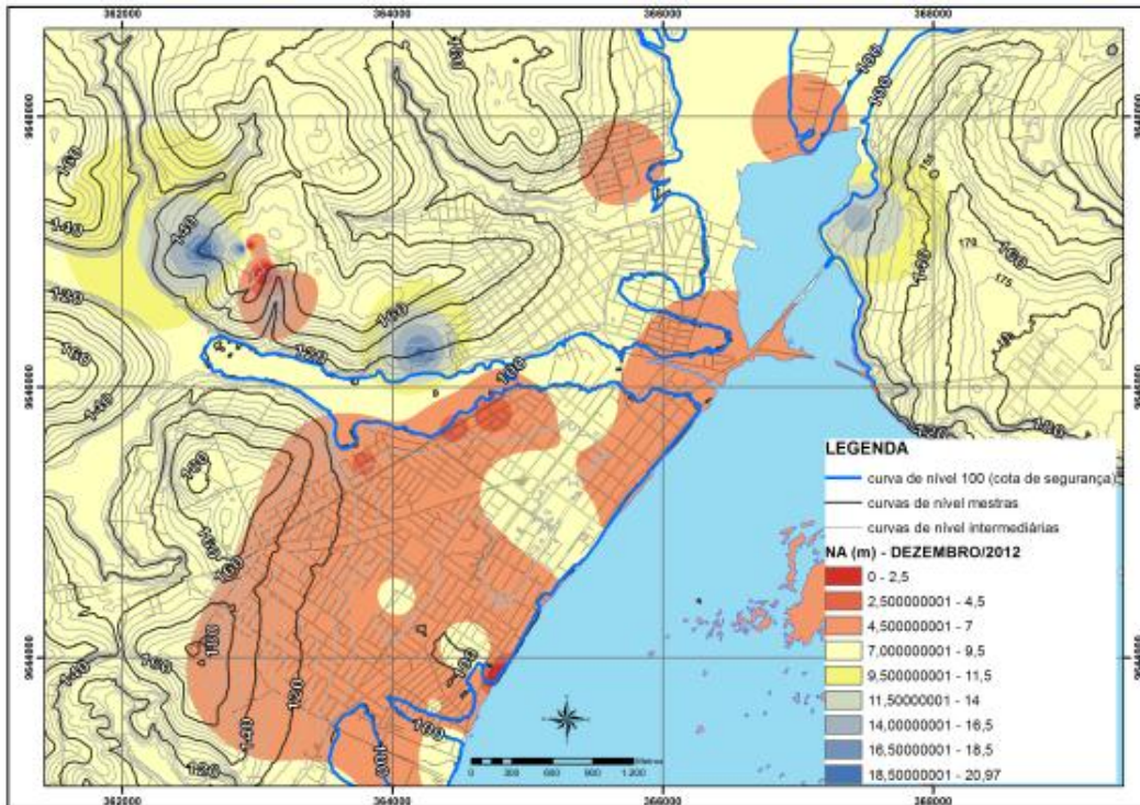
Figura 11.3.1 - 5 - Variações de NA (m) - Dezembro/2012, em Altamira.
