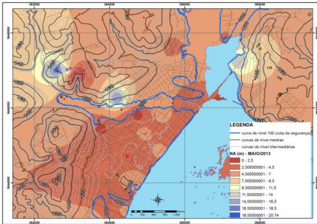
Figura 11.3.1 - 8 - Variações de NA (m) - Maio/2013, em Altamira.
