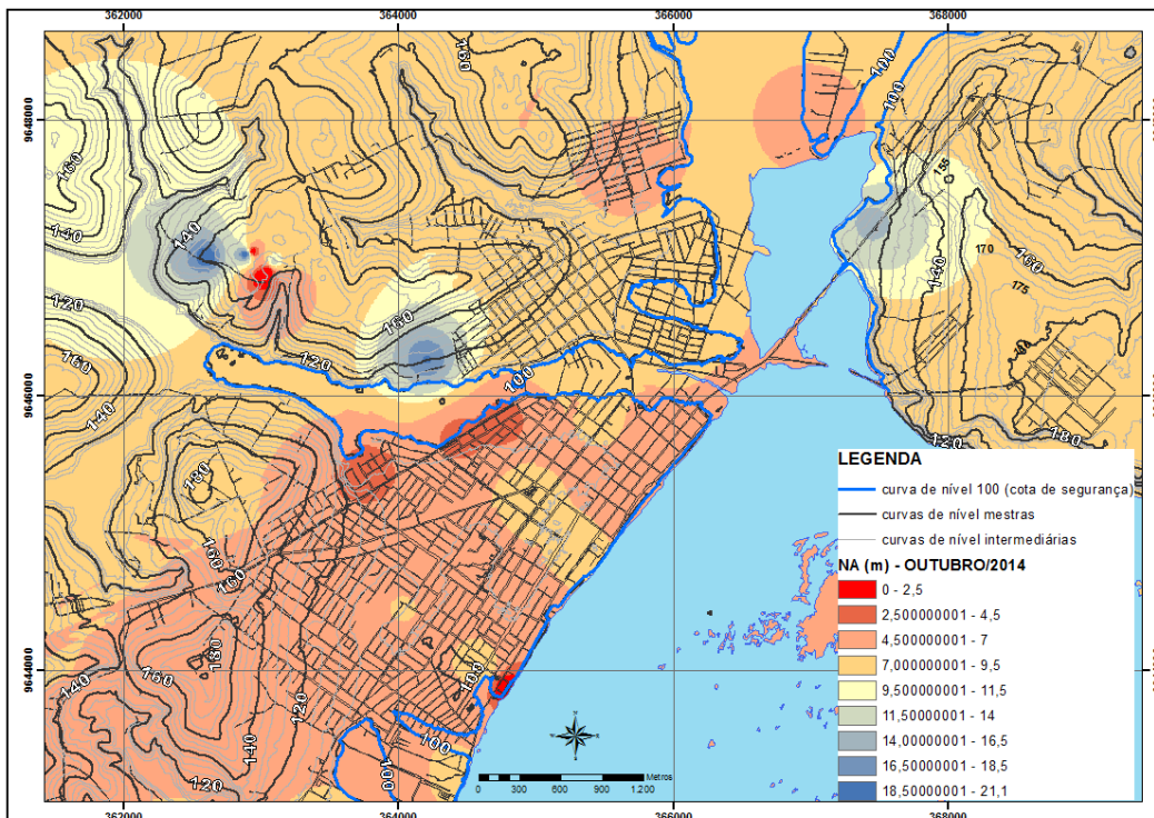
Figura 11.3.1 - 4 - Mapa da espacialização dos níveis freáticos (m) em Outubro/2014 (seca), em Altamira.
