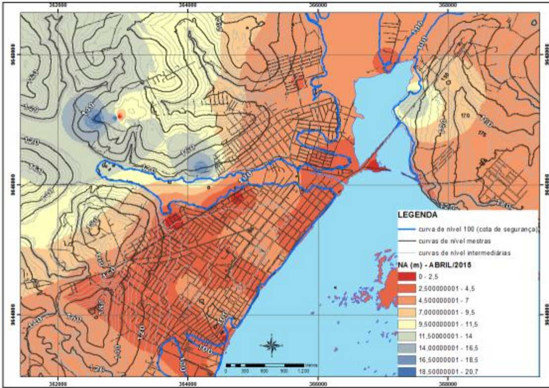
Figura 11.3.1 - 10 - Variações de NA (m) - Abril/2015, em Altamira.
