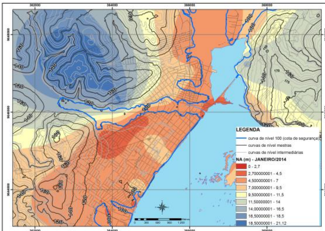
Figura 11.3.1 - 6 - Variações de NA (m) - Janeiro/2014, em Altamira.
