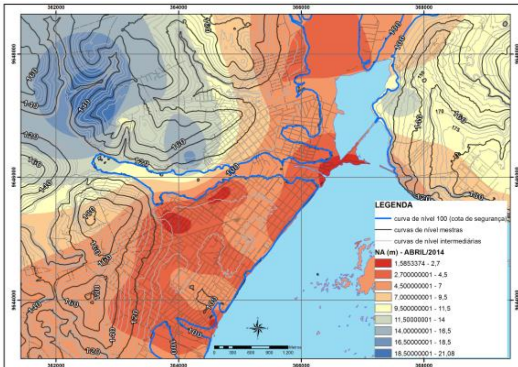
Figura 11.3.1 - 9 - Variações de NA (m) - Abril/2014, em Altamira.
