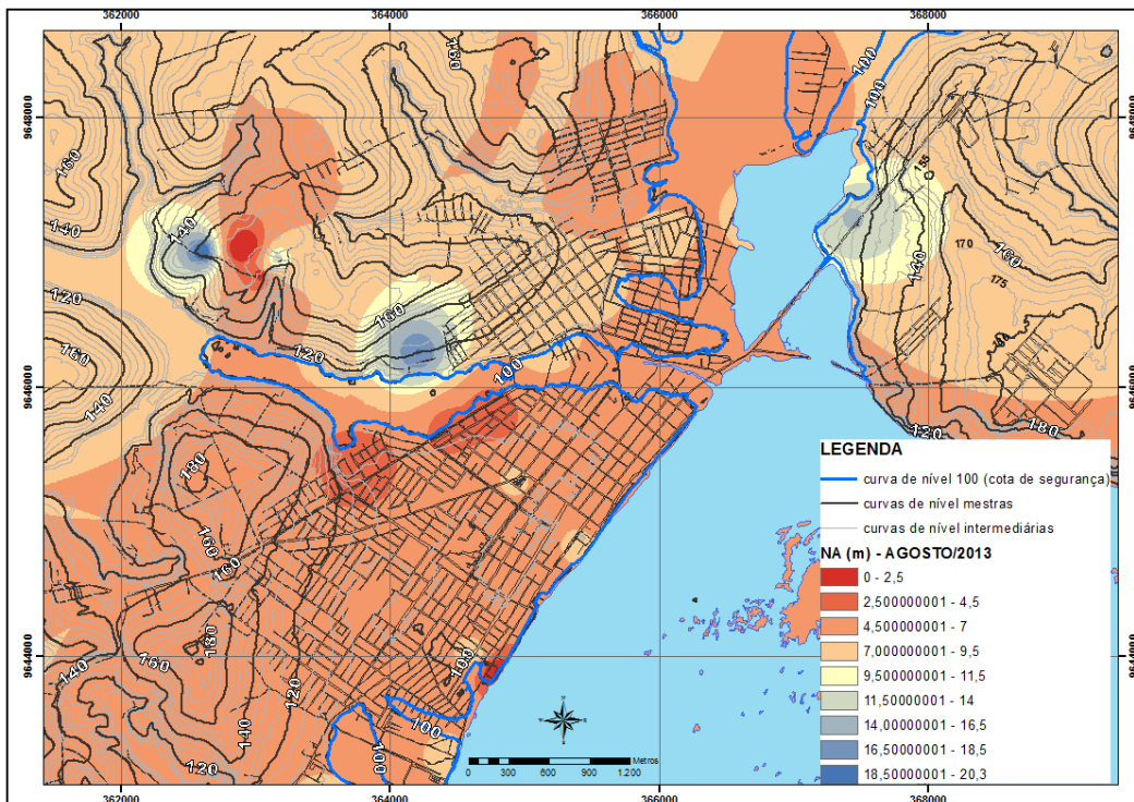
Figura 11.3.1 - 1 - Mapa da espacialização dos níveis freáticos (m) em Agosto/2013 (vazante), em Altamira.
