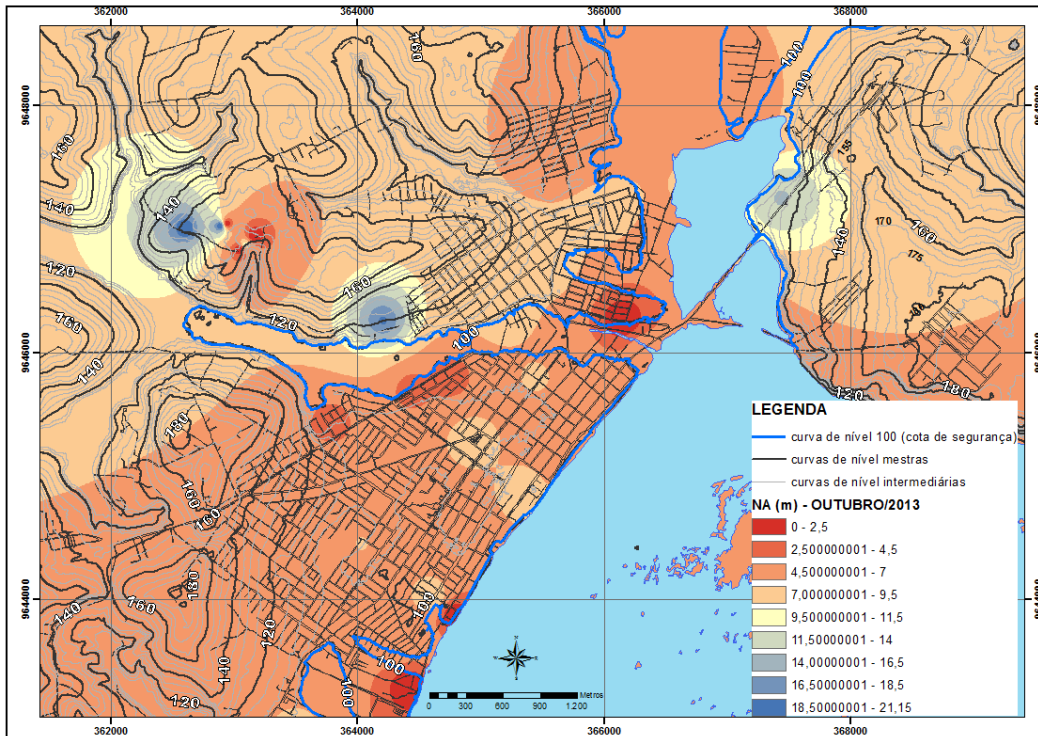
Figura 11.3.1 - 3 - Mapa da espacialização dos níveis freáticos (m) em Outubro/2013 (seca), em Altamira.
