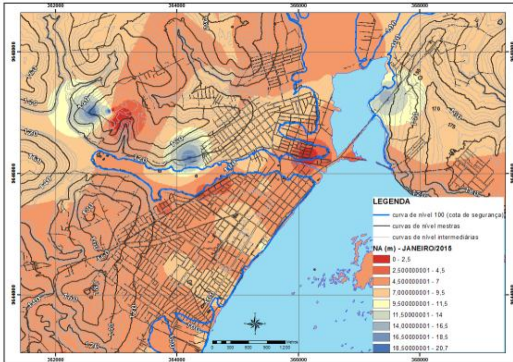
Figura 11.3.1 - 7 - Variações de NA (m) - Janeiro/2015, em Altamira.
