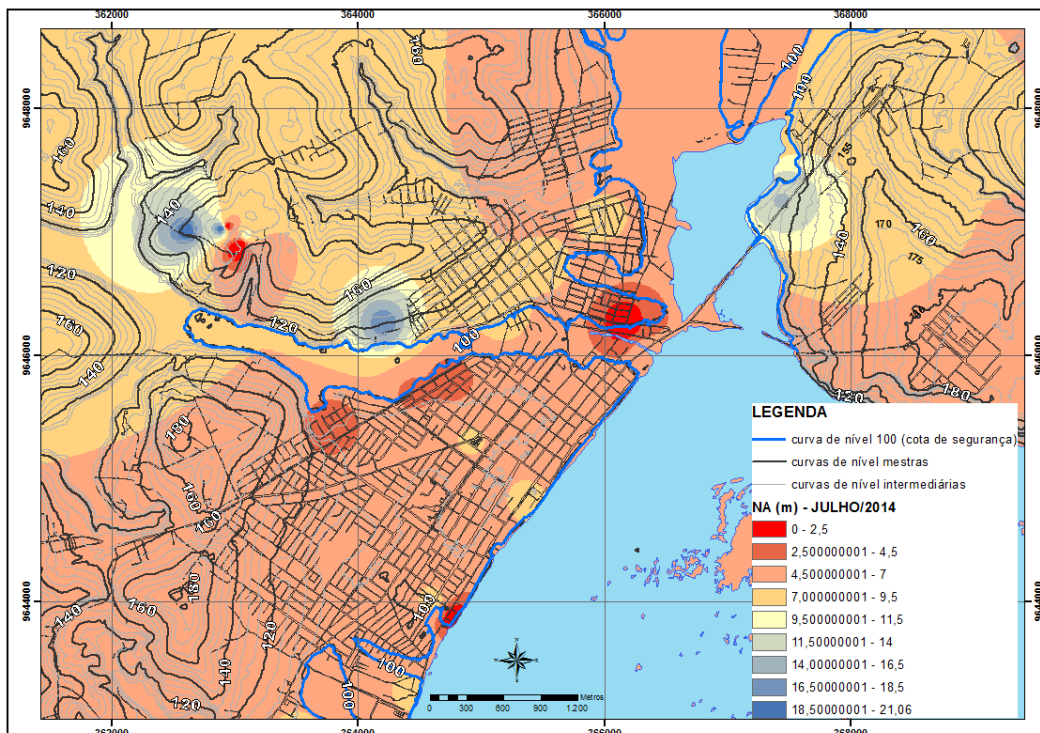
Figura 11.3.1 - 2 - Mapa da espacialização dos níveis freáticos (m) em Julho/2014 (vazante), em Altamira.
