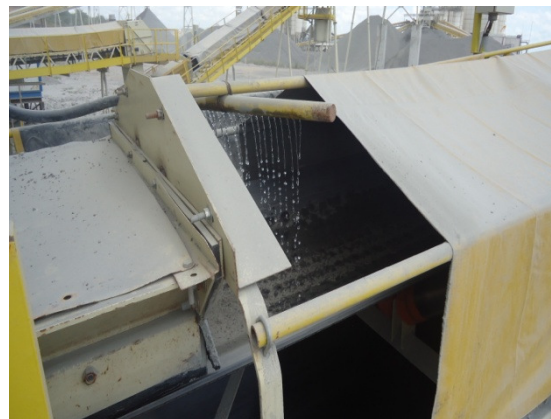
Figura - 2 – Sistema de aspersão de material particulado na central de britagem do canteiro de Belo Monte
