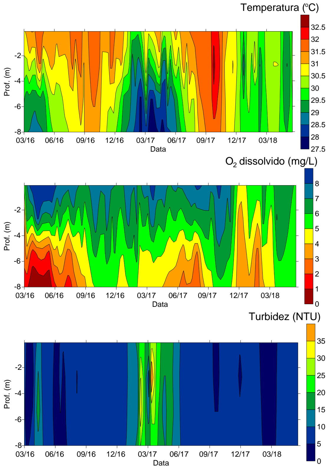
Figura 11.4.1 - 114 – Gráficos de isolinhas de temperatura, oxigênio dissolvido e turbidez no ponto Palhal, localizado no braço formado pelo igarapé Palhal na área do RX (abril de 2016 a maio de 2018).
