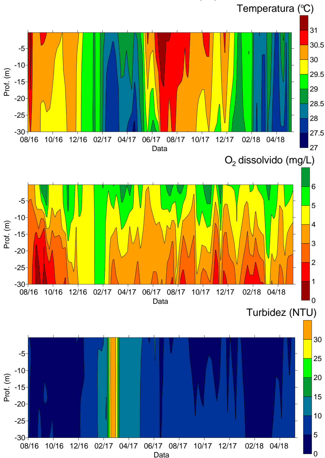
Figura 11.4.1 - 135 – Gráficos de isolinhas de temperatura, oxigênio dissolvido e turbidez no ponto CN 07, localizado no RI, na bacia do igarapé Aturiá, 5,0 km a montante da Casa de Força Principal em Belo Monte (agosto de 2016 a maio de 2018).
