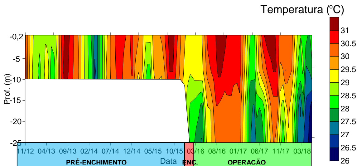
Figura 11.4.1 - 110 – Gráficos de isolinhas de temperatura registrada no rio Xingu, no ponto de coleta RX 03, entre novembro de 2012 e maio de 2018, no âmbito do monitoramento limnológico do PBA da UHE Belo Monte.
