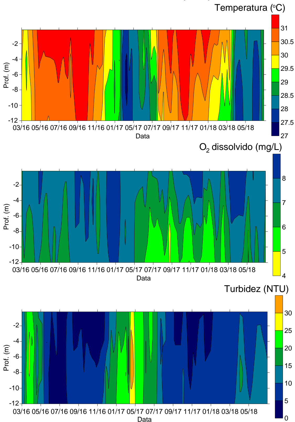
Figura 11.4.1 - 144 – Gráficos de isolinhas de temperatura, oxigênio dissolvido e turbidez no ponto PTRV 03, localizado no rio Xingu, na área do TRV, a jusante 9 km do Canal de Fuga (abril de 2016 a maio de 2018).
