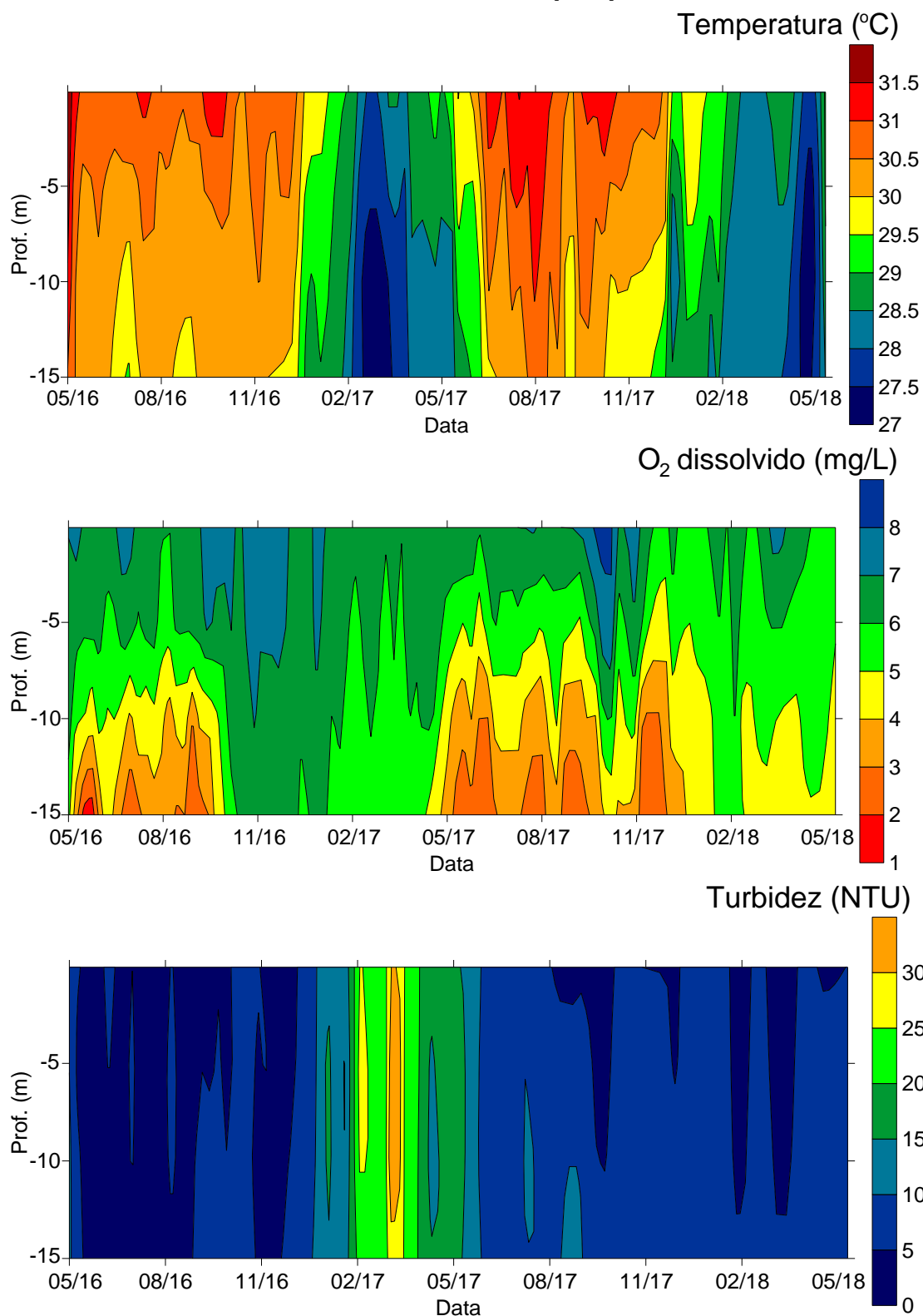
Figura 11.4.1 - 117 – Gráficos de isolinhas de temperatura, oxigênio dissolvido e turbidez no ponto Di Maria, localizado no braço formado pelo igarapé Di Maria na área do RX (maio de 2016 a maio de 2018).
