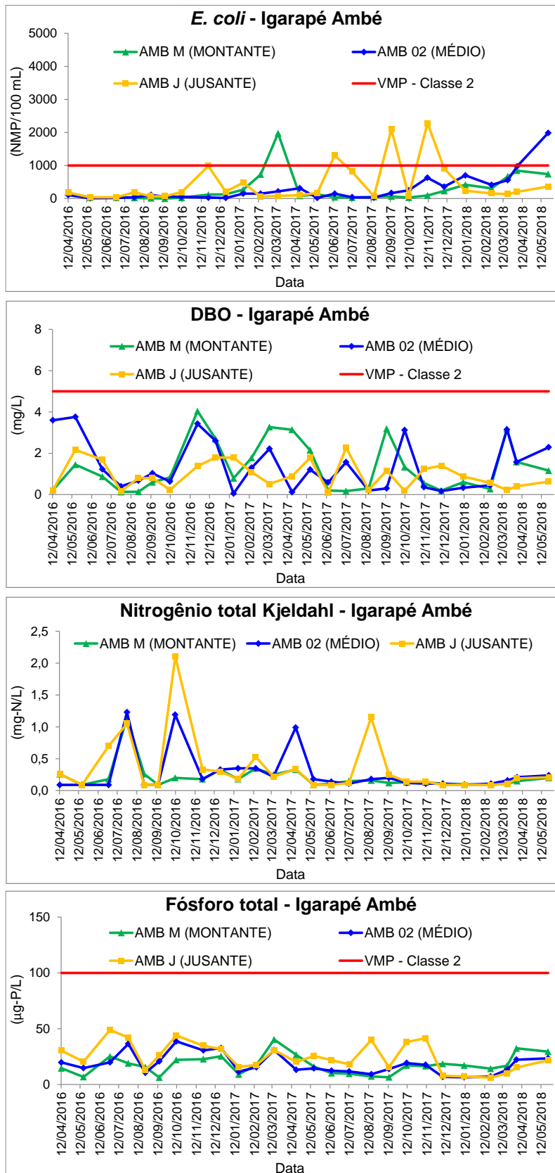
Figura 11.4.1 - 123 - Gráficos de variação temporal de E. coli , DBO, nitrogênio total Kjeldahl e fósforo total nos pontos localizados no igarapé Ambé durante a fase de pós-enchimento do RX (abril de 2016 a maio de 2018).
