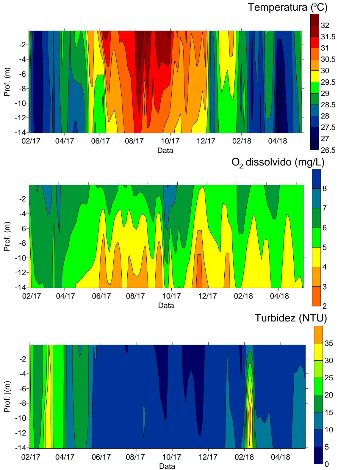
Figura 11.4.1 - 155 – Gráficos de isolinhas de temperatura, oxigênio dissolvido e turbidez no ponto RX-RB-10, próximo às comunidades ribeirinhas do entorno do reservatório do Xingu (fevereiro de 2017 a maio de 2018).
