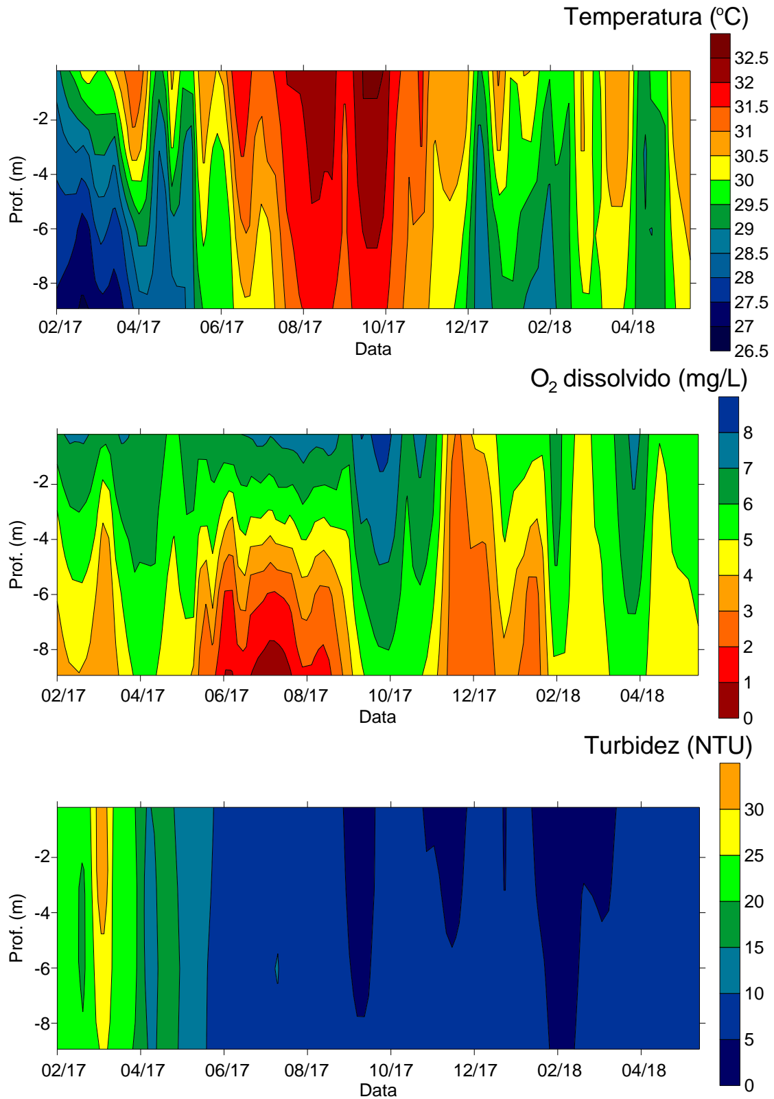
Figura 11.4.1 - 153 – Gráficos de isolinhas de temperatura, oxigênio dissolvido e turbidez no ponto RX-RB-08, próximo às comunidades ribeirinhas do entorno do reservatório do Xingu (fevereiro de 2017 a maio de 2018).
