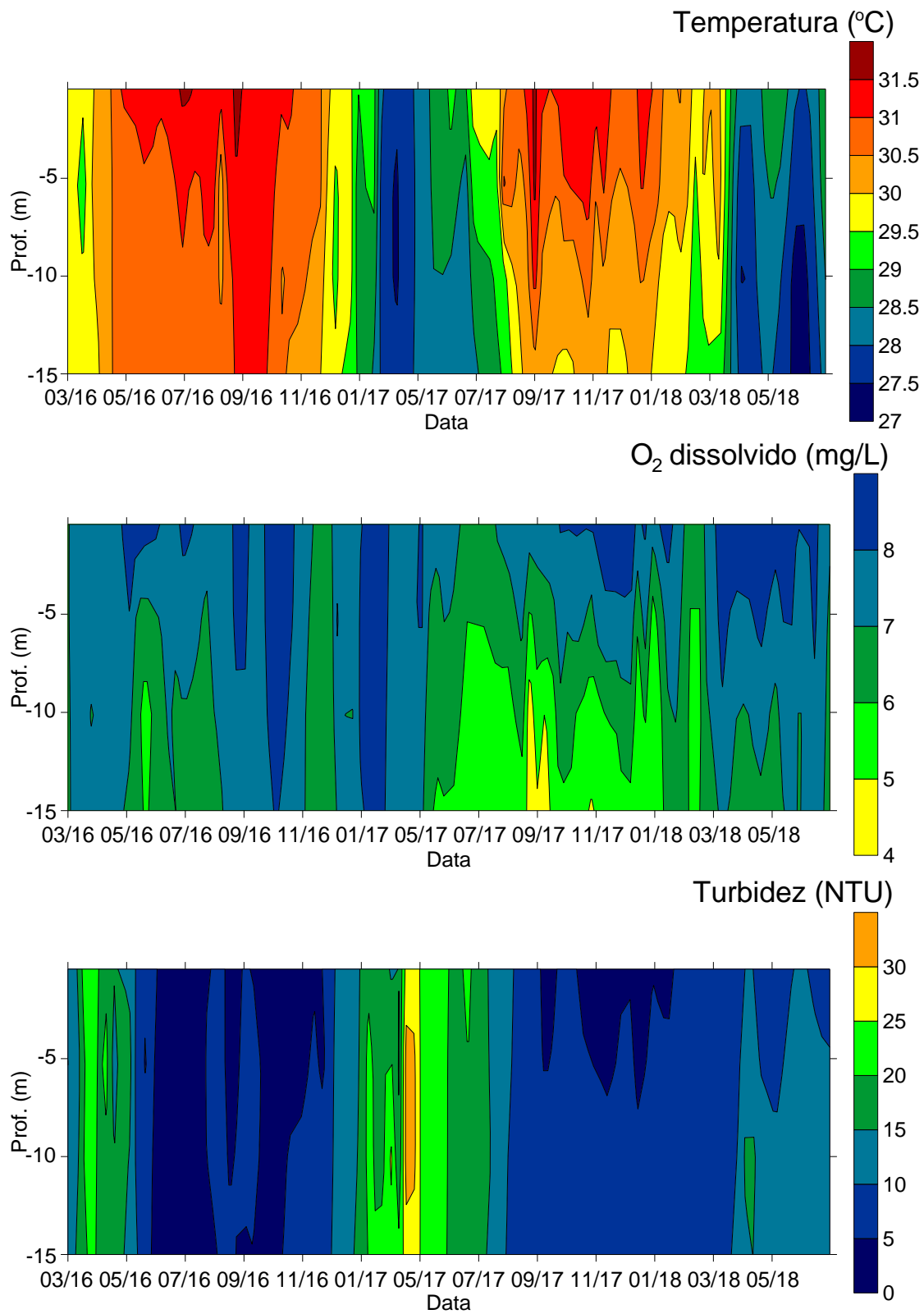
Figura 11.4.1 - 142 – Gráficos de isolinhas de temperatura, oxigênio dissolvido e turbidez no ponto PTRV 01, localizado no rio Xingu, na área do TRV, a jusante 4 km do Canal de Fuga (abril de 2016 a maio de 2018).
