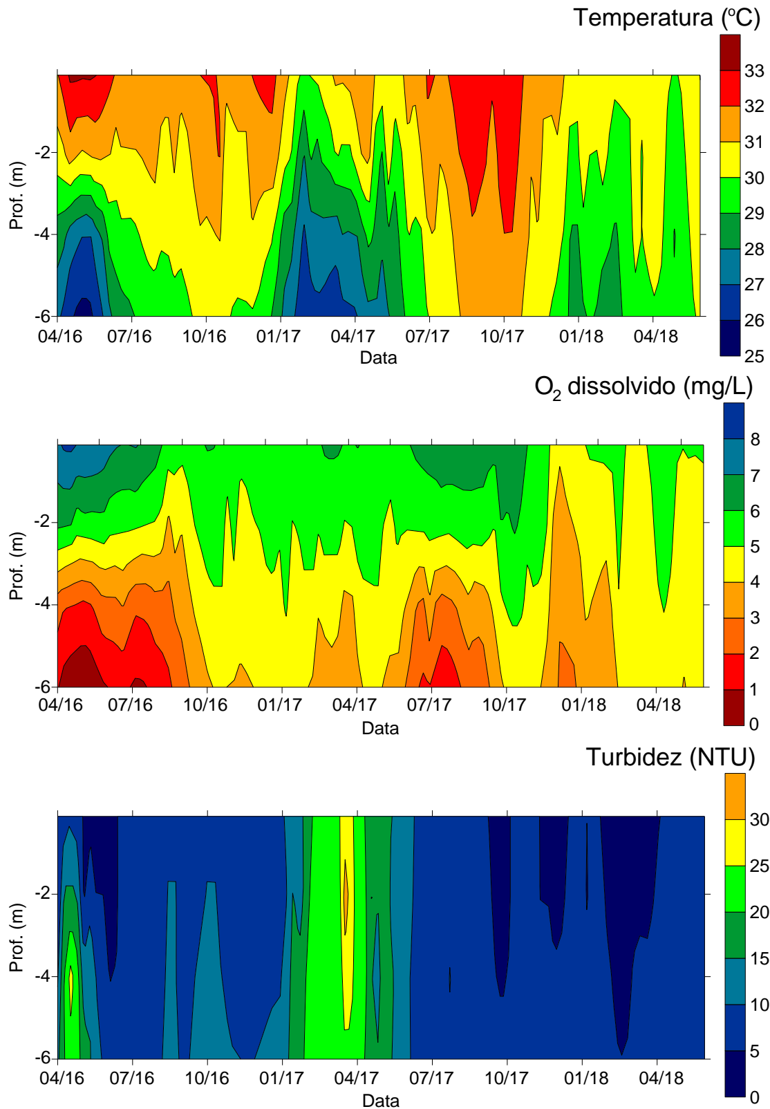
Figura 11.4.1 - 115 – Gráficos de isolinhas de temperatura, oxigênio dissolvido e turbidez no ponto Palhal 2, localizado no braço formado pelo igarapé Palhal na área do RX (abril de 2016 a maio de 2018).
