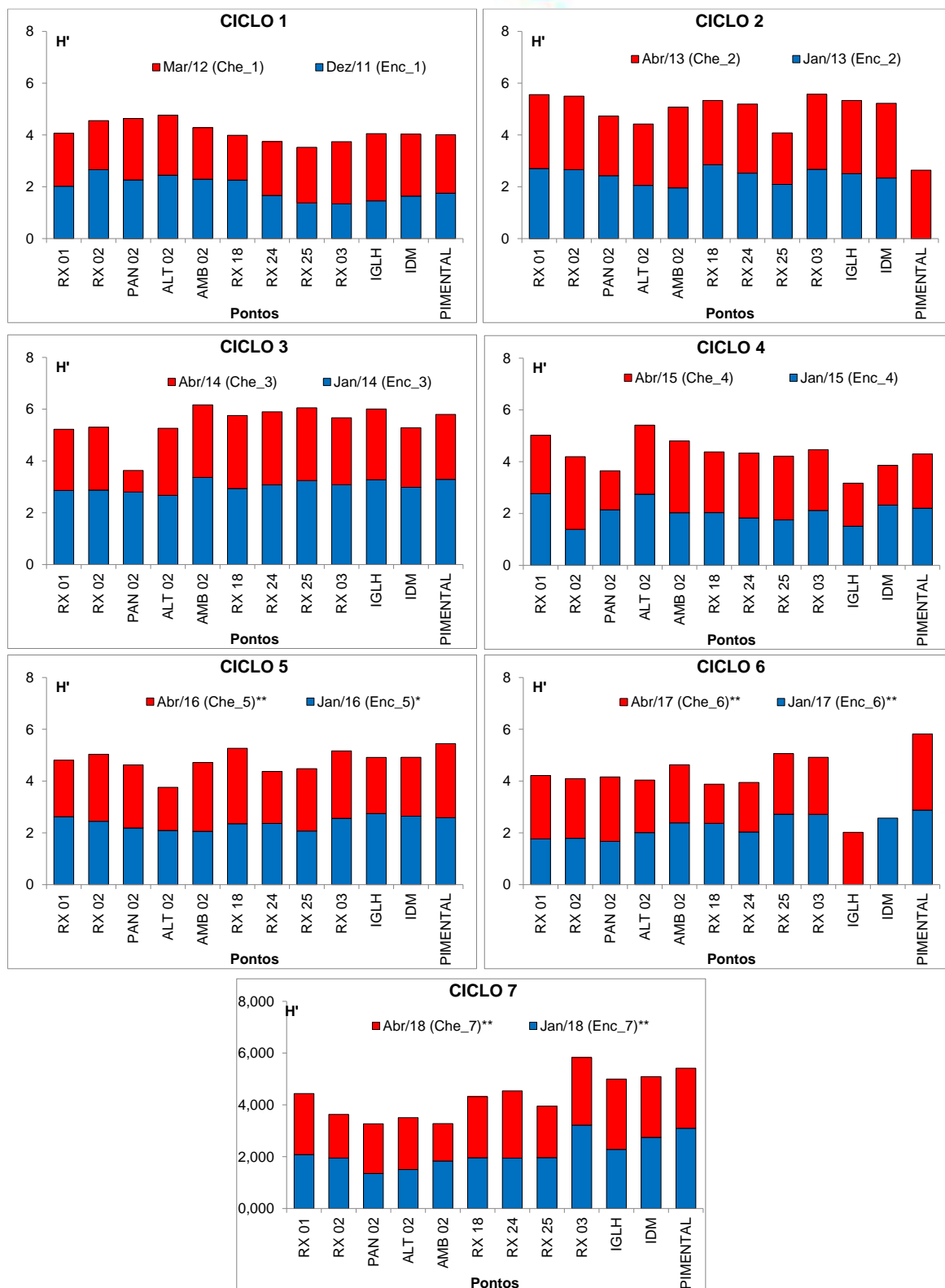
Figura 11.4.1 - 83 – Diversidade de Shannon-Wiener ( H' , bits/indivíduo) da comunidade zooplancônica acumulada nos pontos localizados na área do Reservatório Xingu (RX) nos sete ciclos hidrológicos de enchente e cheia (dezembro 2011 a abril de 2018). Ciclo 1: 2011/2012; Ciclo 2: 2013; Ciclo 3: 2014; Ciclo 4: 2015; Ciclo 5: 2016; Ciclo 6: 2017; Ciclo 7: 2018. *: fase de enchimento; **: fase de operação.
