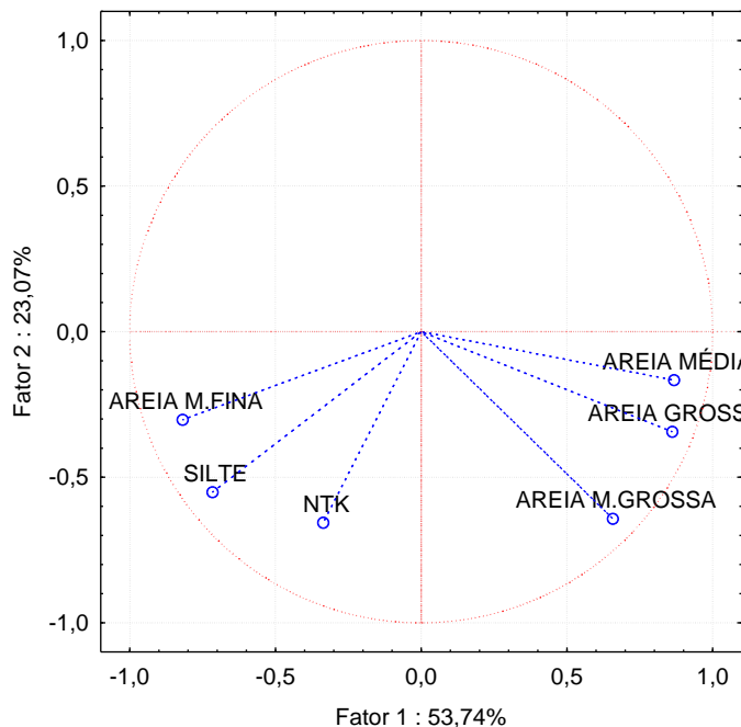
Projeção dos pontos de coleta de sedim. no plano fatorial (1 x 2) Área do Trecho de Restituição de Vazão (TRV)
