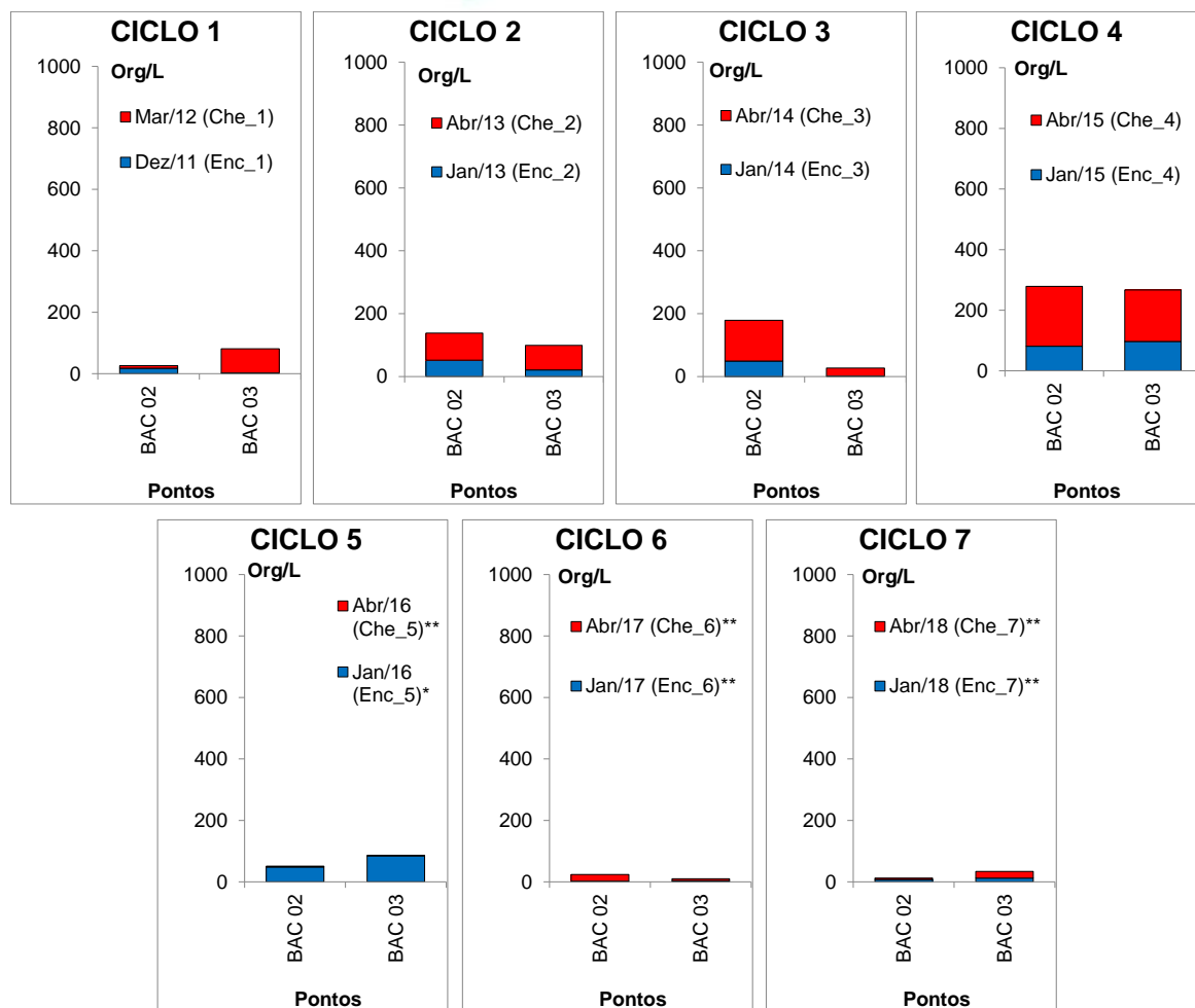
Figura 11.4.1 - 102 – Abundância (org/m 2 ) da comunidade bentônica nos pontos localizados no Rio Bacajá nos sete ciclos hidrológicos de enchente e cheia (dezembro 2011 a abril de 2018). Ciclo 1: 2011/2012; Ciclo 2: 2013; Ciclo 3: 2014; Ciclo 4: 2015; Ciclo 5: 2016; Ciclo 6: 2017; Ciclo 7: 2018. *: fase de enchimento; **: fase de operação.
