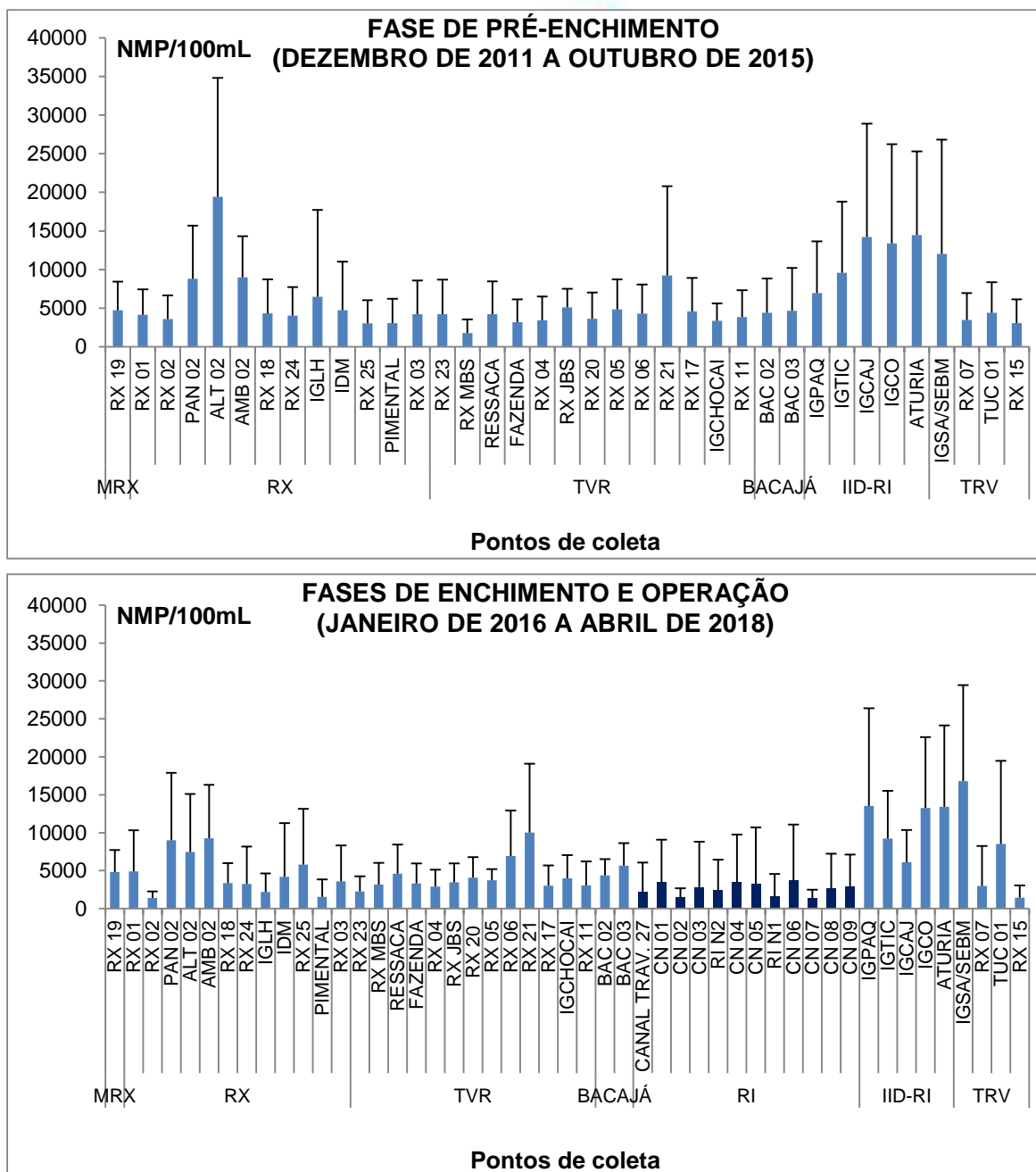
Figura 11.4.1 - 17 – Médias e desvio padrão das concentrações de coliformes totais nas campanhas trimestrais referentes à fase de pré-enchimento (dezembro de 2011 a outubro de 2015) e à fase de operação (janeiro de 2016 a abril de 2018). MRX: Montante do Reservatório do Xingu; RX: Reservatório do Xingu; TVR: Trecho de Vazão Reduzida; TRV: Trecho de Restituição de Vazão; IID-RI: Igarapés Interceptados pelos Diques; RI: Reservatório Intermediário; BAC: rio Bacajá. *: dados do RI (em azul mais escuro) são referentes ao período entre abril de 2016 e abril de 2018, após a sua formação.
