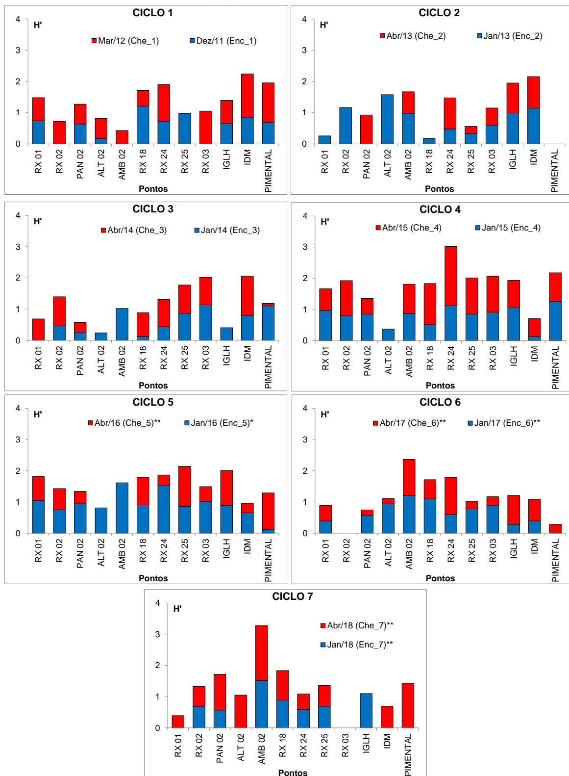
Figura 11.4.1 - 104 – Diversidade de Shannon-Wiener ( H' , bits/indivíduo) da comunidade bentônica nos pontos localizados na área do Reservatório do Xingu (RX) nos sete ciclos hidrológicos de enchente e cheia (dezembro 2011 a abril de 2018). Ciclo 1: 2011/2012; Ciclo 2: 2013; Ciclo 3: 2014; Ciclo 4: 2015; Ciclo 5: 2016; Ciclo 6: 2017; Ciclo 7: 2018. *: fase de enchimento; **: fase de operação.
