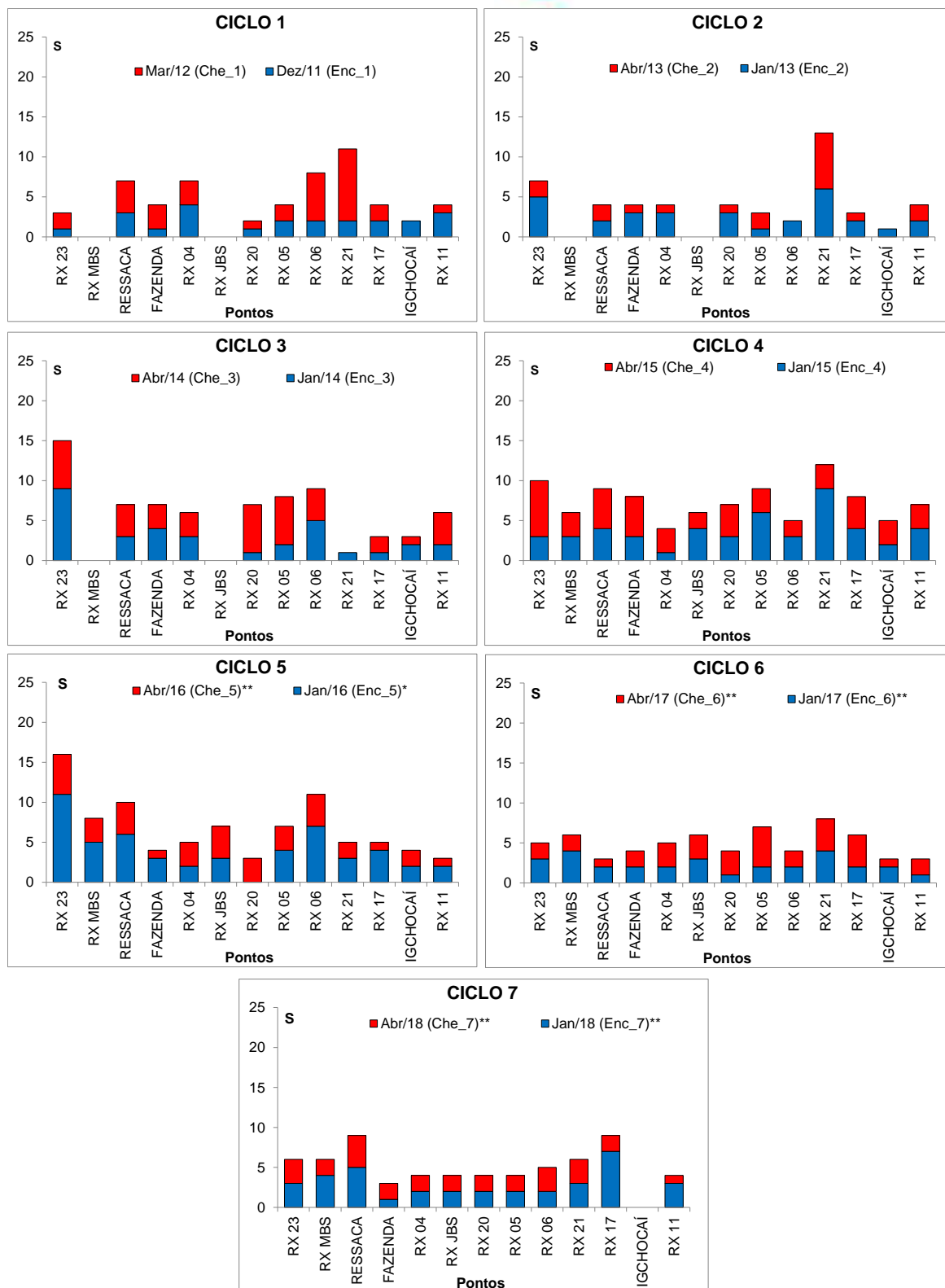
Figura 11.4.1 - 91 – Riqueza total (S) da comunidade bentônica nos pontos localizados na área do Trecho de Vazão Reduzida (TVR) nos sete ciclos hidrológicos de enchente e cheia (dezembro 2011 a abril de 2018). Ciclo 1: 2011/2012; Ciclo 2: 2013; Ciclo 3: 2014; Ciclo 4: 2015; Ciclo 5: 2016; Ciclo 6: 2017; Ciclo 7: 2018. *: fase de enchimento; **: fase de operação.
