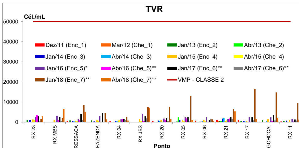
Figura 11.4.1 - 59 – Densidade de cianobactérias (células/mL) nos pontos localizados na Área do Trecho de Vazão Reduzida (TVR) nos sete ciclos hidrológicos de enchente e cheia (dezembro 2011 a abril de 2018). *: fase de enchimento; **: fase de operação. VMP – CLASSE 2: limite estabelecido pela Resolução CONAMA nº 357/2005 para águas doces de classe 2.
