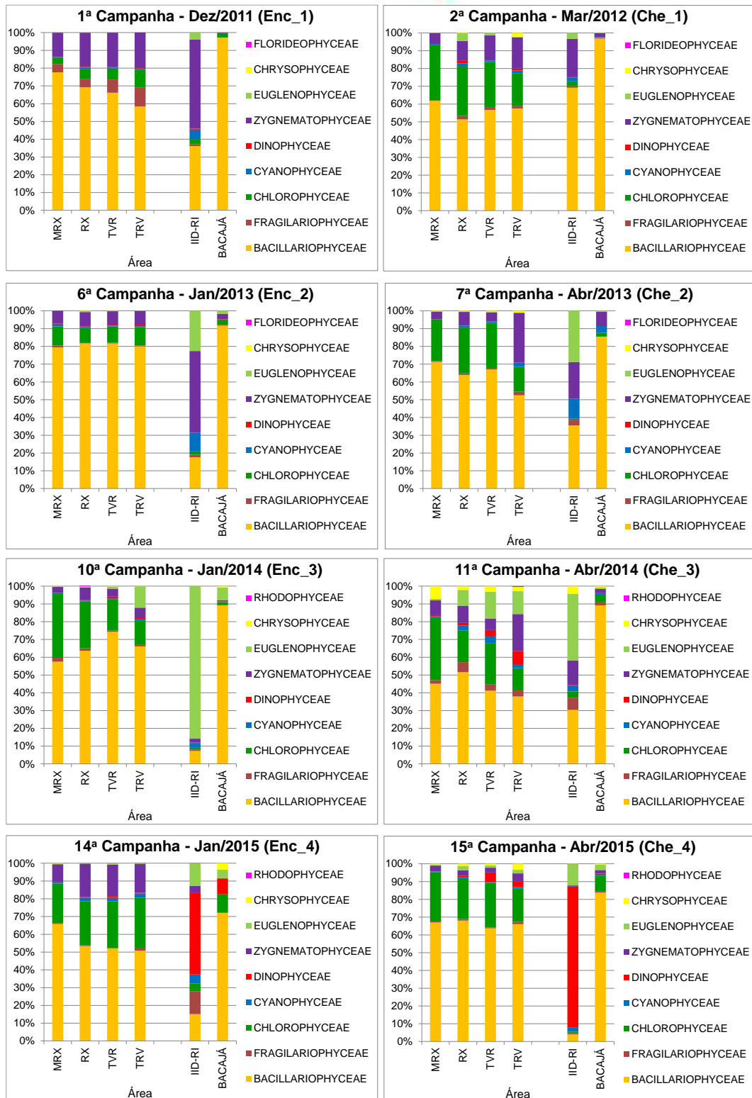
Figura 11.4.1 - 40 – Abundâncias relativas totais (%) das Classes de fitoplâncton registradas nas áreas a Montante do Reservatório do Xingu (MRX), Reservatório do Xingu (RX), Trecho de Vazão Reduzida (TVR), Rio Bacajá (BACAJÁ), Trecho de Restituição de Vazão (TRV) e Igarapés Interceptados pelos Diques do Reservatório Intermediário (IID-RI) nas campanhas trimestrais considerando somente os períodos de enchente e cheia do 1º ao 4º ciclo hidrológico (dezembro de 2011 a abril de 2015) durante a fase de pré-enchimento.
