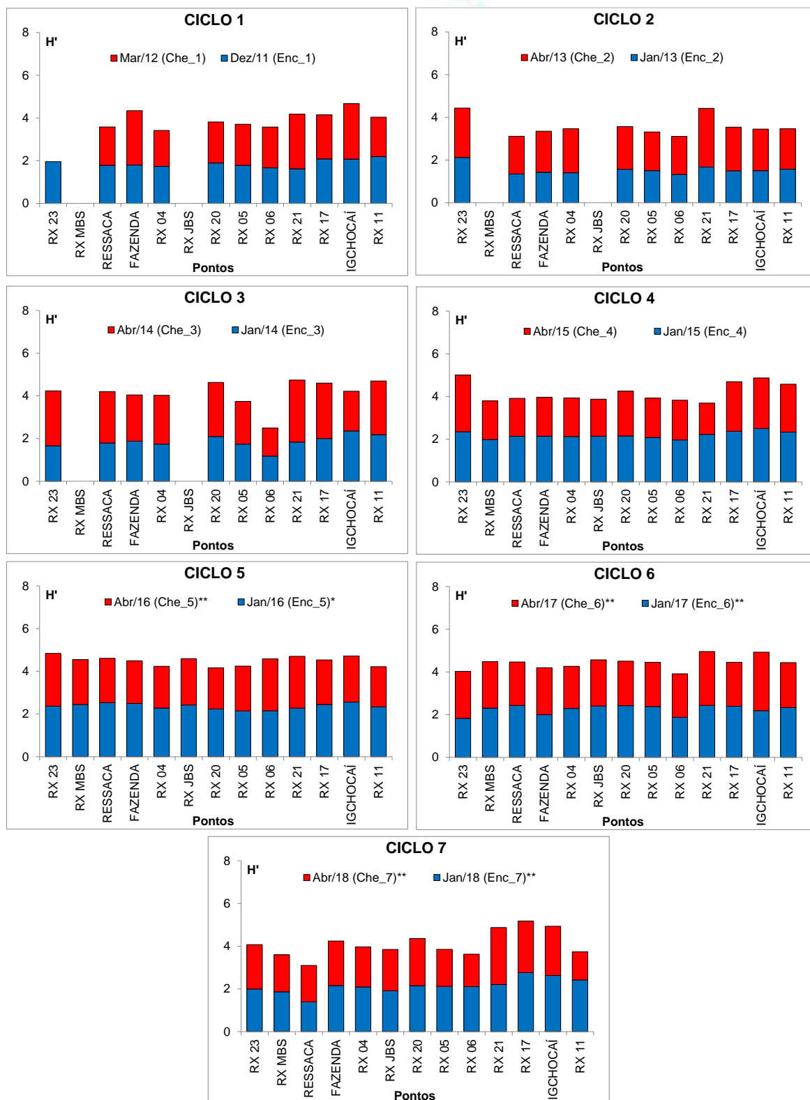
Figura 11.4.1 - 52 – Diversidade de Shannon-Wiener ( H' , bits/indivíduo) da comunidade fitoplanctônica acumulada nos pontos localizados na Área do Trecho de Vazão Reduzida (TVR) nos sete ciclos hidrológicos de enchente e cheia (dezembro 2011 a abril de 2018). Ciclo 1: 2011/2012; Ciclo 2: 2013; Ciclo 3: 2014; Ciclo 4: 2015; Ciclo 5: 2016; Ciclo 6: 2017; Ciclo 7: 2018. *: fase de enchimento; **: fase de operação.
