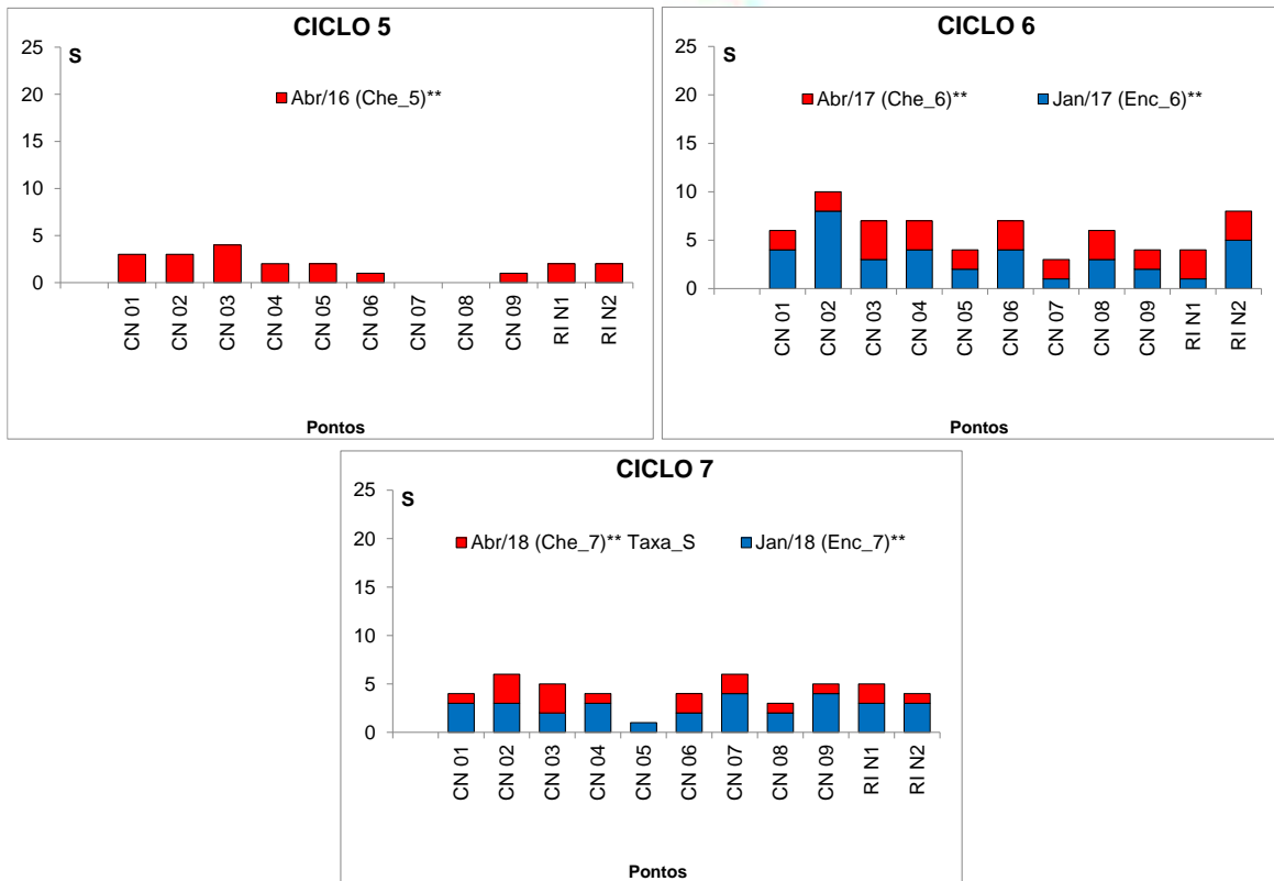
Figura 11.4.1 - 93 – Riqueza total (S) da comunidade bentônica nos pontos no Reservatório Intermediário (RI) no 5º ao 7º ciclo hidrológico de enchente e cheia, durante a fase de operação (abril de 2016 a abril de 2018).
