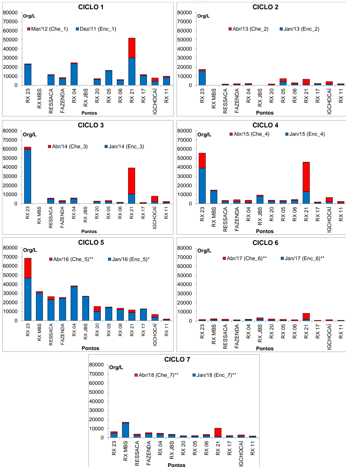
Figura 11.4.1 - 77 – Abundância de organismos zooplânctônicos nos pontos localizados na Área do Trecho de Vazão Reduzida (TVR) nos sete ciclos hidrológicos de enchente e cheia (dezembro 2011 a abril de 2018). Ciclo 1: 2011/2012; Ciclo 2: 2013; Ciclo 3: 2014; Ciclo 4: 2015; Ciclo 5: 2016; Ciclo 6: 2017; Ciclo 7: 2018. *: fase de enchimento; **: fase de operação.
