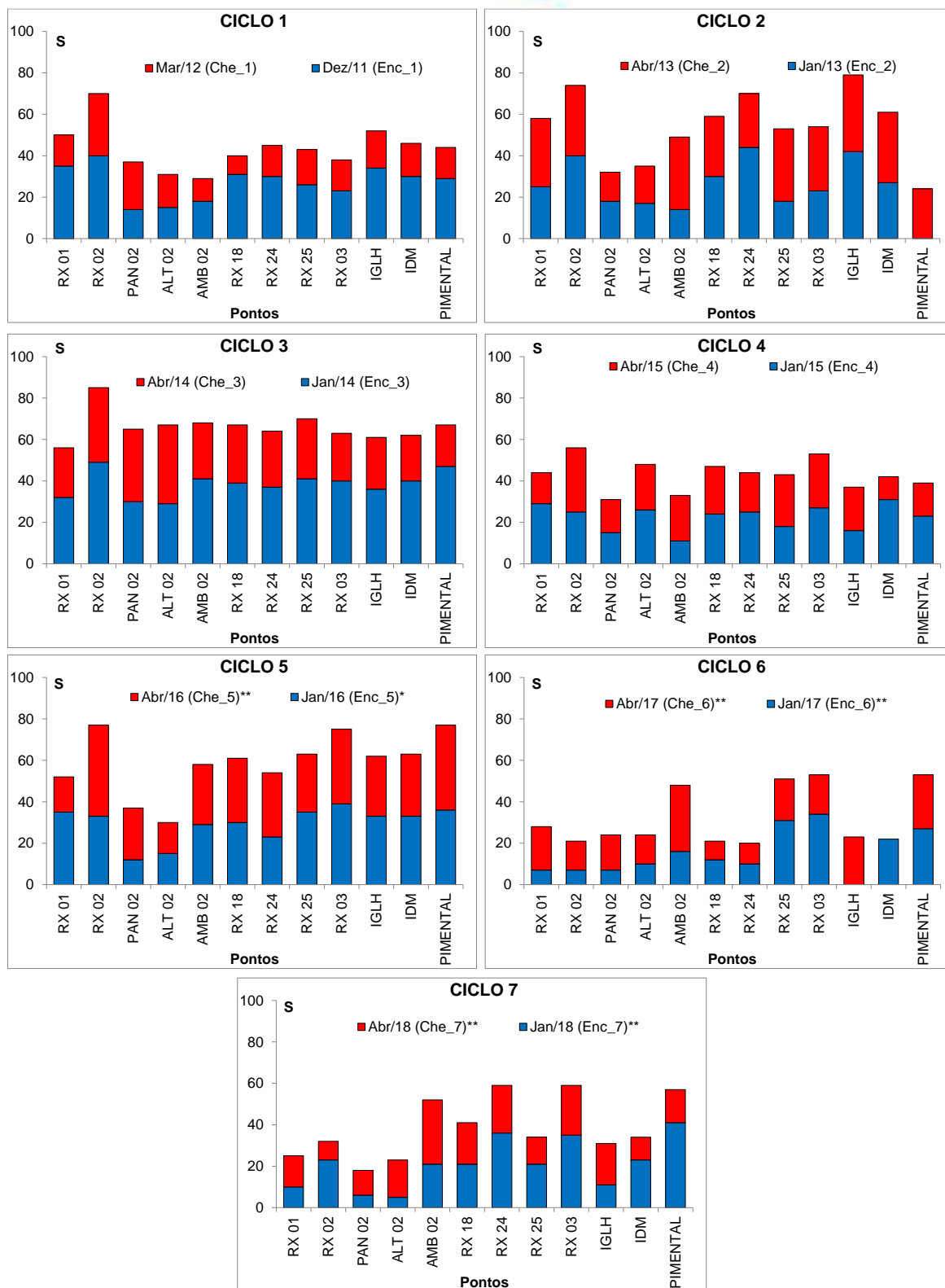
Figura 11.4.1 - 66 – Riqueza total (S) do zooplâncton (espécies) acumulada nos pontos localizados na Área do Reservatório Xingu (RX) nos sete ciclos hidrológicos de enchente e cheia (dezembro 2011 a abril de 2018). Ciclo 1: 2011/2012; Ciclo 2: 2013; Ciclo 3: 2014; Ciclo 4: 2015; Ciclo 5: 2016; Ciclo 6: 2017; Ciclo 7: 2018.*: fase de enchimento; **: fase de operação.
