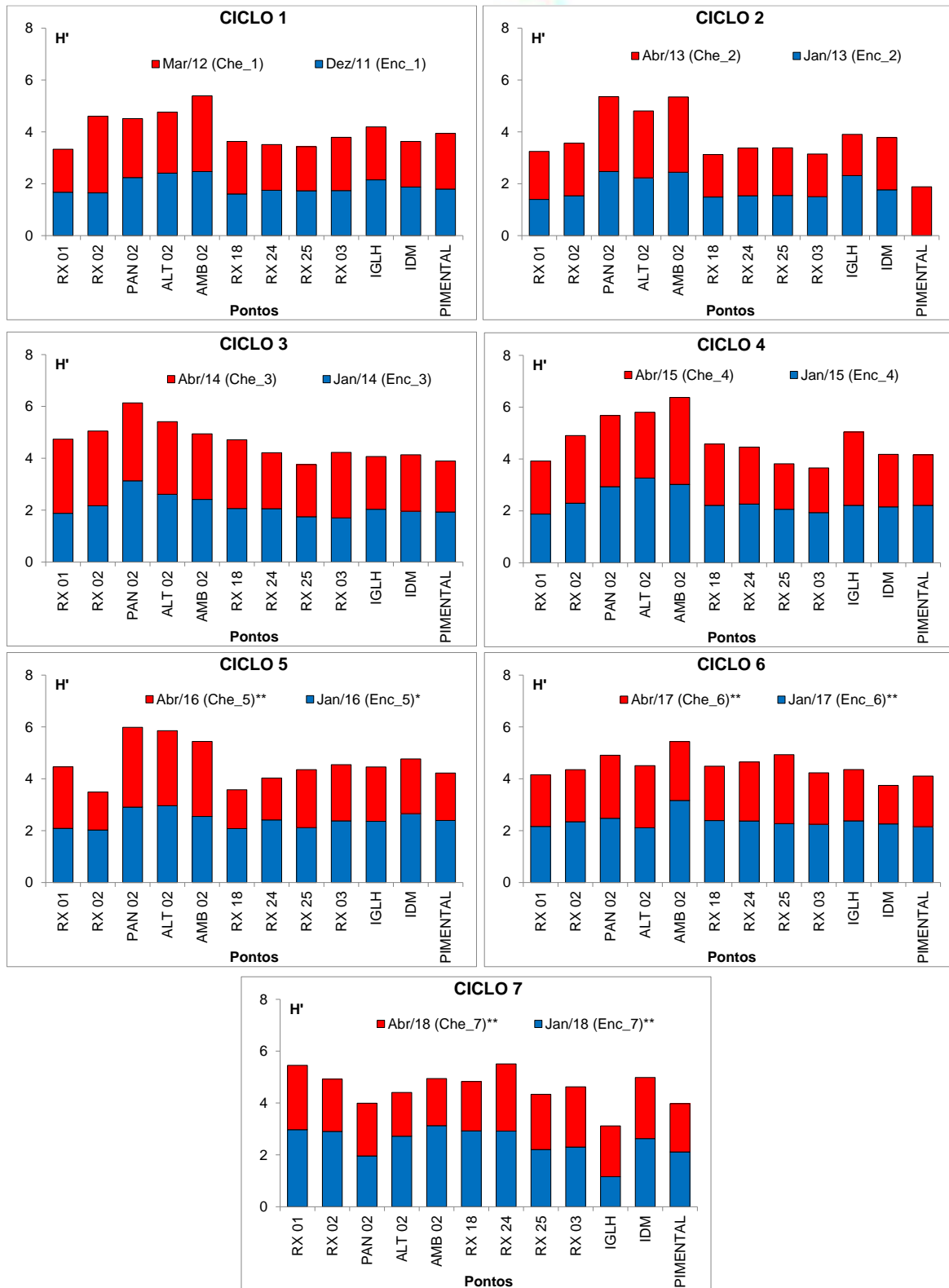
Figura 11.4.1 - 51 – Diversidade de Shannon-Wiener ( H' , bits/indivíduo) da comunidade fitoplanctônica acumulada de organismos fitoplanctônicos nos pontos localizados na Área do Reservatório Xingu (RX) nos sete ciclos hidrológicos de enchente e cheia (dezembro 2011 a abril de 2018). Ciclo 1: 2011/2012; Ciclo 2: 2013; Ciclo 3: 2014; Ciclo 4: 2015; Ciclo 5: 2016; Ciclo 6: 2017; Ciclo 7: 2018. *: fase de enchimento; **: fase de operação.
