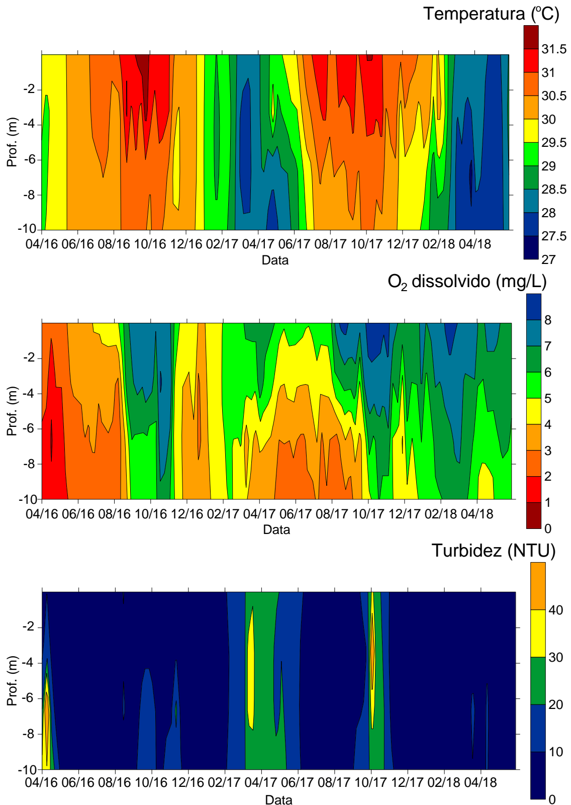
Figura 11.4.1 - 140 – Gráficos de isolinhas de temperatura, oxigênio dissolvido e turbidez no ponto Canal de Fuga-J, localizado próximo à foz do Canal de Fuga no rio Xingu (abril de 2016 a maio de 2018).
