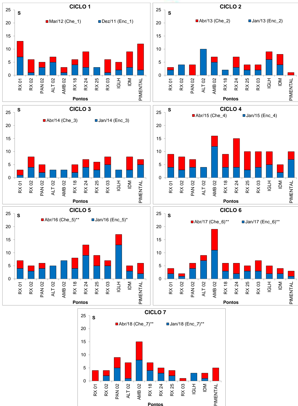
Figura 11.4.1 - 90 – Riqueza total (S) da comunidade bentônica nos pontos localizados na área do Reservatório do Xingu (RX) nos sete ciclos hidrológicos de enchente e cheia (dezembro 2011 a abril de 2018). Ciclo 1: 2011/2012; Ciclo 2: 2013; Ciclo 3: 2014; Ciclo 4: 2015; Ciclo 5: 2016; Ciclo 6: 2017; Ciclo 7: 2018. *: fase de enchimento; **: fase de operação.
