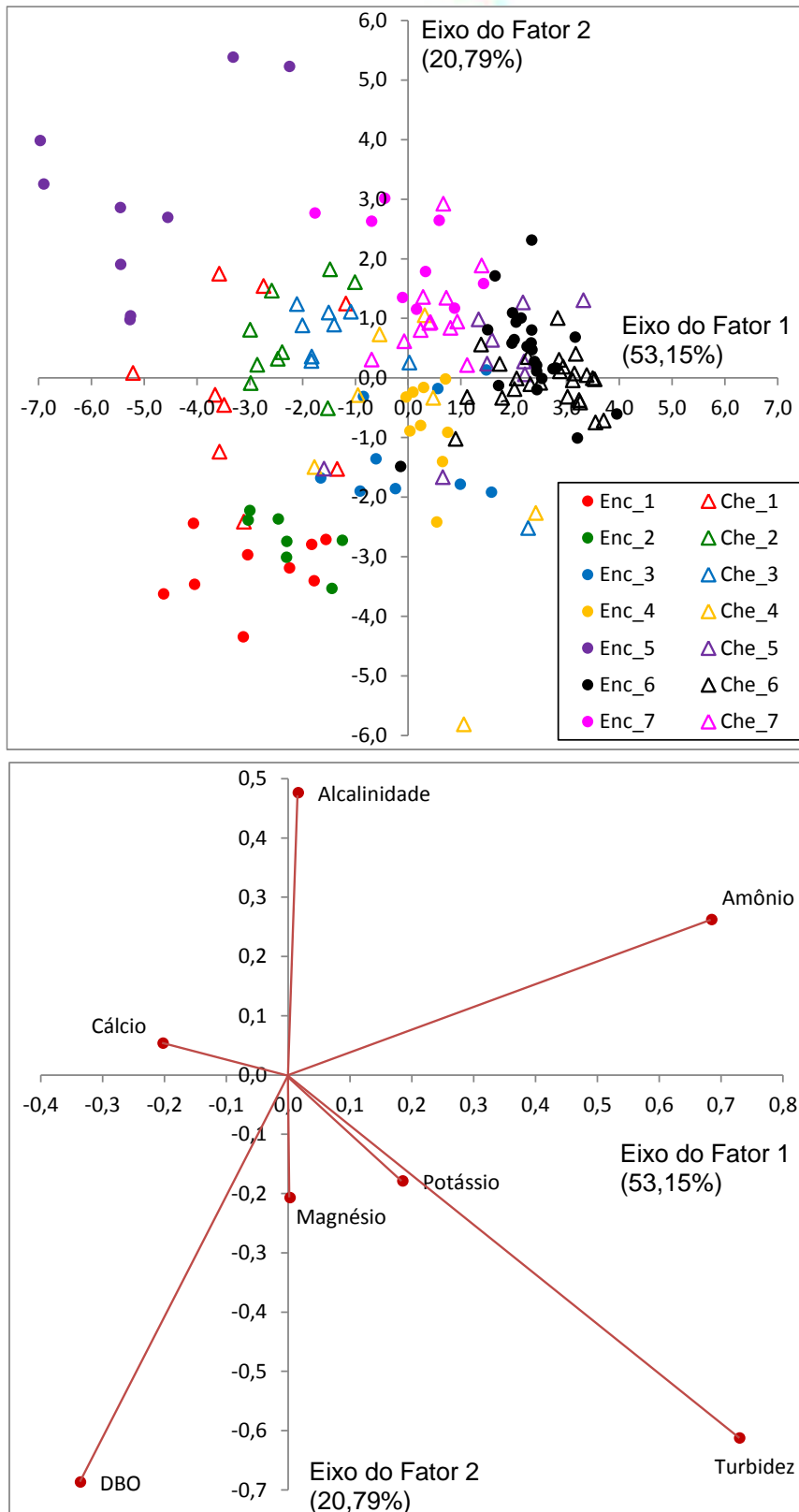
Figura 11.4.1 - 4 – Representação gráfica da Análise de Discriminante e vetores obtidos por meio das variáveis de qualidade da água nos pontos de coleta localizados na área do Reservatório do Xingu nos sete ciclos hidrológicos de enchente e cheia (dezembro de 2011 a abril de 2018).
