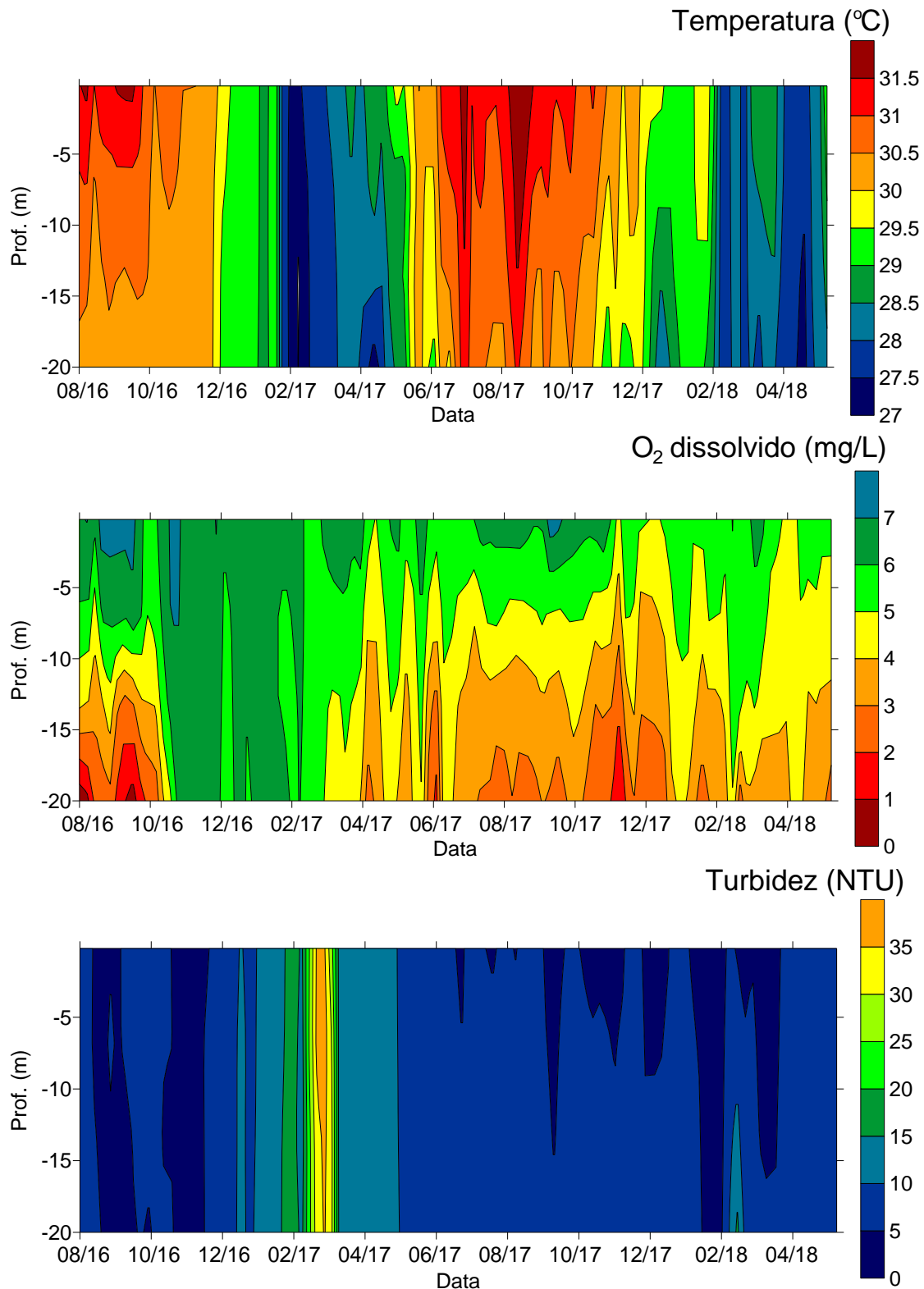
Figura 11.4.1 - 129 – Gráficos de isolinhas de temperatura, oxigênio dissolvido e turbidez no ponto CN 01, localizado no RI, na bacia do igarapé Paquiçamba, aproximadamente 20 km a montante da Casa de Força Principal em de Belo Monte (agosto de 2016 a maio de 2018).
