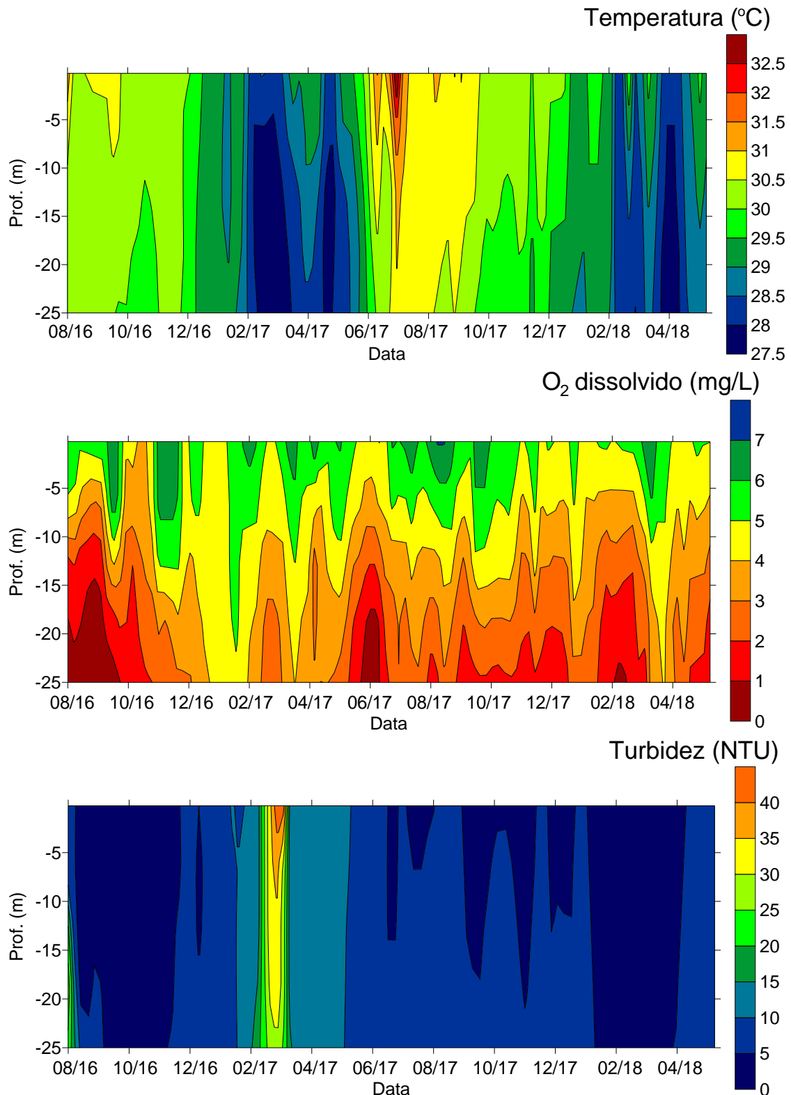
Figura 11.4.1 - 136 – Gráficos de isolinhas de temperatura, oxigênio dissolvido e turbidez no ponto CN 08, localizado no RI, na bacia do igarapé Aturiá, 8,5 km a montante da Casa de Força Principal em Belo Monte (agosto de 2016 a maio de 2018).
