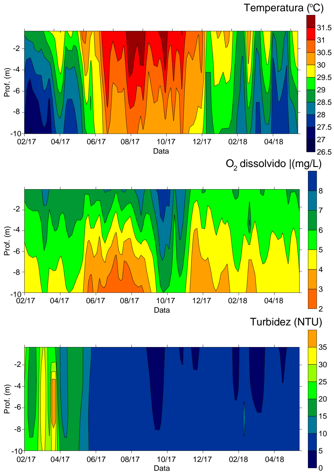
Figura 11.4.1 - 154 – Gráficos de isolinhas de temperatura, oxigênio dissolvido e turbidez no ponto RX-RB-09, próximo às comunidades ribeirinhas do entorno do reservatório do Xingu (fevereiro de 2017 a maio de 2018).
