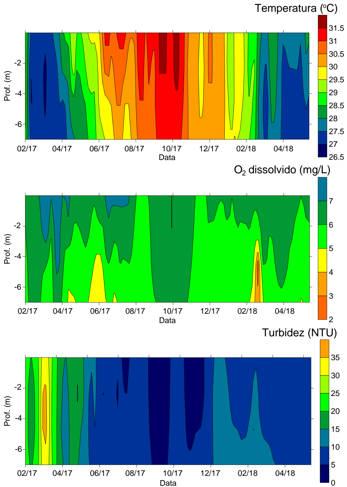
Figura 11.4.1 - 145 – Gráficos de isolinhas de temperatura, oxigênio dissolvido e turbidez no ponto RX-RB-01-M, próximo às comunidades ribeirinhas do entorno do reservatório do Xingu (fevereiro de 2017 a maio de 2018).
