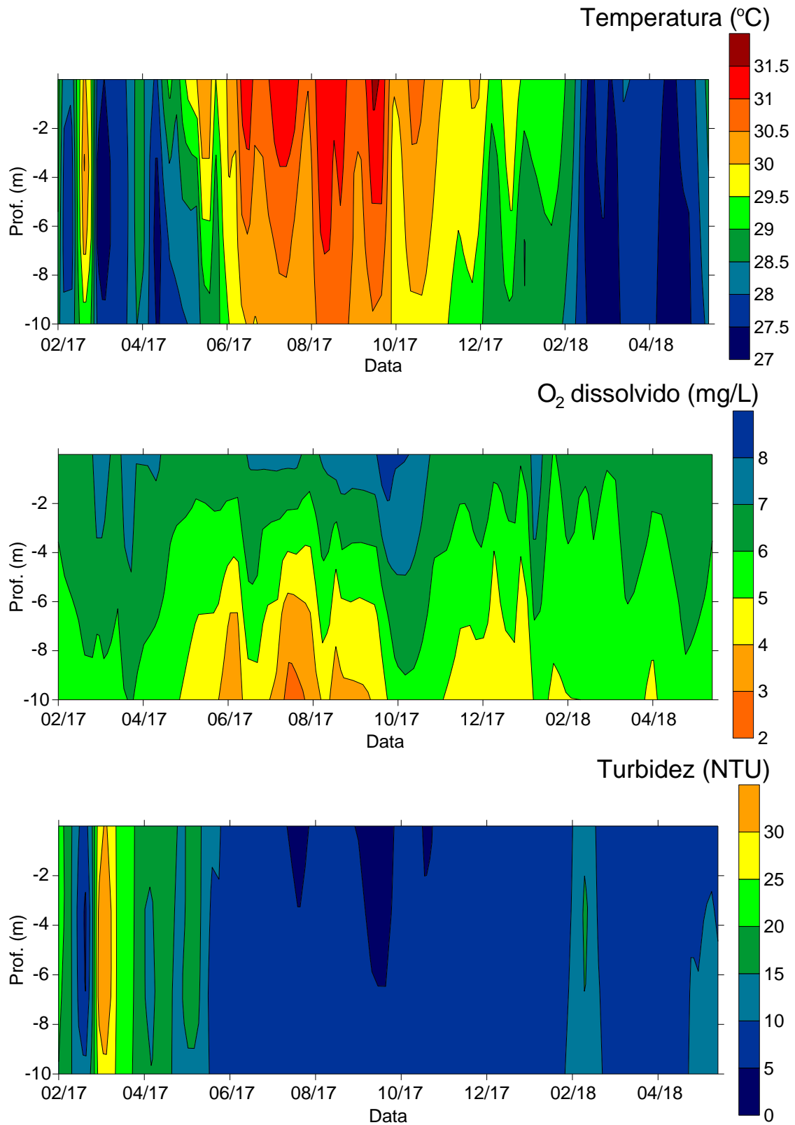
Figura 11.4.1 - 148 – Gráficos de isolinhas de temperatura, oxigênio dissolvido e turbidez no ponto RX-RB-03, próximo às comunidades ribeirinhas do entorno do reservatório do Xingu (fevereiro de 2017 a maio de 2018).
