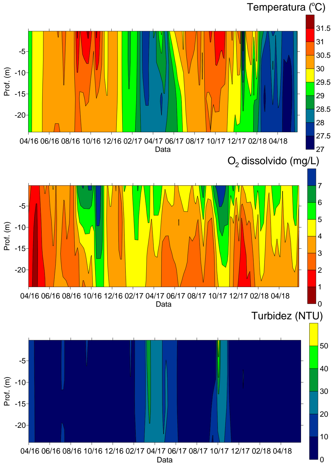
Figura 11.4.1 - 139 – Gráficos de isolinhas de temperatura, oxigênio dissolvido e turbidez no ponto Canal de Fuga-M, localizado junto à barragem de Belo Monte (abril de 2016 a maio de 2018).
