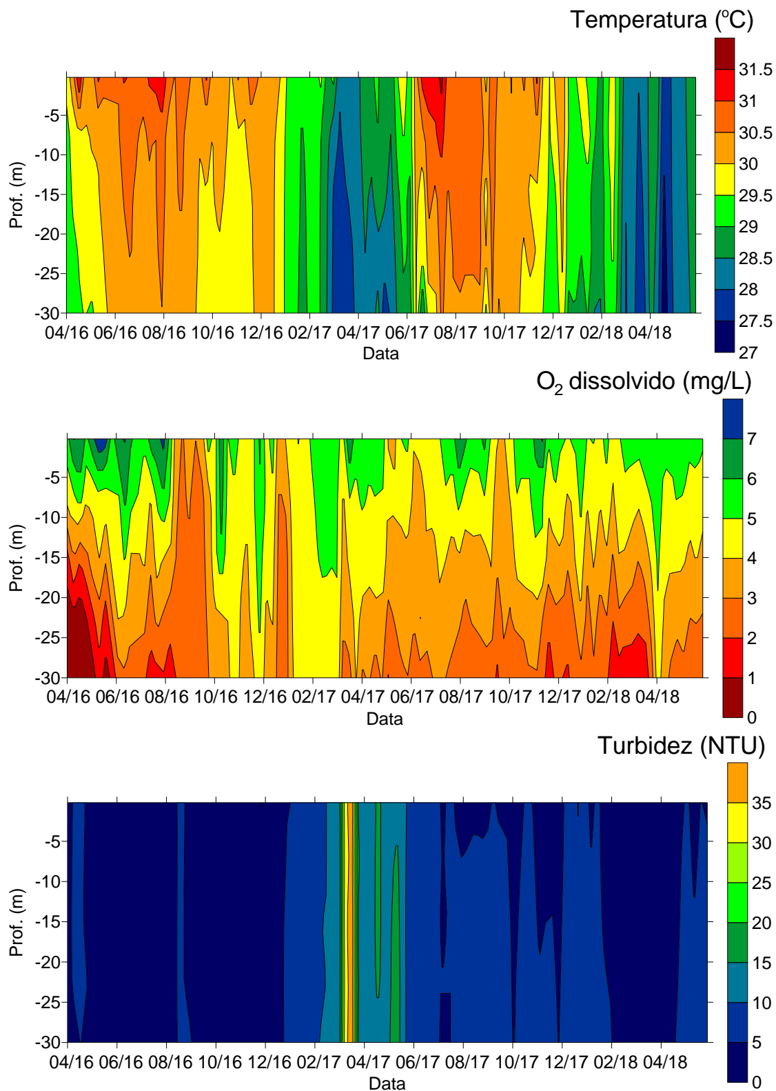
Figura 11.4.1 - 124 – Gráficos de isolinhas de temperatura, oxigênio dissolvido e turbidez no ponto CN 09, localizado no RI, próximo à tomada d' água, na porção central da barragem (abril de 2016 a maio de 2018).
