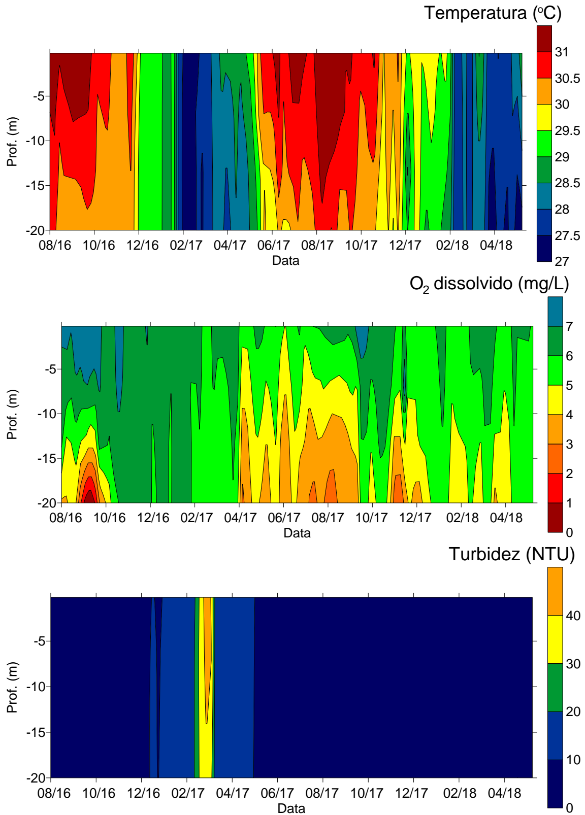
Figura 11.4.1 - 128 – Gráficos de isolinhas de temperatura, oxigênio dissolvido e turbidez no ponto Travessão 27, localizado no Canal de Derivação do RI, próximo à ponte do Travessão 27 (agosto de 2016 a maio de 2018).
