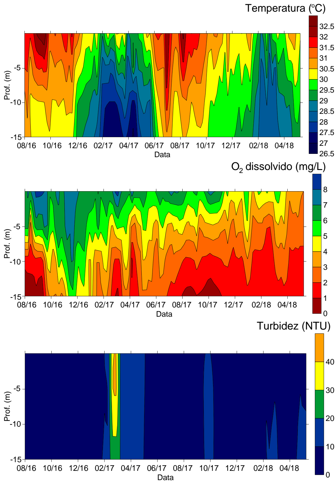
Figura 11.4.1 - 130 – Gráficos de isolinhas de temperatura, oxigênio dissolvido e turbidez no ponto CN 02, localizado no RI, na bacia do igarapé Ticaruca, 18 km a montante do da Casa de Força Principal em Belo Monte (agosto de 2016 a maio de 2018).
