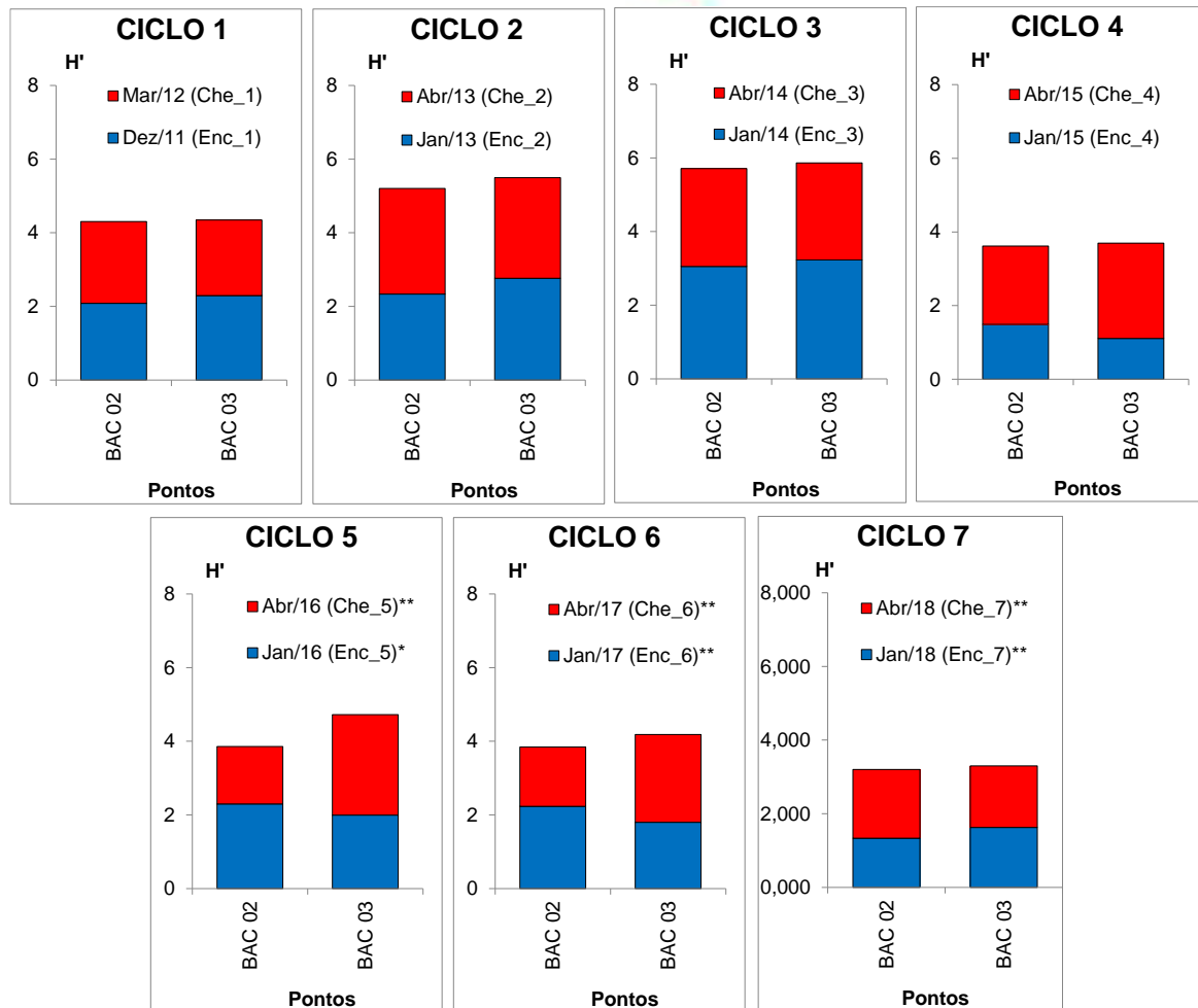
Figura 11.4.1 - 88 – Diversidade de Shannon-Wiener ( H' , bits/indivíduo) da comunidade zooplânctônica acumulada nos pontos localizados na área do Rio Bacajá nos sete ciclos hidrológicos de enchente e cheia (dezembro 2011 a abril de 2018). Ciclo 1: 2011/2012; Ciclo 2: 2013; Ciclo 3: 2014; Ciclo 4: 2015; Ciclo 5: 2016; Ciclo 6: 2017; Ciclo 7: 2018. *: fase de enchimento; **: fase de operação.
