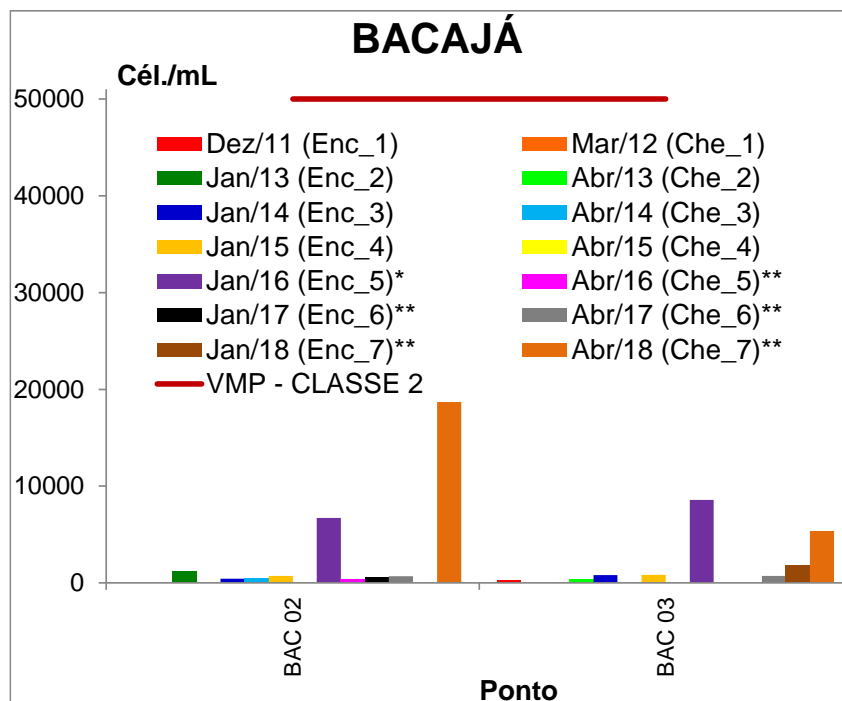
Figura 11.4.1 - 60 – Densidade de cianobactérias (células/mL) nos pontos localizados na área do rio Bacajá nos sete ciclos hidrológicos de enchente e cheia (dezembro 2011 a abril de 2018). *: fase de enchimento; **: fase de operação. VMP – CLASSE 2: limite estabelecido pela Resolução CONAMA nº 357/2005 para águas doces de classe 2.
