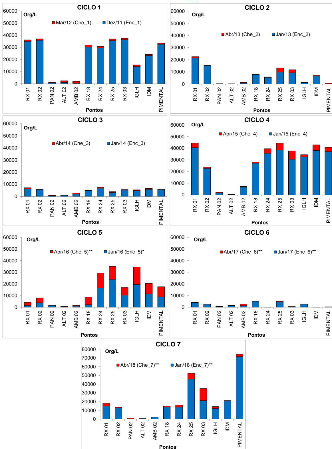
Figura 11.4.1 - 44 – Abundância de organismos fitoplanctônicos nos pontos localizados na Área do Reservatório Xingu (RX) nos sete ciclos hidrológicos de enchente e cheia (dezembro 2011 a abril de 2018). Ciclo 1: 2011/2012; Ciclo 2: 2013; Ciclo 3: 2014; Ciclo 4: 2015; Ciclo 5: 2016; Ciclo 6: 2017; Ciclo 7: 2018. *: fase de enchimento; **: fase de operação.
