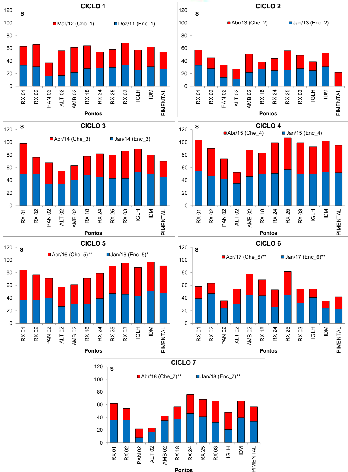
Figura 11.4.1 - 34 – Riqueza total (S) do fitoplâncton (gêneros) acumulada nos pontos localizados na Área do Reservatório Xingu (RX). Campanhas nos sete ciclos hidrológicos de enchente e cheia (dezembro 2011 a abril de 2018). Ciclo 1: 2011/2012; Ciclo 2: 2013; Ciclo 3: 2014; Ciclo 4: 2015; Ciclo 5: 2016; Ciclo 6: 2017; Ciclo 7: 2018. *: fase de enchimento; **: fase de operação.
