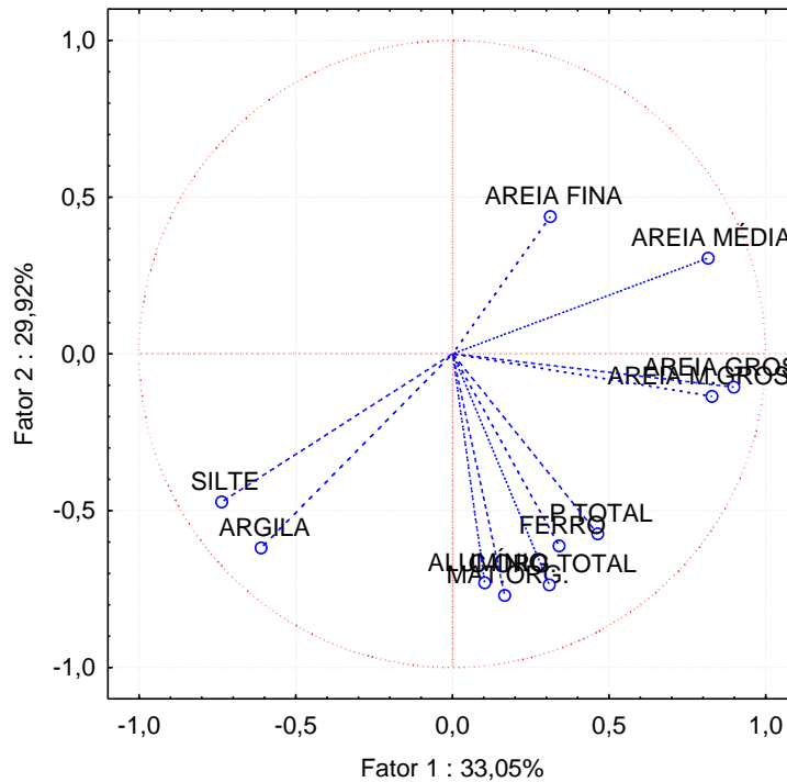
Projeção dos pontos de coleta de sedim. no plano fatorial (1 x 2) Igarapés de Altamira - RX
