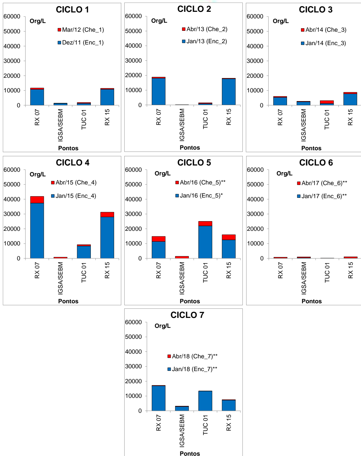
Figura 11.4.1 - 46 – Abundância de organismos fitoplanctônicos nos pontos localizados na área do Trecho de Restituição de Vazão (TRV) nos sete ciclos hidrológicos de enchente e cheia (dezembro 2011 a abril de 2018). Ciclo 1: 2011/2012; Ciclo 2: 2013; Ciclo 3: 2014; Ciclo 4: 2015; Ciclo 5: 2016; Ciclo 6: 2017; Ciclo 7: 2018. *: fase de enchimento; **: fase de operação.
