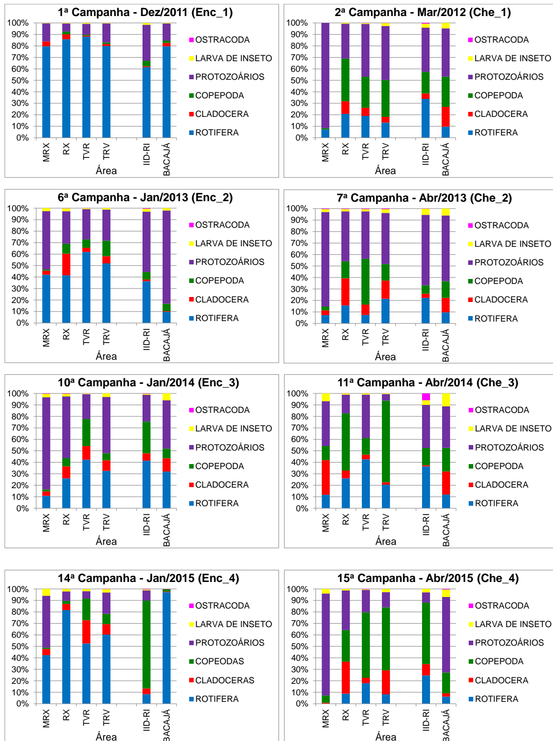
Figura 11.4.1 - 72 – Abundâncias relativas totais (%) das Classes de zooplâncton registradas nas áreas a Montante do Reservatório do Xingu (MRX), Reservatório do Xingu (RX), Trecho de Vazão Reduzida (TVR), Rio Bacajá (BACAJÁ), Trecho de Restituição de Vazão (TRV) e Igarapés Interceptados pelos Diques do Reservatório Intermediário (IID-RI) nas campanhas trimestrais do 1º ao 4º ciclo hidrológico de enchente e cheia (dezembro de 2011 a abril de 2015), durante a fase de pré-enchimento.
