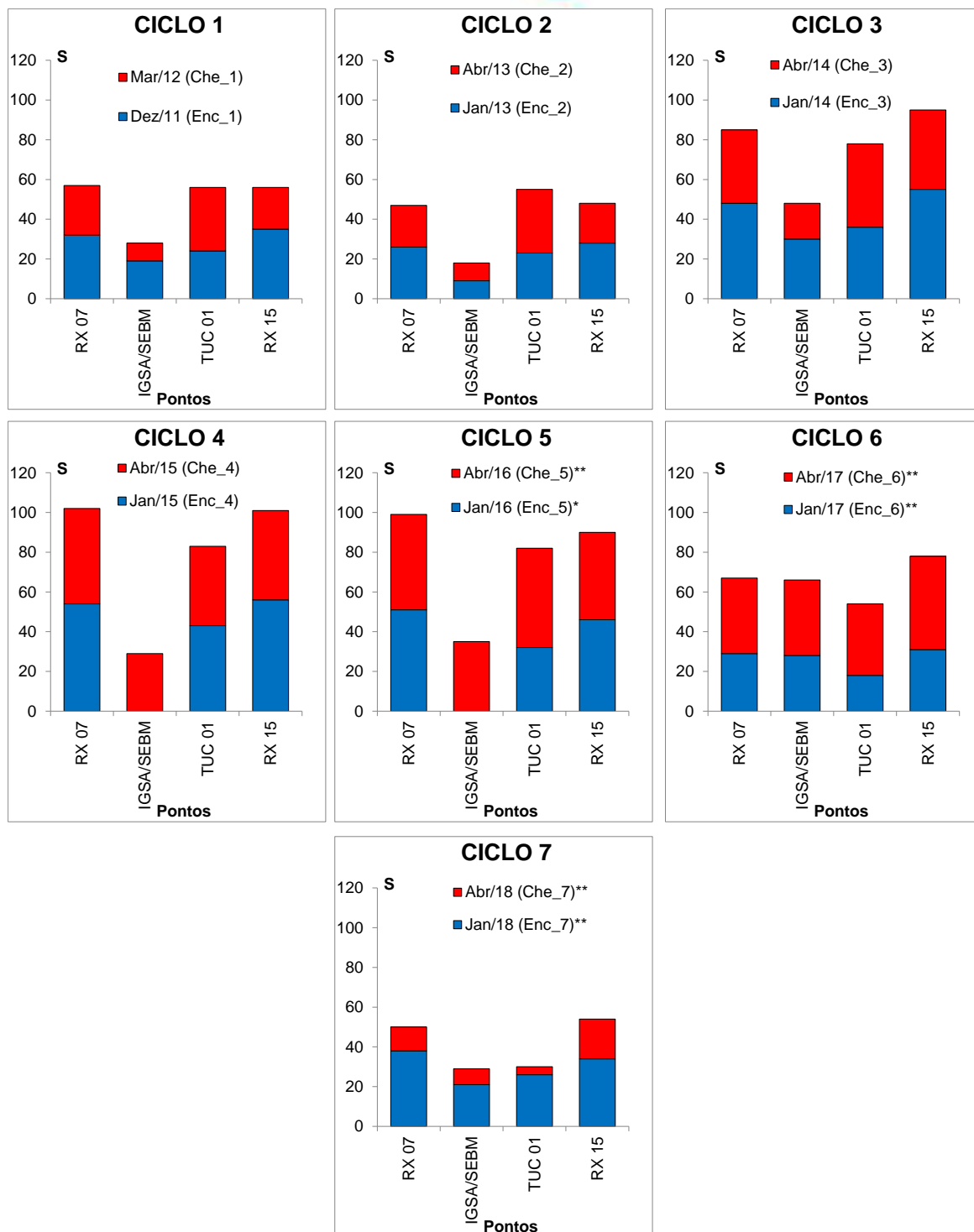
Figura 11.4.1 - 36 – Riqueza total (S) do fitoplâncton (gêneros) acumulada nos pontos localizados na área do Trecho de Restituição de Vazão (TRV). Campanhas nos sete ciclos hidrológicos de enchente e cheia (dezembro 2011 a abril de 2018). Ciclo 1: 2011/2012; Ciclo 2: 2013; Ciclo 3: 2014; Ciclo 4: 2015; Ciclo 5: 2016; Ciclo 6: 2017; Ciclo 7: 2018. *: fase de enchimento; **: fase de operação.
