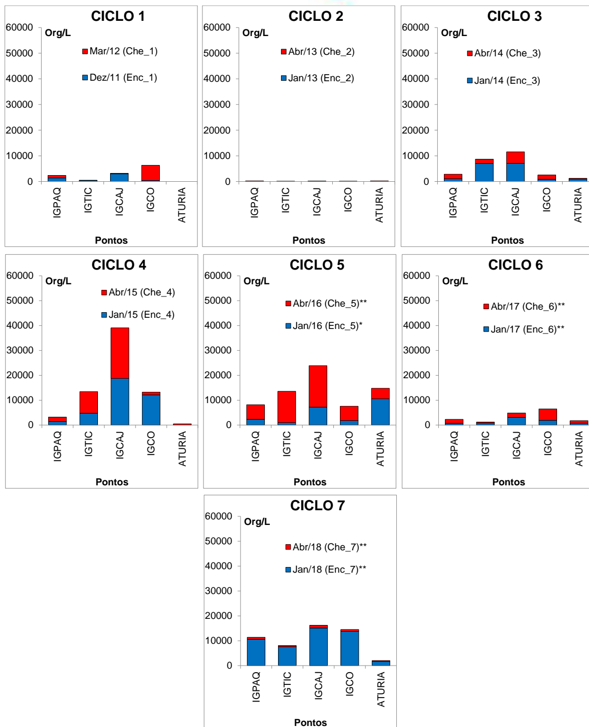
Figura 11.4.1 - 48 – Abundância de organismos fitoplanctônicos nos pontos localizados nos Igarapés Interceptados pelos Diques do RI (IID-RI nos sete ciclos hidrológicos de enchente e cheia (dezembro 2011 a abril de 2018). Ciclo 1: 2011/2012; Ciclo 2: 2013; Ciclo 3: 2014; Ciclo 4: 2015; Ciclo 5: 2016; Ciclo 6: 2017; Ciclo 7: 2018. *: fase de enchimento; **: fase de operação.
