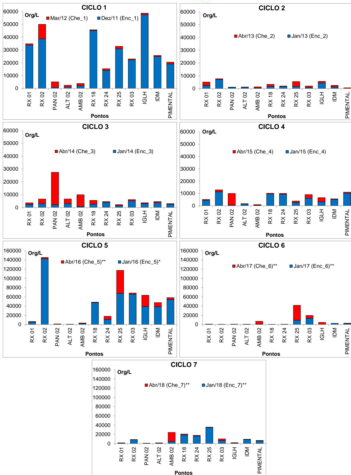
Figura 11.4.1 - 76 – Abundância de organismos zooplancônicos nos pontos localizados na Área do Reservatório do Xingu (RX) nos sete ciclos hidrológicos de enchente e cheia (dezembro 2011 a abril de 2018). Ciclo 1: 2011/2012; Ciclo 2: 2013; Ciclo 3: 2014; Ciclo 4: 2015; Ciclo 5: 2016; Ciclo 6: 2017; Ciclo 7: 2018. *: fase de enchimento; **: fase de operação.
