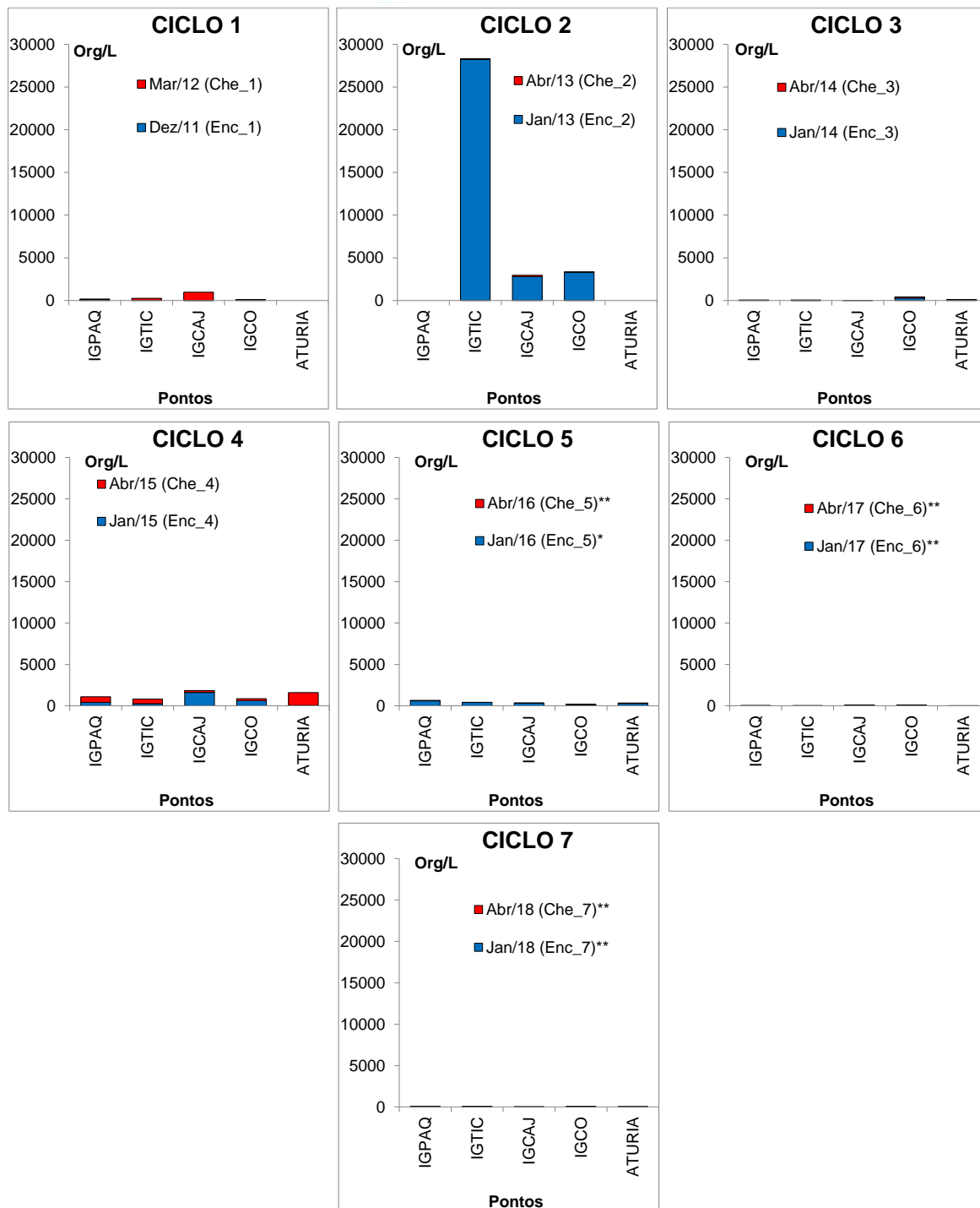
Figura 11.4.1 - 101 – Abundância (org/m 2 ) da comunidade bentônica nos pontos localizados nos Igarapés Interceptados pelos Diques do RI (IID-RI) nos sete ciclos hidrológicos de enchente e cheia (dezembro 2011 a abril de 2018). Ciclo 1: 2011/2012; Ciclo 2: 2013; Ciclo 3: 2014; Ciclo 4: 2015; Ciclo 5: 2016; Ciclo 6: 2017; Ciclo 7: 2018. *: fase de enchimento; **: fase de operação.
