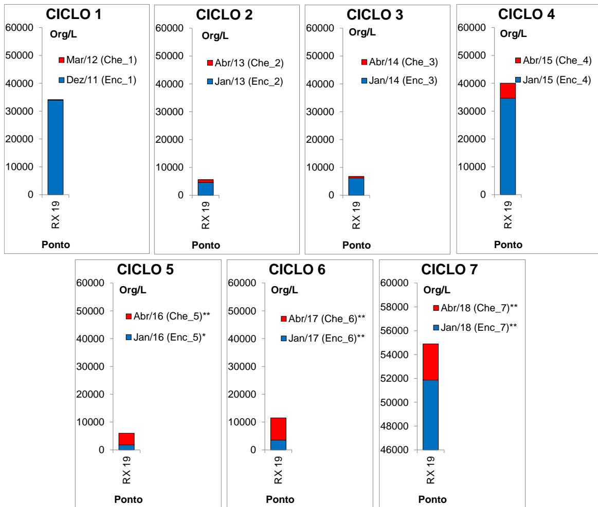
Figura 11.4.1 - 43 – Abundância de organismos fitoplanctônicos no ponto RX 19, localizado na Área a Montante do Reservatório Xingu (MRX) nos sete ciclos hidrológicos de enchente e cheia (dezembro 2011 a abril de 2018). Ciclo 1: 2011/2012; Ciclo 2: 2013; Ciclo 3: 2014; Ciclo 4: 2015; Ciclo 5: 2016; Ciclo 6: 2017; Ciclo 7: 2018. *: fase de enchimento; **: fase de operação.
