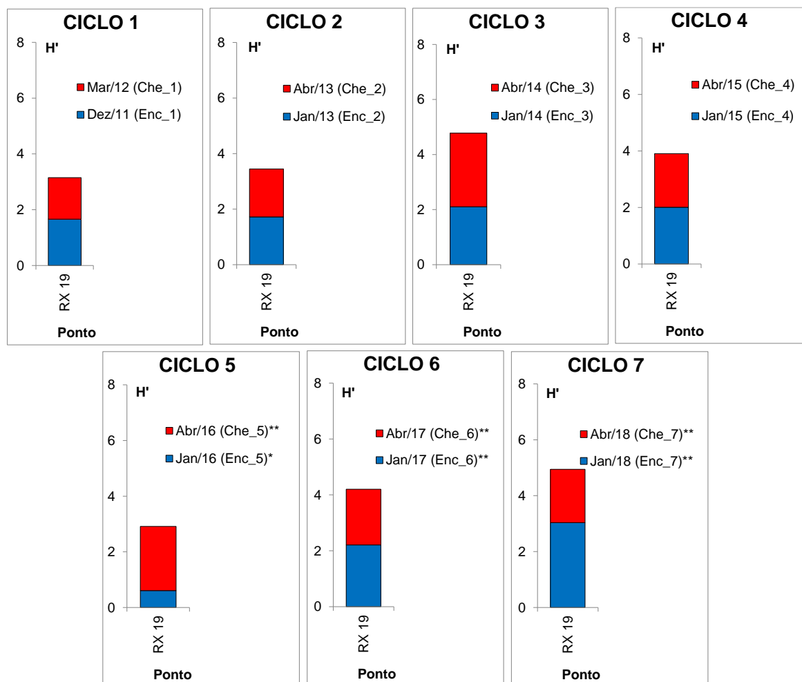
Figura 11.4.1 - 50 – Diversidade de Shannon-Wiener (H', bits/indivíduo) da comunidade fitoplanctônica acumulada no ponto RX 19, localizado na Área a Montante do Reservatório Xingu (MRX) nos sete ciclos hidrológicos de enchente e cheia (dezembro 2011 a abril de 2018). Ciclo 1: 2011/2012; Ciclo 2: 2013; Ciclo 3:
