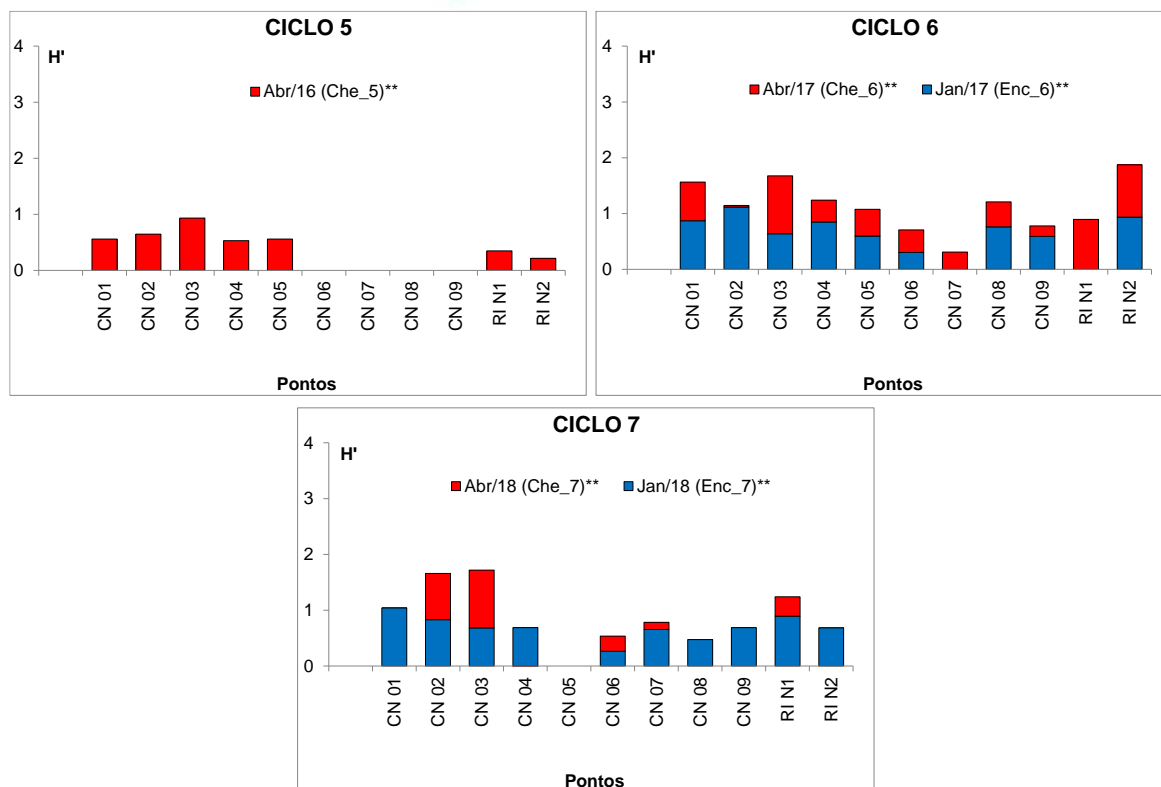
Figura 11.4.1 - 107 – Diversidade de Shannon-Wiener ( H' , bits/indivíduo) da comunidade bentônica nos pontos localizados no Reservatório Intermediário no 5º ao 7º ciclo hidrológico de enchente e cheia, durante a fase de operação (abril de 2016 a abril de 2018).
