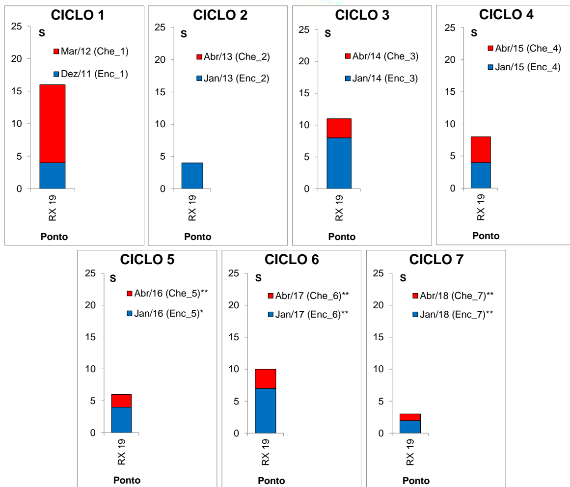
Figura 11.4.1 - 89 – Riqueza total (S) da comunidade bentônica no ponto RX 19, localizado na área a Montante do Reservatório do Xingu (MRX) nos sete ciclos hidrológicos de enchente e cheia (dezembro 2011 a abril de 2018). Ciclo 1: 2011/2012; Ciclo 2: 2013; Ciclo 3: 2014; Ciclo 4: 2015; Ciclo 5: 2016; Ciclo 6: 2017; Ciclo 7: 2018. *: fase de enchimento; **: fase de operação.
