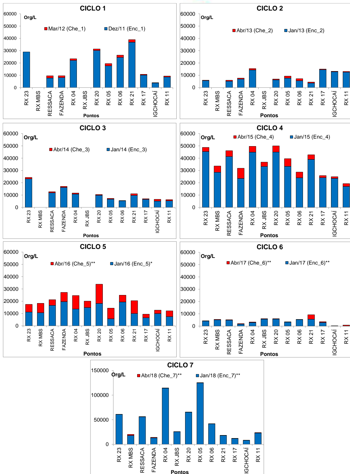
Figura 11.4.1 - 45 – Abundância de organismos fitoplanctônicos nos pontos localizados na Área do Trecho de Vazão Reduzida (TVR) nos sete ciclos hidrológicos de enchente e cheia (dezembro 2011 a abril de 2018). Ciclo 1: 2011/2012; Ciclo 2: 2013; Ciclo 3: 2014; Ciclo 4: 2015; Ciclo 5: 2016; Ciclo 6: 2017; Ciclo 7: 2018. *: fase de enchimento; **: fase de operação.
