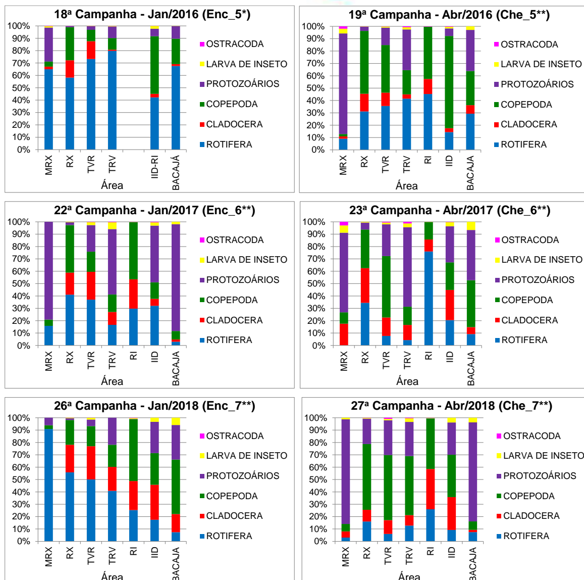
Figura 11.4.1 - 74 – Abundâncias relativas totais (%) das Classes de zooplâncton registradas nas áreas Montante do Reservatório do Xingu (MRX), Reservatório do Xingu (RX), Trecho de Vazão Reduzida (TVR), Rio Bacajá (BACAJÁ), Trecho de Restituição de Vazão (TRV) e Igarapés Interceptados pelos Diques do Reservatório Intermediário (IID-RI) nas campanhas trimestrais do 5º ao 7º ciclo hidrológico de enchente e cheia (janeiro de 2016 a abril de 2018). *: fase de enchimento; **: fase de operação.
