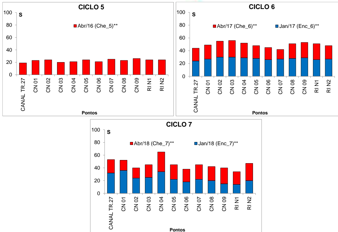
Figura 11.4.1 - 69 – Riqueza total (S) do zooplâncton (espécies) acumulada nos pontos localizados no Reservatório Intermediário (RI) durante o 5º ao 7º ciclo hidrológico de enchente e cheia na fase de operação (abril de 2016 a abril de 2018).
