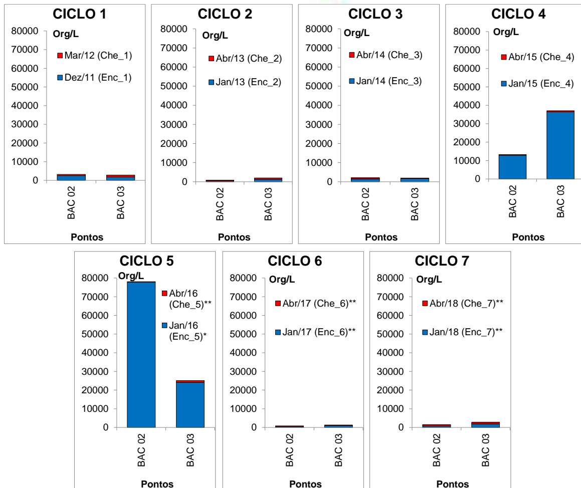
Figura 11.4.1 - 81 – Abundância de organismos zooplanctônicos nos pontos localizados na Área do rio Bacajá nos sete ciclos hidrológicos de enchente e cheia (dezembro 2011 a abril de 2018). Ciclo 1: 2011/2012; Ciclo 2: 2013; Ciclo 3: 2014; Ciclo 4: 2015; Ciclo 5: 2016; Ciclo 6: 2017; Ciclo 7: 2018. *: fase de enchimento; **: fase de operação.
