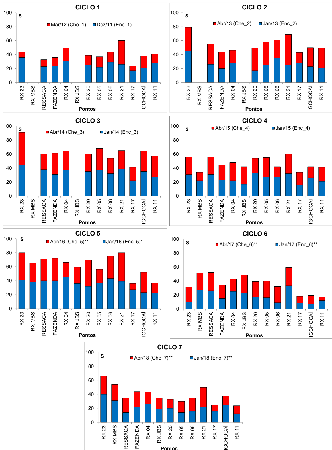
Figura 11.4.1 - 67 – Riqueza total (S) do zooplâncton (espécies) acumulada no ponto localizado na Área do Trecho de Vazão Reduzida (TVR) nos sete ciclos hidrológicos de enchente e cheia (dezembro 2011 a abril de 2018). Ciclo 1: 2011/2012; Ciclo 2: 2013; Ciclo 3: 2014; Ciclo 4: 2015; Ciclo 5: 2016; Ciclo 6: 2017; Ciclo 7: 2018. *: fase de enchimento; **: fase de operação.
