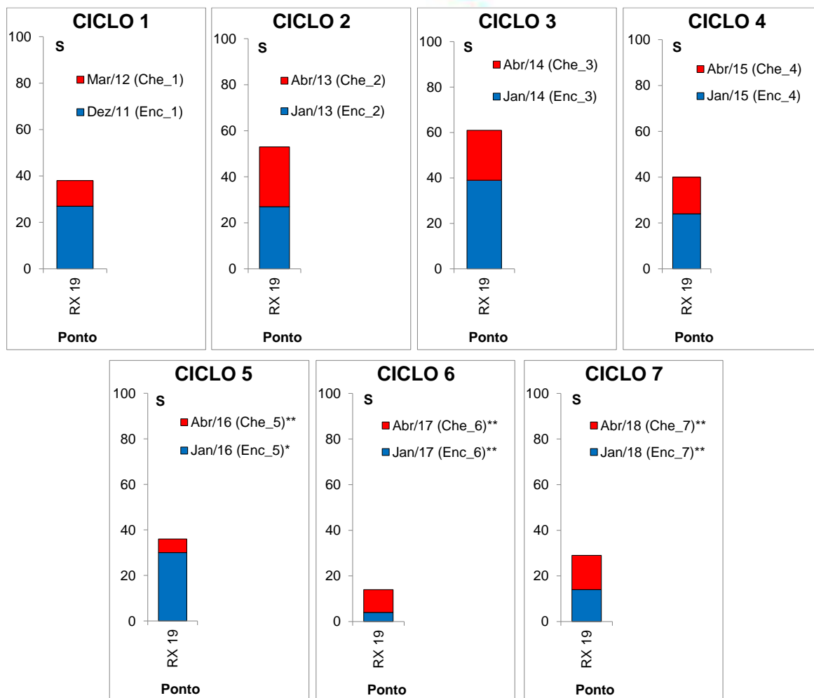
Figura 11.4.1 - 65 – Riqueza total (S) do zooplâncton (espécies) acumulada no ponto RX 19, localizado na Área a Montante do Reservatório Xingu (MRX) nos sete ciclos hidrológicos de enchente e cheia (dezembro 2011 a abril de 2018). Ciclo 1: 2011/2012; Ciclo 2: 2013; Ciclo 3: 2014; Ciclo 4: 2015; Ciclo 5: 2016; Ciclo 6: 2017; Ciclo 7: 2018. *: fase de enchimento; **: fase de operação.
