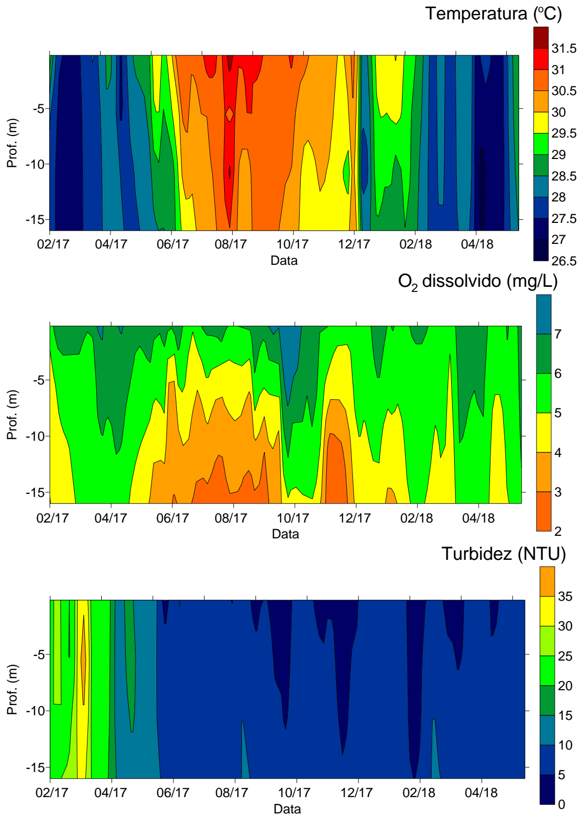
Figura 11.4.1 - 156 – Gráficos de isolinhas de temperatura, oxigênio dissolvido e turbidez no ponto RX-RB-11, próximo às comunidades ribeirinhas do entorno do reservatório do Xingu (fevereiro de 2017 a maio de 2018).
