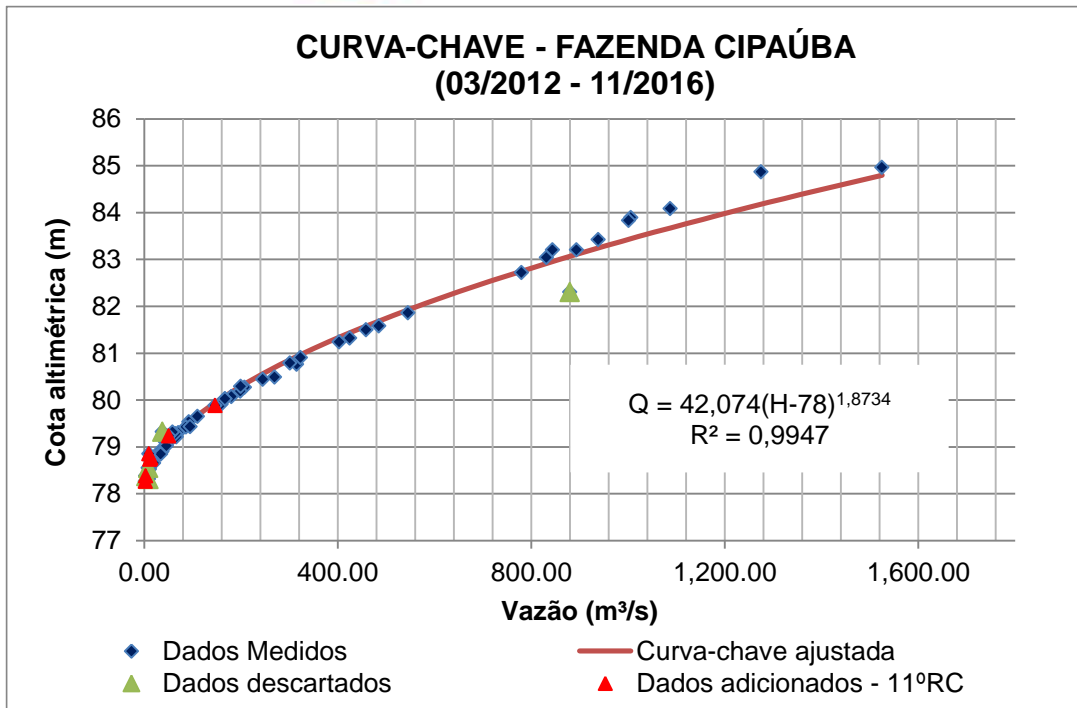
Curva Chave - Rio Bacajá – Estação Fazenda Cipaúba.
