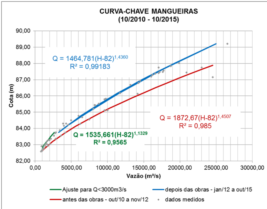
Curva-Chave - Rio Xingu – Estação UHE Belo Monte Mangueiras.
