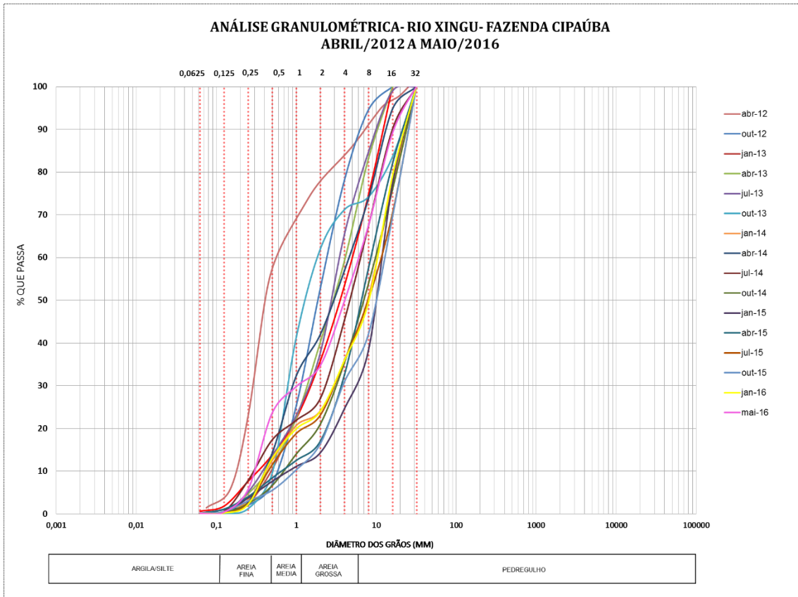
Envoltória das Curvas Granulométricas do Leito do Rio Bacajá - Estação Fazenda Cipaúba.
