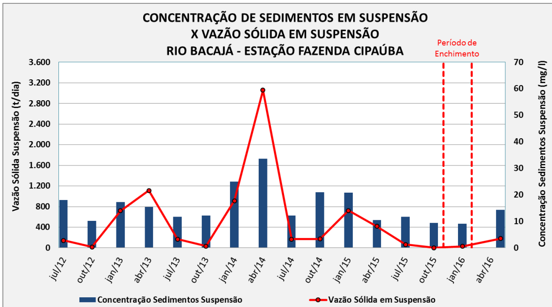
Concentração x Vazão Sólida de Sedimentos em Suspensão Rio Bacajá - Estação Fazenda Cipaúba.
