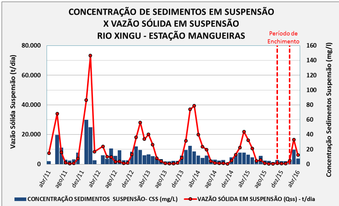
Concentração x Vazão Sólida de Sedimentos em Suspensão Rio Xingu - UHE Belo Monte Mangueiras.
