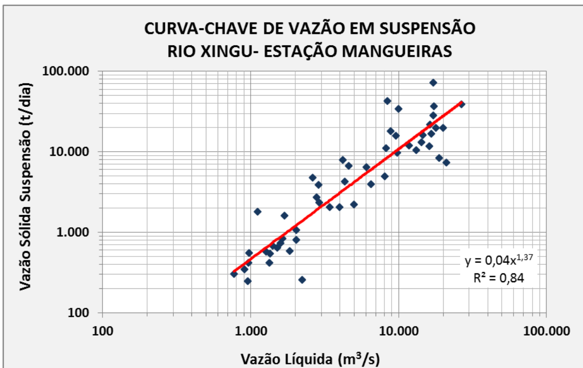
Curva-Chave de Sedimentos em Suspensão Rio Xingu - UHE Belo Monte Mangueiras.
