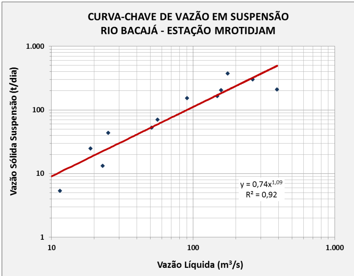
Curva-Chave de Sedimentos em Suspensão Rio Bacajá - Estação Mrotidjã.
