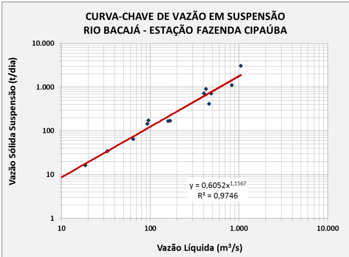
Curva-Chave de Sedimentos em Suspensão Rio Bacajá - Estação Fazenda Cipaúba.
