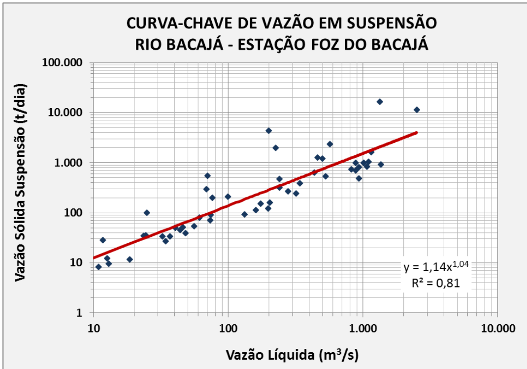
Curva-Chave de Sedimentos em Suspensão - Rio Bacajá – UHE Belo Monte Foz do Bacajá.
