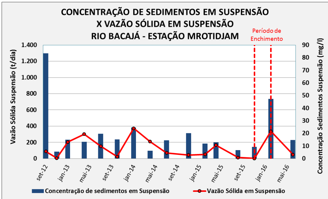
Concentração x Vazão Sólida de Sedimentos em Suspensão Rio Bacajá - Estação Mrotidjâm.
