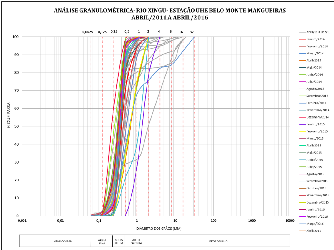
Envoltória das Curvas Granulométricas do Leito - Rio Xingu - Estação UHE Belo Monte Mangueiras.
