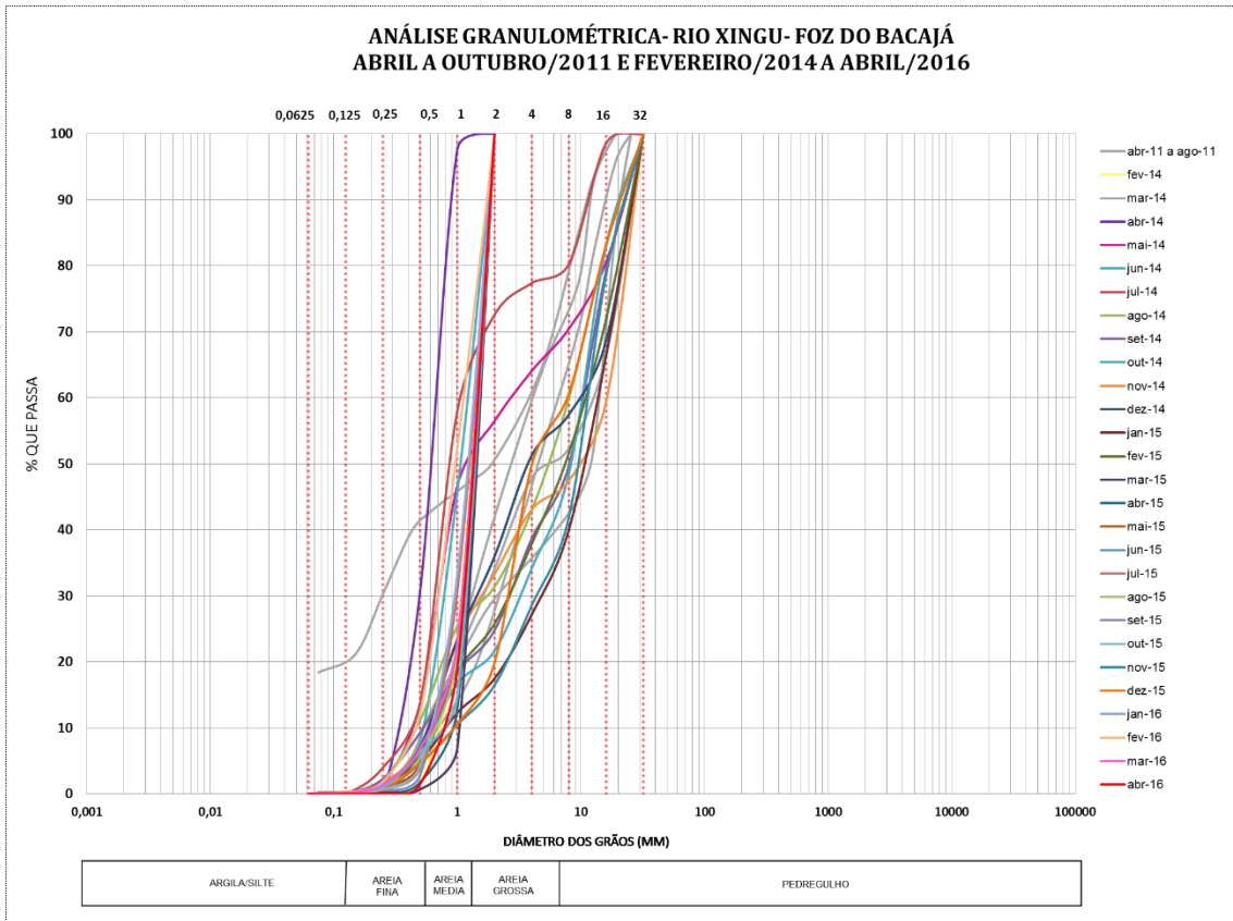
Envoltória das Curvas Granulométricas do Leito do Rio Bacajá - Estação UHE Belo Monte Foz do Bacajá.
