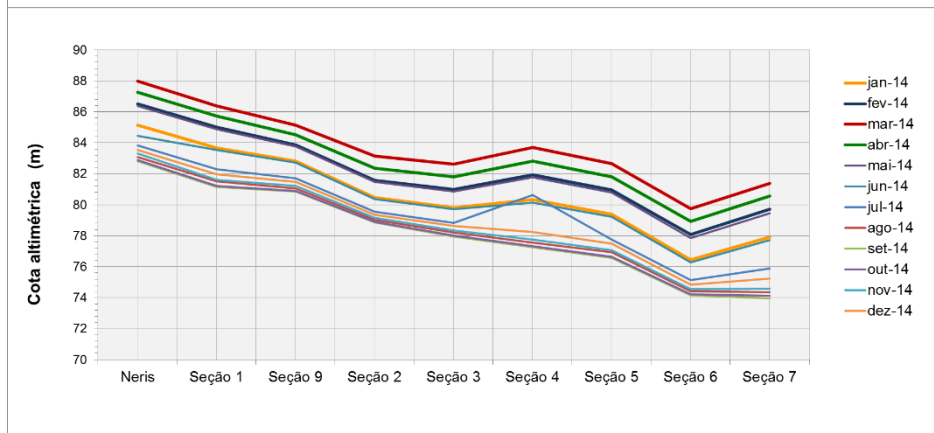
Perfis da Linha D'Água Simultâneos - TVR - Margem Direita.
