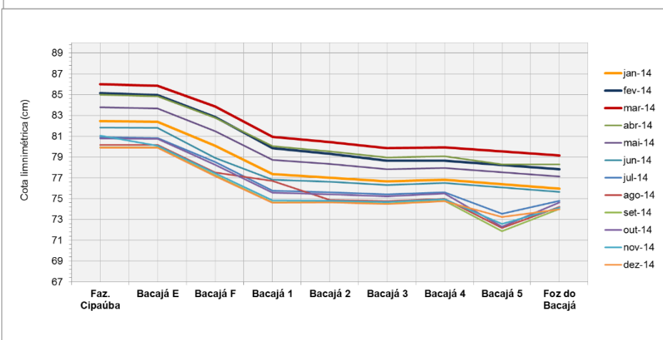
Perfil da Linha d'Água Simultâneo - Rio Bacajá.
