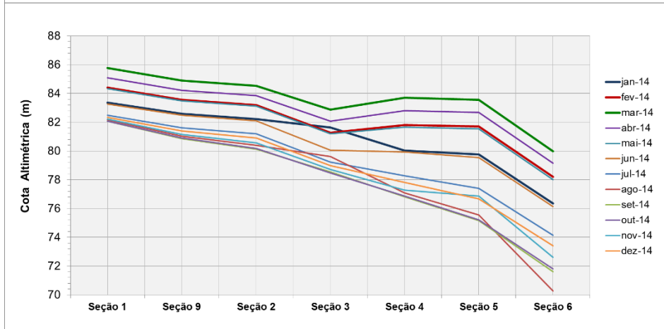
Perfis da Linha d'Água Simultâneo - TVR - Margem Esquerda.
