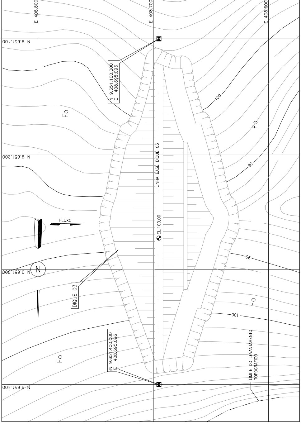
PLANTA 0 10 20 40m ESC. 1:1000
