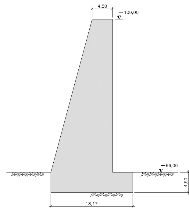
CORTE 2-2
