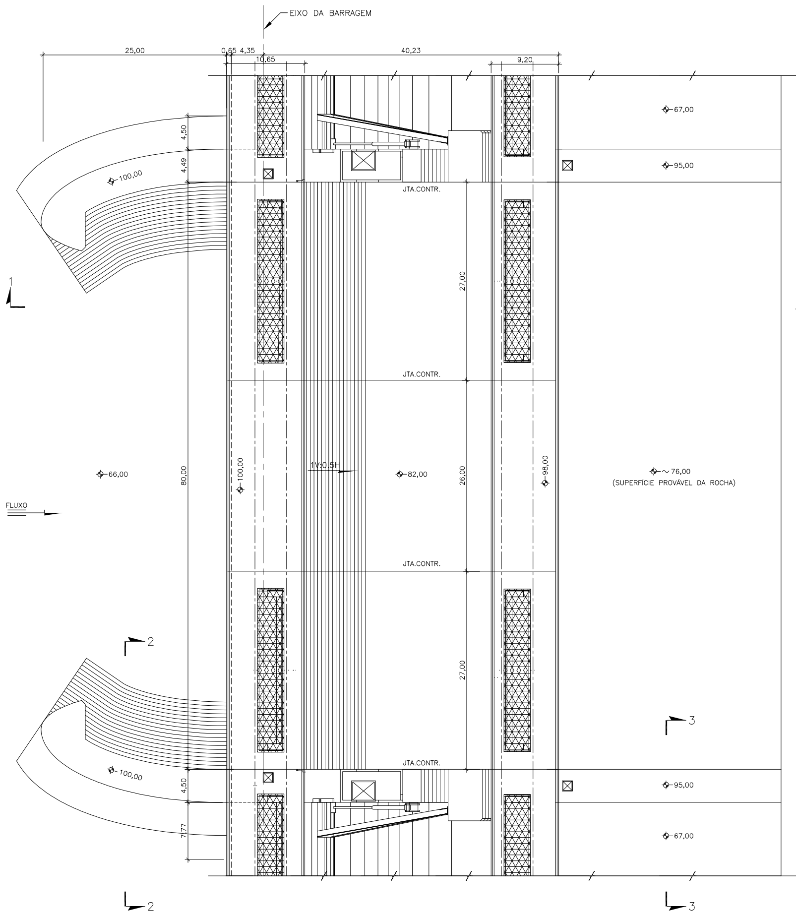
PLANTA NA EL.100,00
