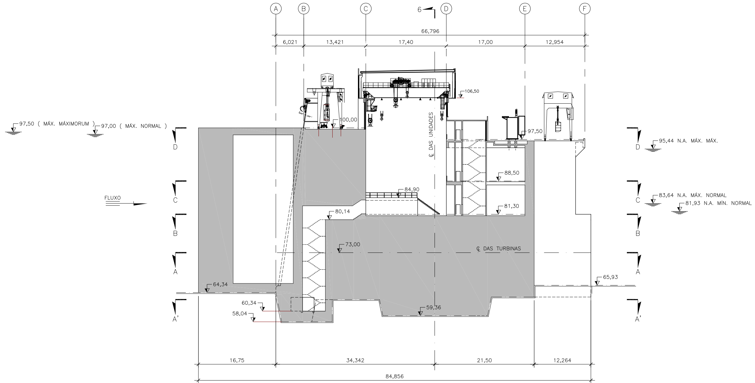
CORTE 1-1
