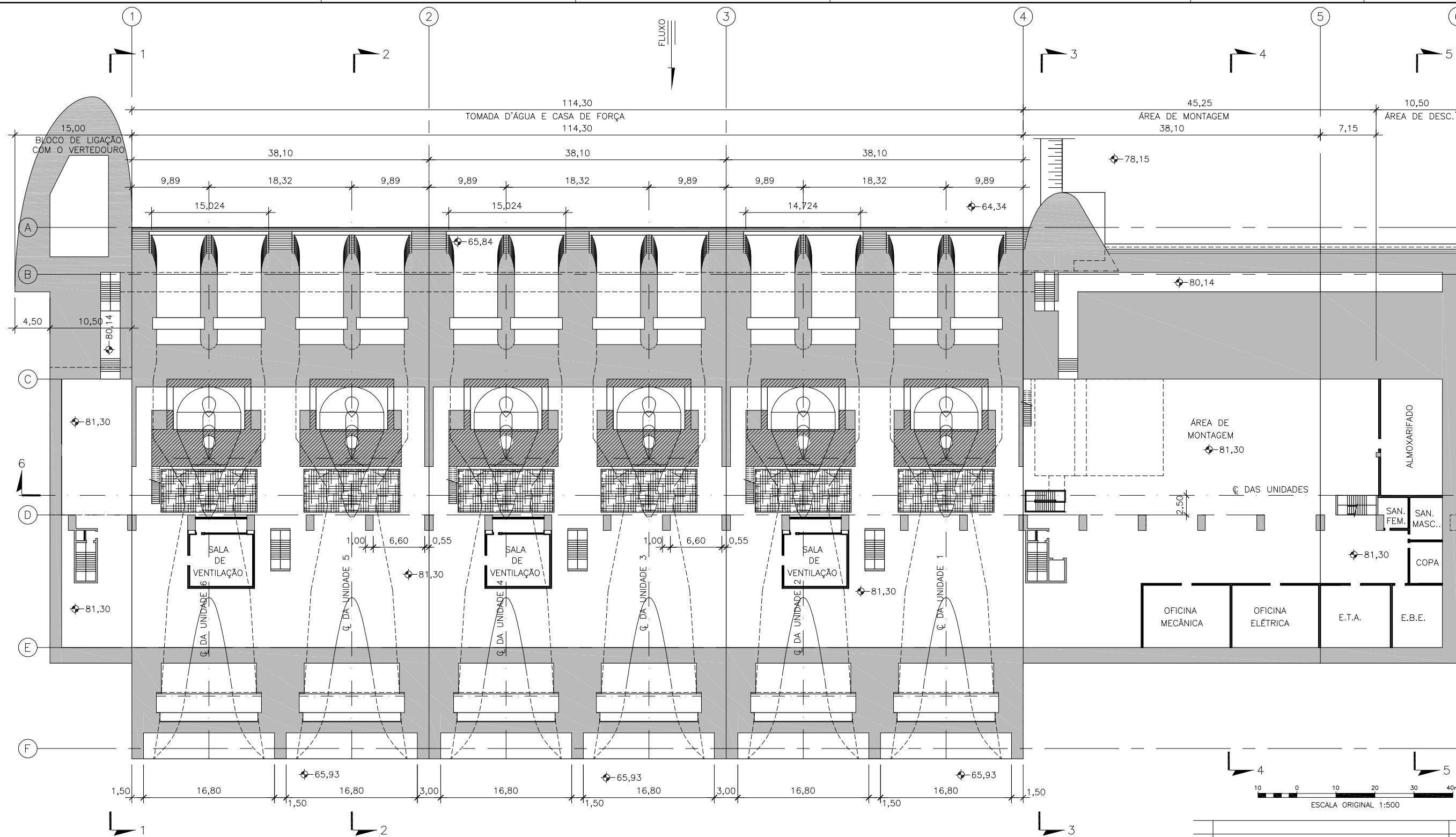
PLANTA B-B
