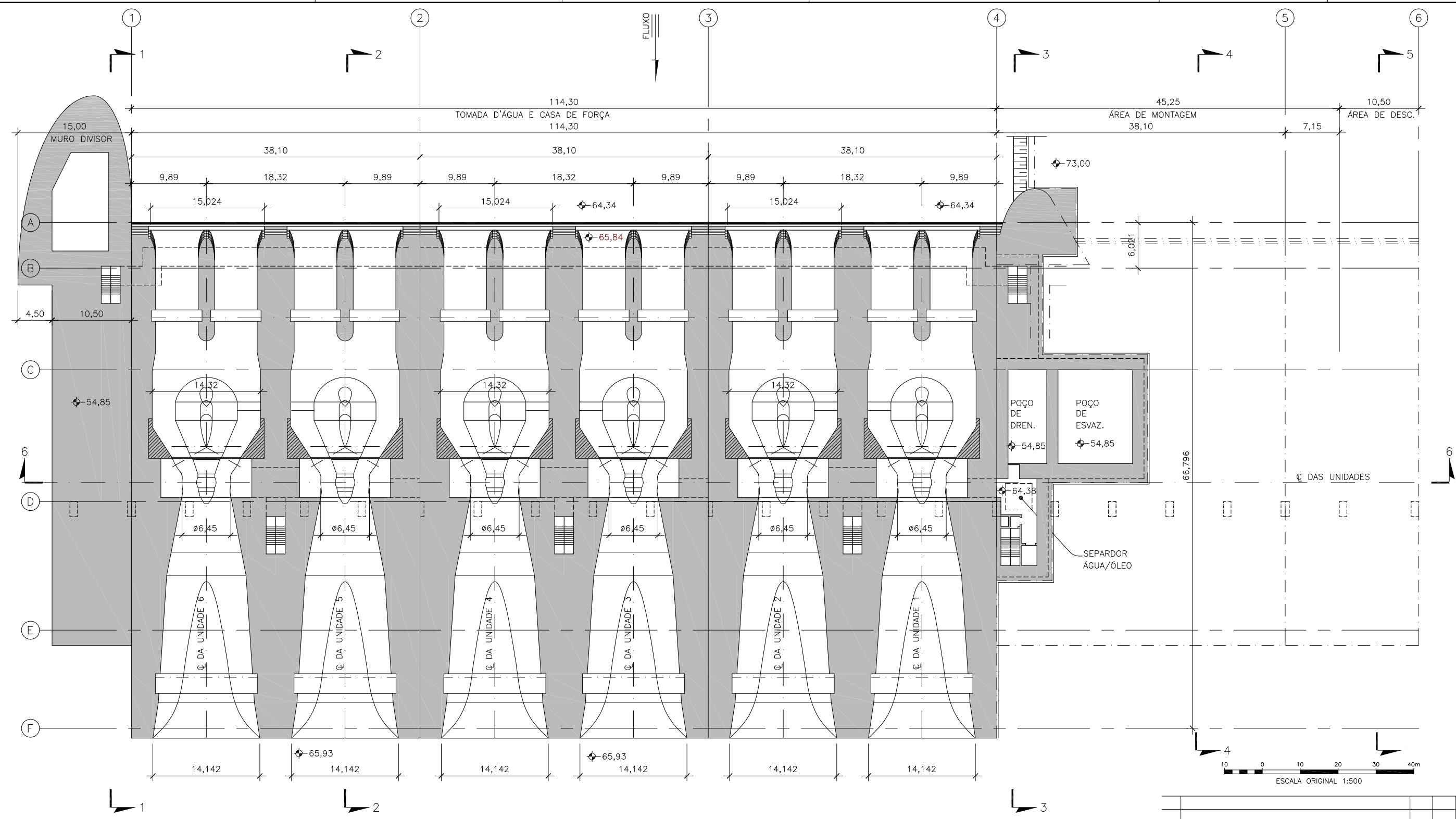
PLANTA A-A
