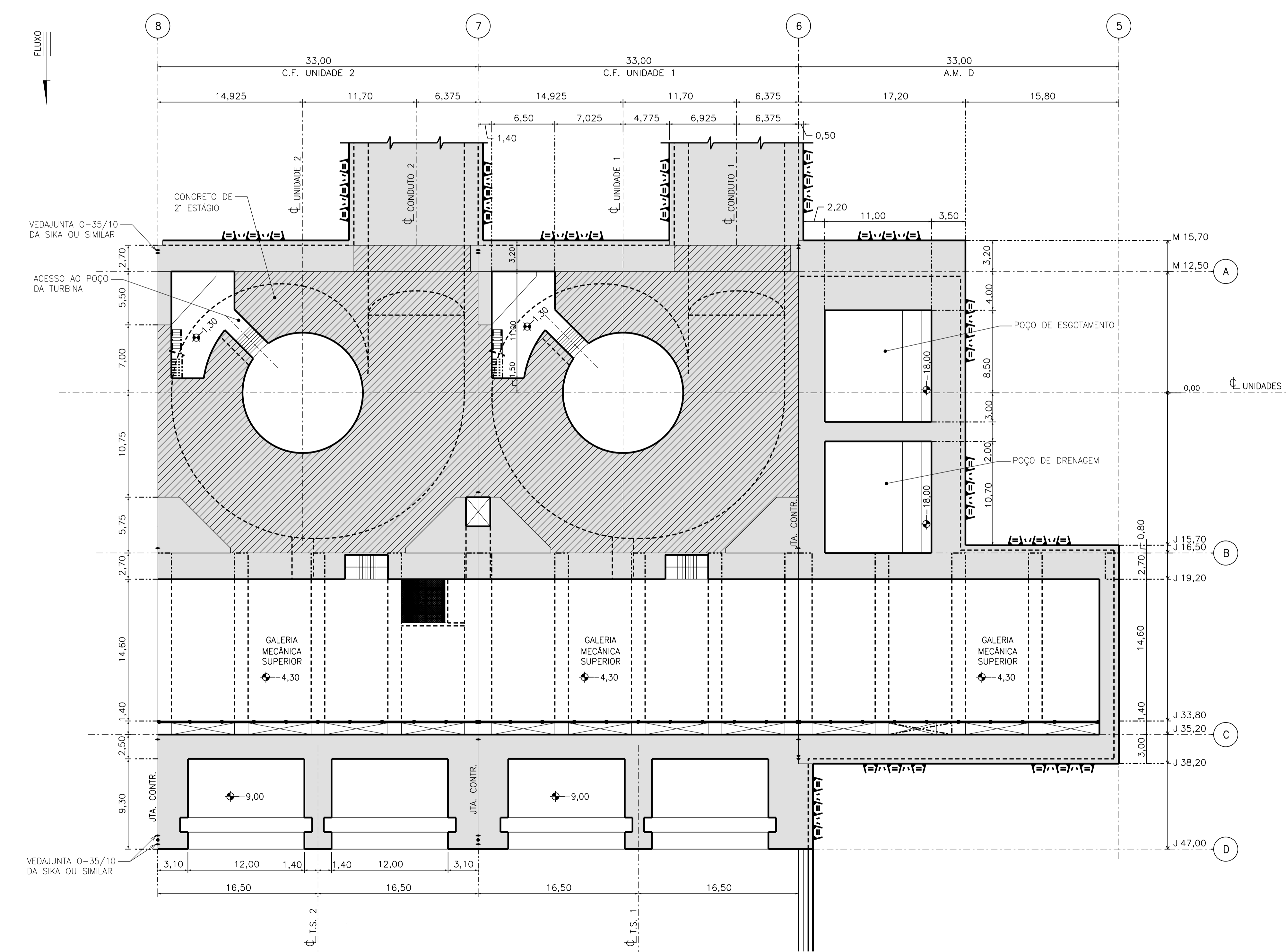
PLANTA NO POÇO DA TURBINA - EL. 1,30
