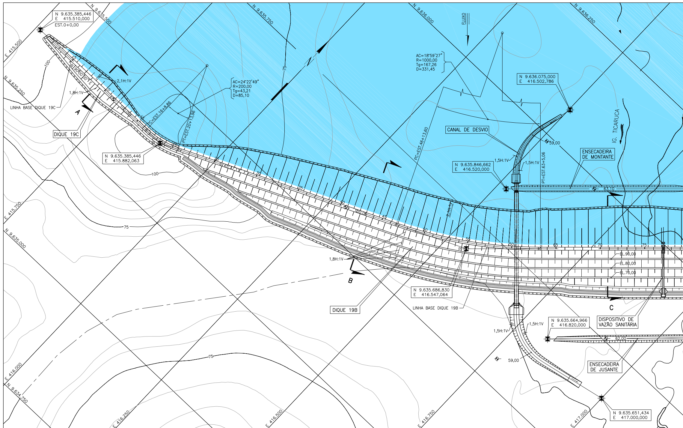
PLANTA
