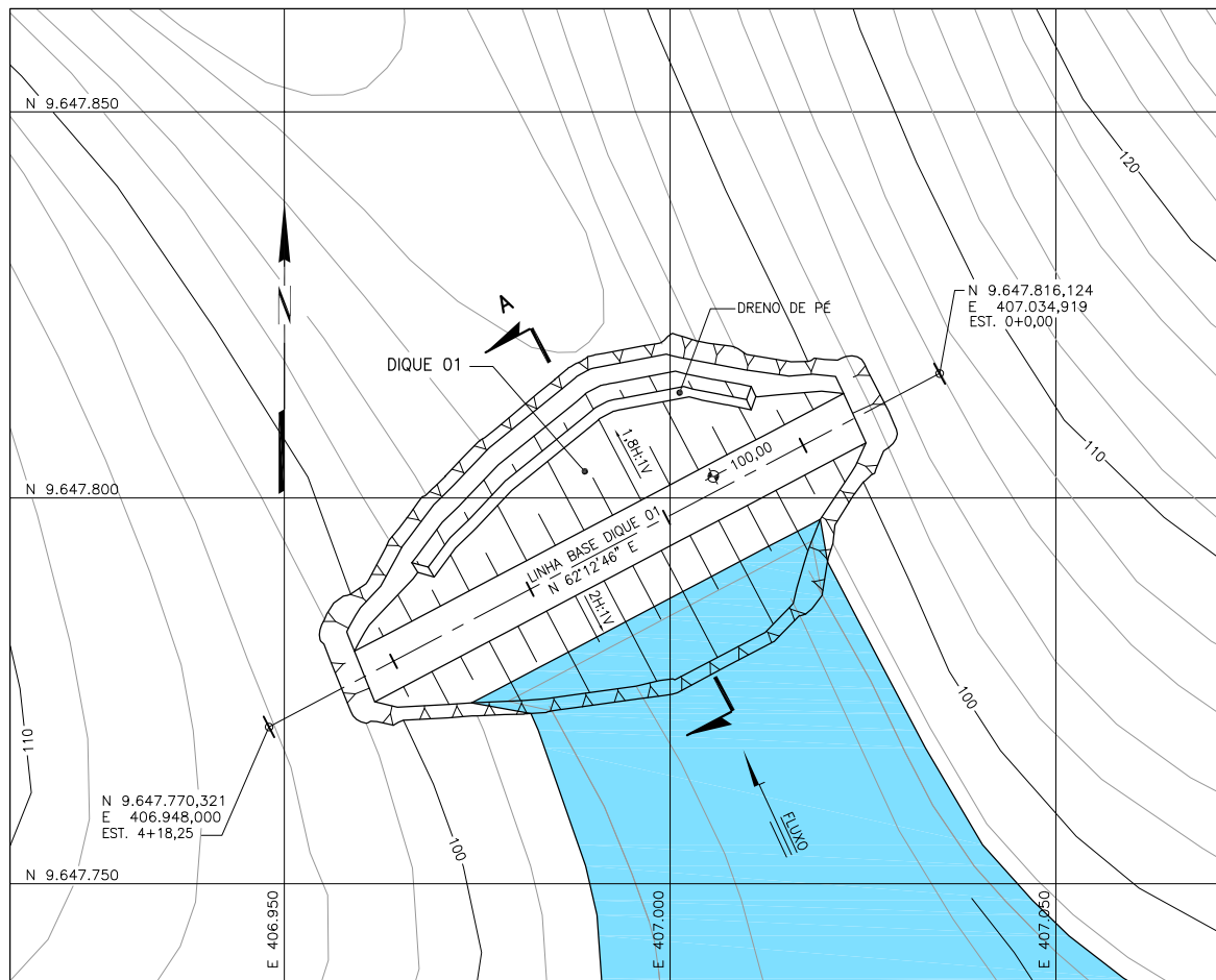
PLANTA
