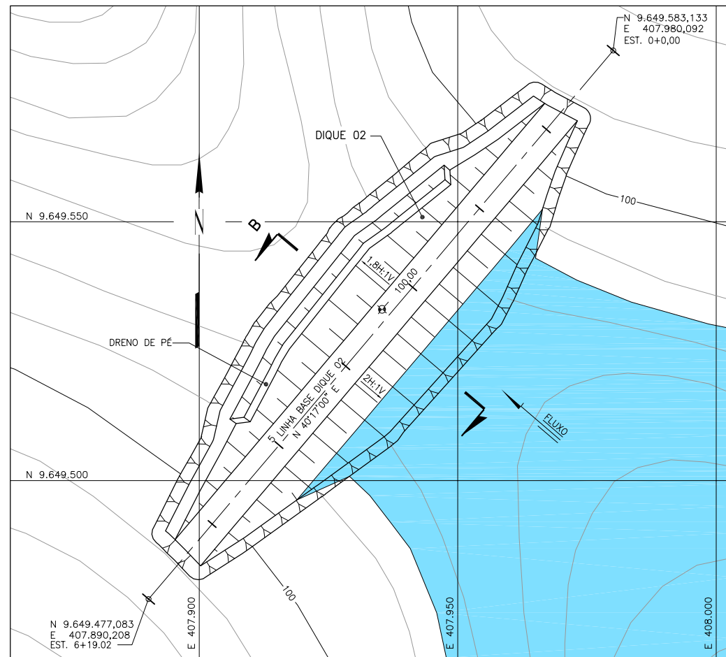
PLANTA
