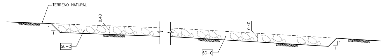
CORTE TÍPICO
