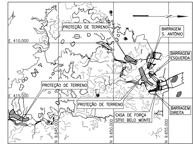
PLANTA CHAVE SEM ESCALA
