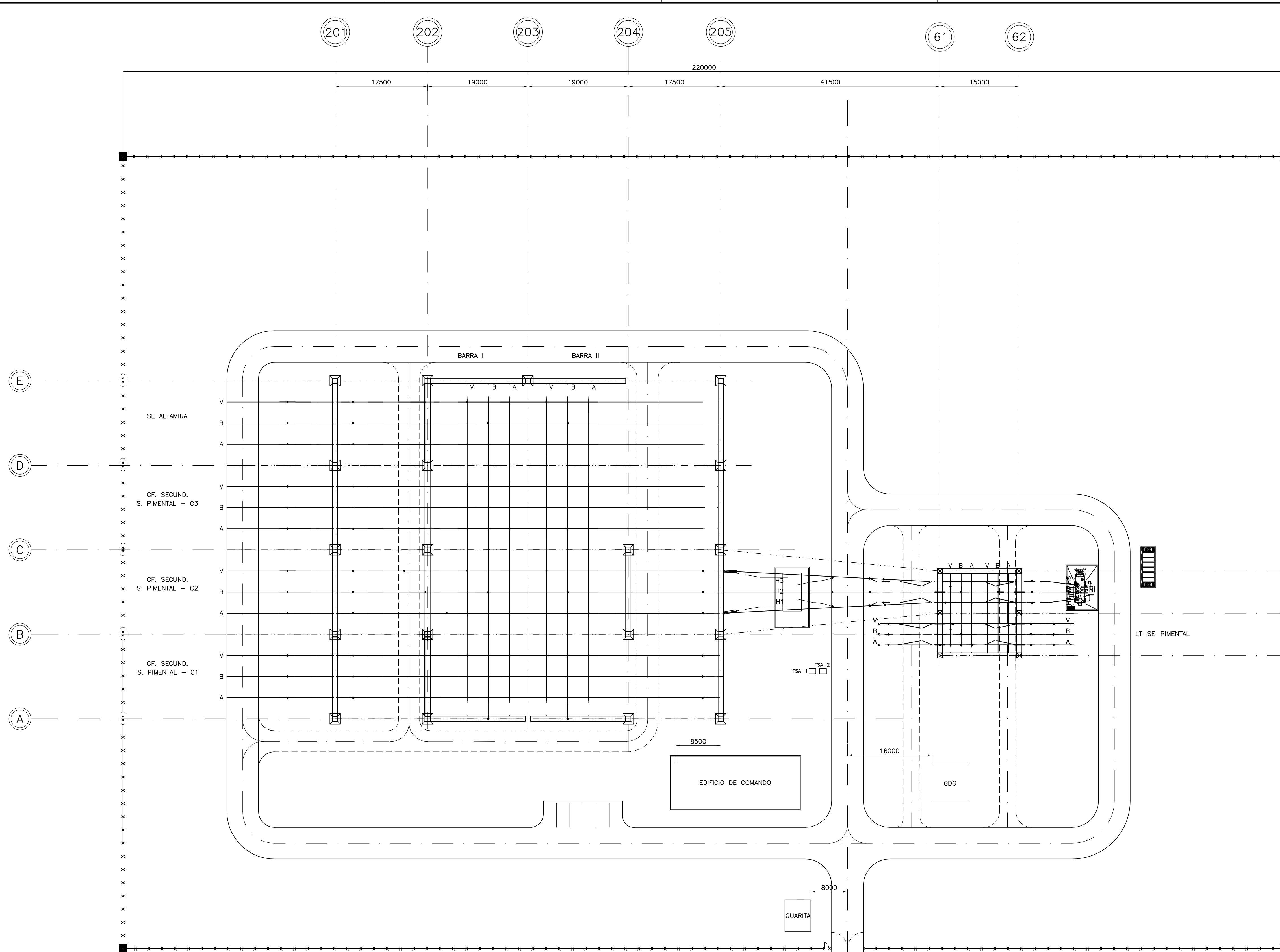
PLANTA ESC. 1:400
