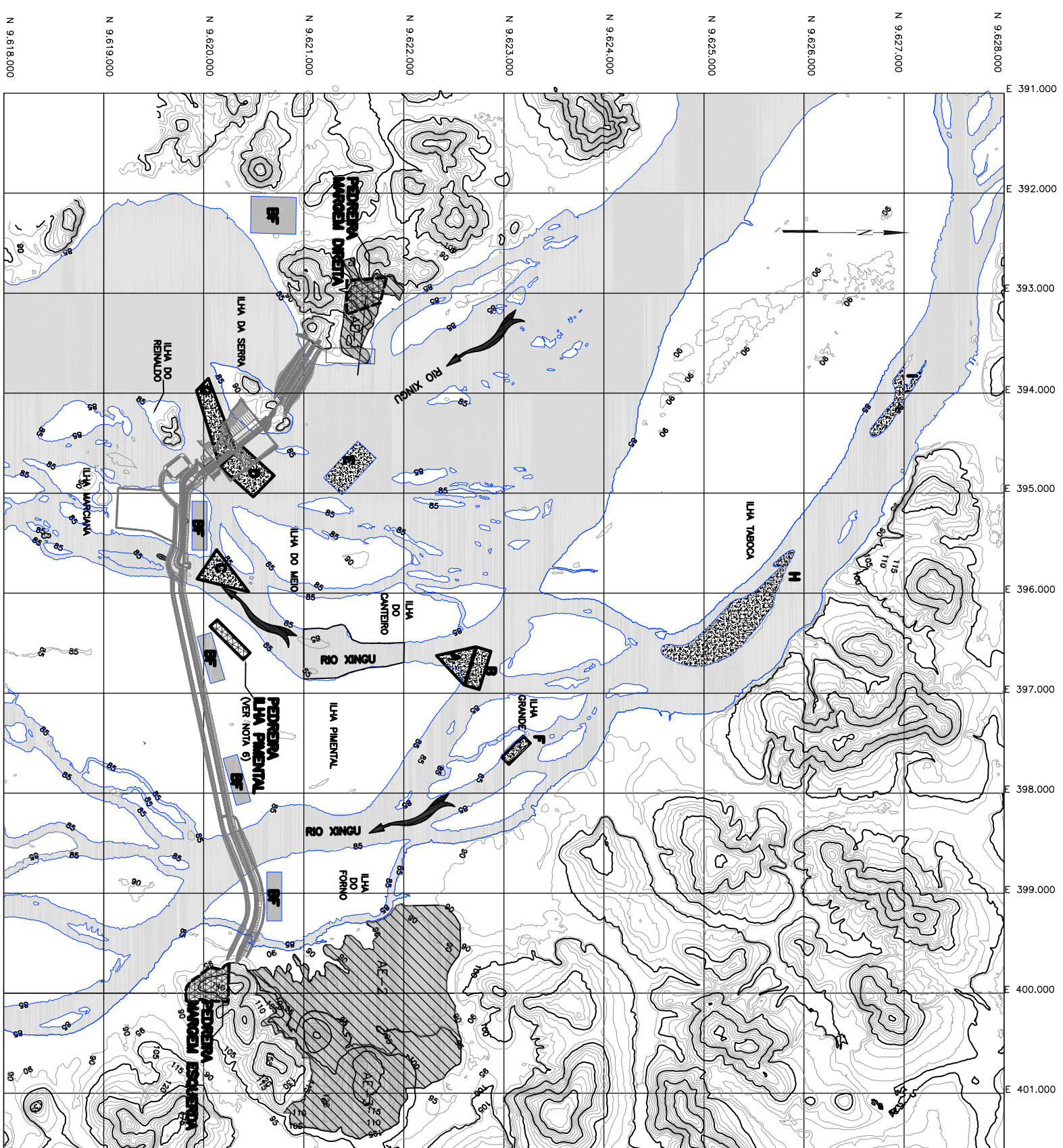
PLANTA ESC:1:1.000
