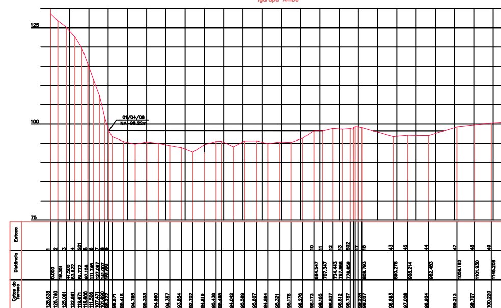
Escala Horizontal 1:5.000 Escala Vertical 1:500
