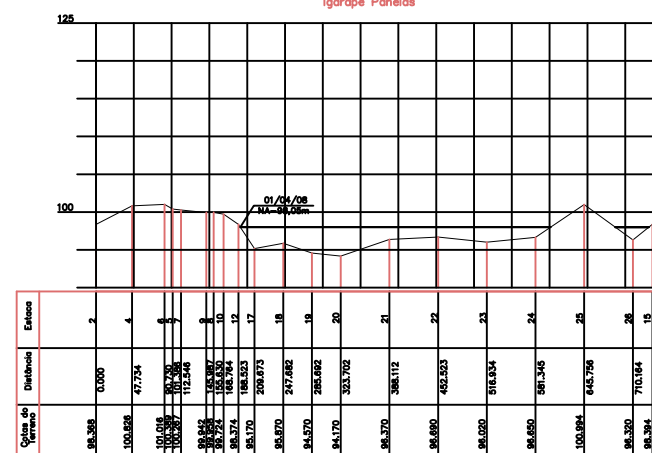
Escala Horizontal 1:5.000 Escala Vertical 1:500
